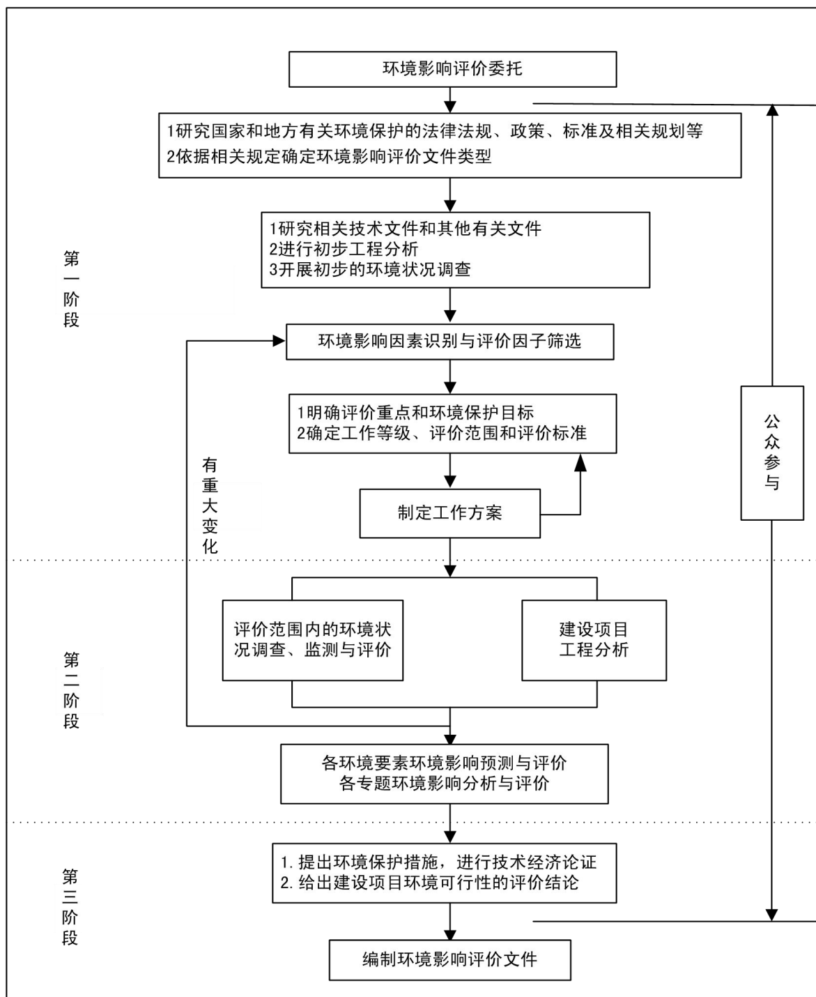
图 1-1 环境影响评价工作流程图
