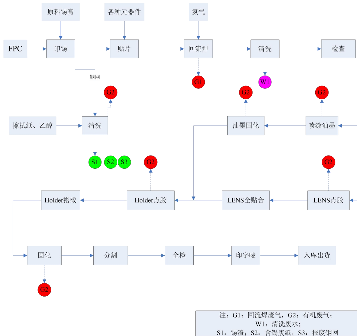
图 4-1 产品生产工艺流程
