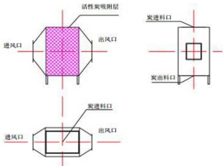
图 9-2 活性炭吸附床示意图
