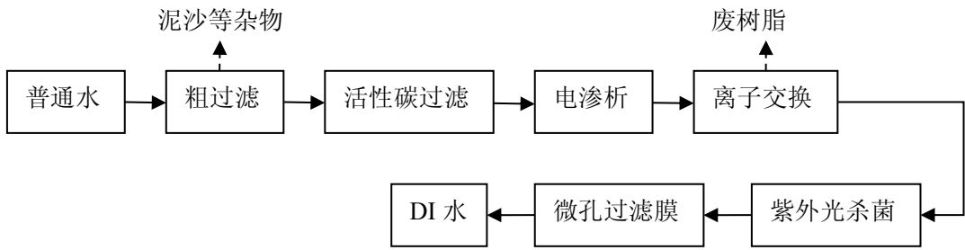
图 4-4 项目纯水制备工艺
