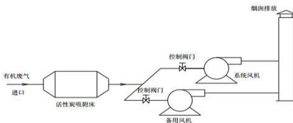
图 9-1 有机废气净化系统流程示意图
