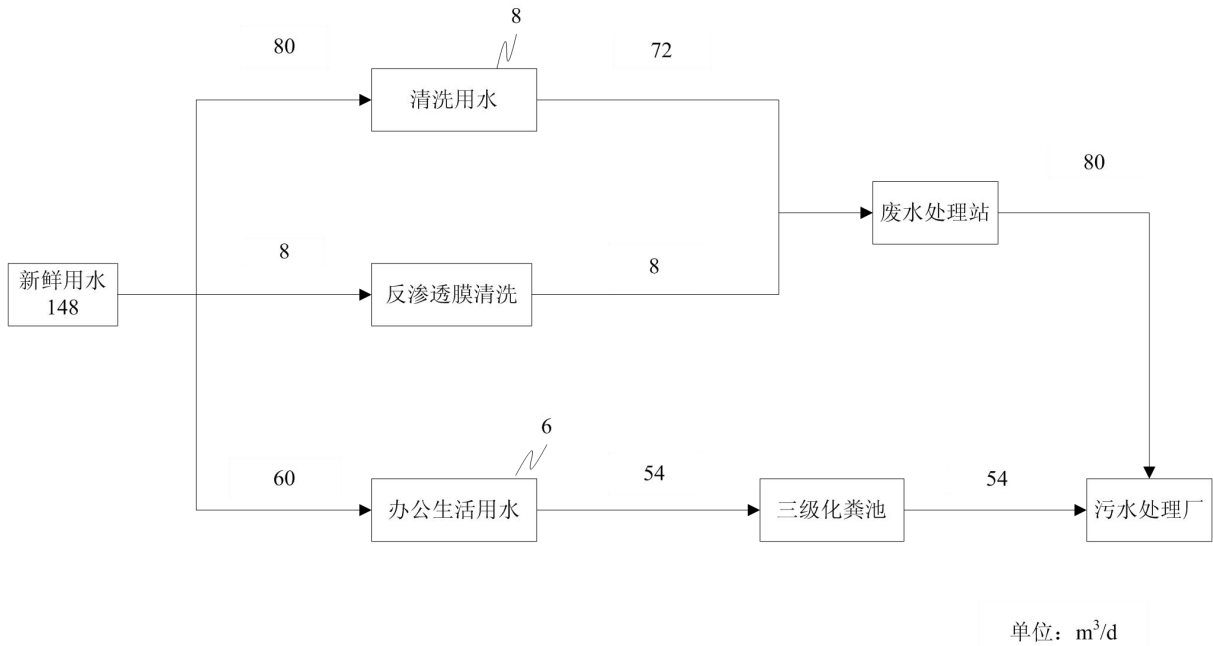
图 4-3 全厂水平衡图
