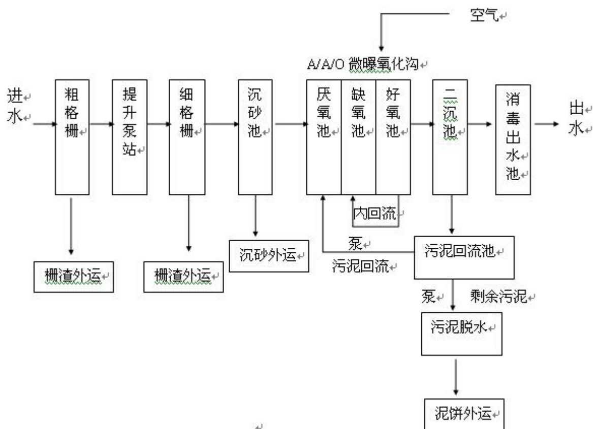
图 9-5 东区污水处理厂处理工艺流程图
