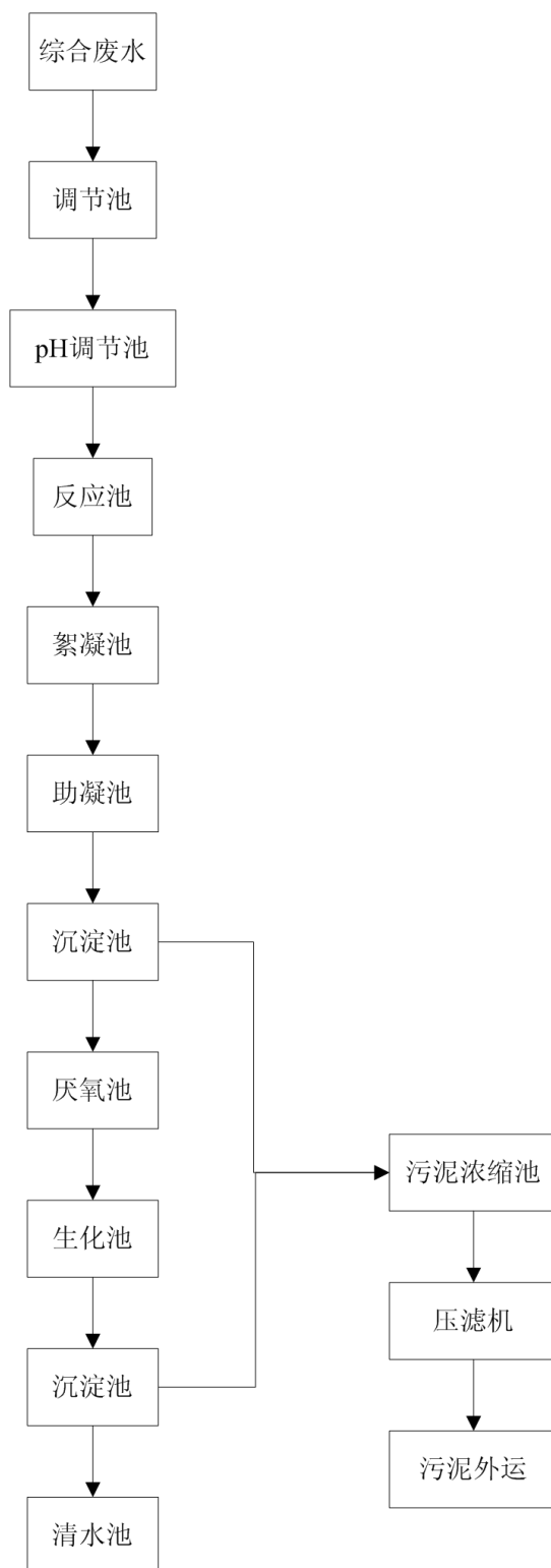
图 9-3 清洗废水处理工艺流程
