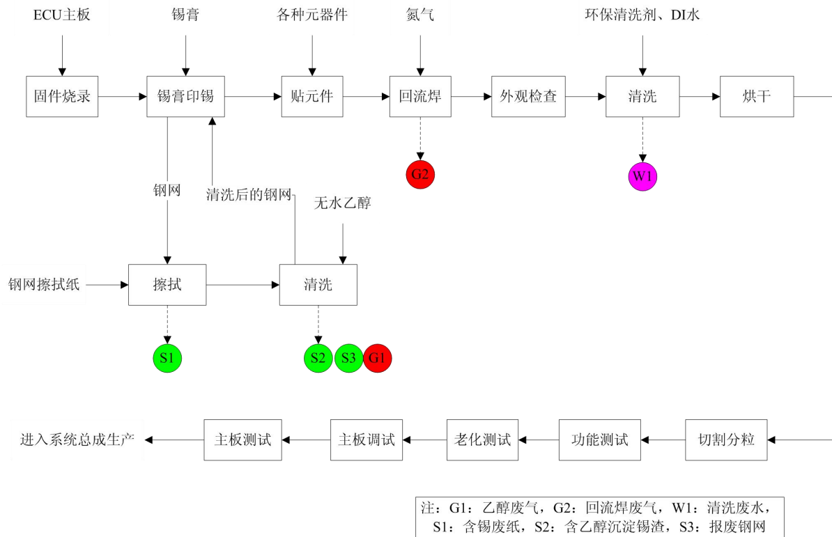
图 4-2 ECU(电子控制单元)主板生产工艺流程
