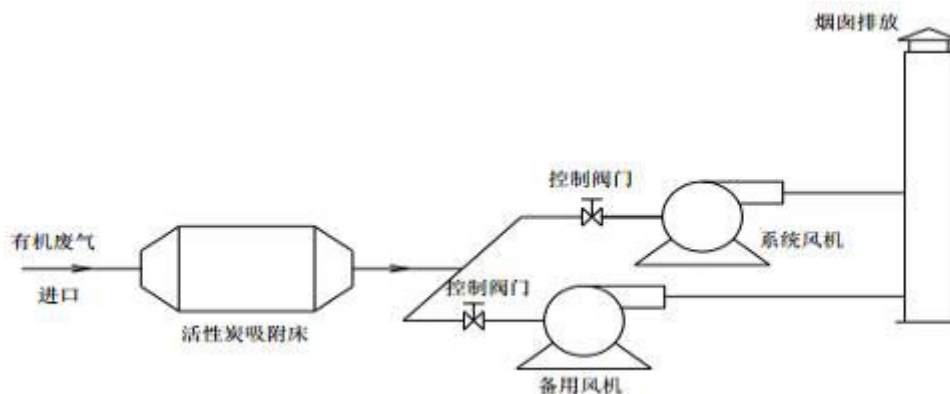
图 10-2 有机废气净化系统流程示意图
