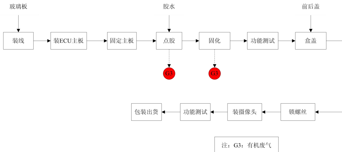
图 4-3 系统总成生产工艺流程
