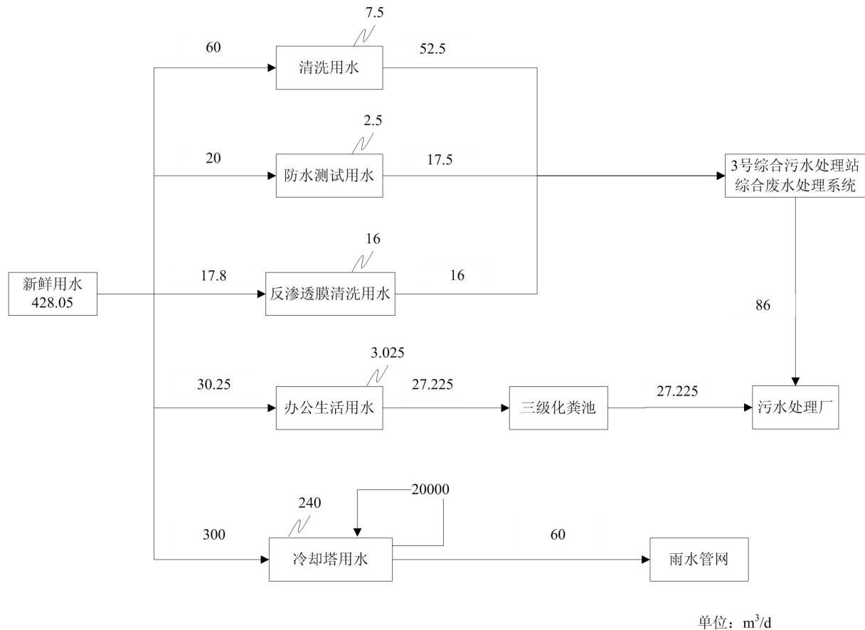
图 4-4 项目车间水平衡图
