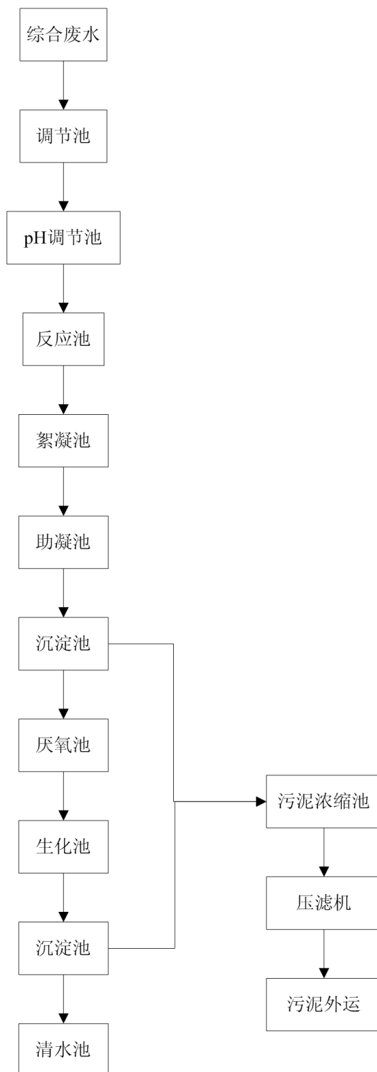
图 10-4 综合生产废水处理工艺流程
