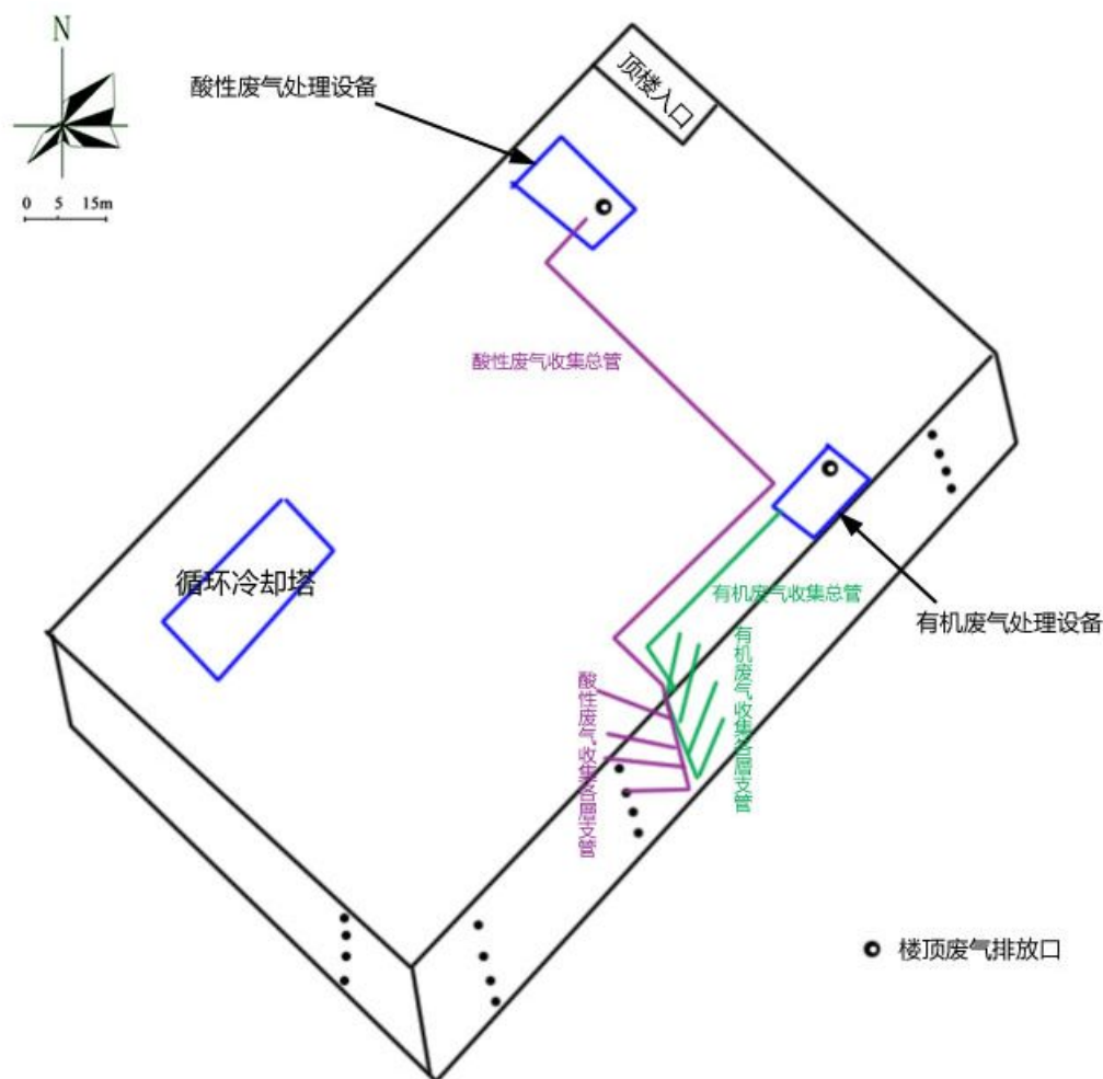
图 10-1 废气分类收集及厂房楼顶平面布置示意图
