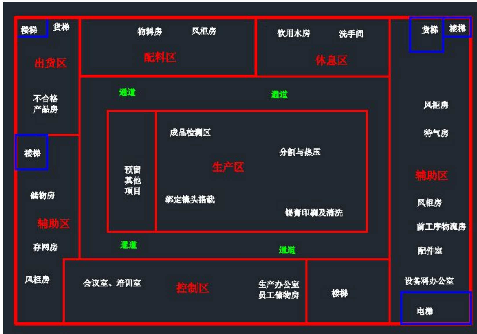
附图 1 项目第四层总平面布置图
