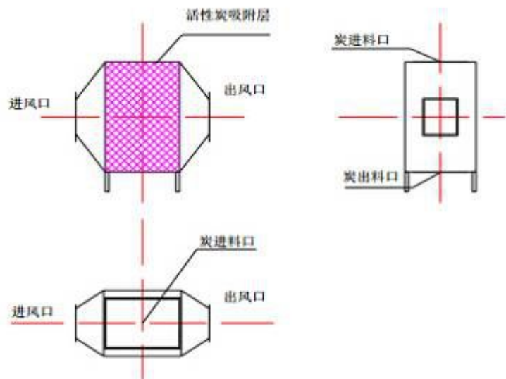
图 10-3 活性炭吸附床示意图
