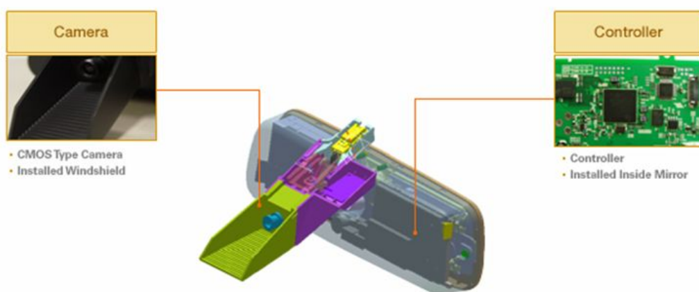
图 3-7 车道偏离报警系统
