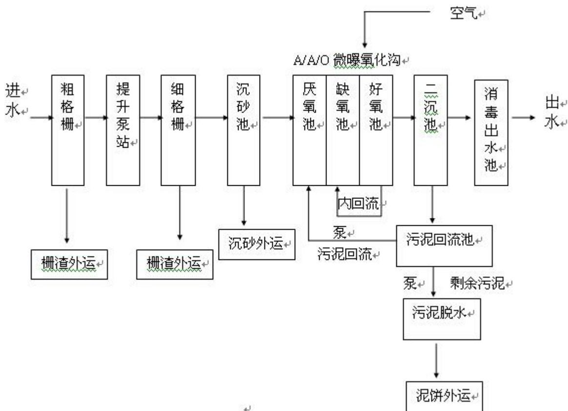
图 10-7 东区污水处理厂处理工艺流程图
