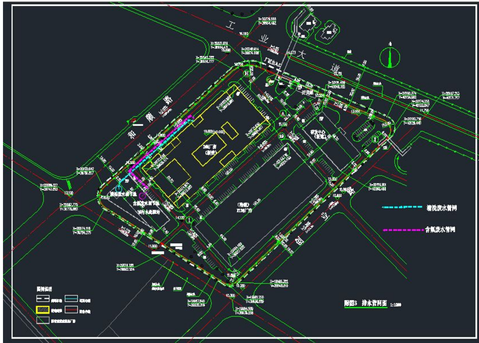
附图 4 排水管网图
