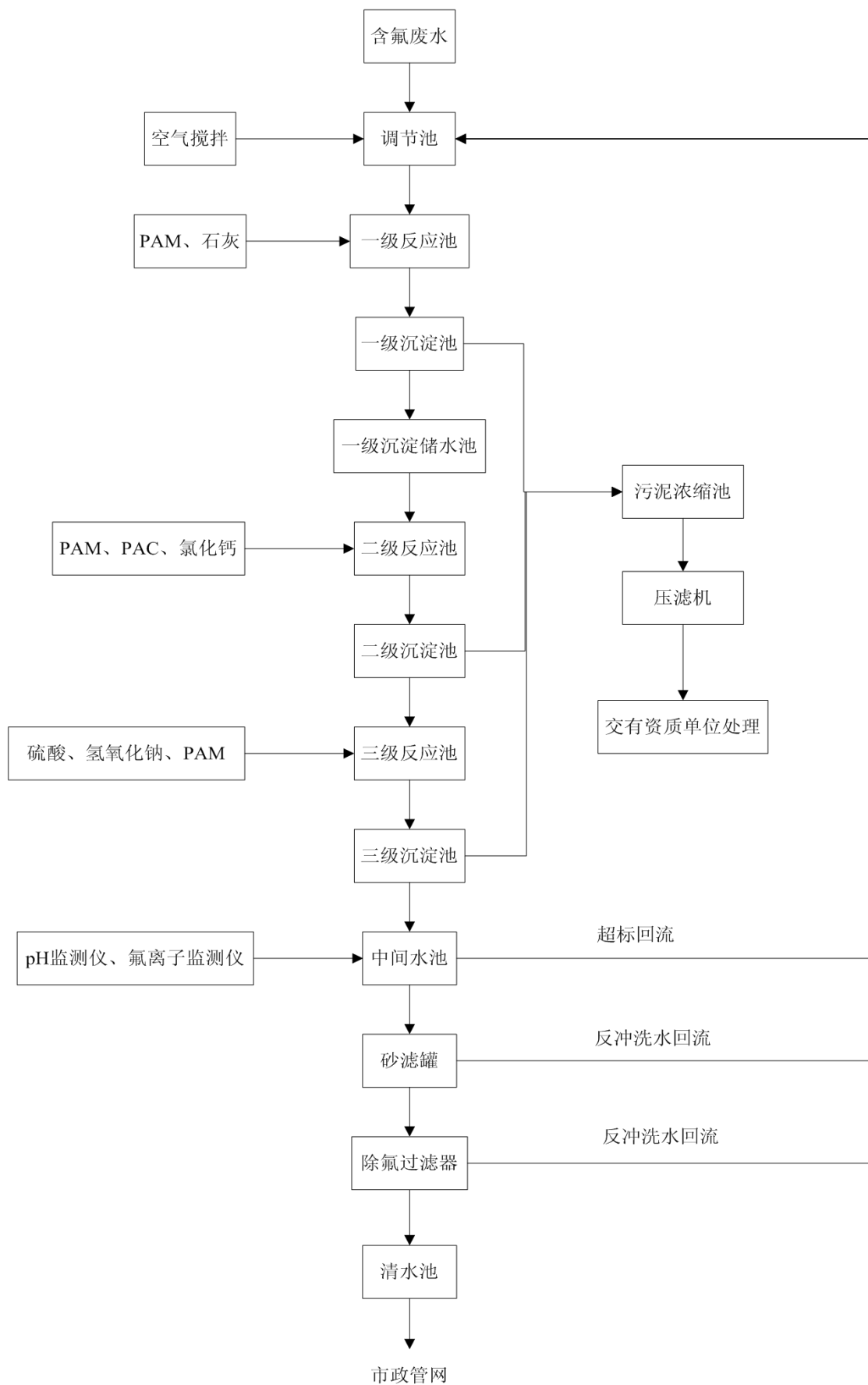
图 10-5 含氟废水处理工艺流程
