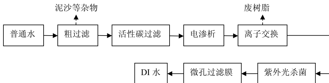
图 4-5 项目纯水制备工艺
