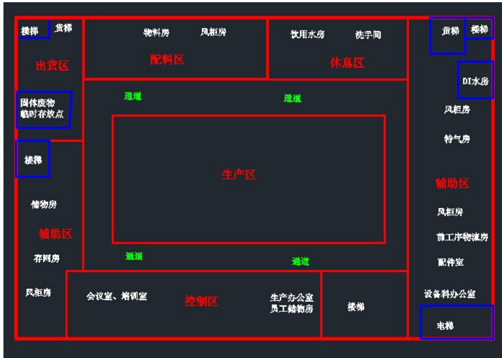
附图2 26号厂房第一层平面布置图
