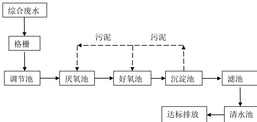
项目污水处理工艺流程图
