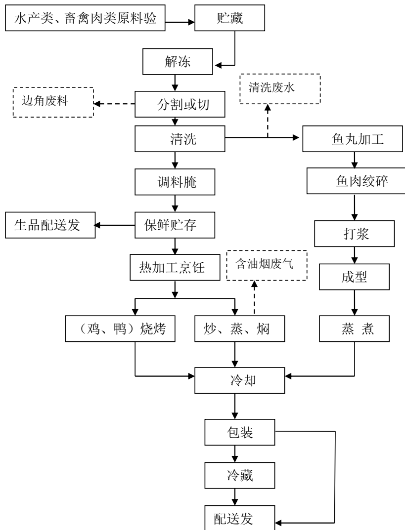
(3) 烹饪热加工类生产工艺流程图:
