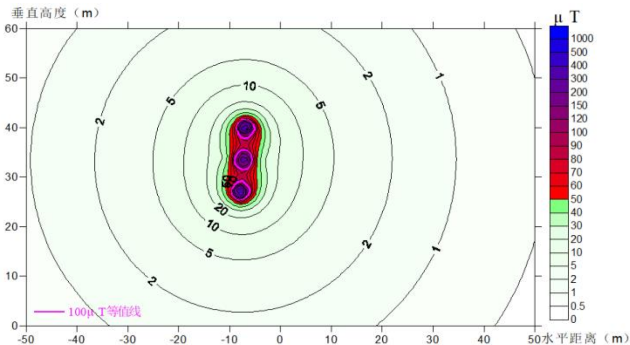
ZT1-图 8.2-7 梅深站至川平站线路（A 线）工频磁感应强度预测结果等值线图
