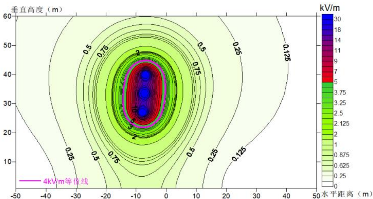
ZT1-图 8.2-6 梅深站至川平站线路 (A 线) 工频电场强度预测结果等值线图
