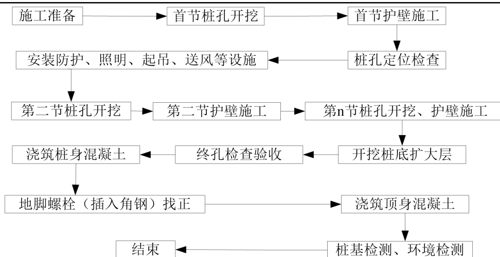
图 2-4 人工挖孔桩基础工艺流程
