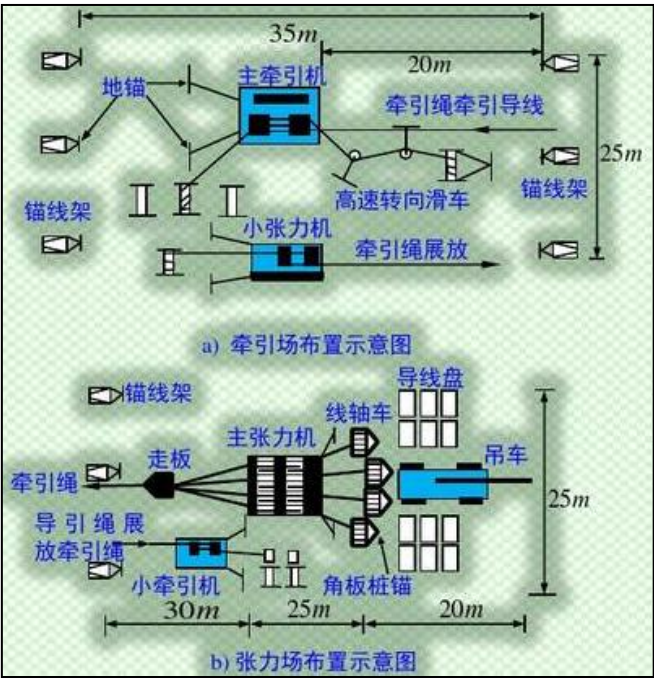
图 2-5 牵张场的布置示意图
