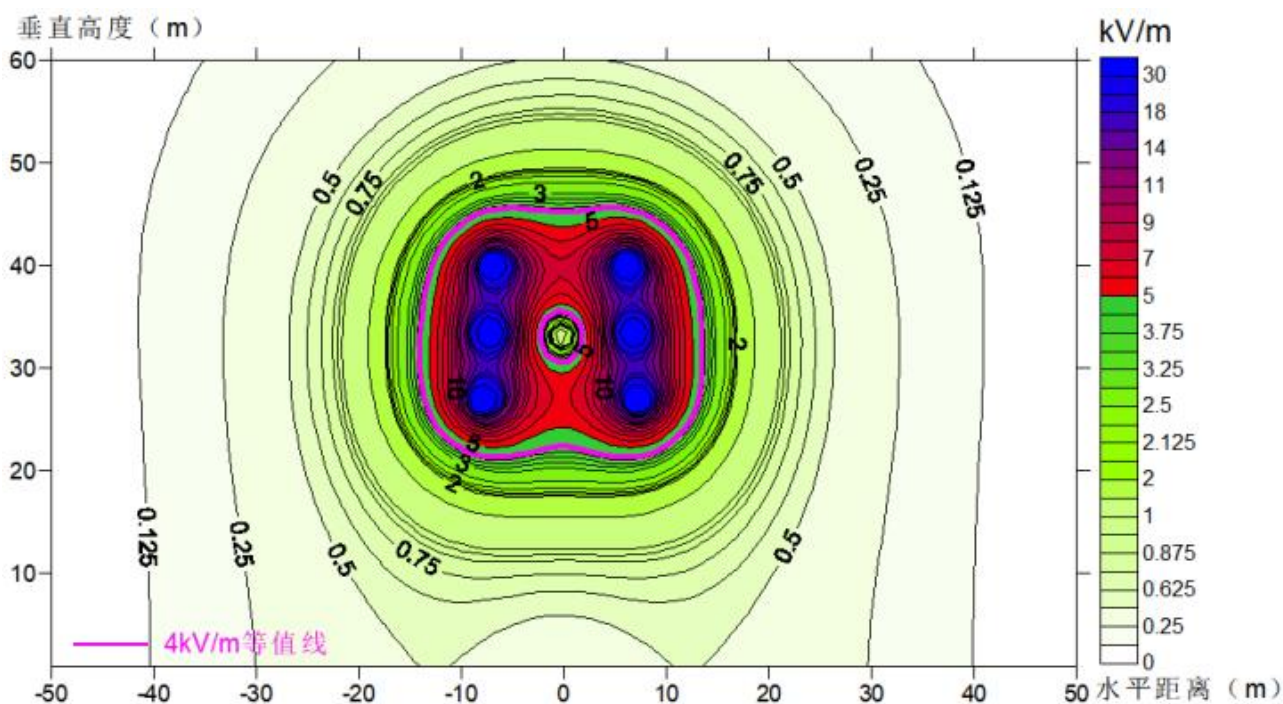
ZT1-图 8.2-18 调整虎地站外 220kV 线路（D 线）工频电场强度预测结果等值线图
