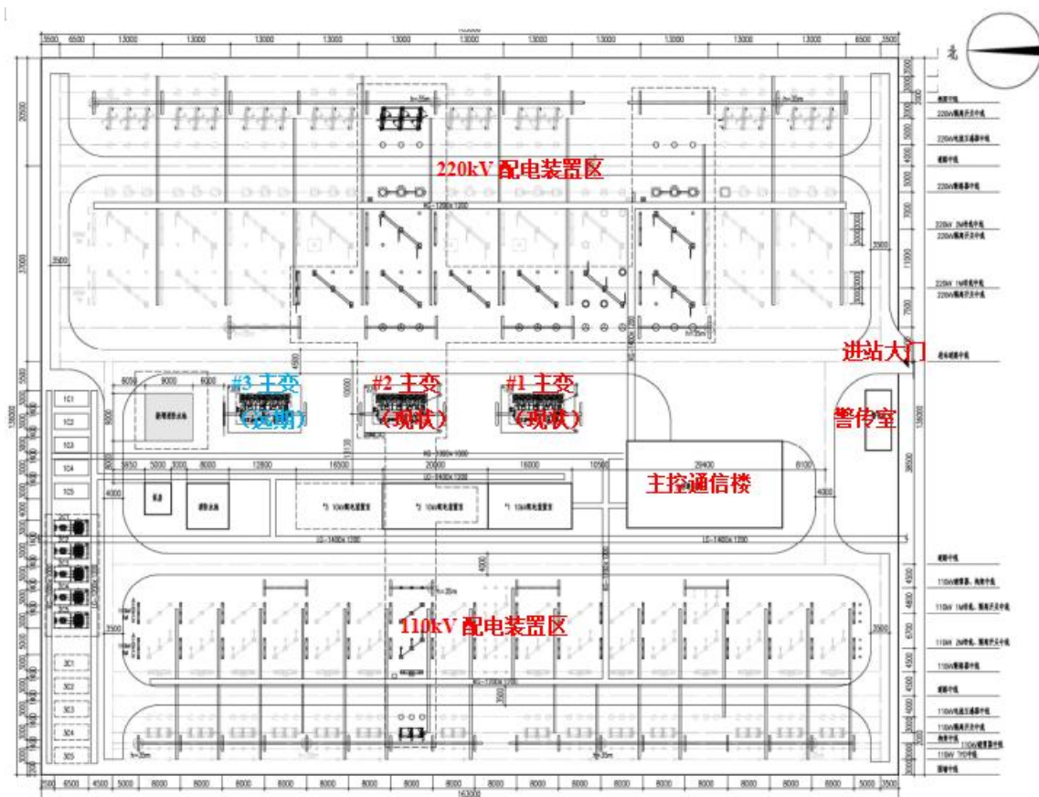
220 千伏虎地站总平面布置示意图
