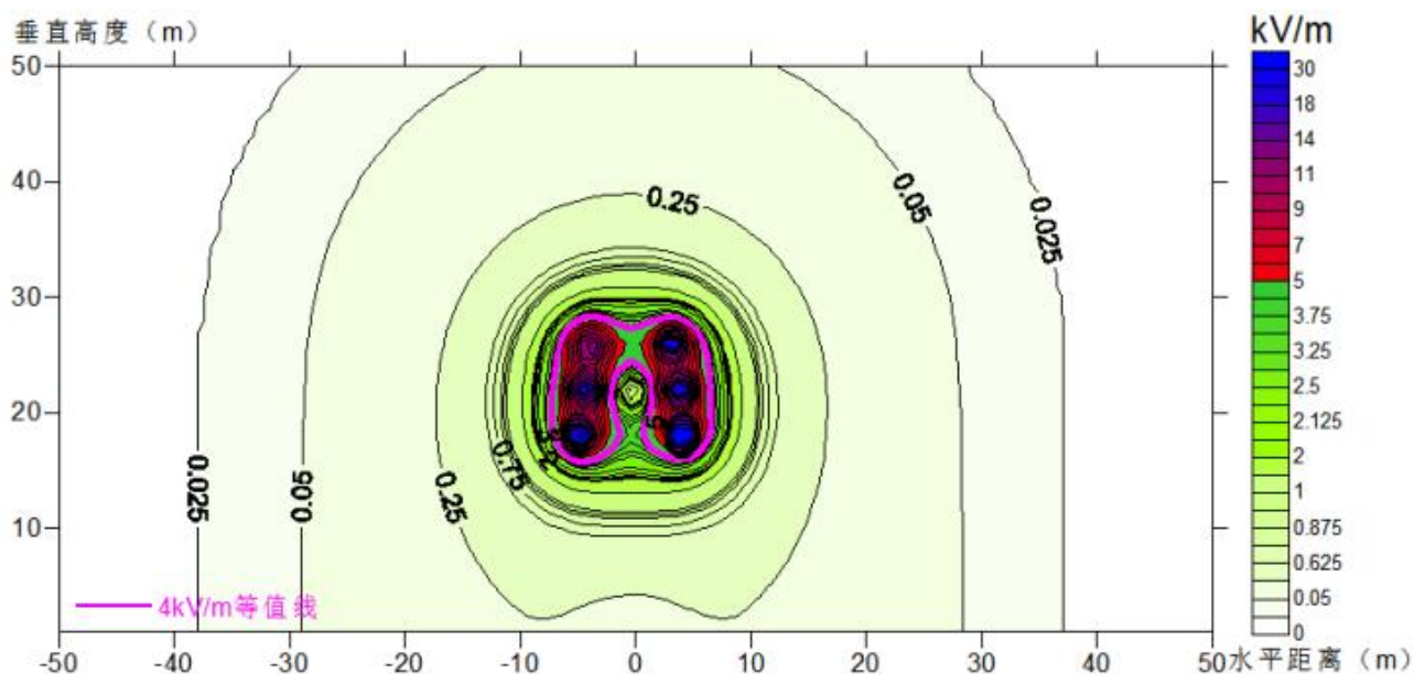
ZT1-图 8.2-22 本项目 110kV 同塔双回线路工频电场强度预测结果等值线图
