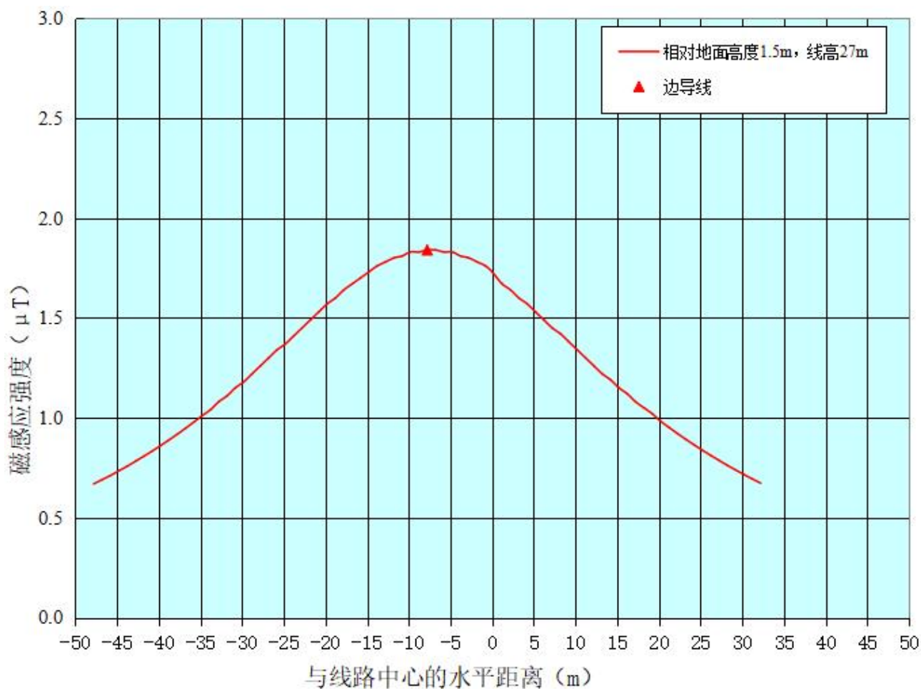
ZT1-图 8.2-5 梅深站至川平站线路 (A 线) 工频磁感应强度预测结果衰减趋势线图
