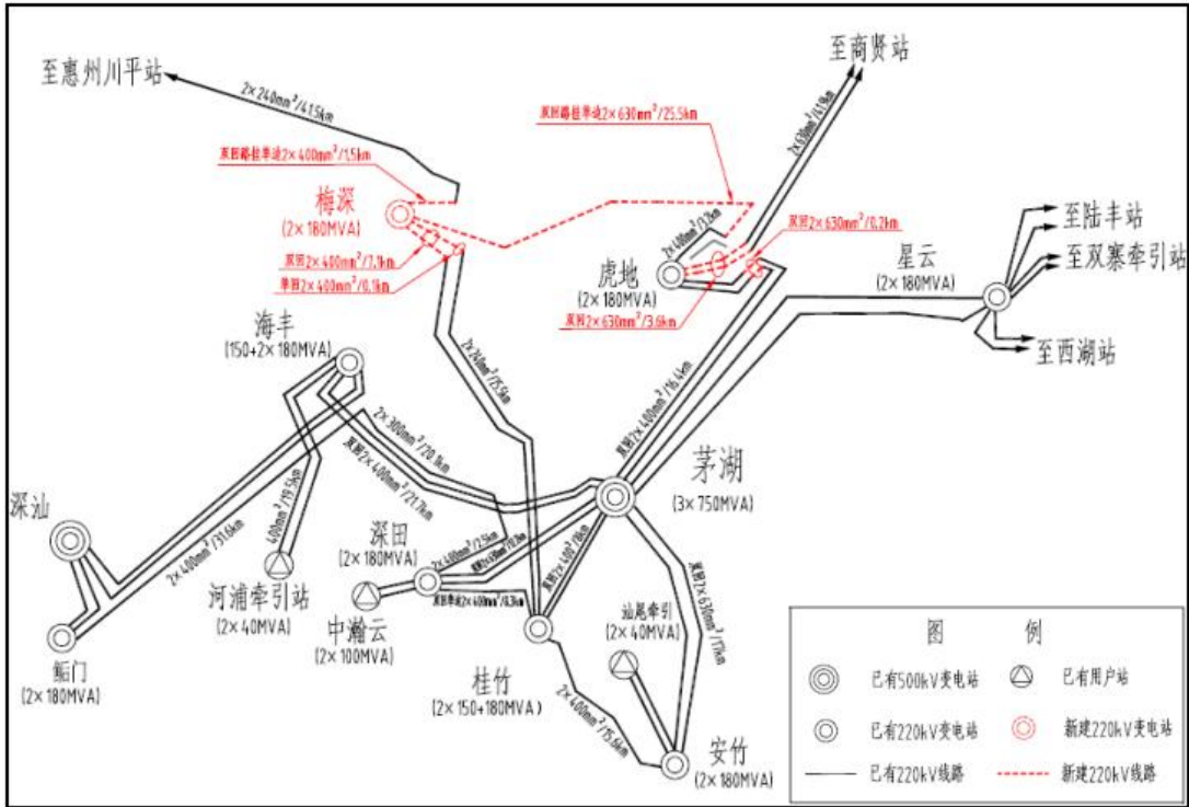
图 2-1 本工程 220kV 线路接入系统示意图
