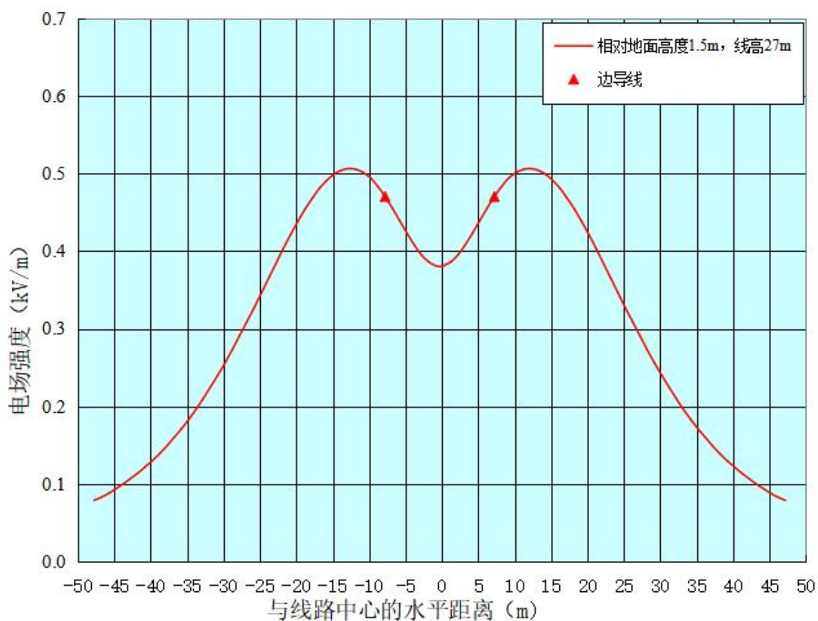
ZT1-图 8.2-16 调整虎地站外 220kV 线路 (D 线) 工频电场强度预测结果衰减趋势线图
