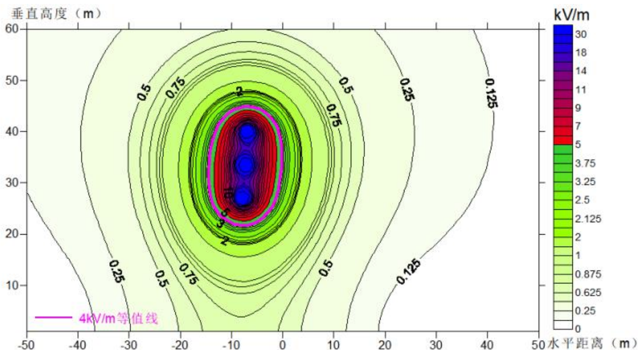
ZT1-图 8.2-10 梅深站至虎地站线路（B 线）工频电场强度预测结果等值线图
