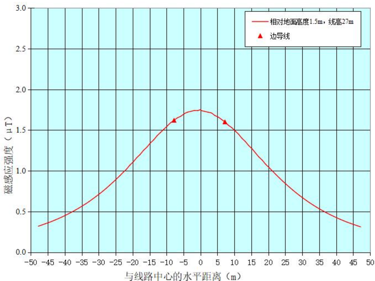
ZT1-图 8.2-13 梅深站至桂竹站线路 (C 线) 工频磁感应强度预测结果衰减趋势线图
