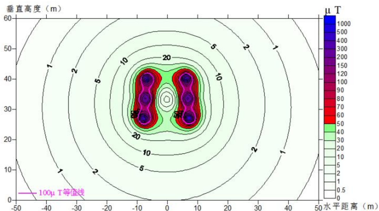
ZT1-图 8.2-19 调整虎地站外 220kV 线路（D 线）工频磁感应强度预测结果等值线图
