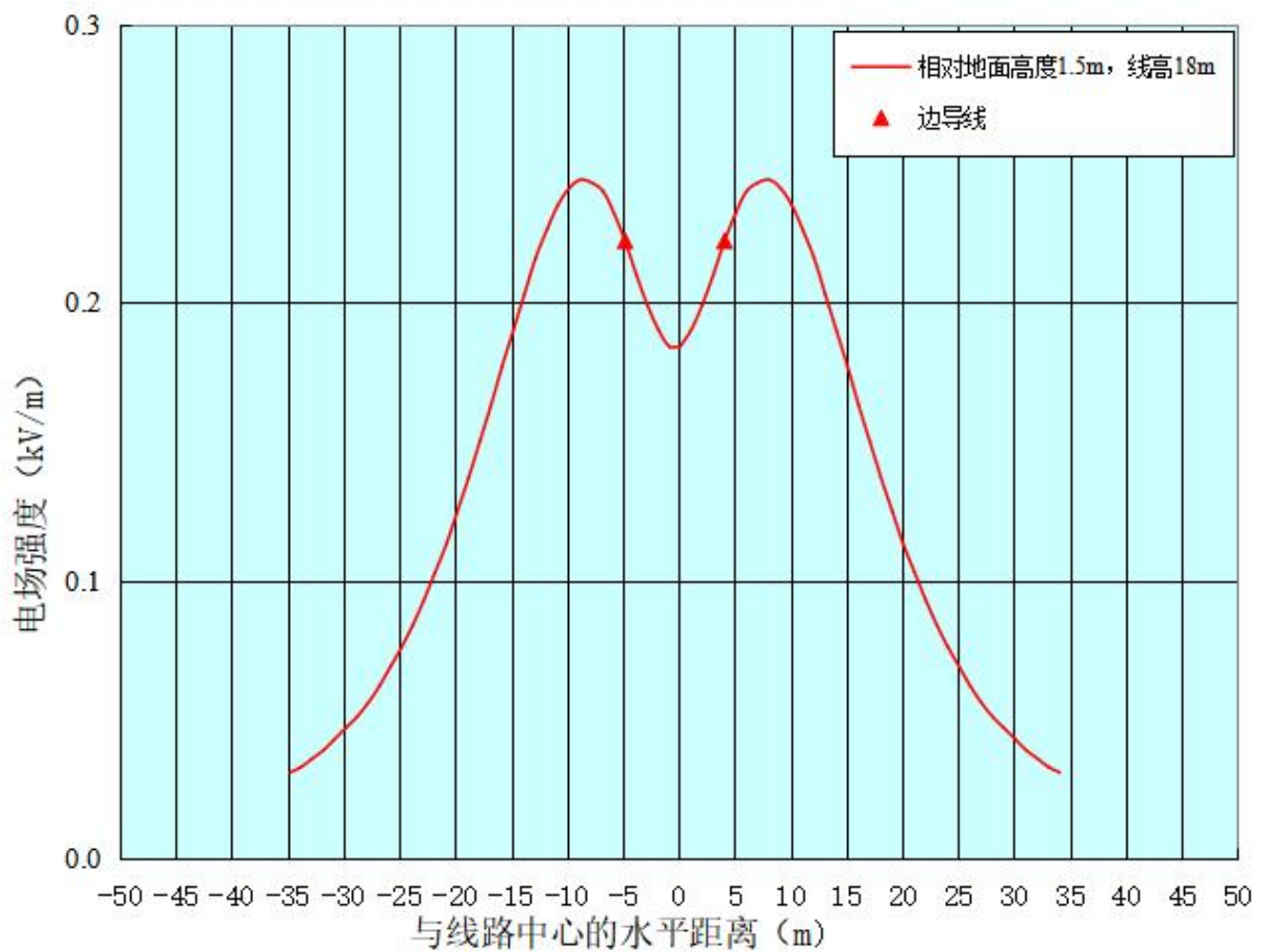
ZT1-图 8.2-20 本项目 110kV 同塔双回线路工频电场强度预测结果衰减趋势线图
