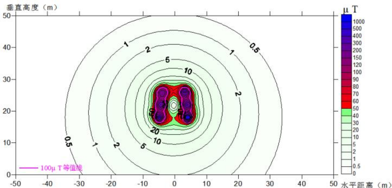
ZT1-图8.2-23 本项目110kV同塔双回线路工频磁感应强度预测结果等值线图
