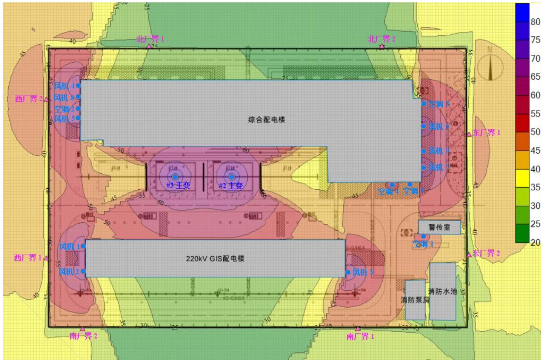
图 4-2 变电站运行期间噪声贡献值等值线图（单位：dB(A)）
