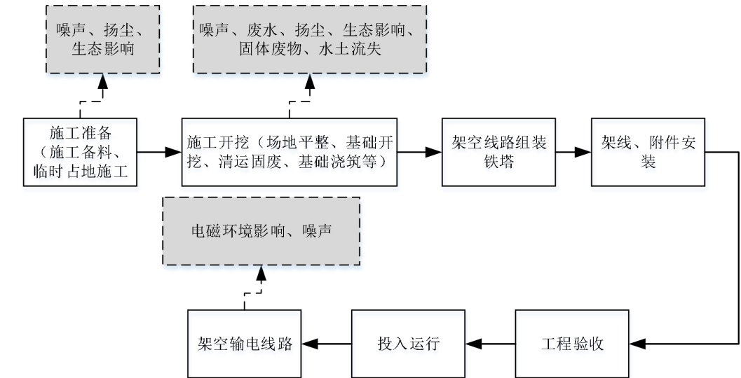
图 2-7 架空线路施工时序及产污环节图
