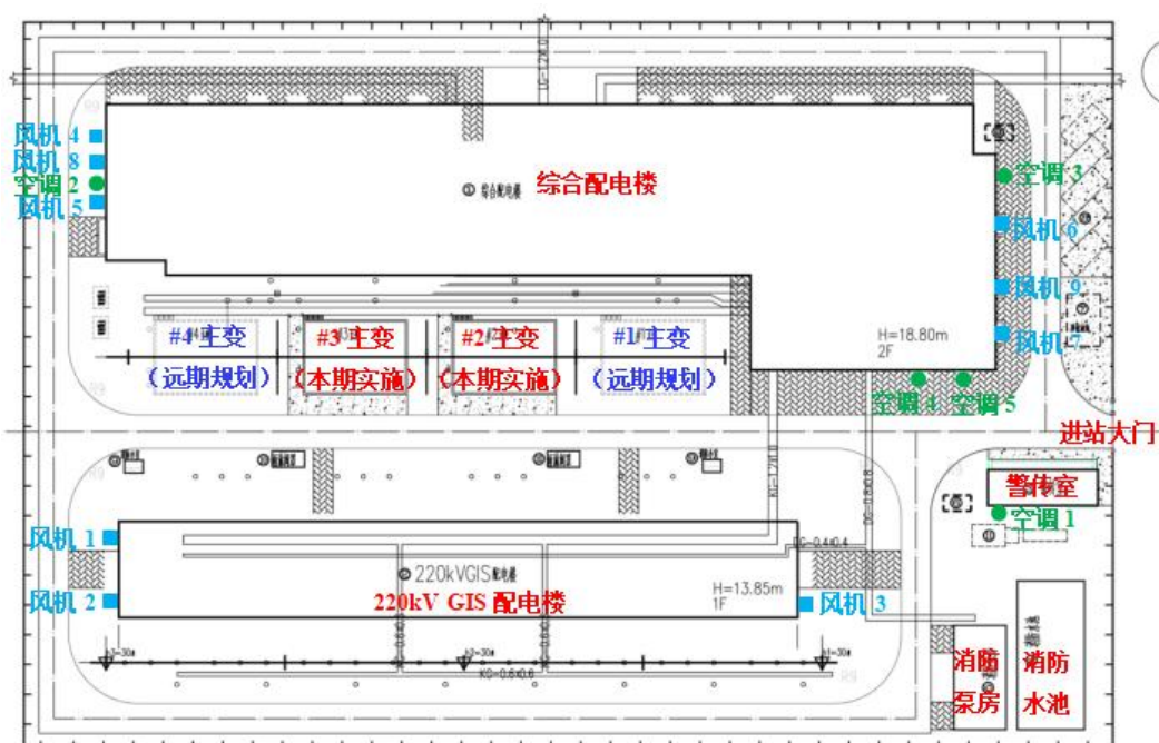
图 4-1 梅深变电站本期声源布局示意图
