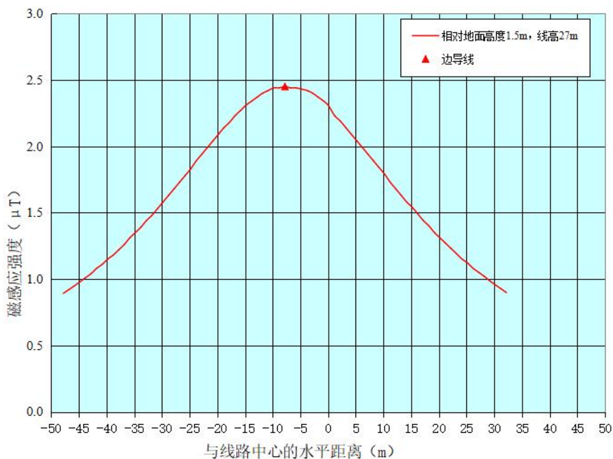
ZT1-图 8.2-9 梅深站至虎地站线路 (B 线) 工频磁感应强度预测结果衰减趋势线图
