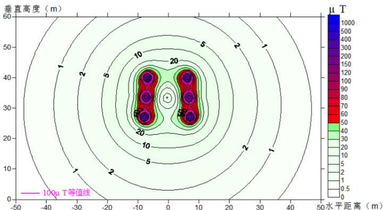
ZT1-图 8.2-15 梅深站至桂竹站线路（C 线）工频磁感应强度预测结果等值线图
