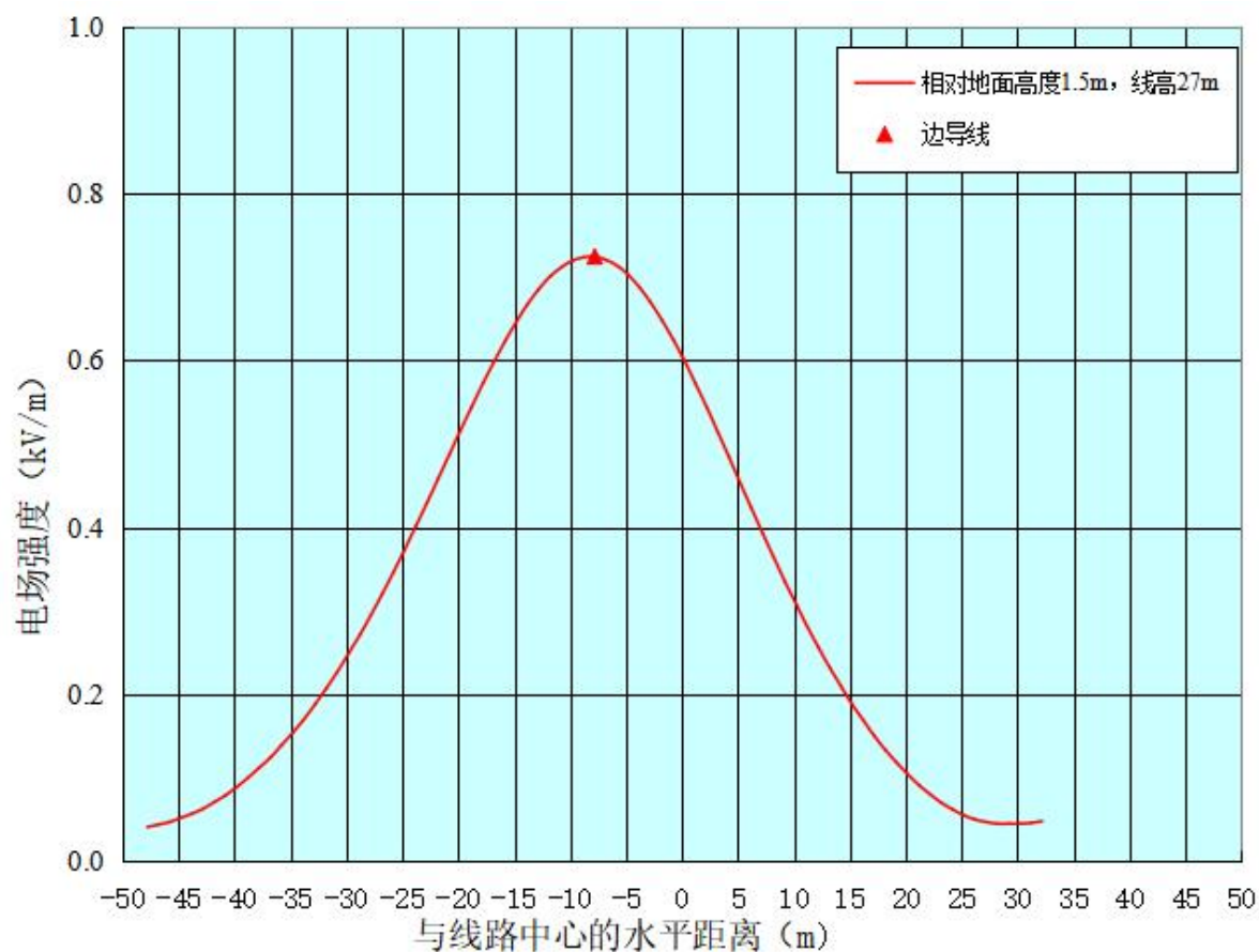
ZT1-ZT1-图 8.2-8 梅深站至虎地站线路 (B 线) 工频电场强度预测结果衰减趋势线图
