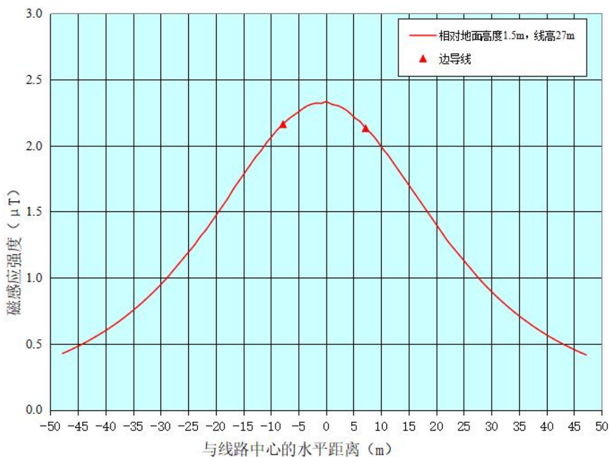
ZT1-图 8.2-17 调整虎地站外 220kV 线路 (D 线) 工频磁感应强度预测结果衰减趋势线图
