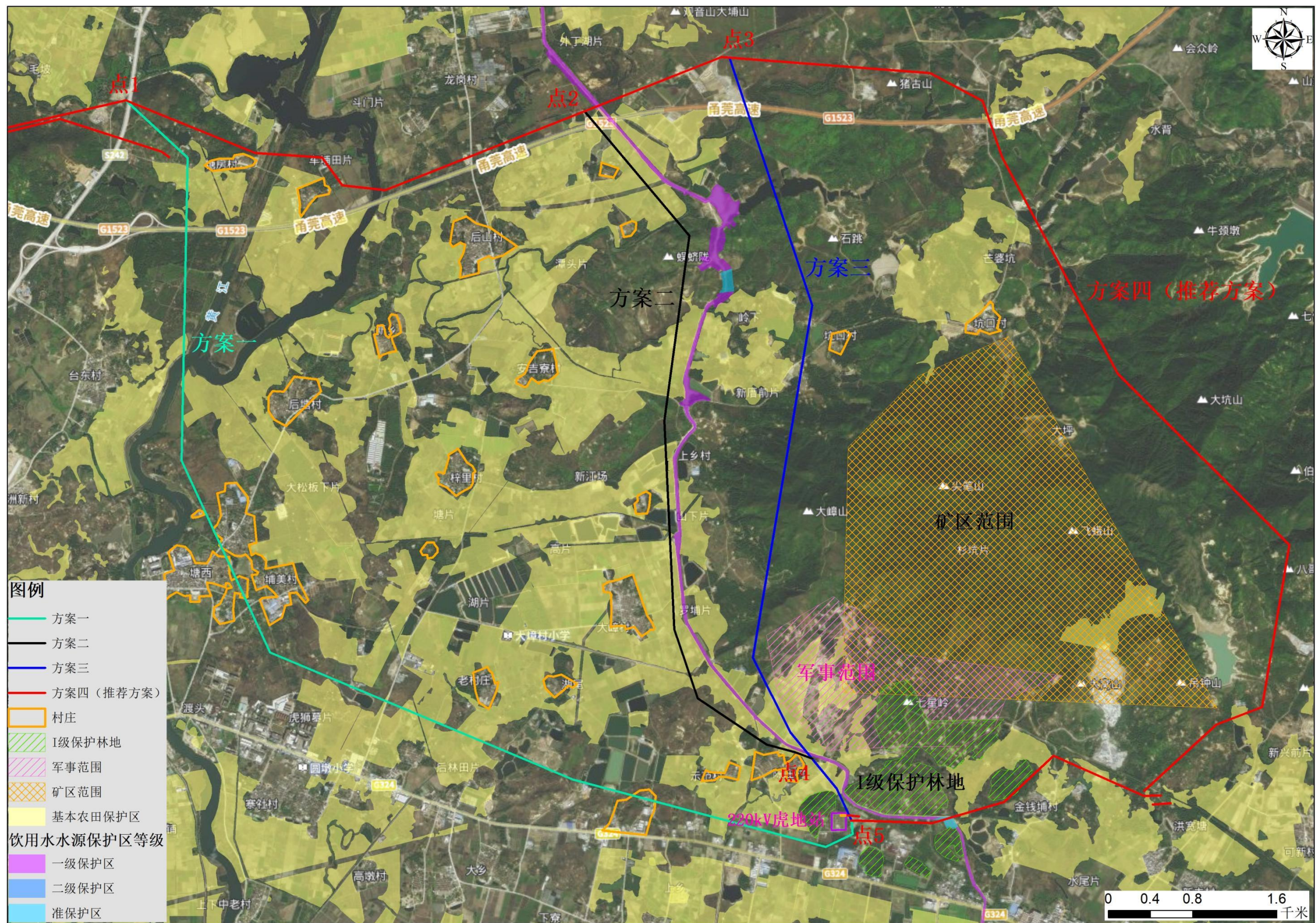
ZT2-图 7.1-1 项目线路工程跨越公平灌渠-赤沙水库饮用水水源保护区的路径比选方案示意图
