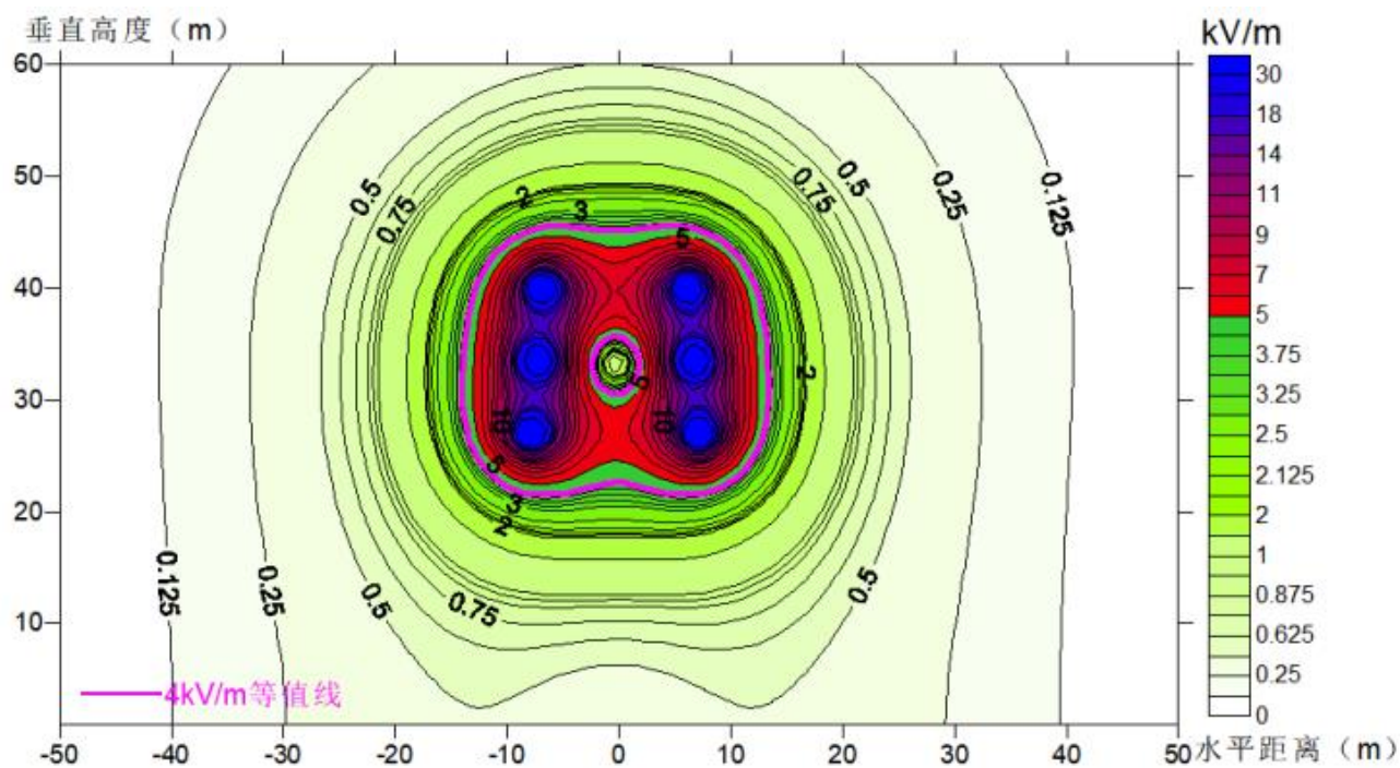
ZT1-图 8.2-14 梅深站至桂竹站线路 (C 线) 工频电场强度预测结果等值线图
