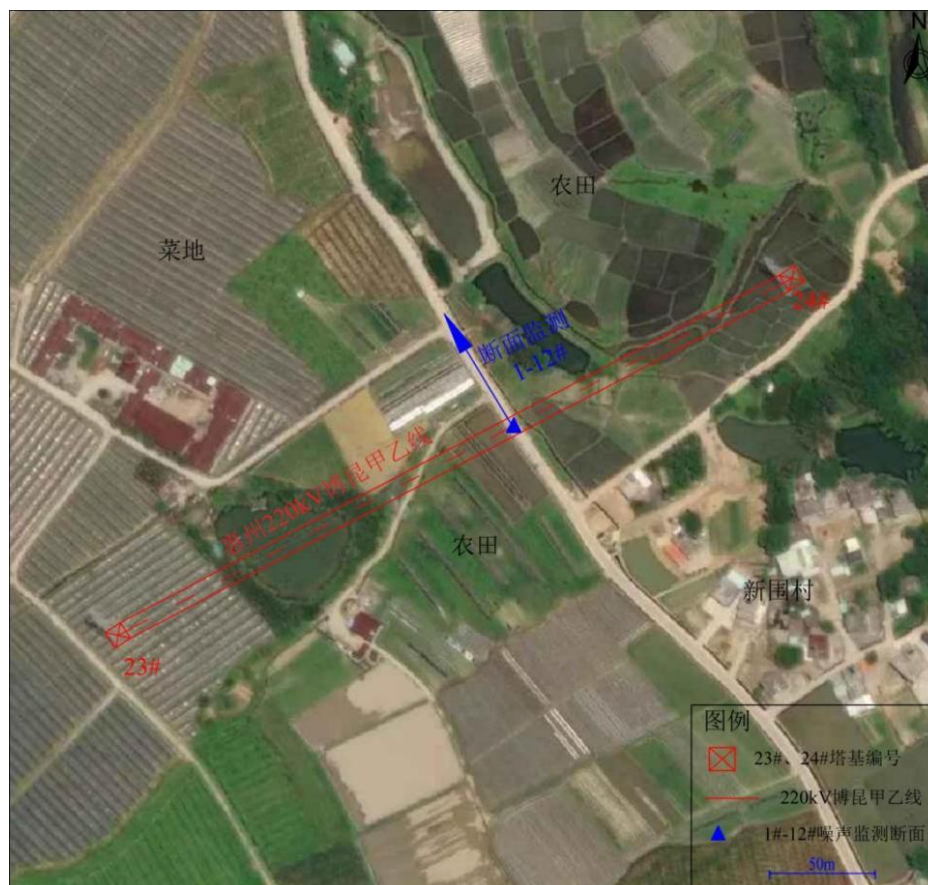
图 4-4 惠州 220kV 博昆甲乙线同塔双回架空线路布点示意图
