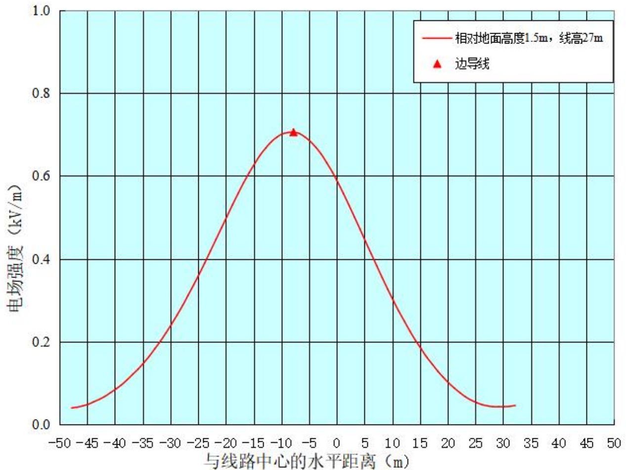
ZT1-图 8.2-4 梅深站至川平站线路（A 线）工频电场强度预测结果衰减趋势线图
