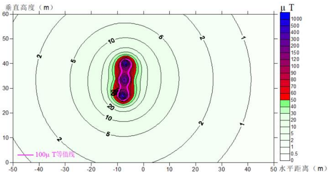
ZT1-图 8.2-11 梅深站至虎地站线路（B 线）工频磁感应强度预测结果等值线图
