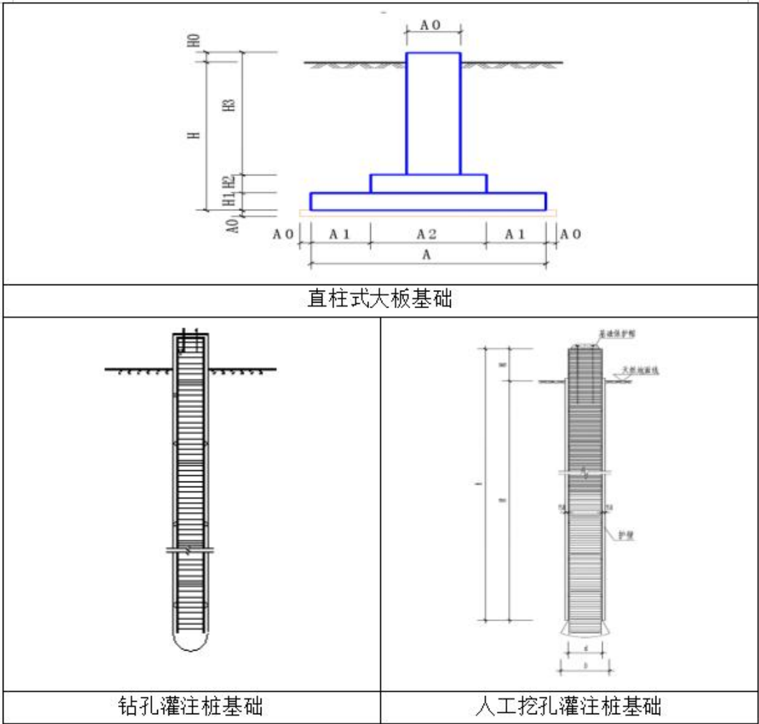
图 2-3 本项目线路工程塔基基础一览图
