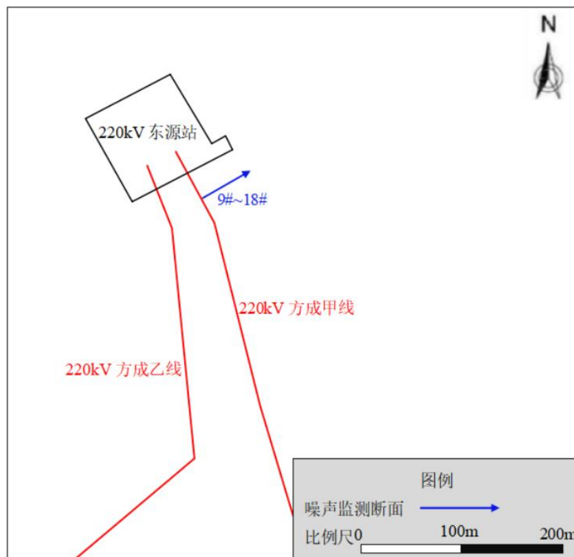
图 4-3 河源 220kV 方成甲线单回架空线路布点示意图
