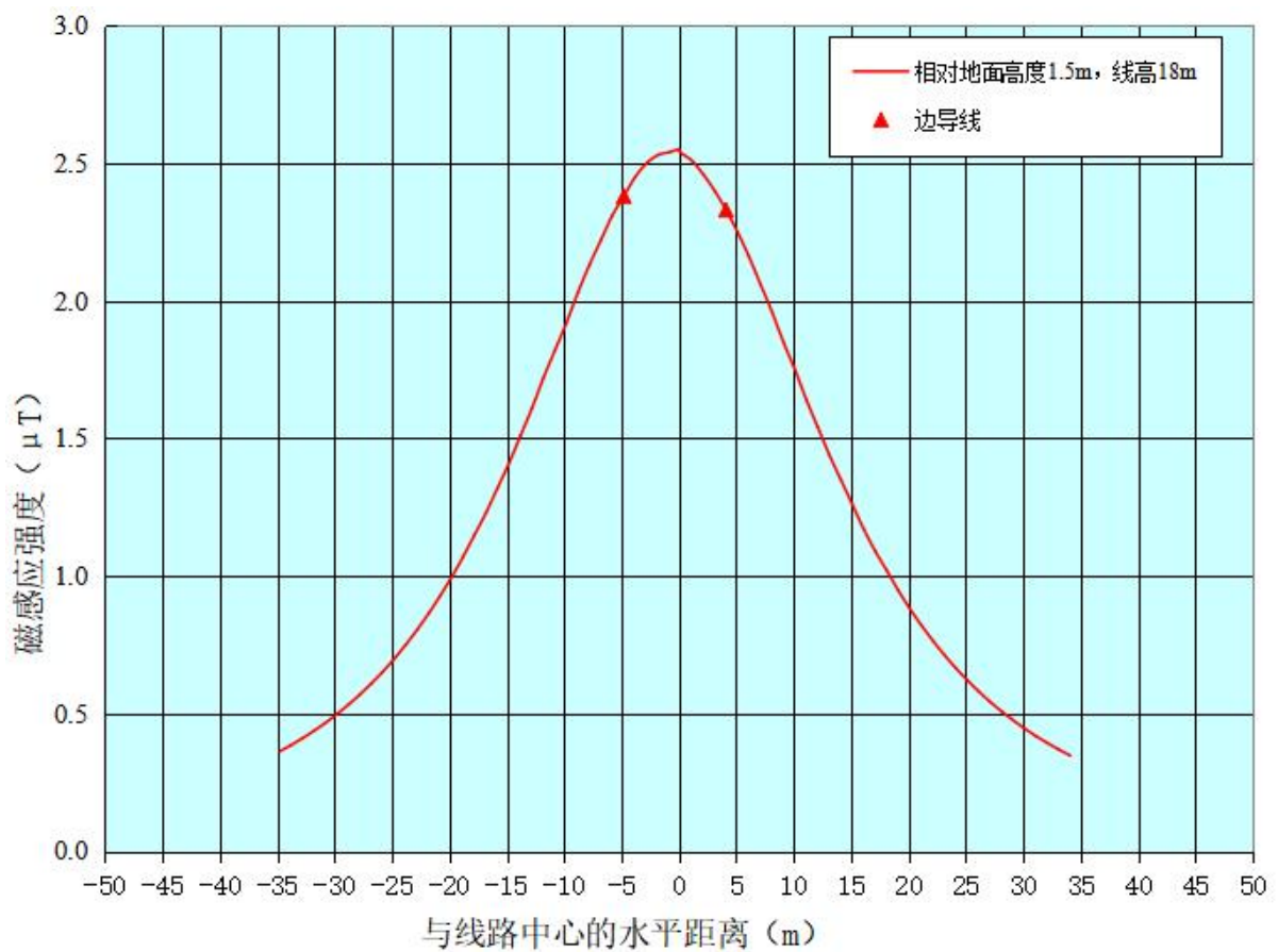
ZT1-图 8.2-21 本项目 110kV 同塔双回线路工频磁感应强度预测结果衰减趋势线图
