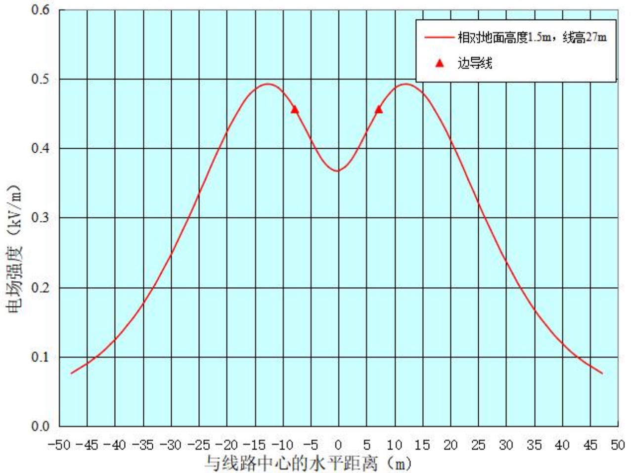
ZT1-图 8.2-12 梅深站至桂竹站线路（C 线）工频电场强度预测结果衰减趋势线图
