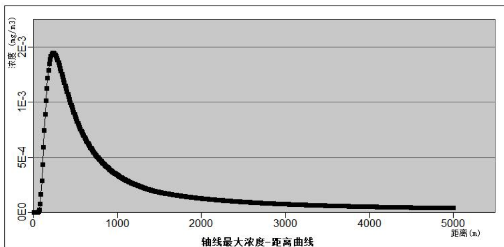
图 6-6 硫酸—轴线最大浓度-距离曲线图（最不利气象）
