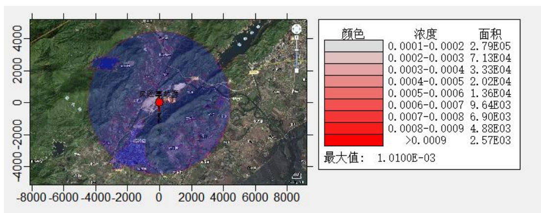
图 6-9 硫酸泄露预测浓度分布图
