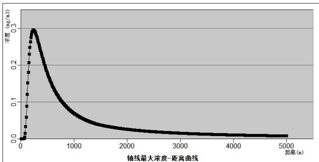
图 6-4 硝酸—轴线最大浓度-距离曲线图（最不利气象）
