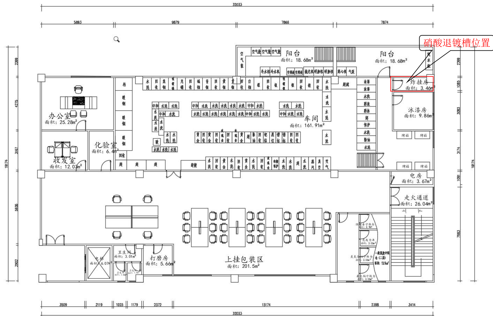
附图 4：本项目平面布置图（硝酸退镀槽位置）
