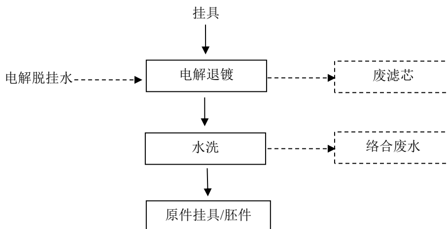
图 2-3 退镀线工艺及产污流程图
