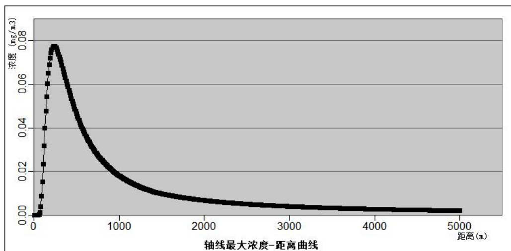
图 6-5 盐酸（氯化氢）—轴线最大浓度-距离曲线图（最不利气象）
