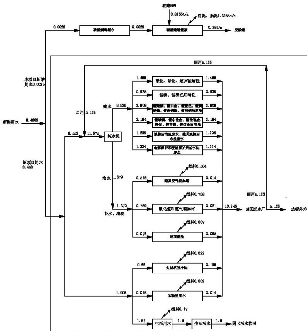
图 2-4 本项目用水平衡图 (m 3 /d)
