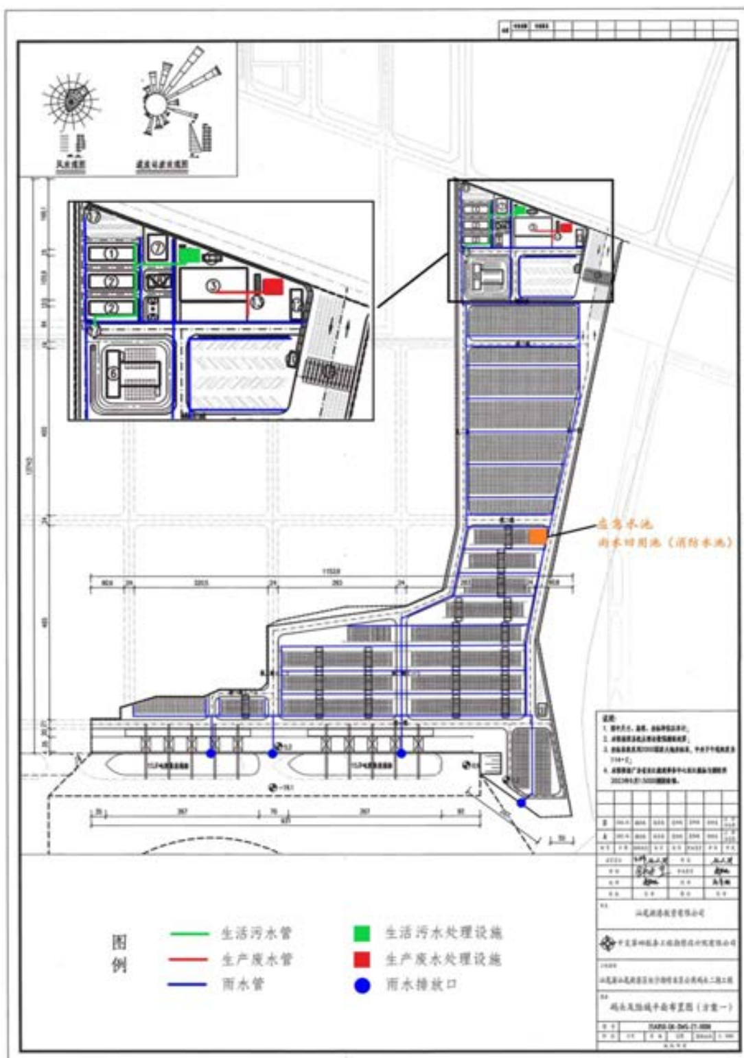
图 3.2-2 本项目雨污水管网设置图
