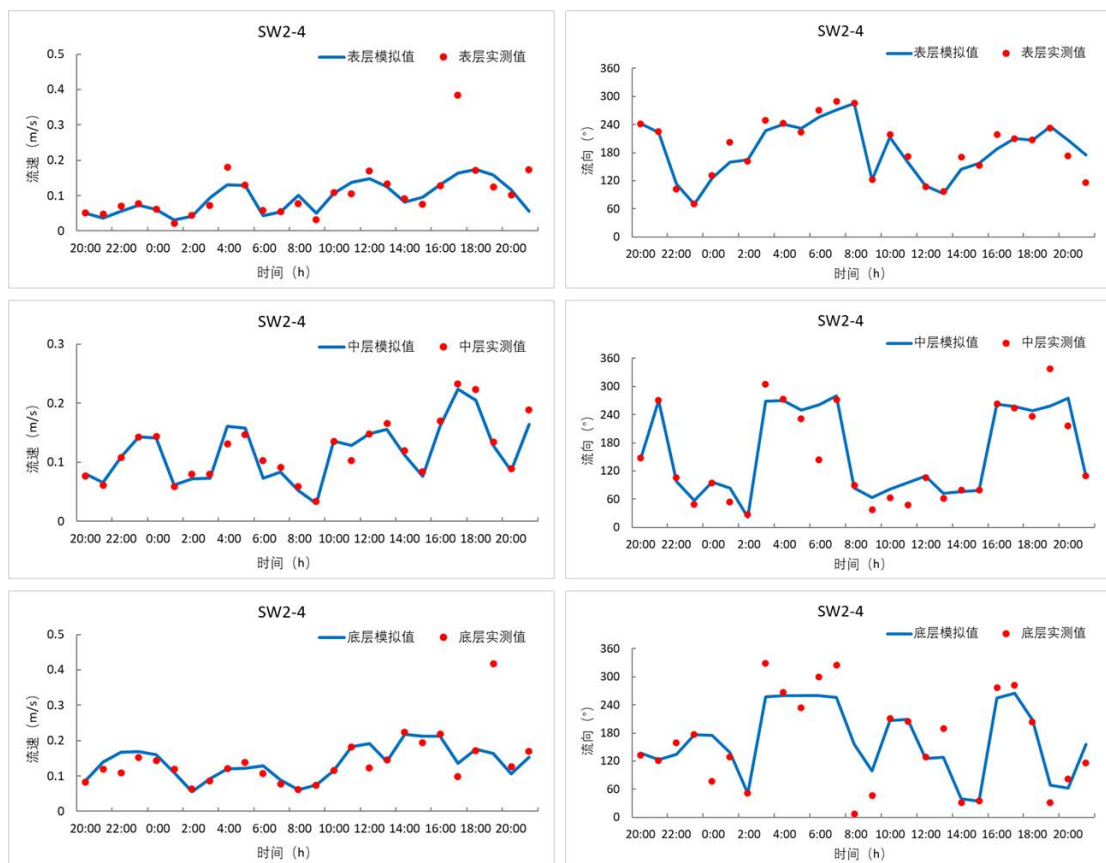
图 6.2-8 SW2-4 站流速和流向验证图（表、中、底层）
