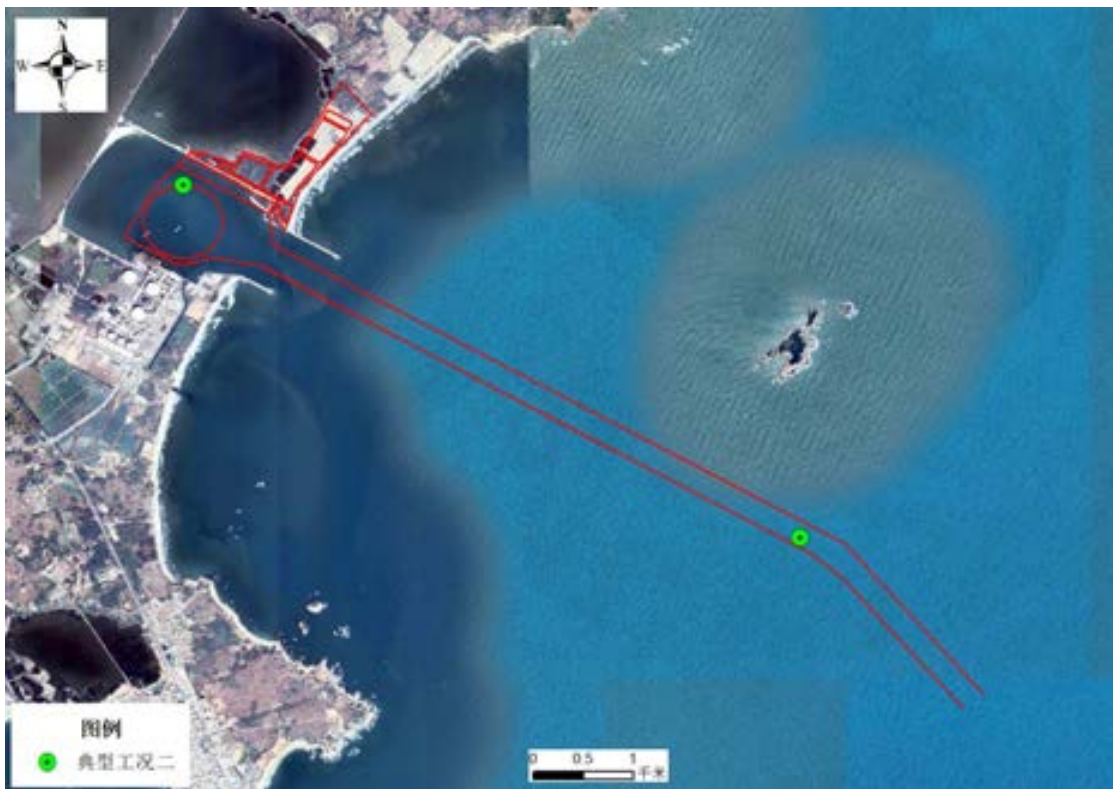
图 6.2-40 施工期典型工况二源强点分布图
