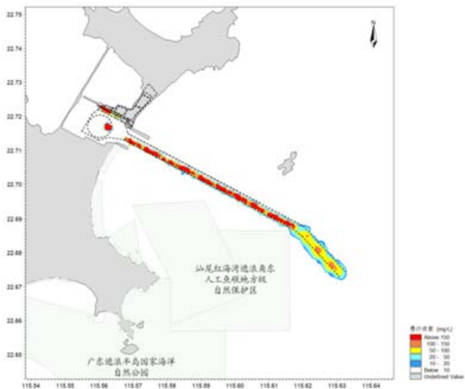
图 6.2-44 典型工况一产生悬沙增量包络线（底层）
