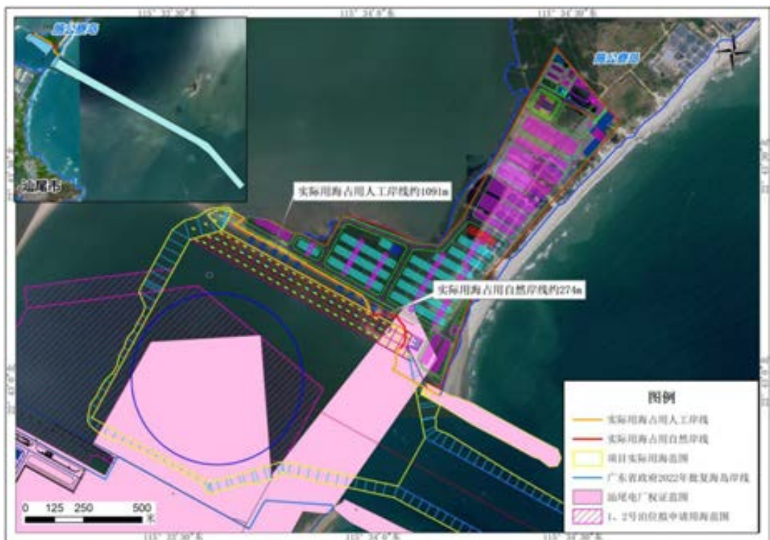
图 9.3-3 本项目实际建设范围占用岸线示意图
