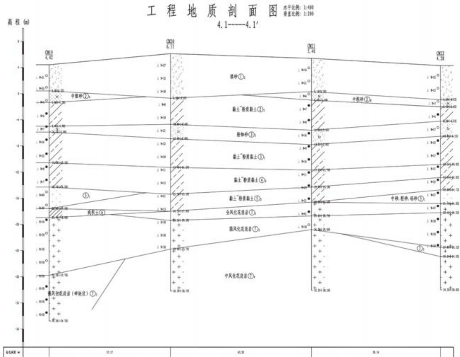
图 4.1-12 工程地质剖面图 (陆域 4.1-4.1')
