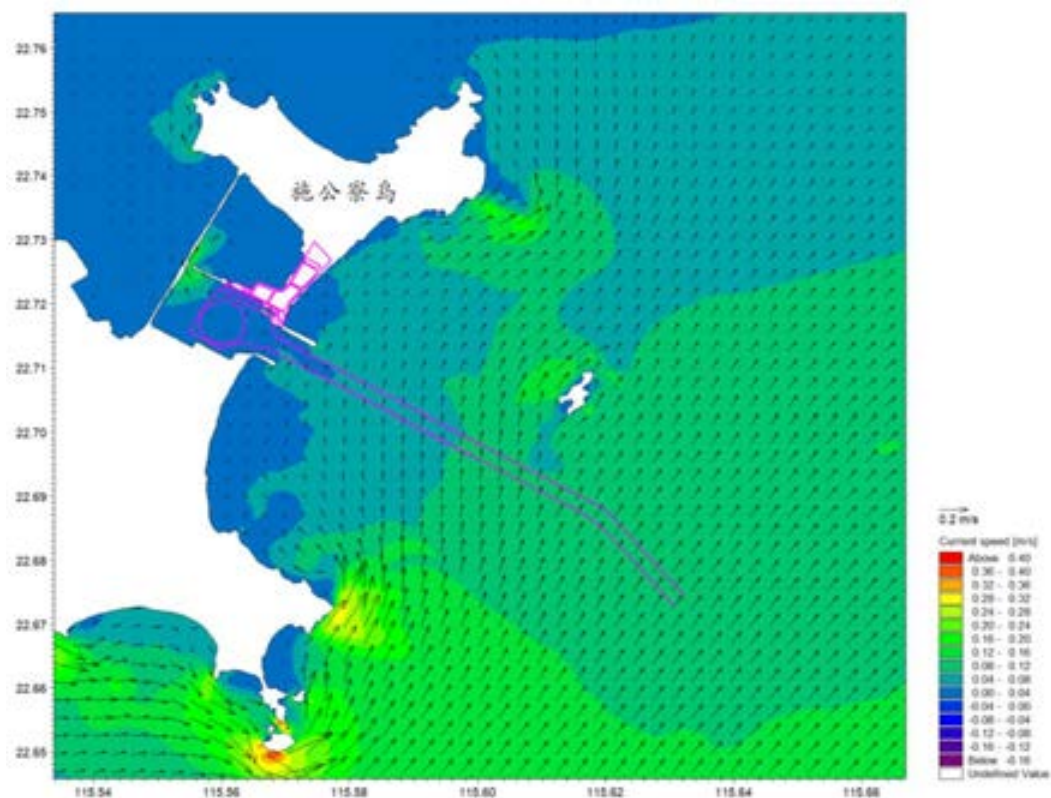
图 6.2-22 项目附近海域大潮落急流场图（底层）
