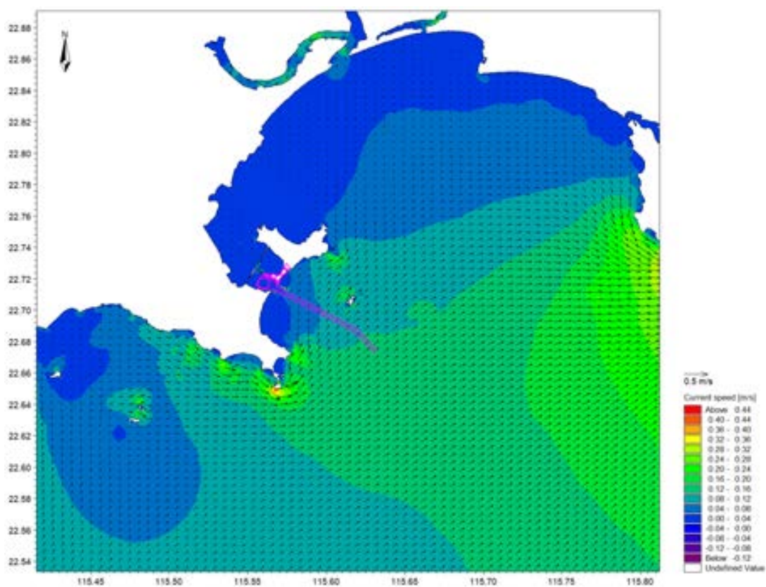
图 6.2-16 项目周边海域大潮落急流场图（底层）
