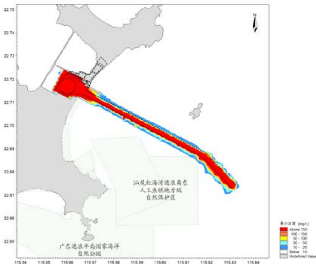
图 6.2-50 最大包络情形产生悬沙增量包络线（底层）
