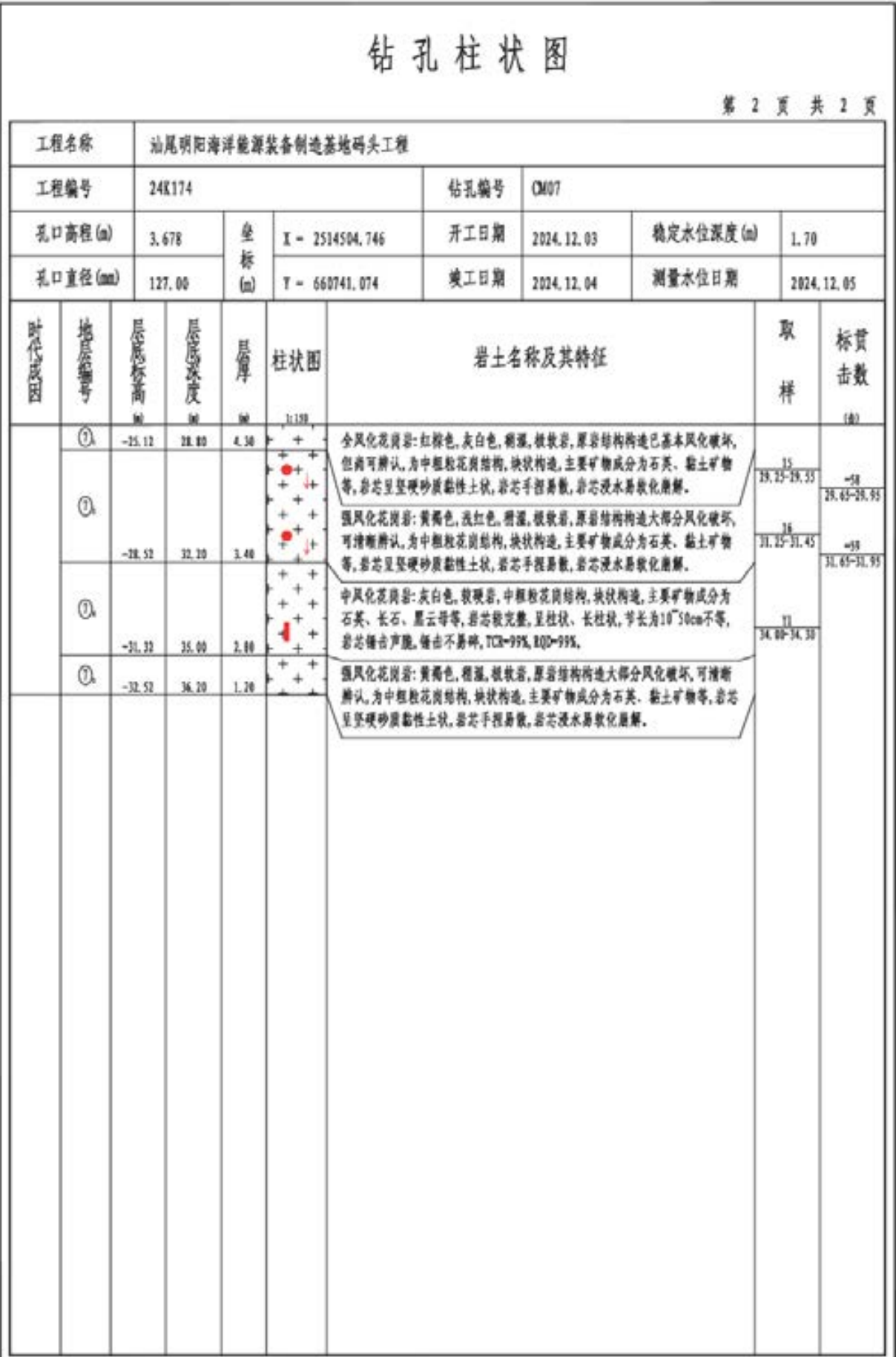
图 4.1-16 钻孔柱状图（二）
