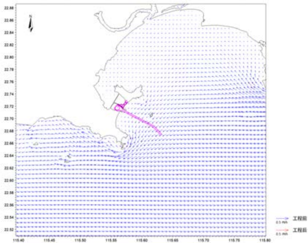
图 6.2-27 工程实施前后项目附近海域涨急流速对比图（中层）
