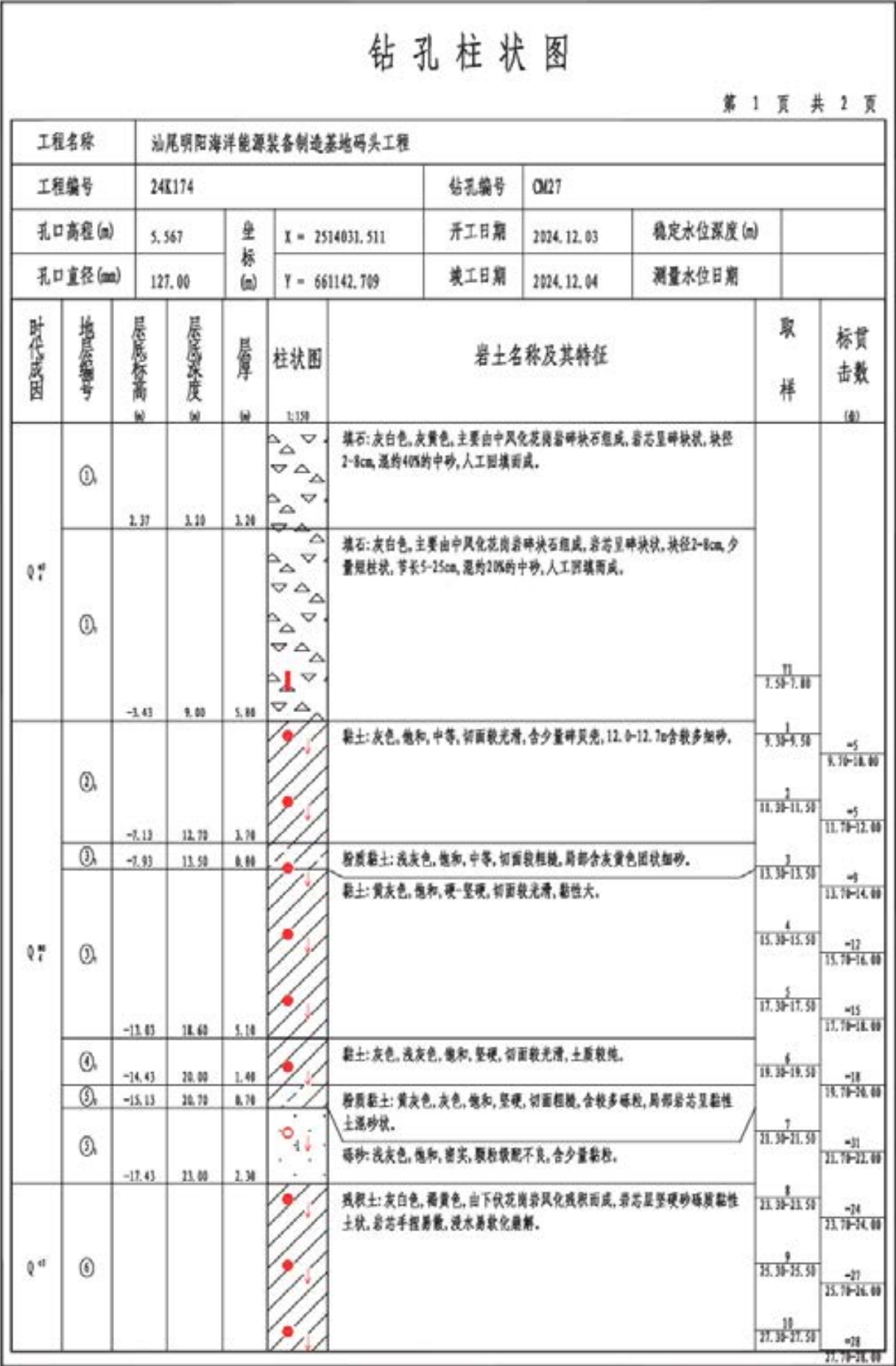
图 4.1-17 钻孔柱状图 (三)
