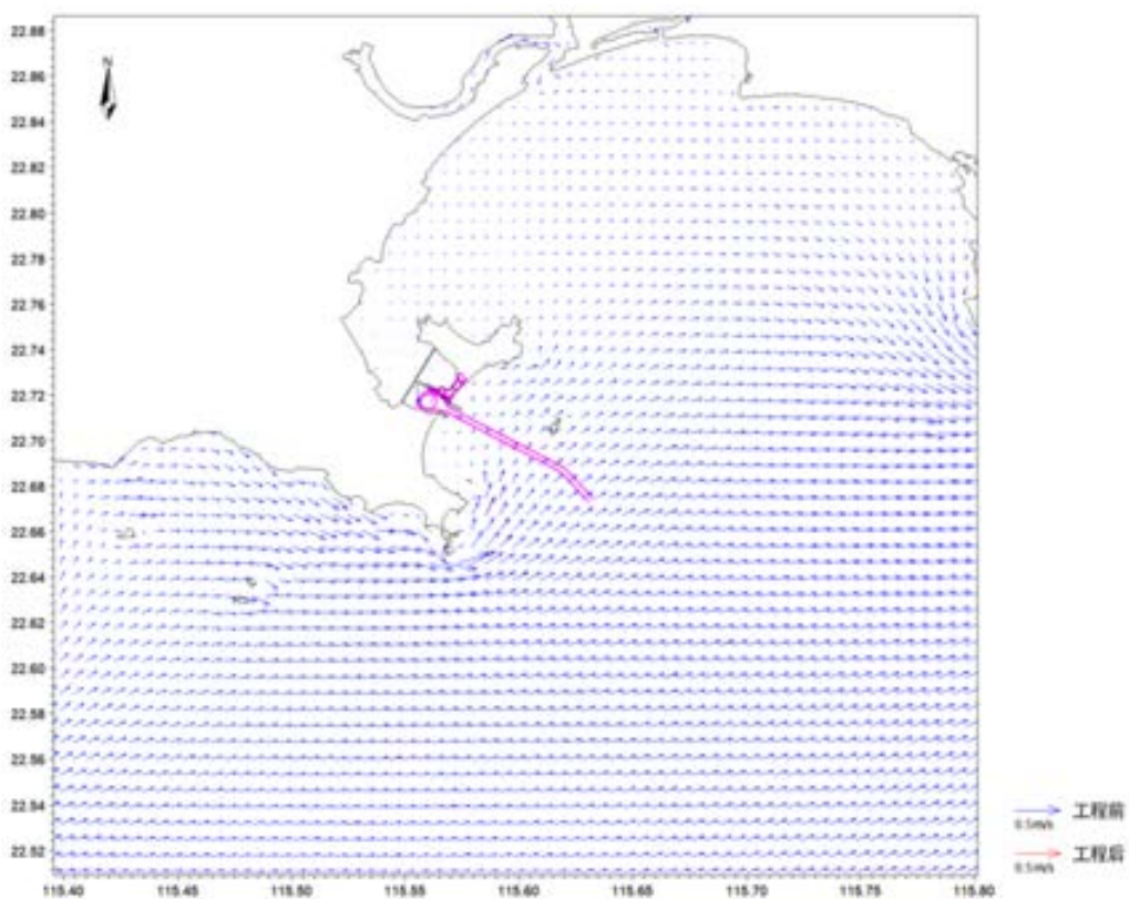
图 6.2-30 工程实施前后项目附近海域落急流速对比图（中层）
