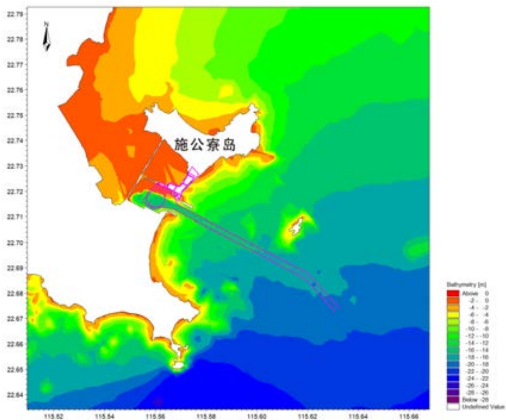
图 6.2-24 工程实施前水动力预测情景的地形分布图
