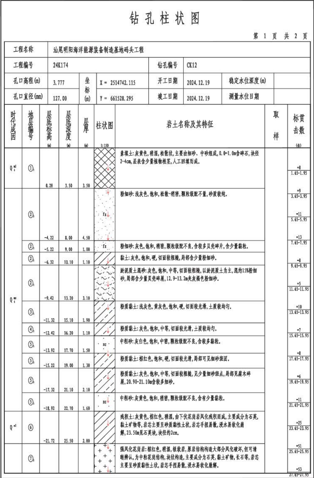
图 4.1-15 钻孔柱状图 (一)
