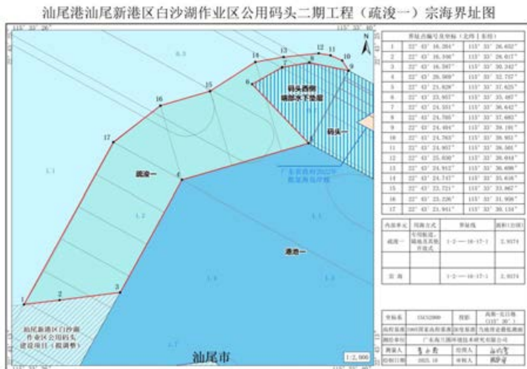
图 3.1-9 本项目宗海界址图（疏浚一）
