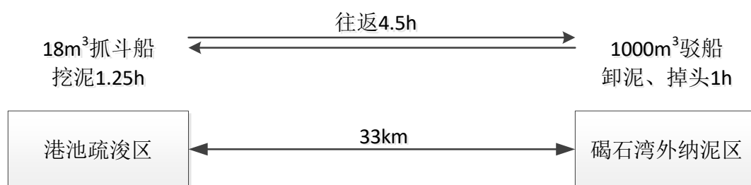
图 3.3-9 本项目港池疏浚投入的抓斗船挖泥运转周期示意图
