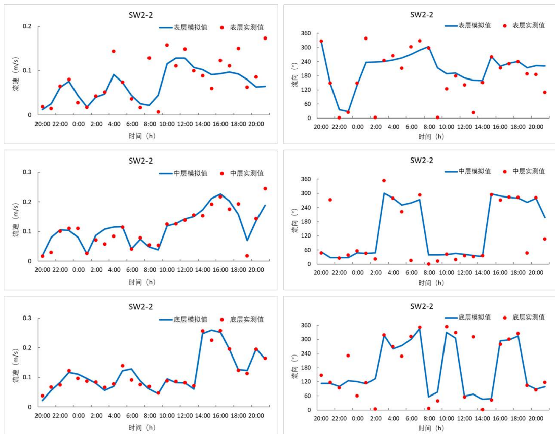
图 6.2-6 SW2-2 站流速和流向验证图（表、中、底层）
