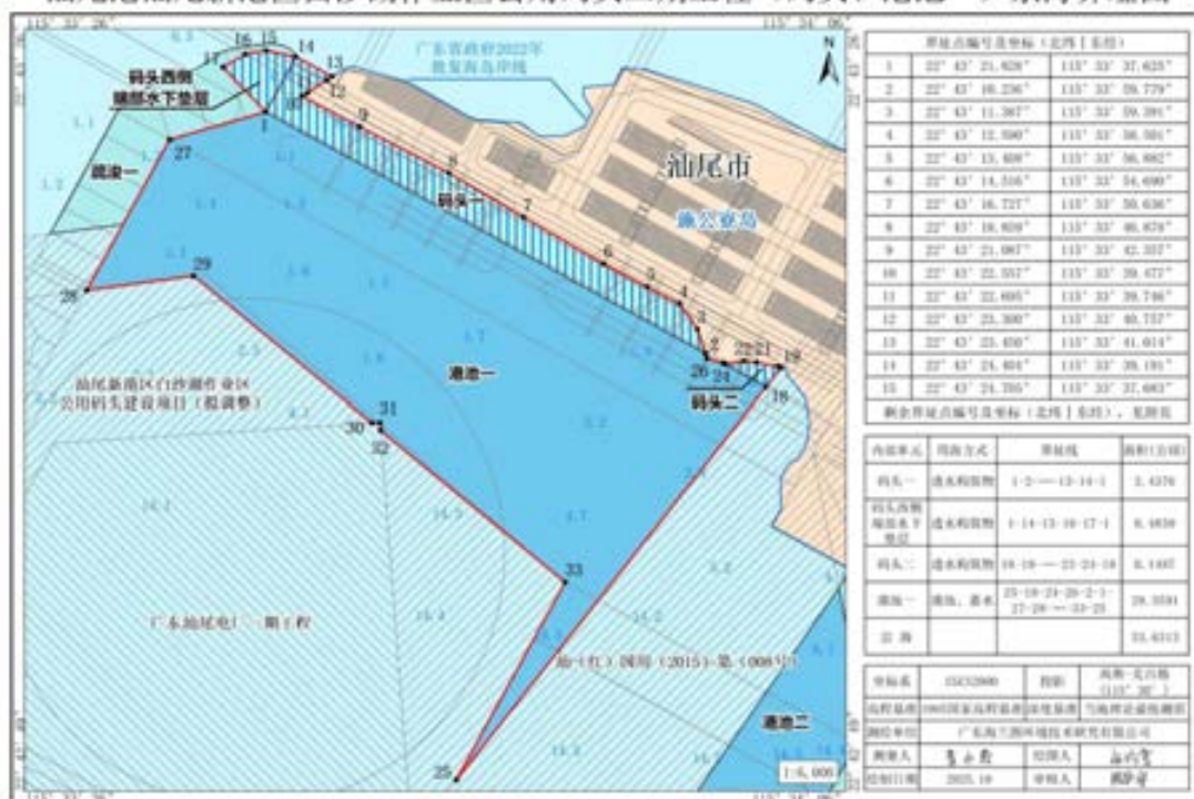
汕尾港汕尾新港区白沙湖作业区公用码头二期工程（码头、港池一）宗海界址图
