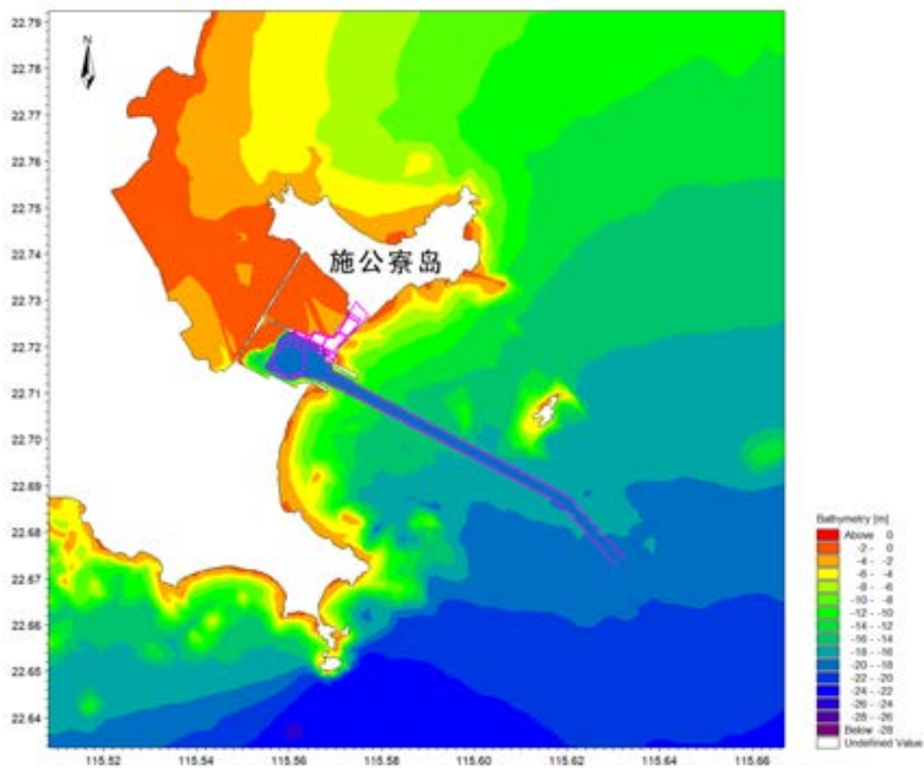
图 6.2-25 工程实施后水动力预测情景的地形分布图
