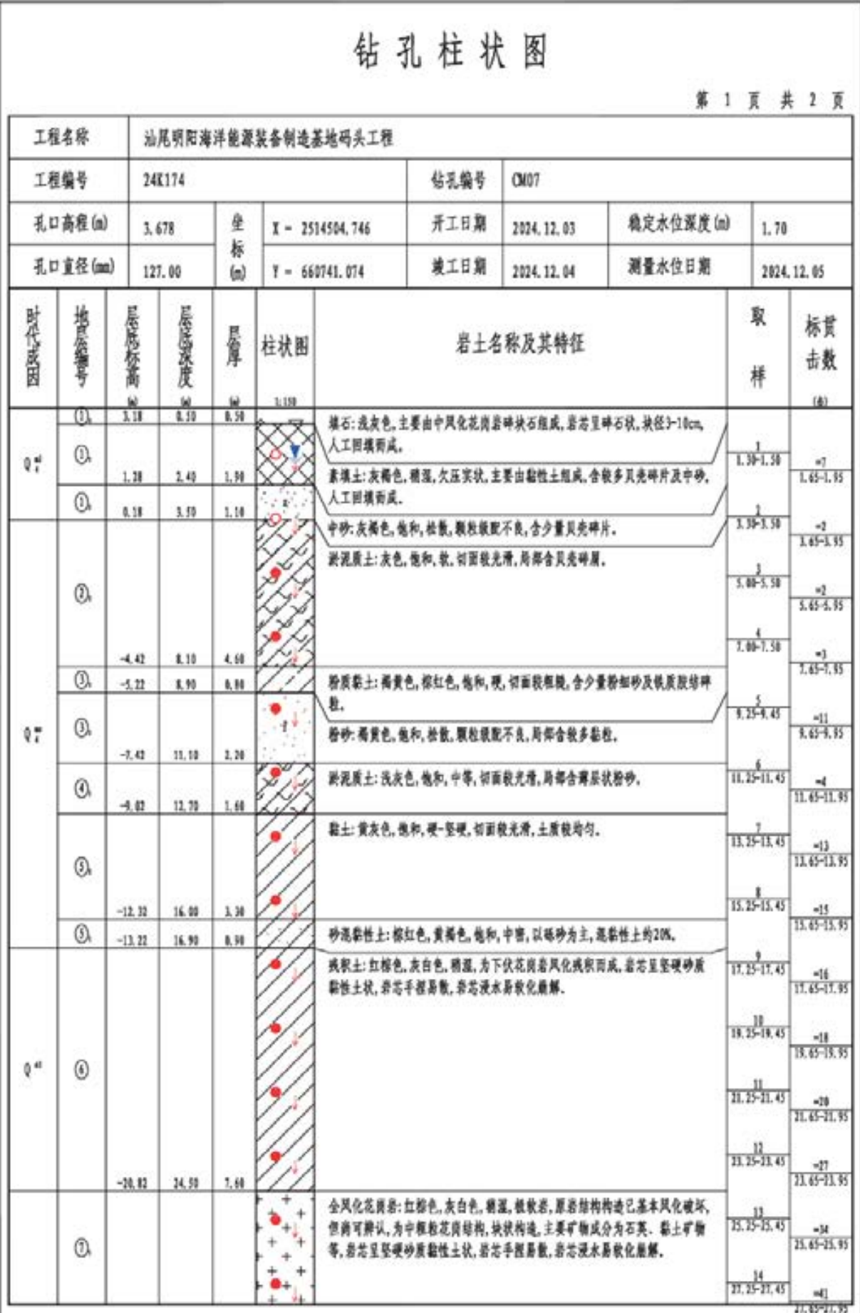
图 4.1-16 钻孔柱状图（二）
