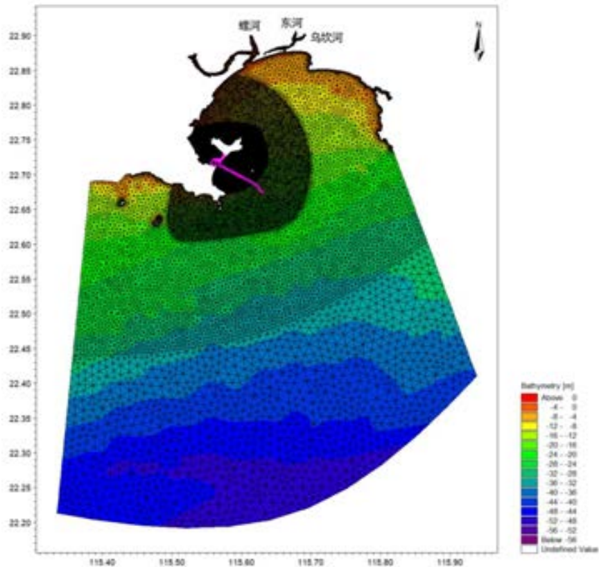
图 6.2-1 模型计算网格以及边界示意图
