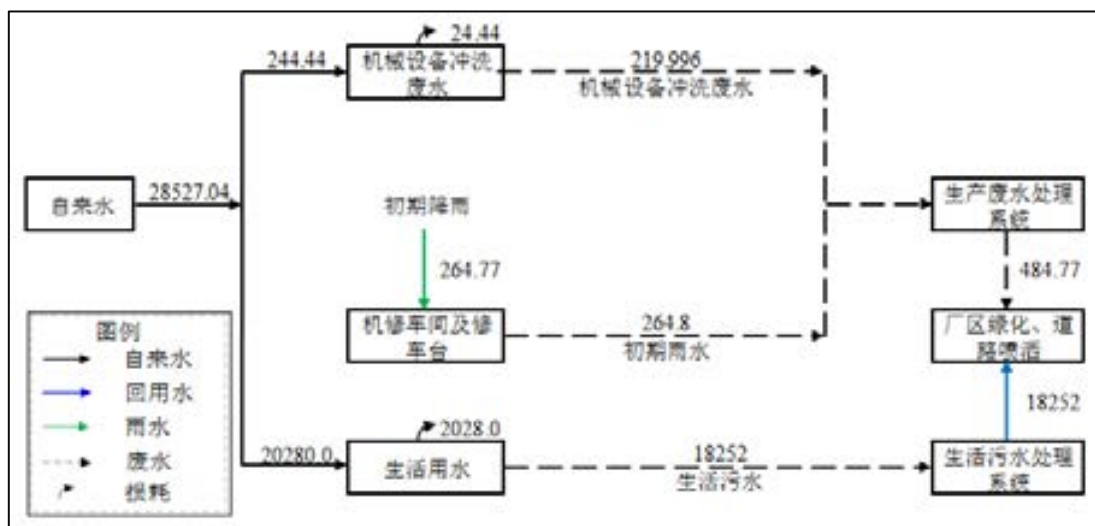
图 3.4-1 本项目水平衡图 (单位: t/a)
