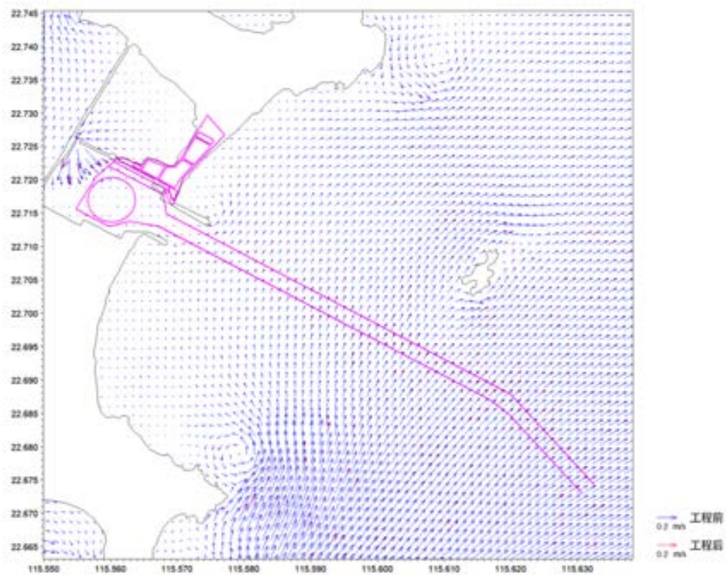
图 6.2-37 工程实施前后项目附近海域落急流速对比图（局部底层）
