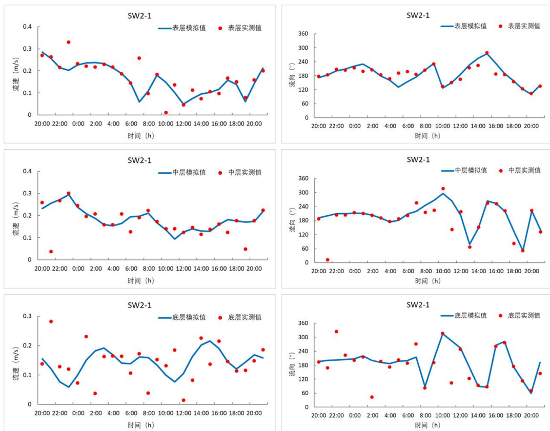
图 6.2-5 SW2-1 站流速和流向验证图（表、中、底层）
