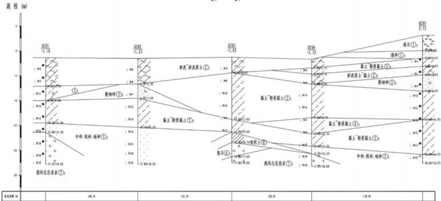
图 4.1-13 工程地质剖面图 (码头区域 27-27')
