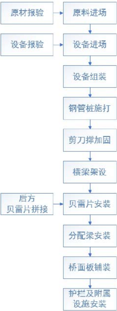
图 3.3-11 施工平台施工工艺流程图
