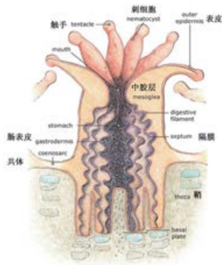
图 4.2-6 珊瑚结构
