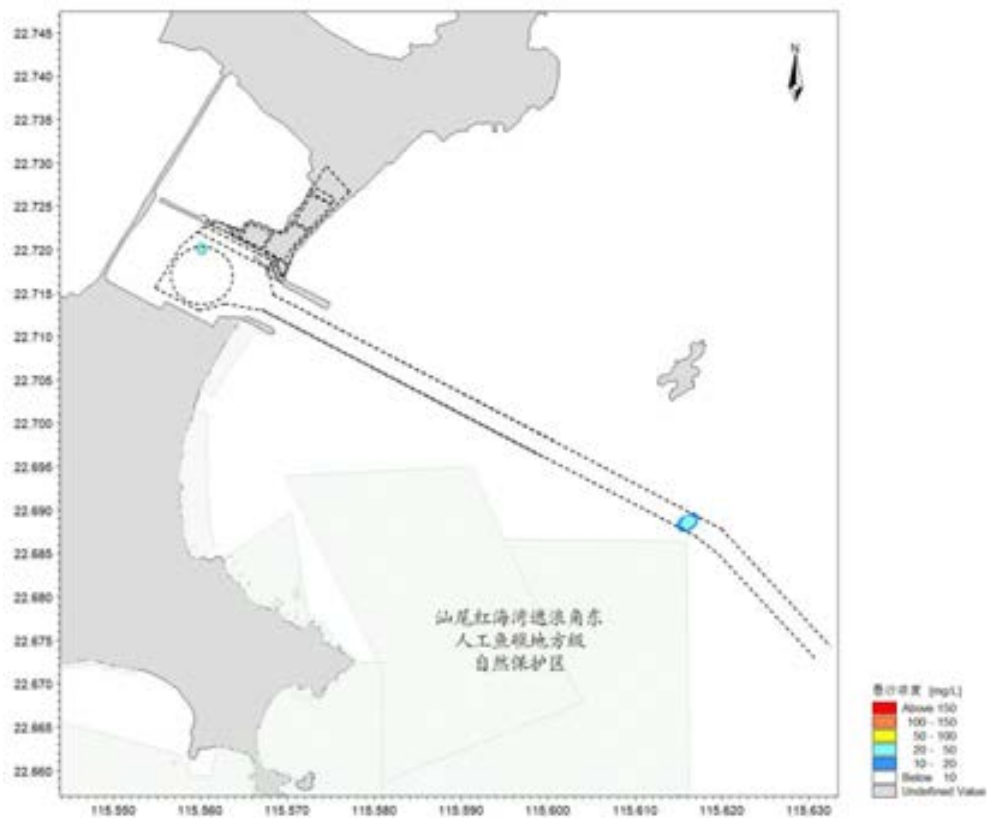
图 6.2-46 典型工况二产生悬沙增量包络线（中层）
