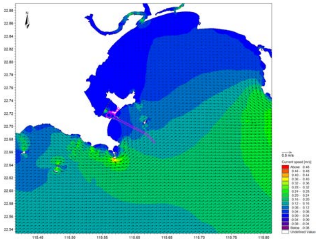
图 6.2-15 项目周边海域大潮落急流场图（中层）
