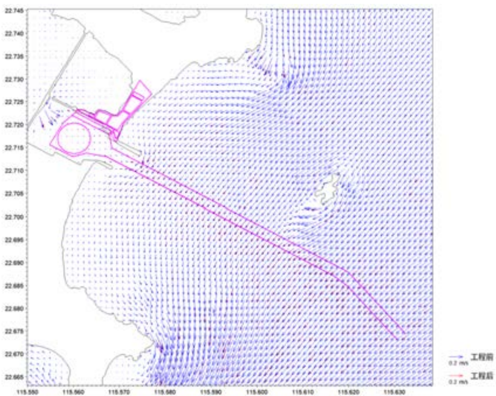
图 6.2-32 工程实施前后项目附近海域涨急流速对比图（局部表层）
