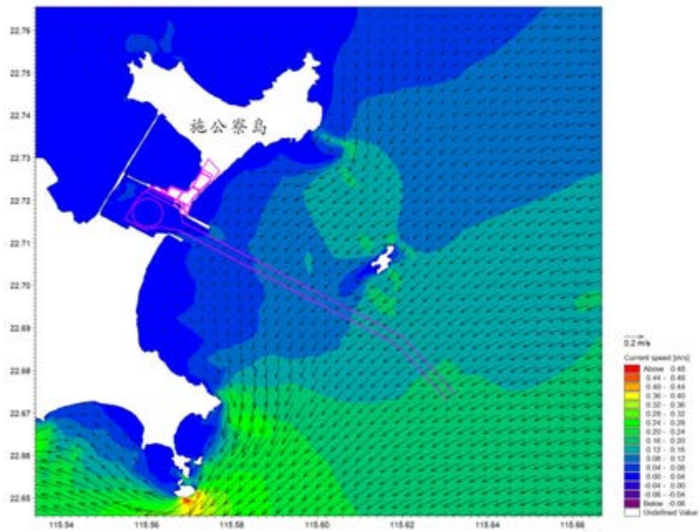
图 6.2-18 项目附近海域大潮涨急流场图（中层）
