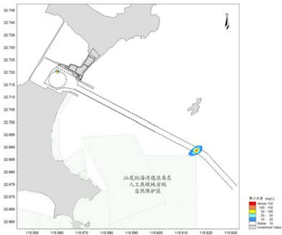
图 6.2-47 典型工况二产生悬沙增量包络线（底层）
