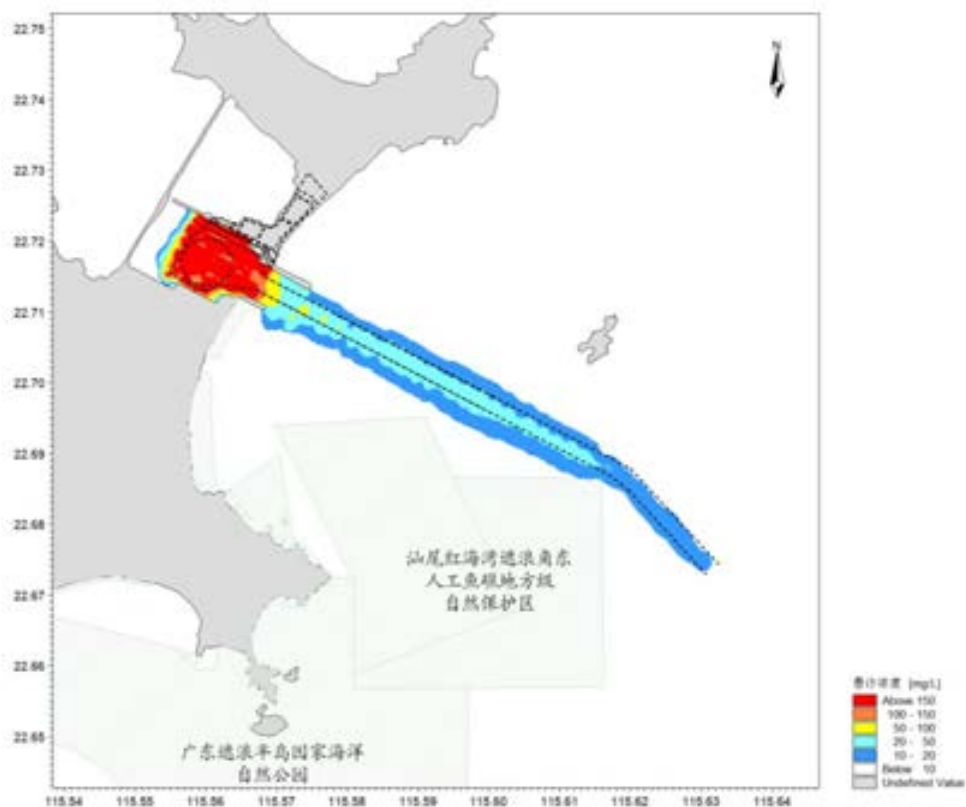
图 6.2-49 最大包络情形产生悬沙增量包络线（中层）
