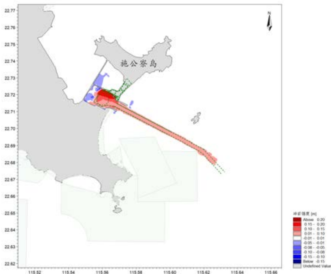
图 6.2-38 工程后附近海区冲淤图（红色淤积、蓝色冲刷）
