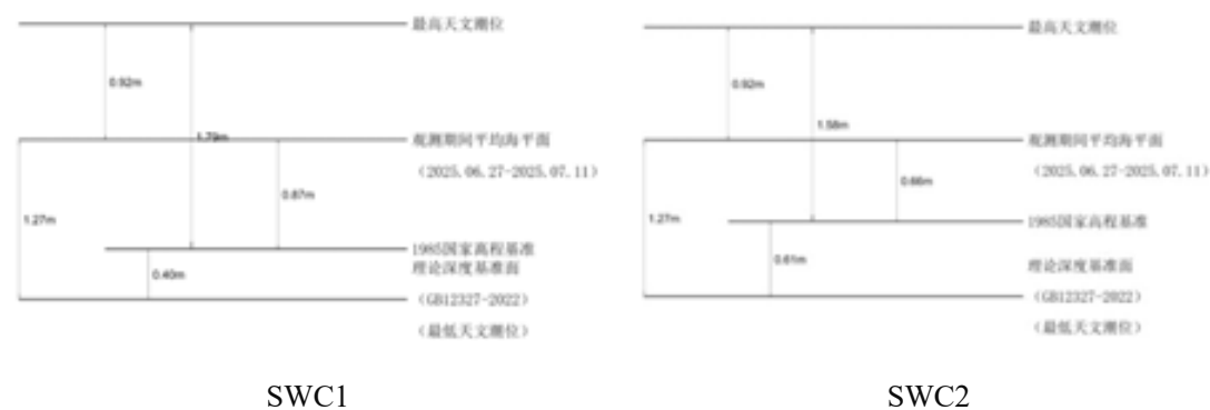
图 5.1-13 临时潮位站各基准面的相互关系
