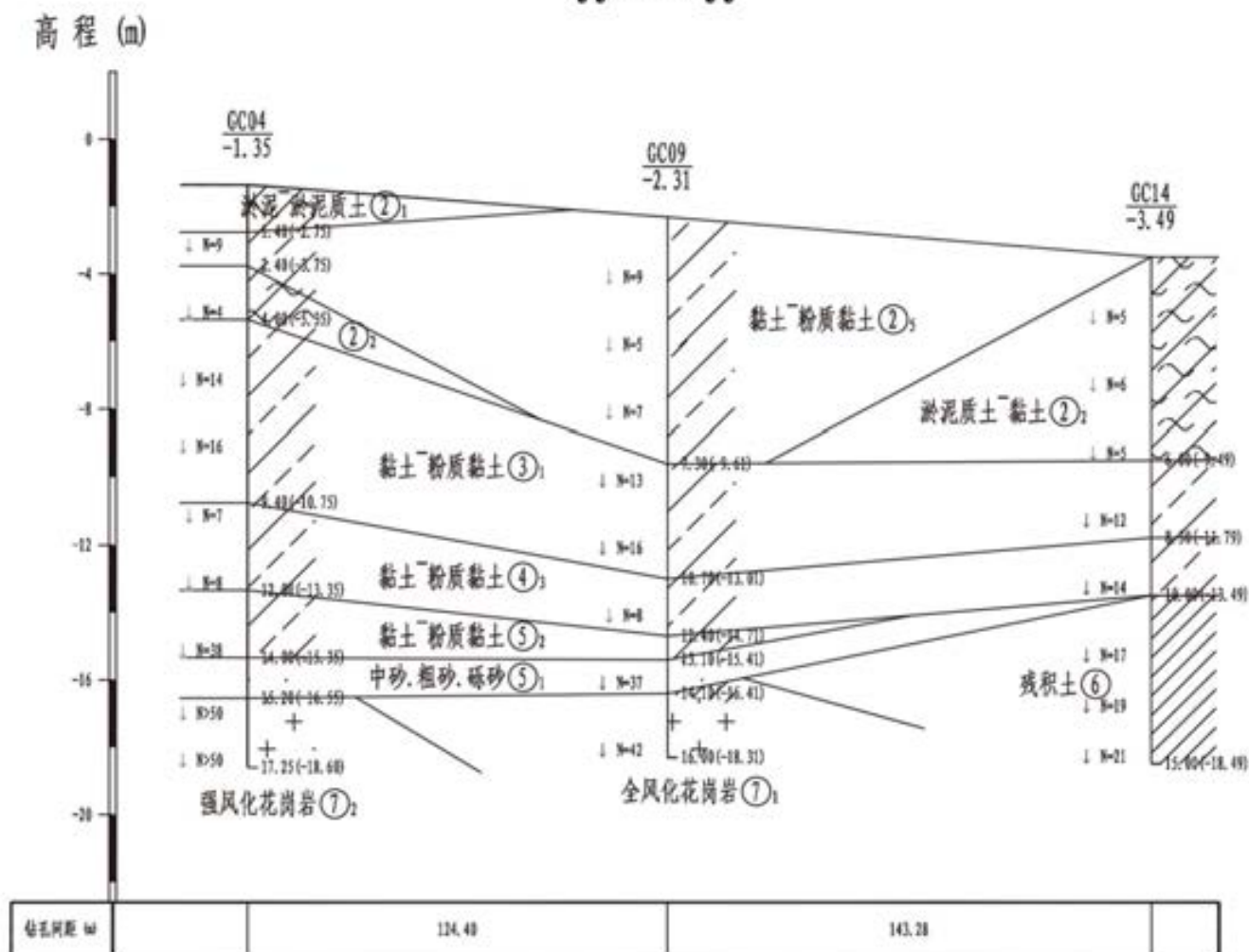
图 4.1-14 工程地质剖面图 (码头区域 33-33')
