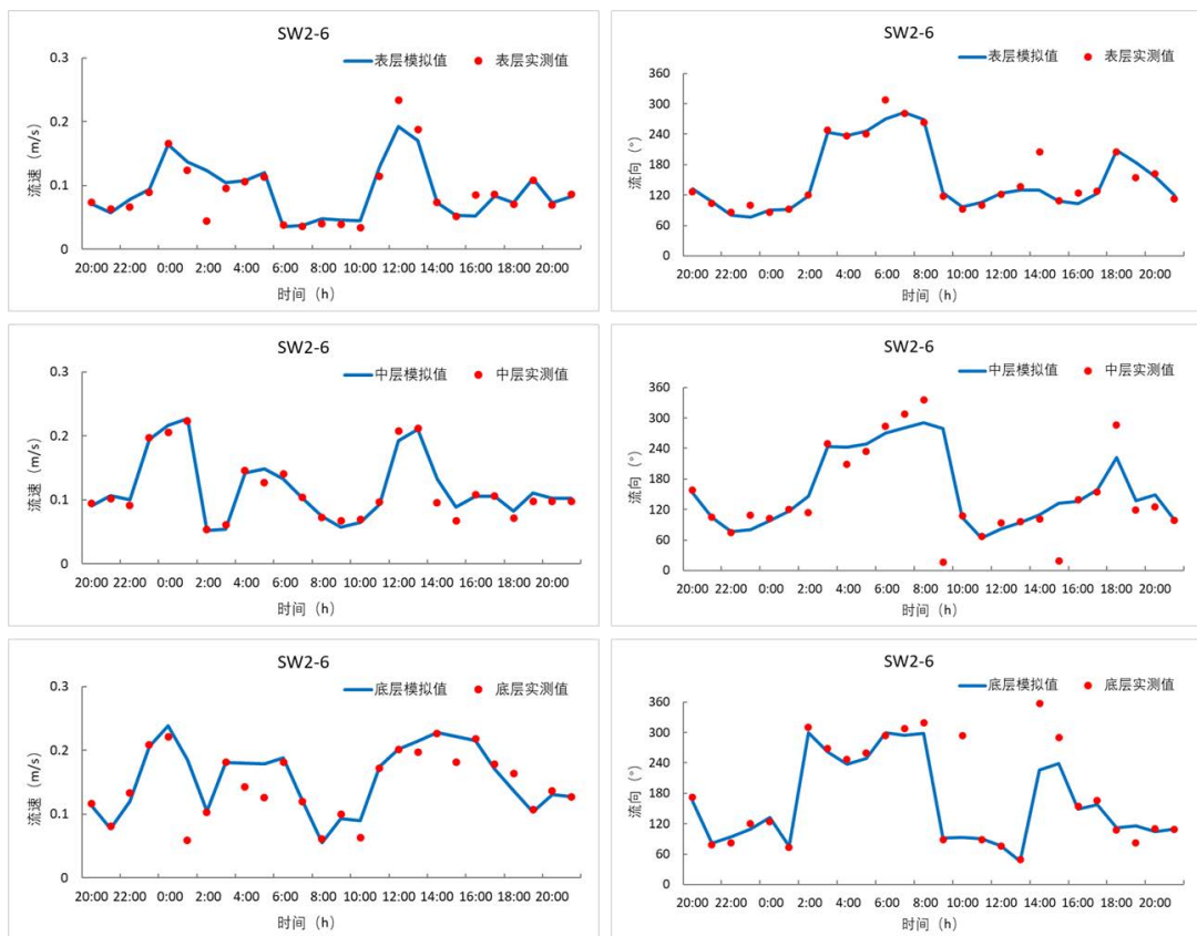
图 6.2-10 SW2-6 站流速和流向验证图（表、中、底层）
