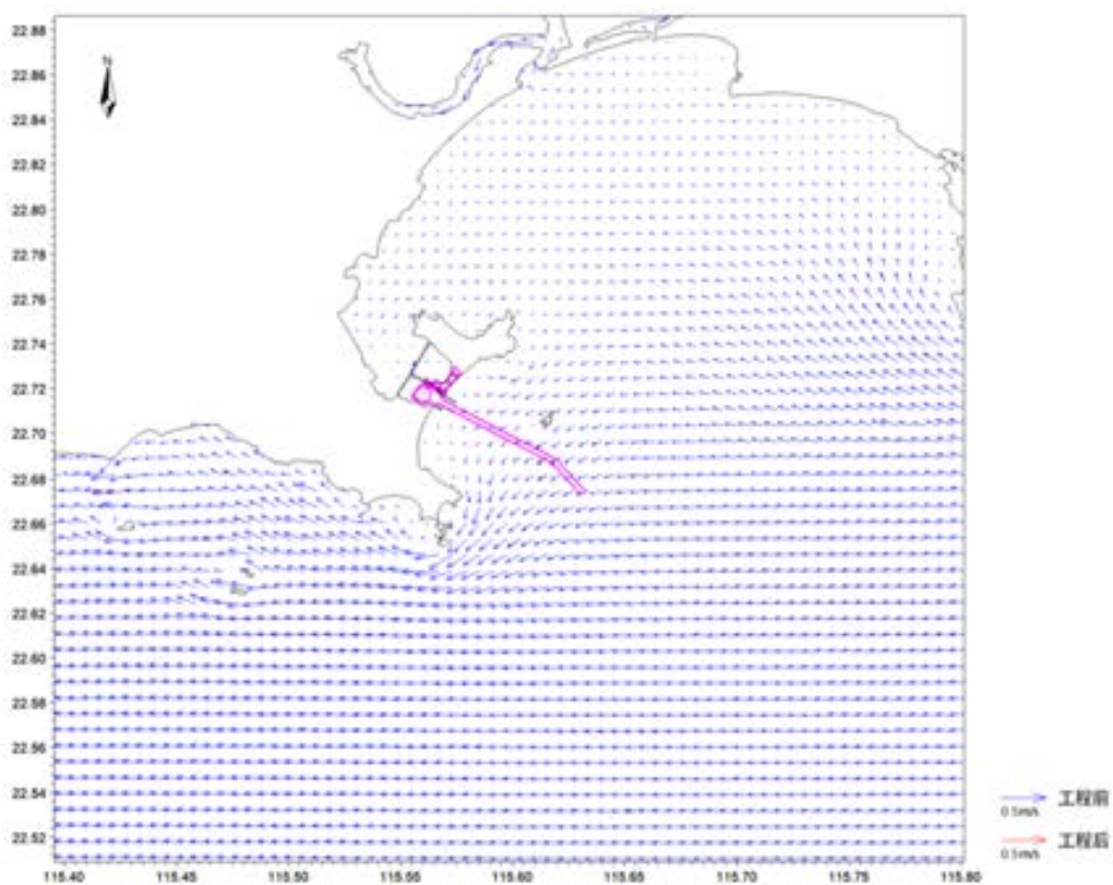
图 6.2-28 工程实施前后项目附近海域涨急流速对比图（底层）
