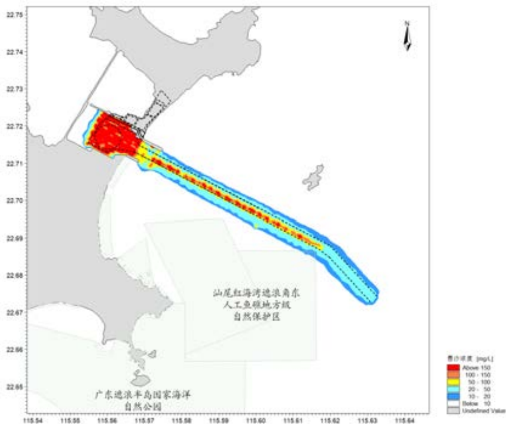
图 6.2-48 最大包络情形产生悬沙增量包络线（表层）
