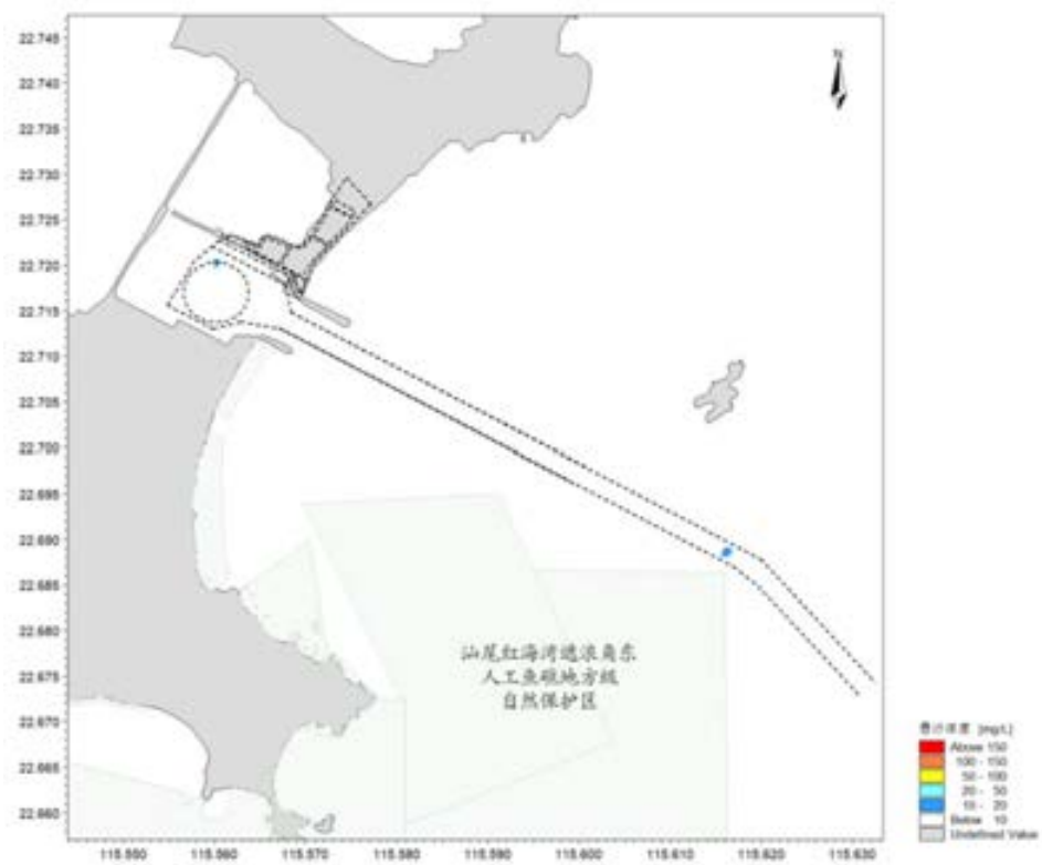
图 6.2-45 典型工况二产生悬沙增量包络线（表层）
