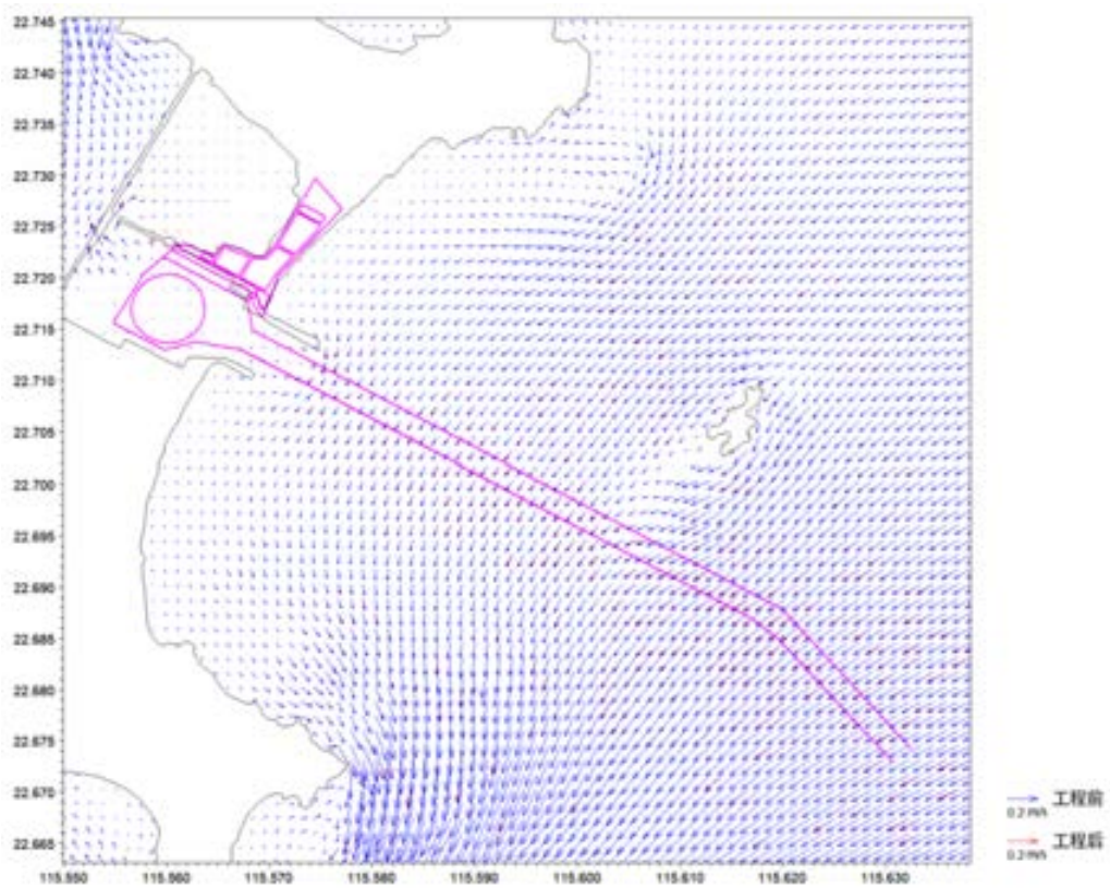
图 6.2-34 工程实施前后项目附近海域涨急流速对比图（局部底层）
