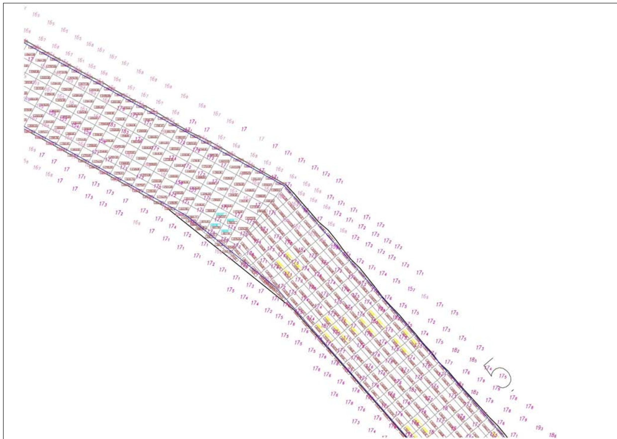
图 3.1-35 本项目疏浚范围局部放大图—4
