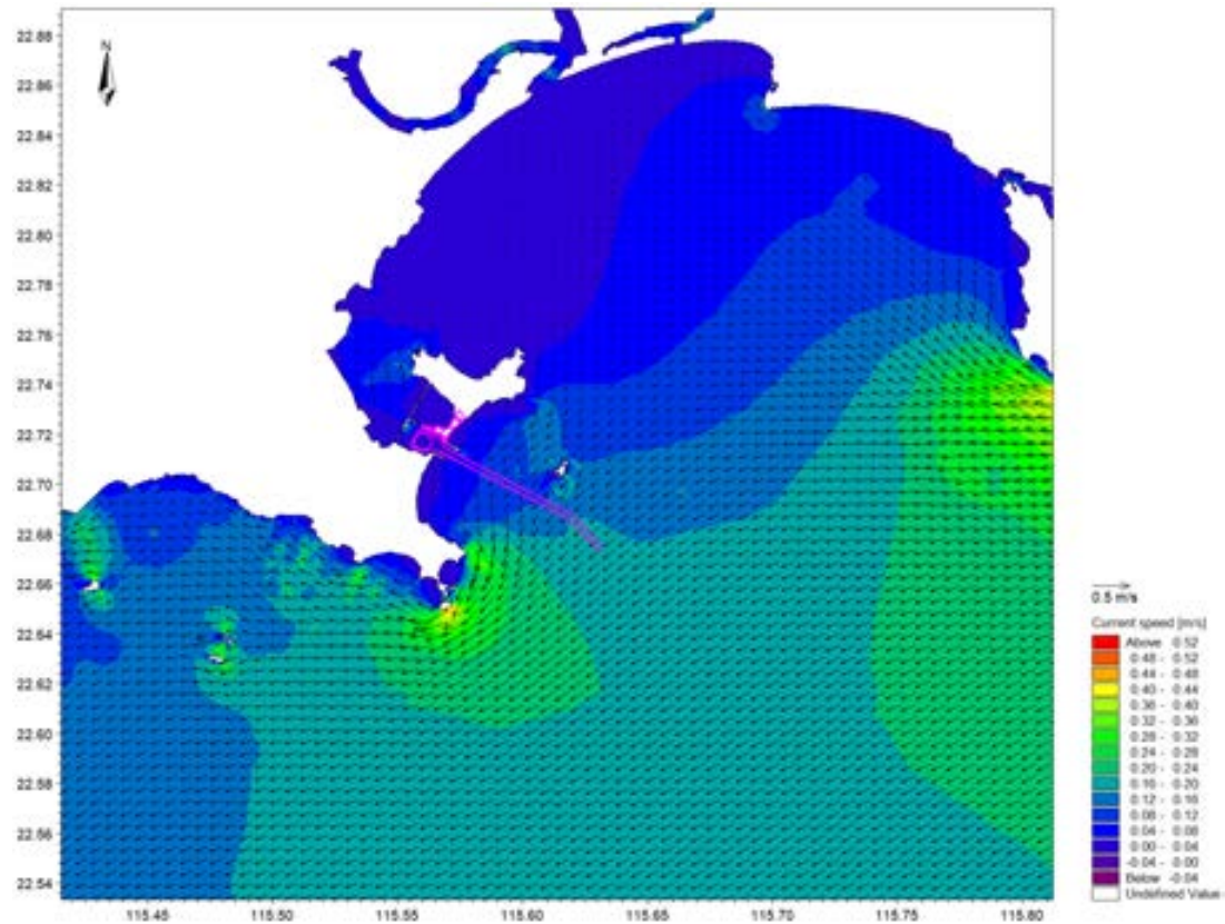
图 6.2-11 项目周边海域大潮涨急流场图（表层）
