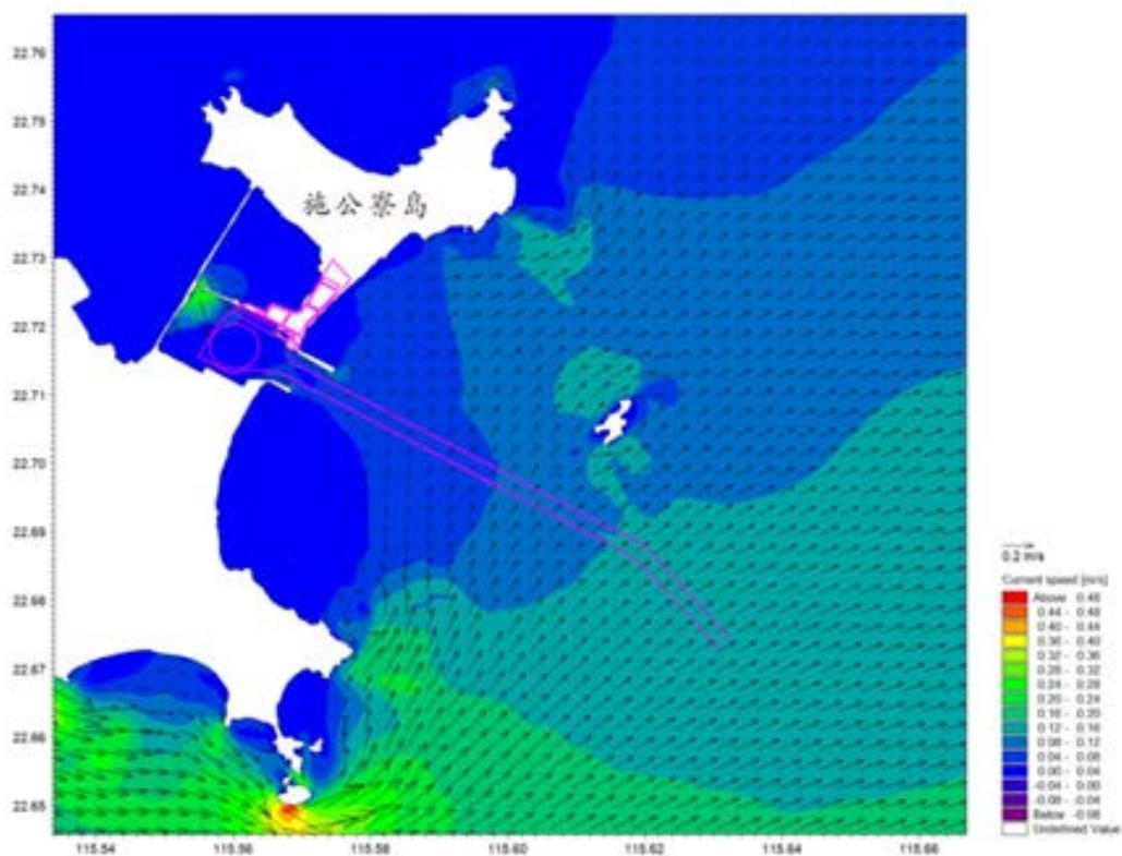
图 6.2-21 项目附近海域大潮落急流场图（中层）
