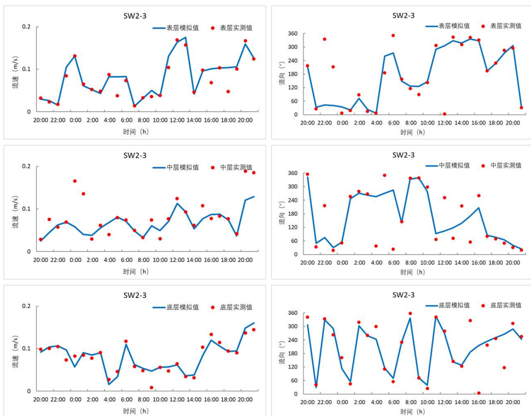
图 6.2-7 SW2-3 站流速和流向验证图（表、中、底层）
