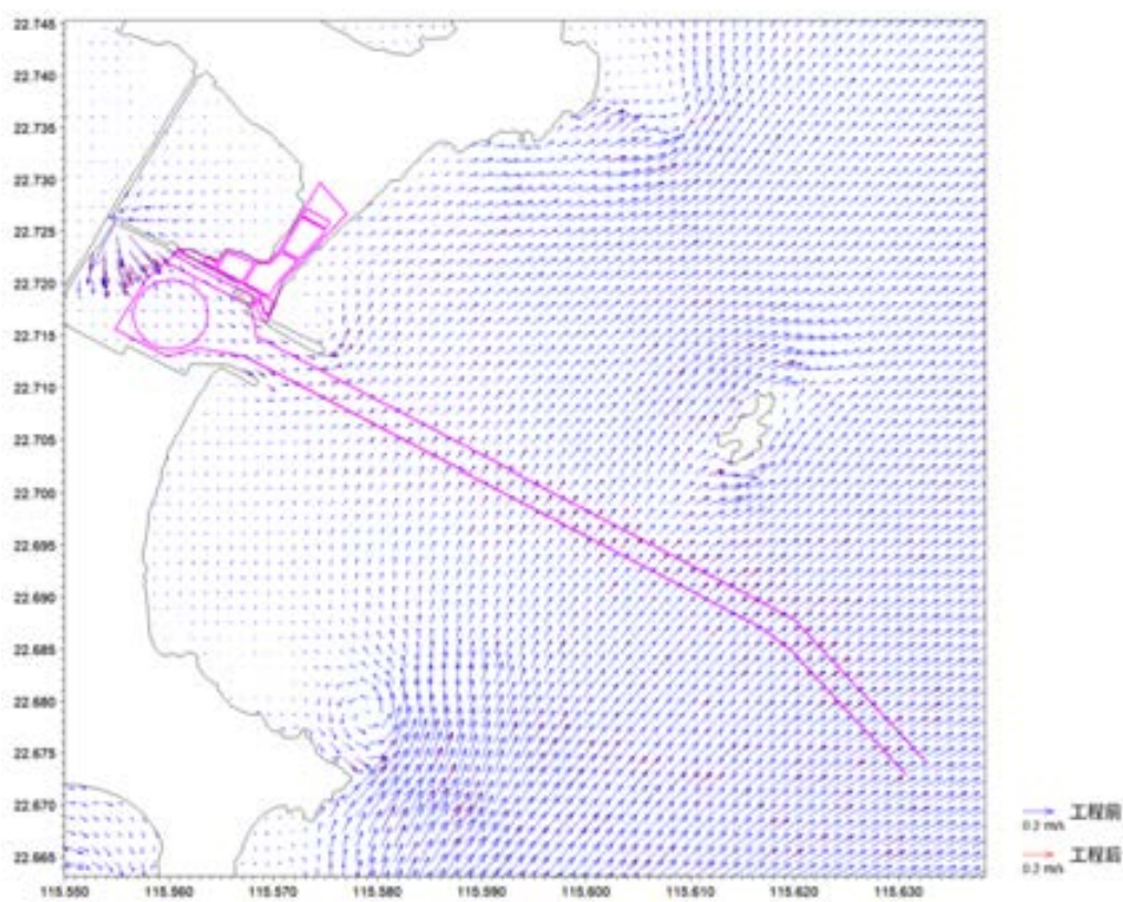
图 6.2-36 工程实施前后项目附近海域落急流速对比图（局部中层）
