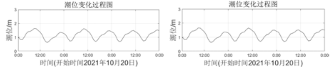
图 5.1-2 SWC3 站、SWC4 站潮位过程曲线
