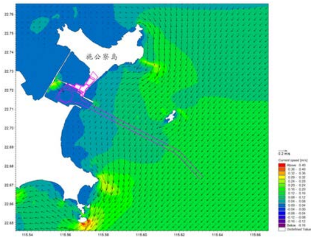
图 6.2-19 项目附近海域大潮涨急流场图（底层）
