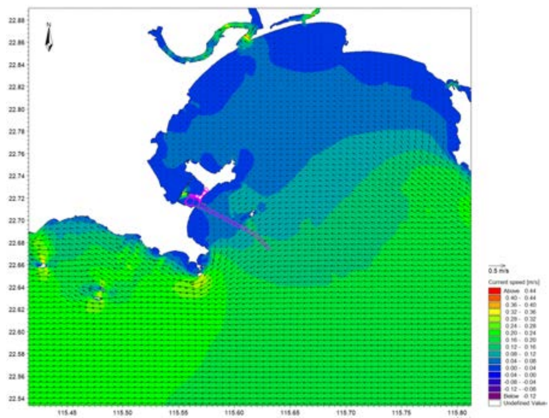
图 6.2-13 项目周边海域大潮涨急流场图（底层）
