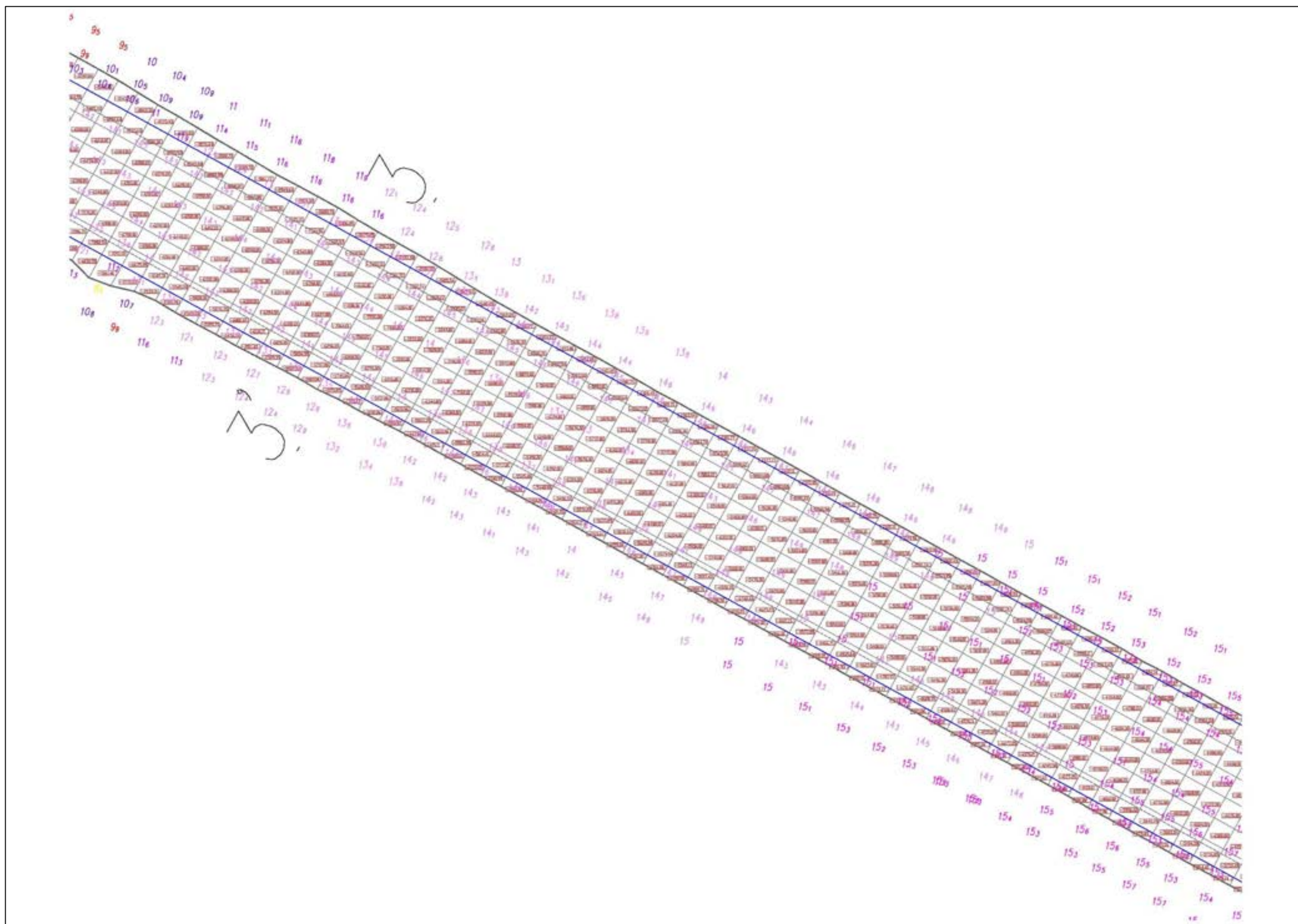
图 3.1-33 本项目疏浚范围局部放大图—2
