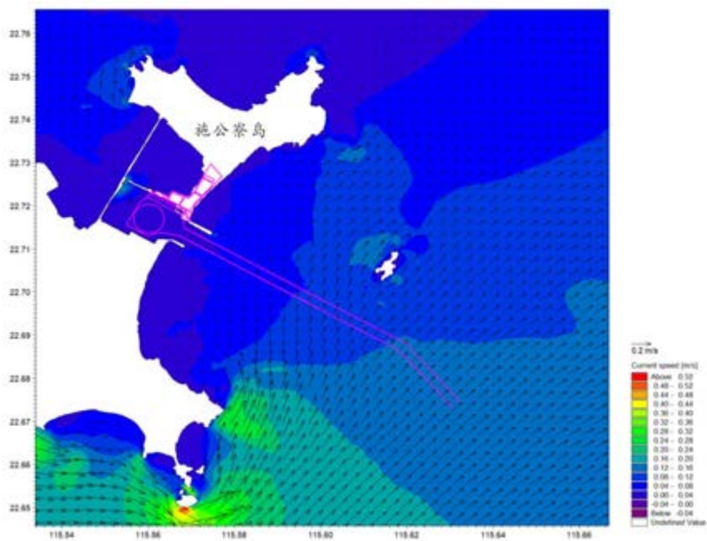
图 6.2-20 项目附近海域大潮落急流场图（表层）
