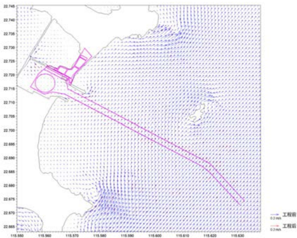
图 6.2-35 工程实施前后项目附近海域落急流速对比图（局部表层）
