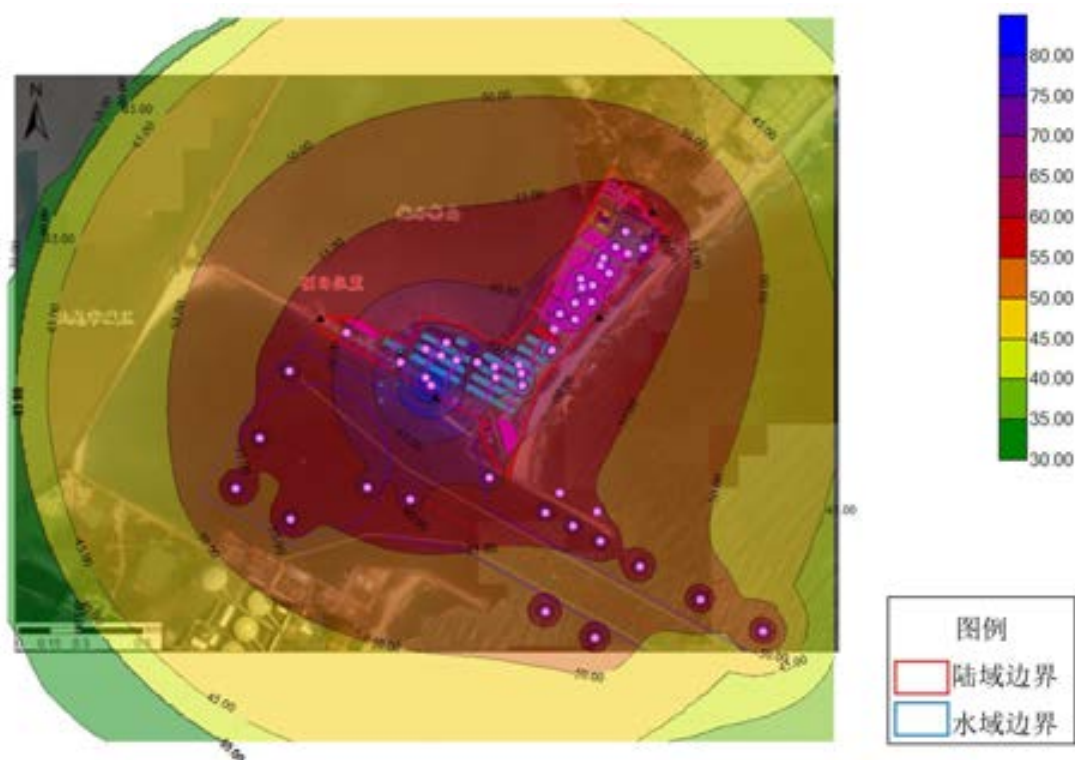
图 6.1-2 本项目昼间施工噪声贡献值等值线图
