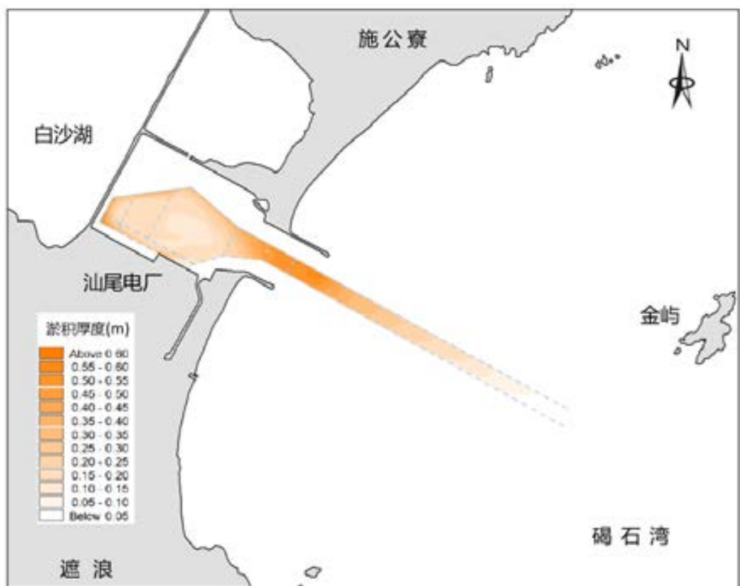
图 4.2-4 现状港池航道年淤积分布图
