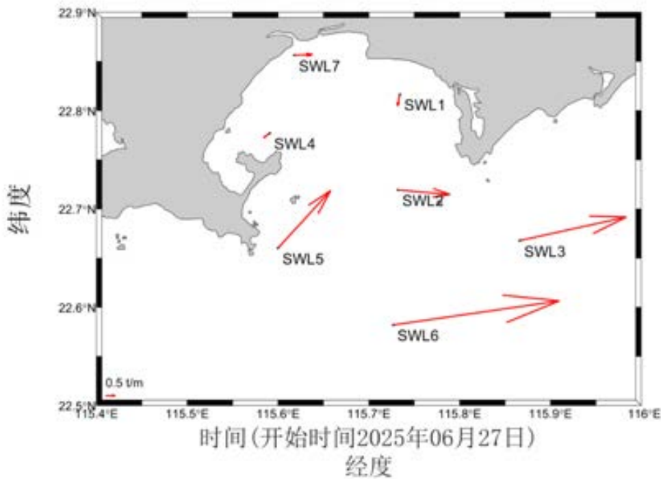
图 5.1-20 各站净输沙示意图
