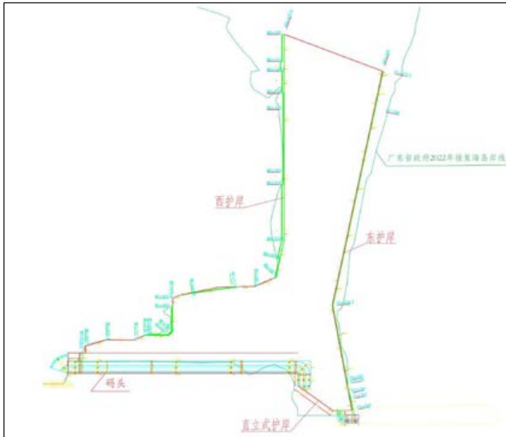
图 3.1-22 本项目码头及护岸平面布置图
