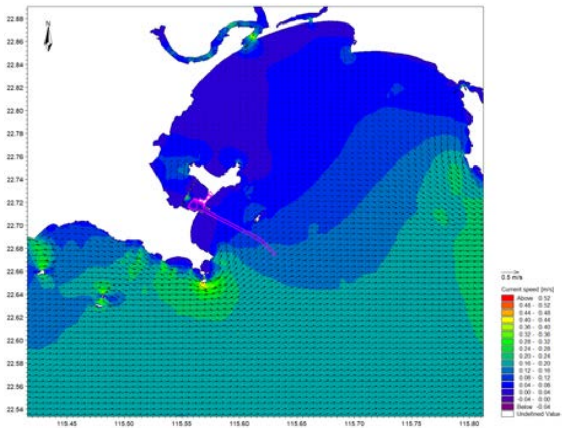
图 6.2-14 项目周边海域大潮落急流场图（表层）
