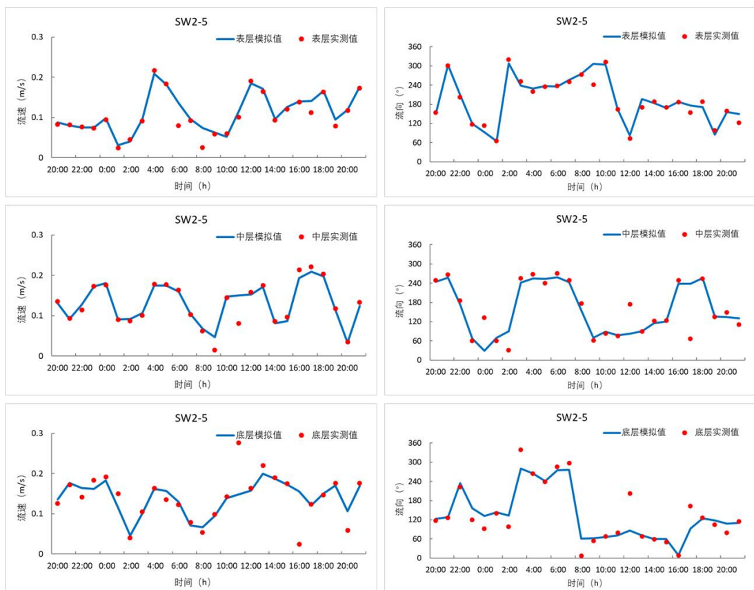
图 6.2-9 SW2-5 站流速和流向验证图（表、中、底层）
