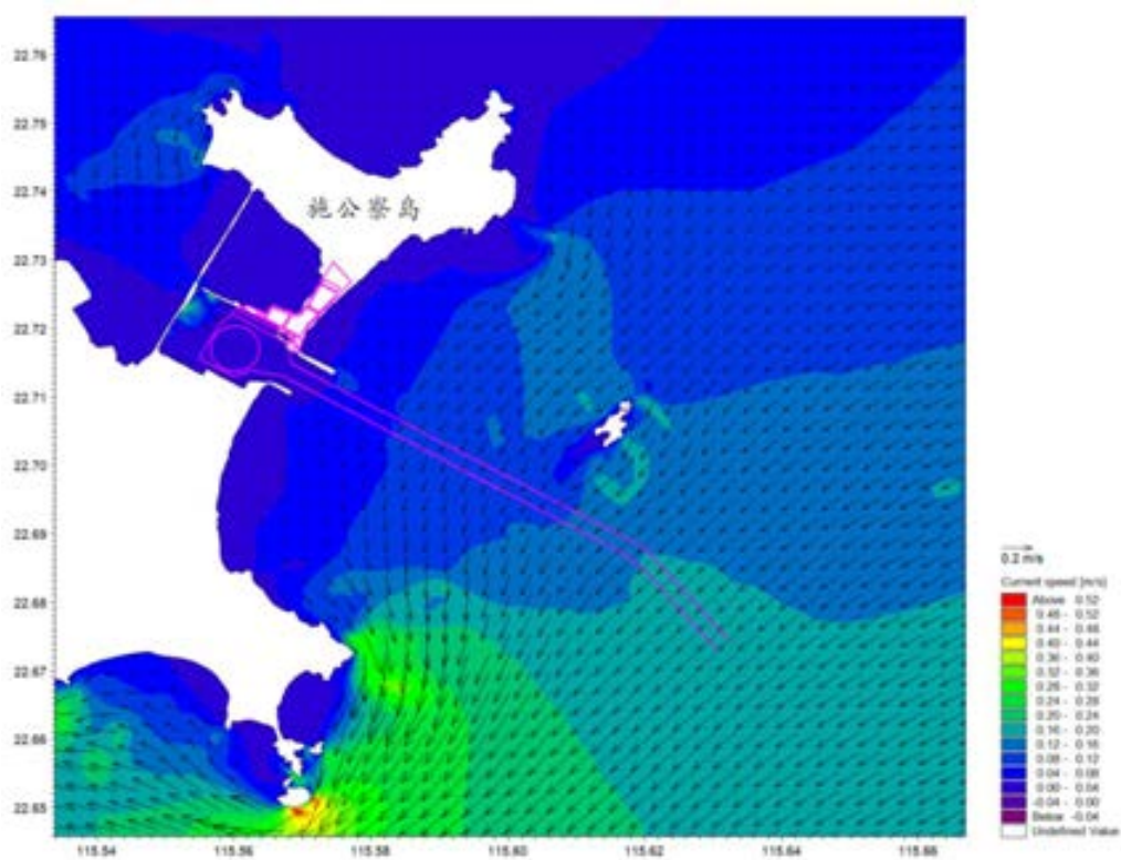
图 6.2-17 项目附近海域大潮涨急流场图（表层）
