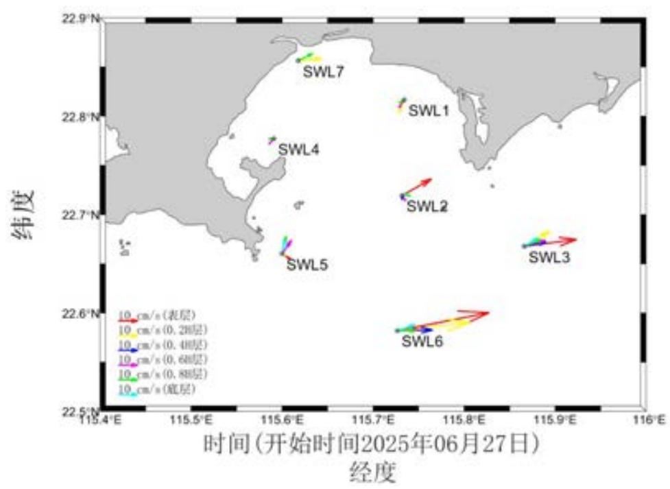
图 5.1-17 观测期各站余流分布图
