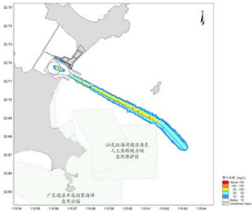
图 6.2-42 典型工况一产生悬沙增量包络线（表层）
