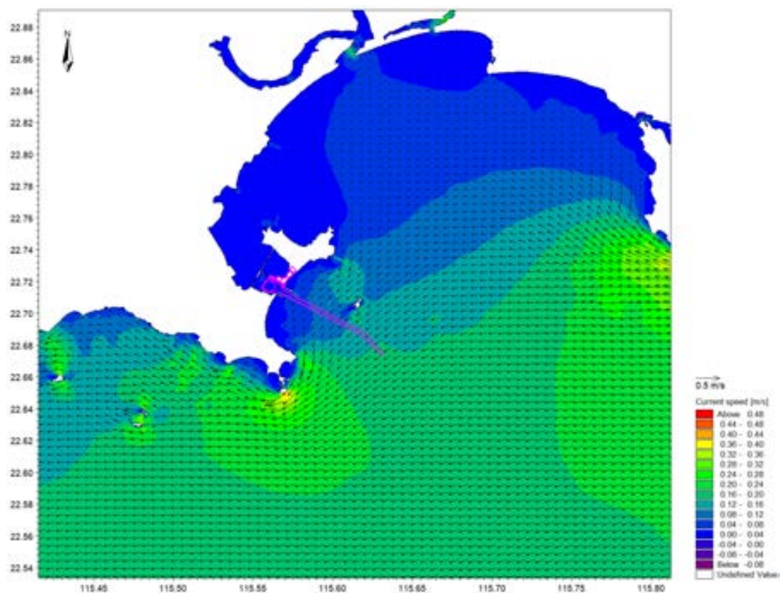
图 6.2-12 项目周边海域大潮涨急流场图（中层）
