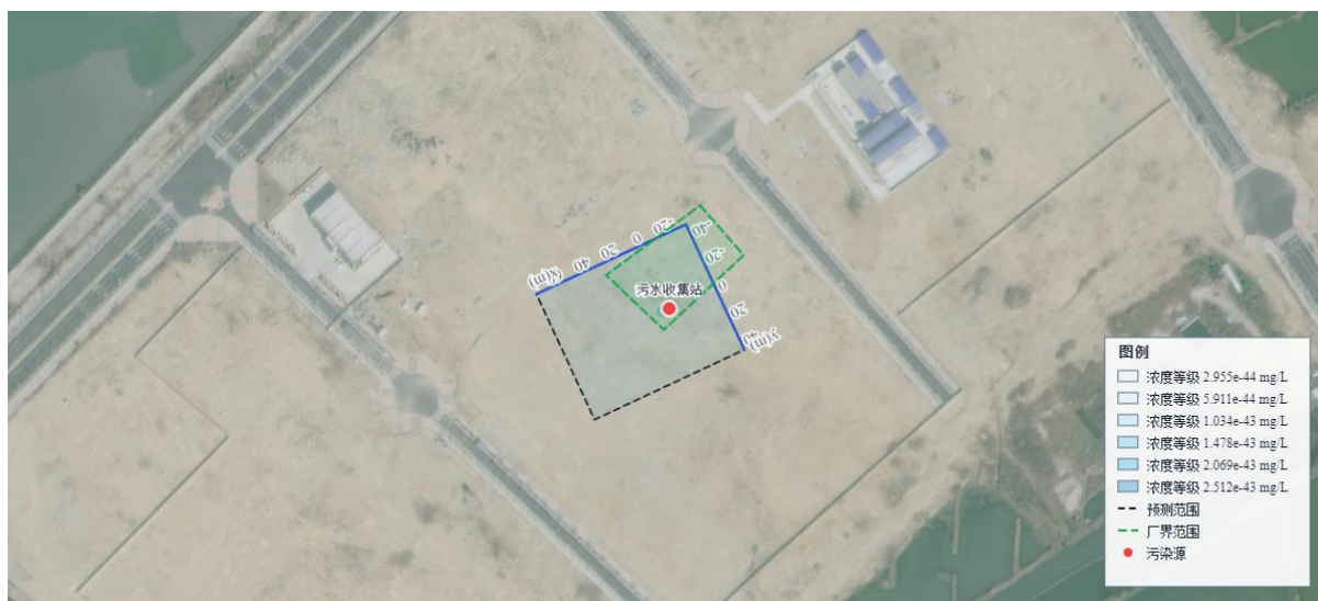
图 6.5.3-11 污水收集站-铬 t=100 d 浓度等值线图
