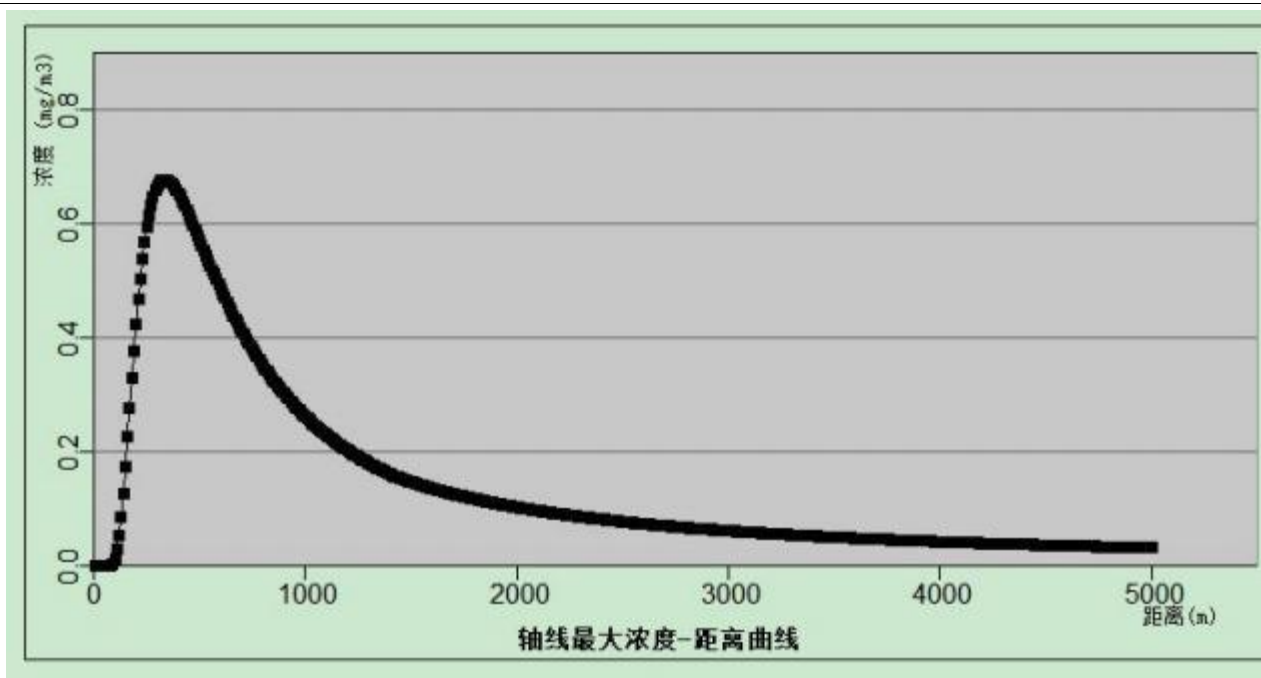
氰化氢轴线最大浓度结果图 图 7.5-1 污染物轴线最大浓度结果图
