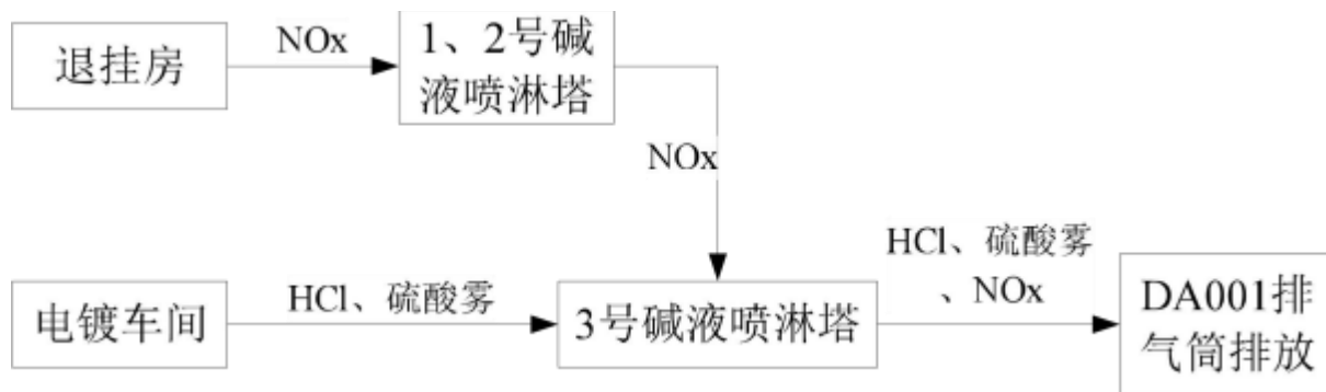
图 8.1.1-1 TA001 碱液喷淋处理系统示意图
