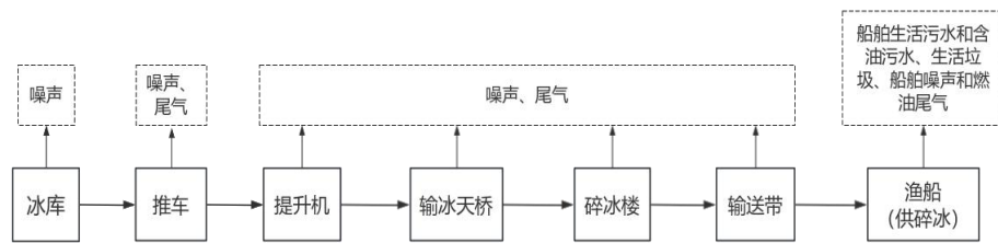
图 3.1.2-3 渔港供冰泊位装卸工艺产污环节
