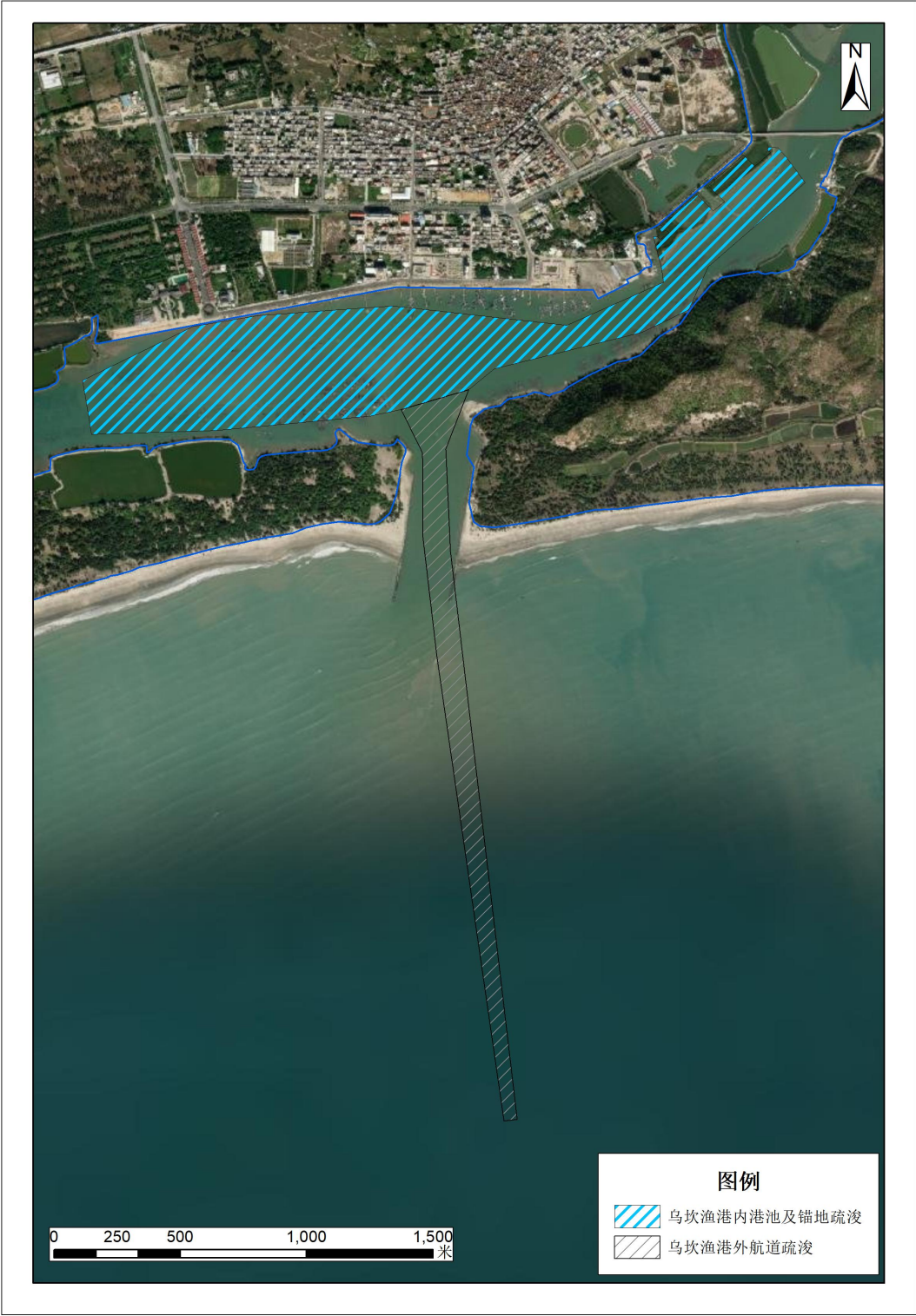
图 2.3.4-2a 乌坎渔港内港池及锚地、乌坎渔港外航道疏浚范围示意图
