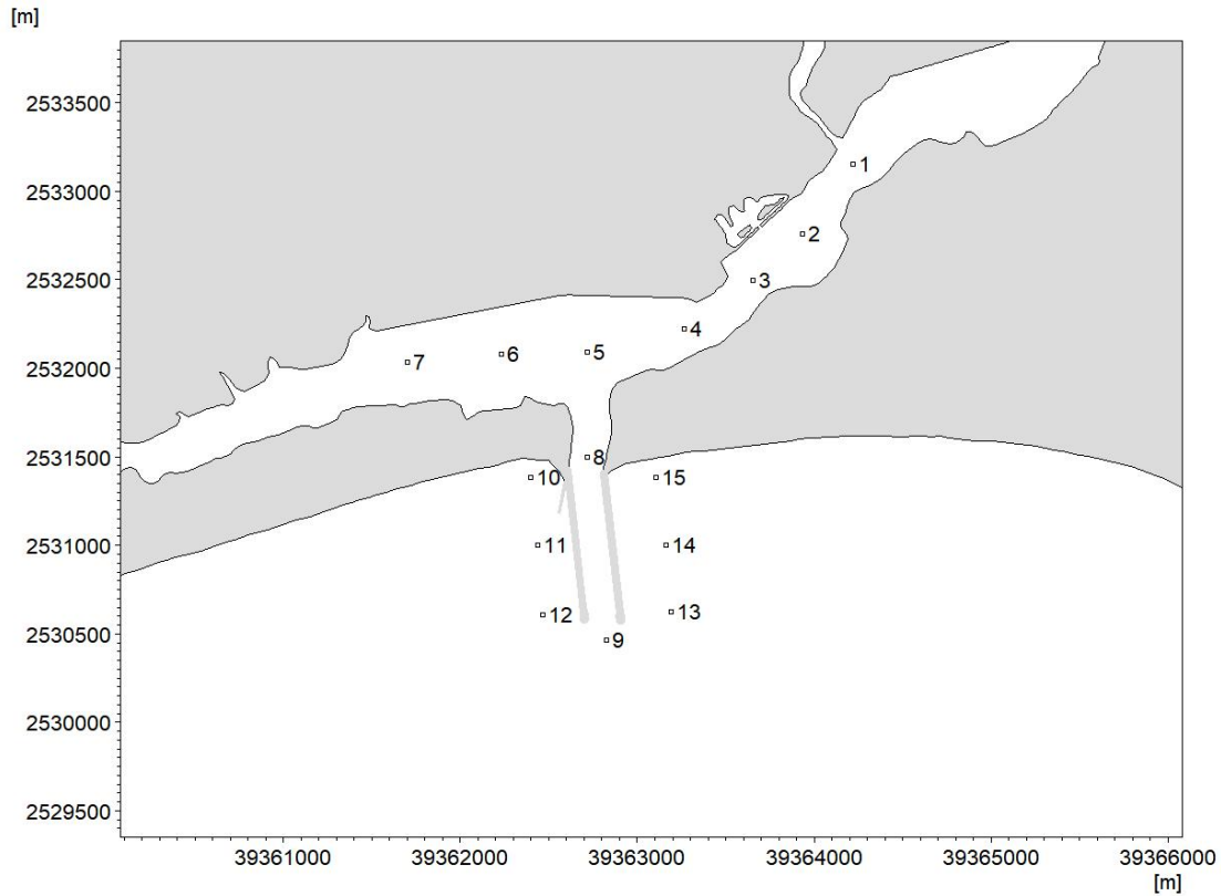
图 6.3.1-13 流速特征点位置
