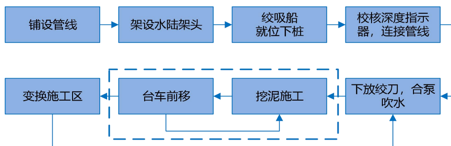
图 2.7.3-10 绞吸挖泥船施工工艺流程图
