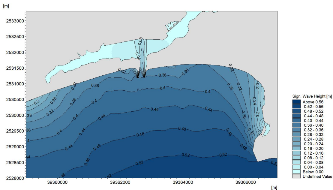
图 6.3.4-7a SSE 向工程前有效波高波浪场分布
