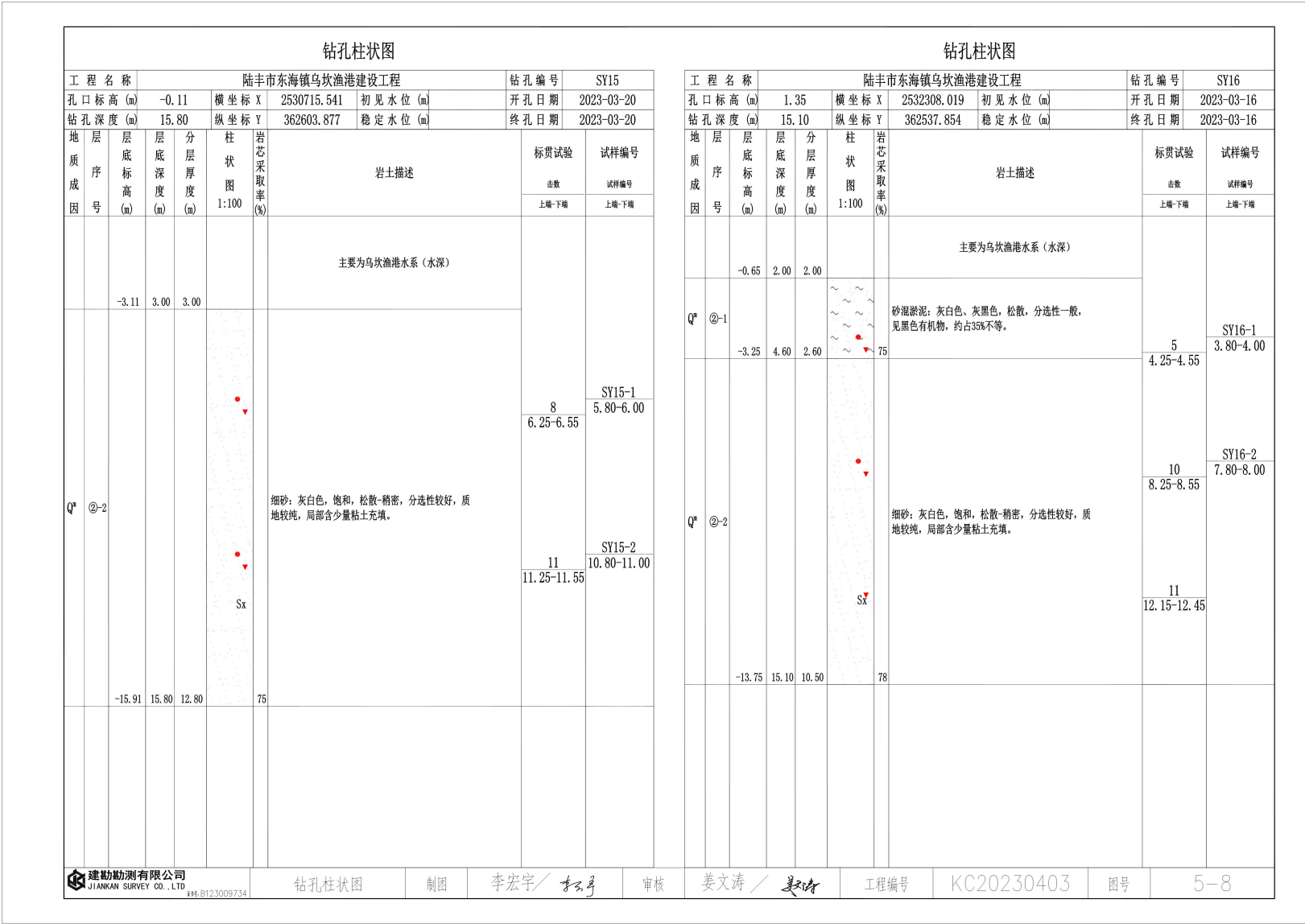
图 5.3.2-10 钻孔柱状图 (锚地)
