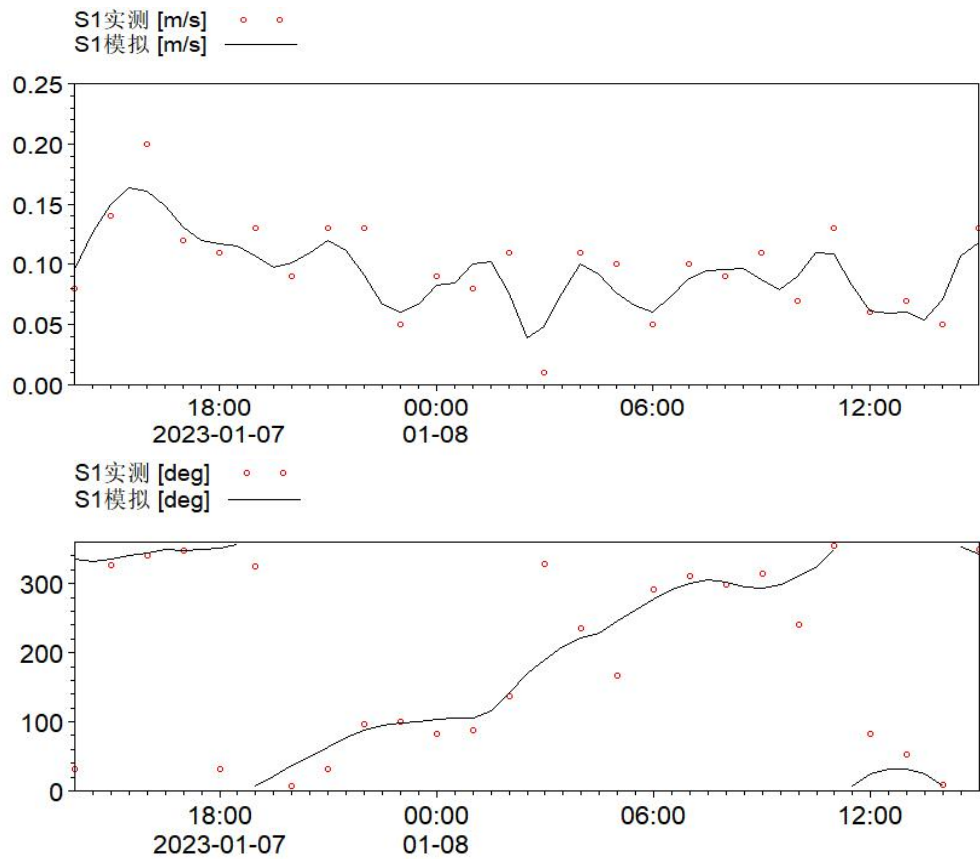
图 4.3.1-6a S1 站位流速流向验证图（2023 年 1 月 7 日—1 月 8 日）
