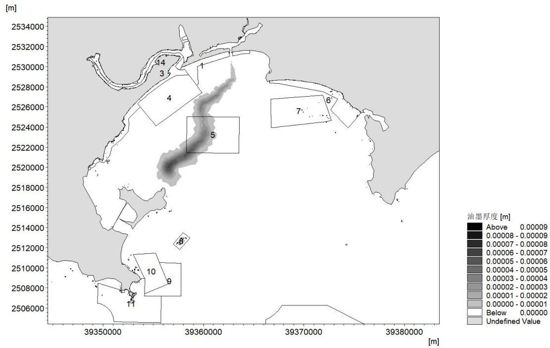
图 7.2.3-3a N 向平均风速落潮时溢油 48h 后最大扫海范围图
