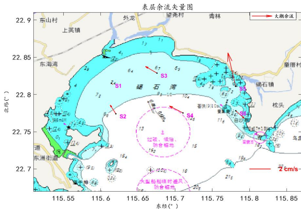
图 5.3.1-13 各站位表层矢量图
