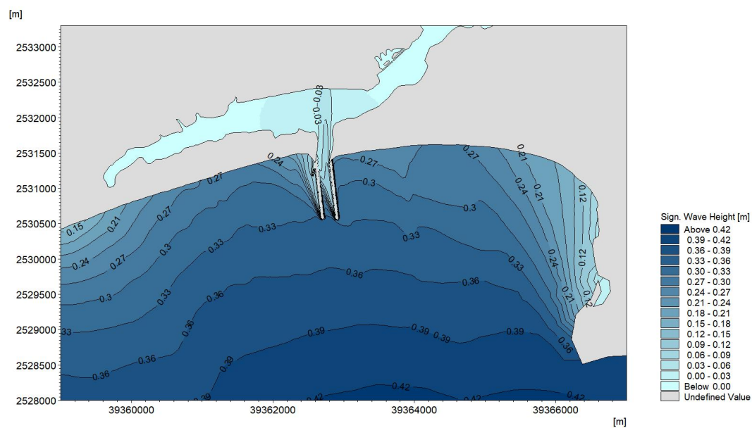
图 6.3.4-6b SE 向工程后有效波高波浪场分布 (2) SSE 向波浪场变化
