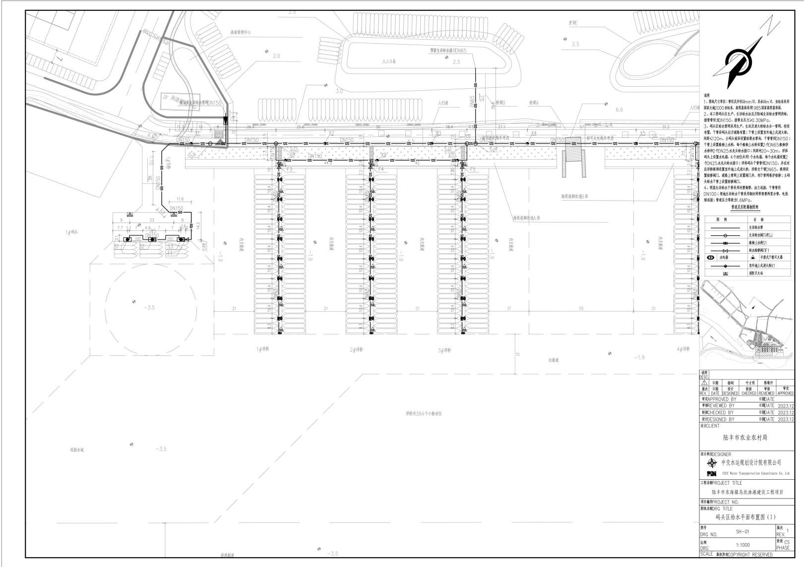
图 2.4.4-1a 码头区给水平面布置图
