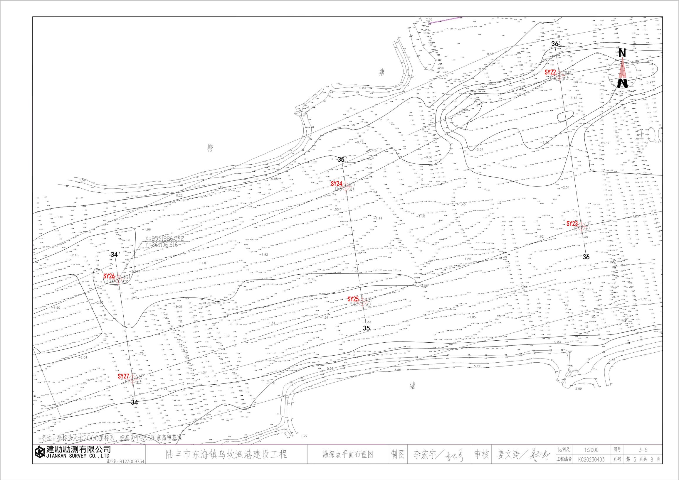
图 5.3.2—2d 地质勘察钻孔平面布置图 (五)
