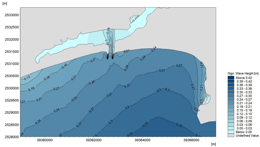
图 6.3.4-10a SW 向工程前有效波高波浪场分布
