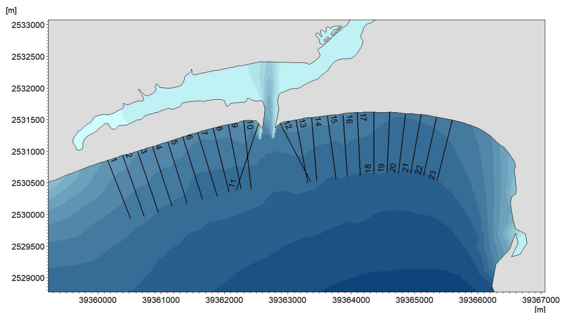
图 6.3.5-9 输沙断面示意图
