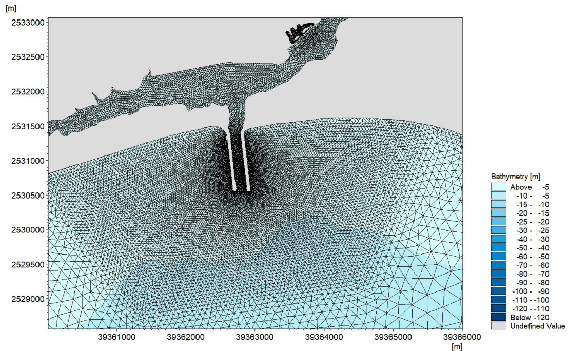
图 6.3.1-2b 工程后拦沙堤附近海域计算网格分布
