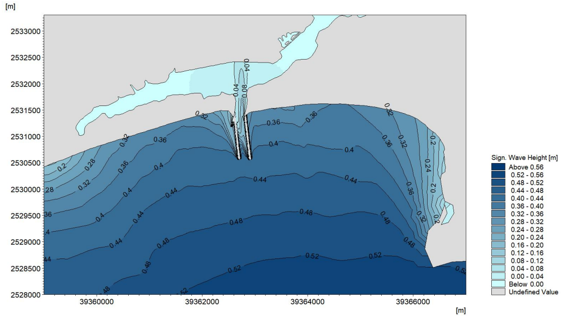
图 6.3.4-7b SSE 向工程后有效波高波浪场分布
