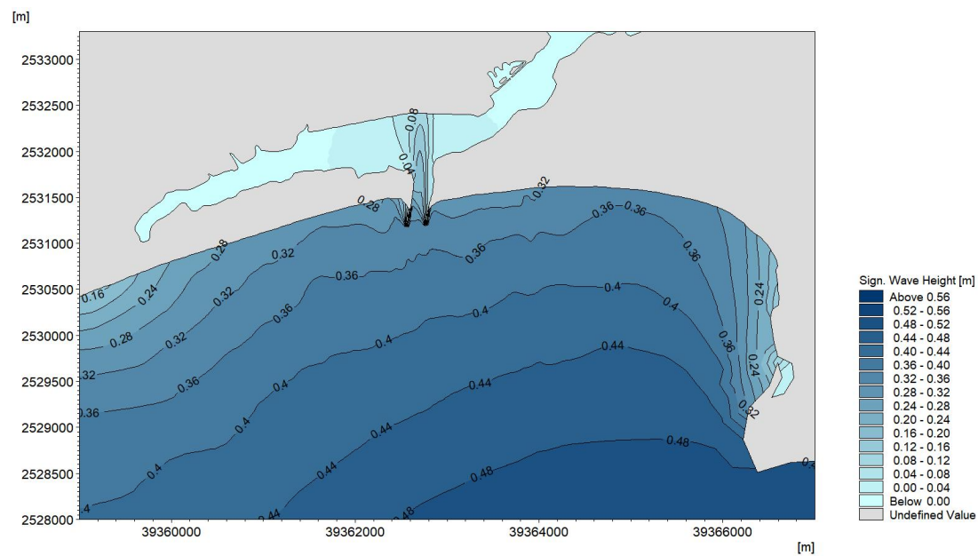
图 6.3.4-8a S 向工程前有效波高波浪场分布
