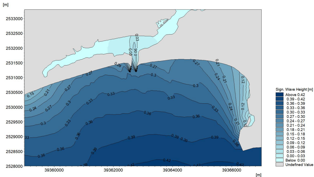
图 6.3.4-6a SE 向工程前有效波高波浪场分布
