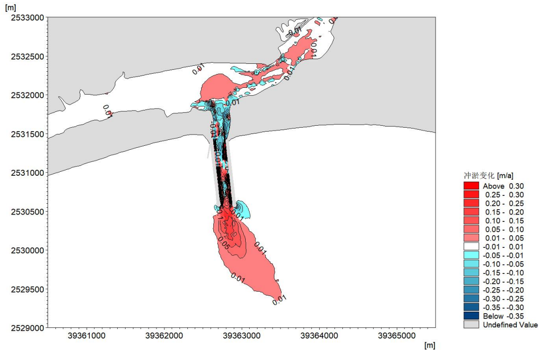
图 6.3.2-5 工程前冲淤环境
