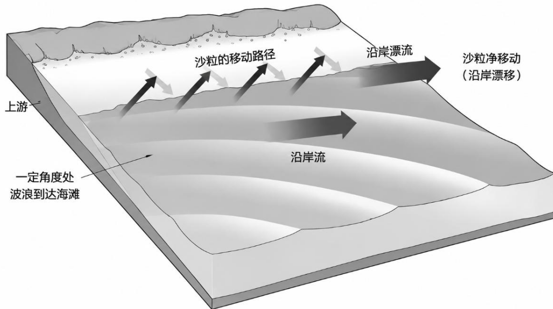
图 6.3.5-1 沿岸输沙示意图
