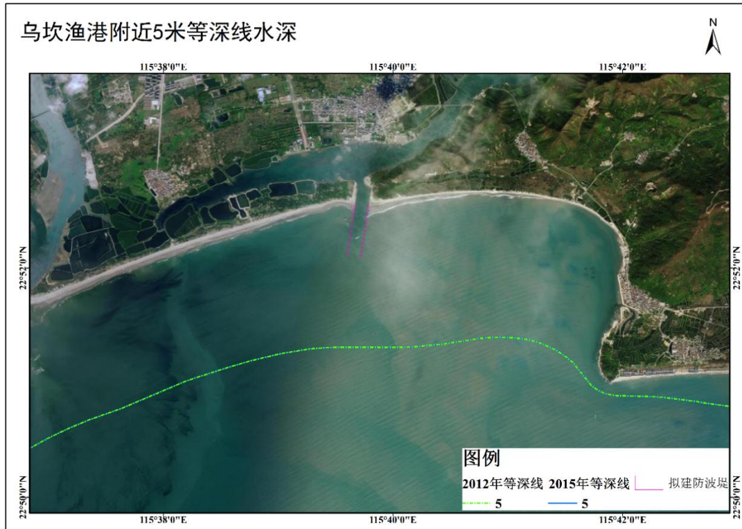
图 6.3.2-4 乌坎渔港附近海域 5 米等深线变化
