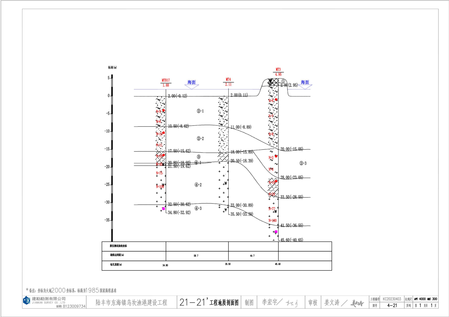
图 5.3.2-5 地质剖面图 (港池)
