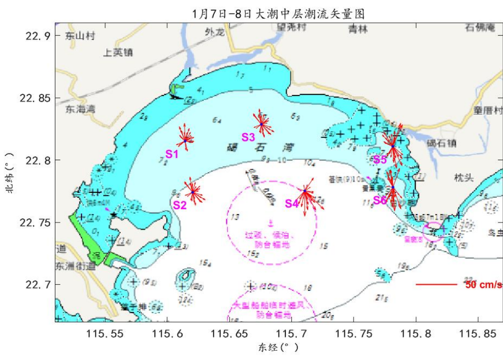
图 5.3.1-10 各站位中层潮流矢量图
