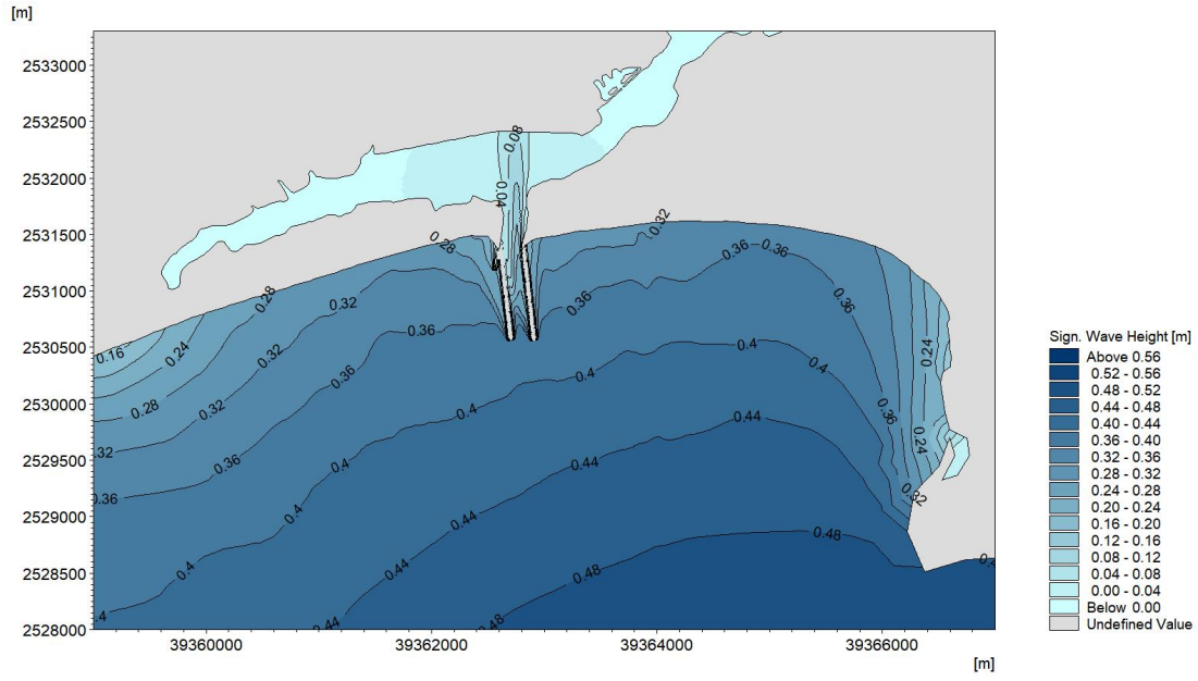
图 6.3.4-8b S 向工程后有效波高波浪场分布
