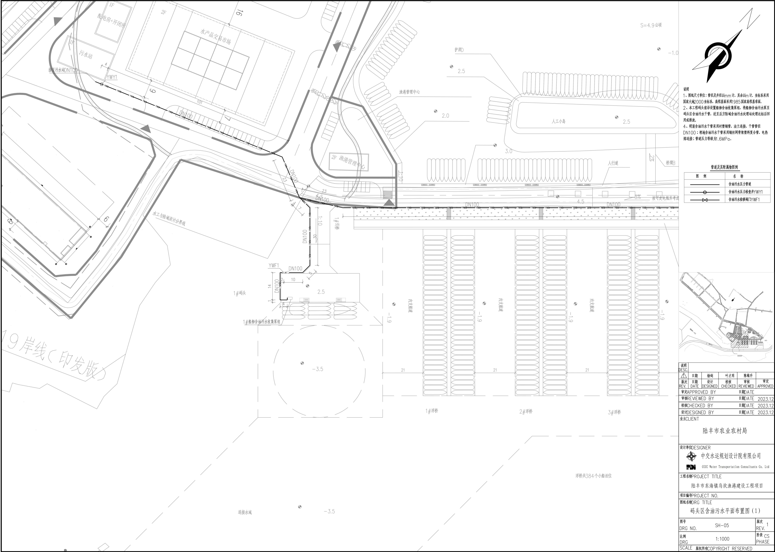
图 2.4.4-3 码头区含油污水平面布置图（一）
