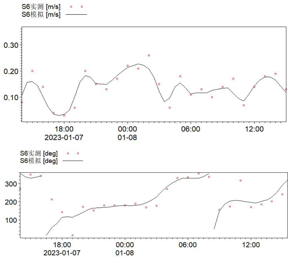
图 4.3.1-6f S6 站位流速流向验证图（2023 年 1 月 7 日—1 月 8 日）
