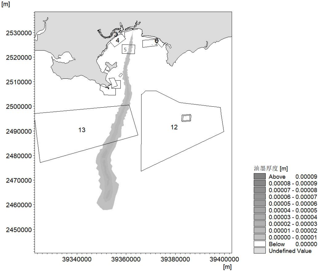
图 7.2.3-6a N 向不利风速涨潮时溢油 48h 后最大扫海范围图
