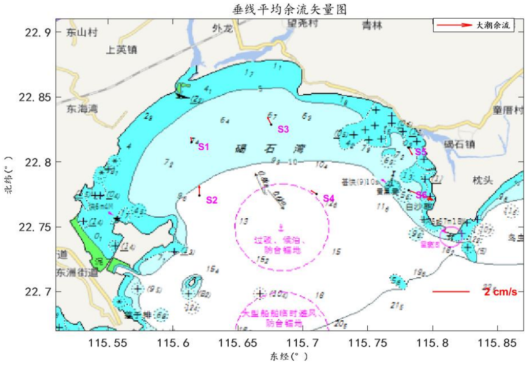
图 5.3.1-16 各站位垂线平均矢量图
