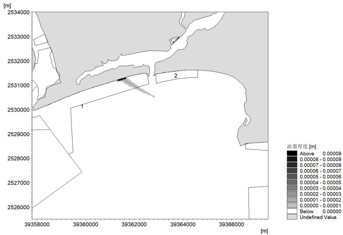
图 7.2.3-4a E 向平均风速涨潮时溢油 48h 后最大扫海范围图
