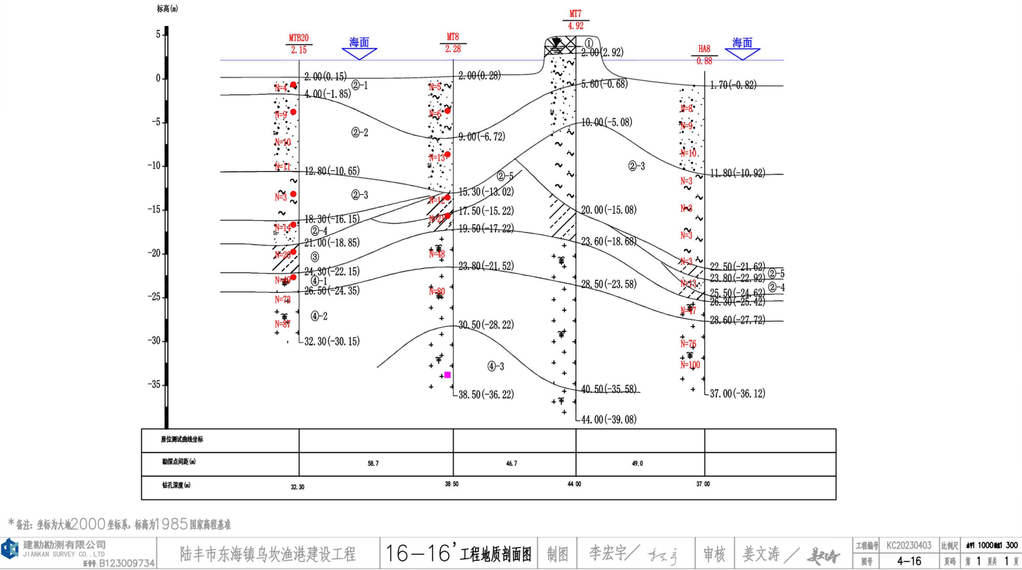
图 5.3.2-4 地质剖面图（内支航道）
