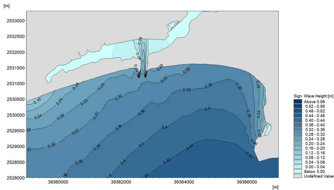
图 6.3.4-9a SSW 向工程前有效波高波浪场分布
