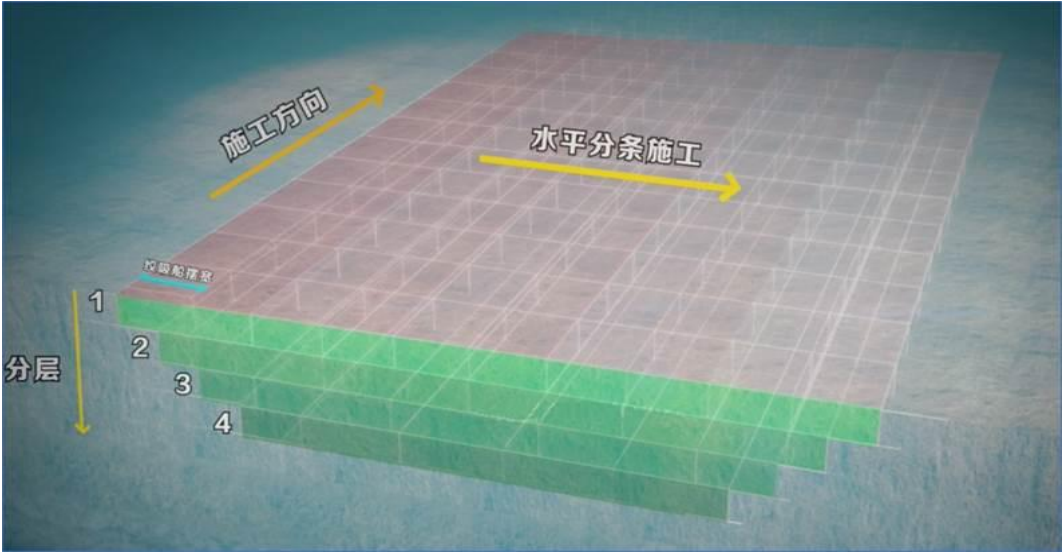
图 2.3.3-12 绞吸挖泥船分层分条施工示意图
