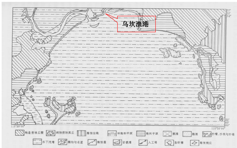
图 4.1.5-1 碣石湾地貌类型分布图
