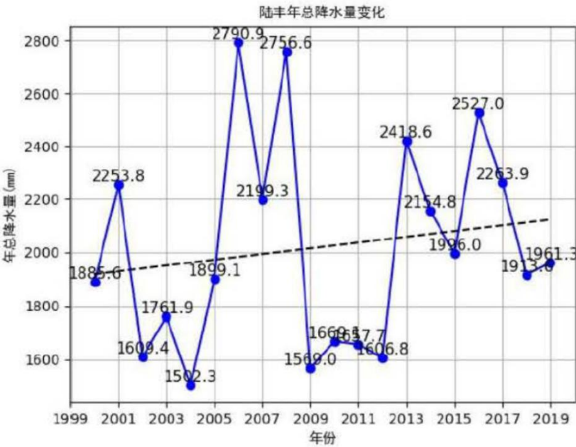
图 4.1.1-4 陆丰（2000-2020）年总降水量（单位：毫米，虚线为趋势线）
