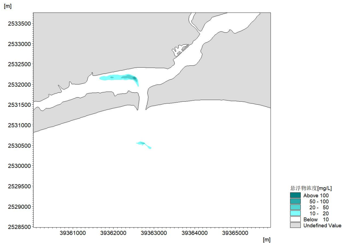
图 6.3.3-5b 疏浚施工（典型工况）悬浮泥沙扩散范围
