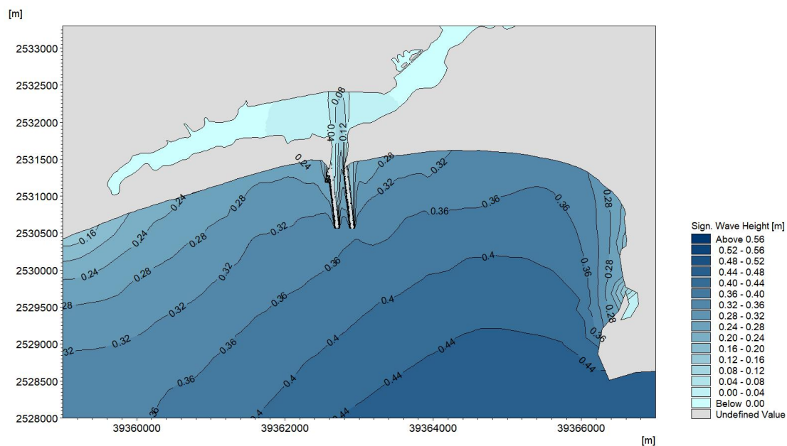
图 6.3.4-9b SSW 向工程后有效波高波浪场分布
