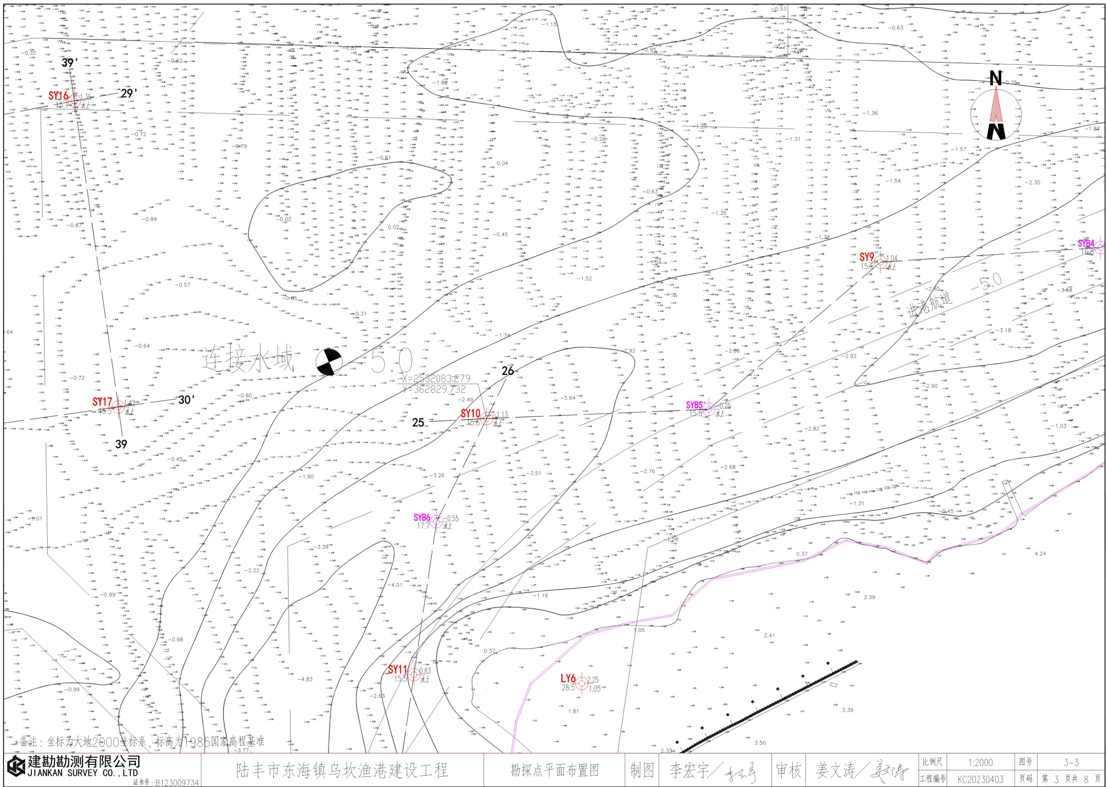
图 5.3.2-2b 地质勘察钻孔平面布置图（三）
