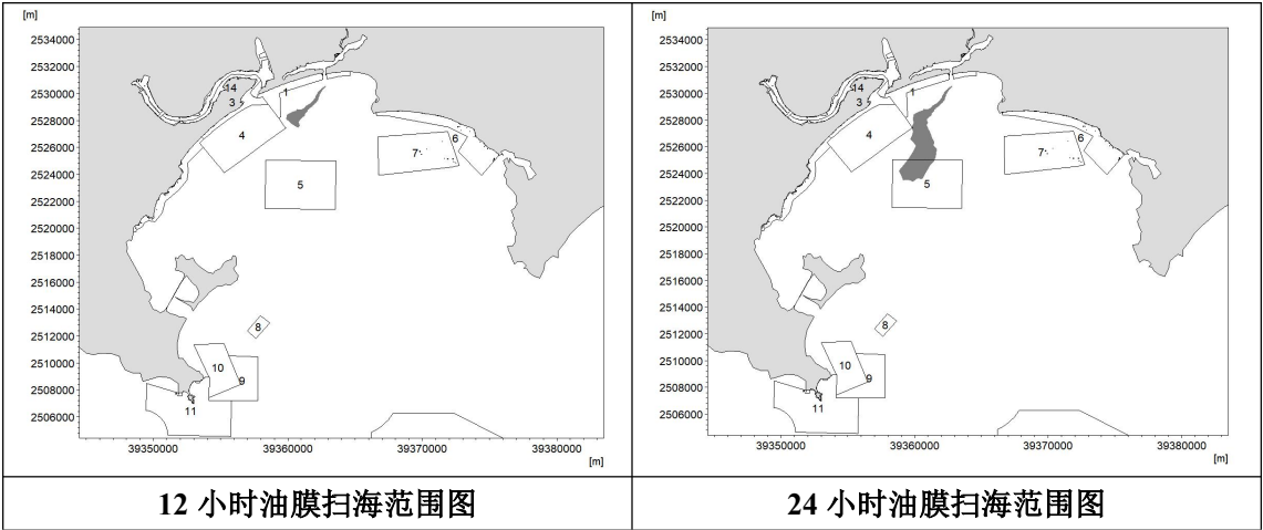
图 7.2.3-2b N 向平均风速涨潮时溢油 12h、24h 后扫海范围图
