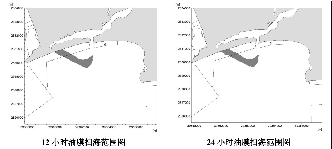
图 7.2.3-4b E 向平均风速落潮时溢油 12h、24h 后扫海范围图
