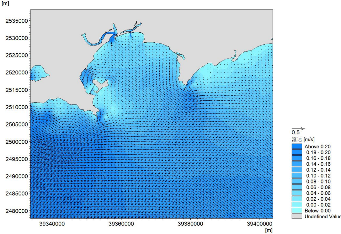
图 6.3.1-7b 工程前落急时刻大范围海域流场图
