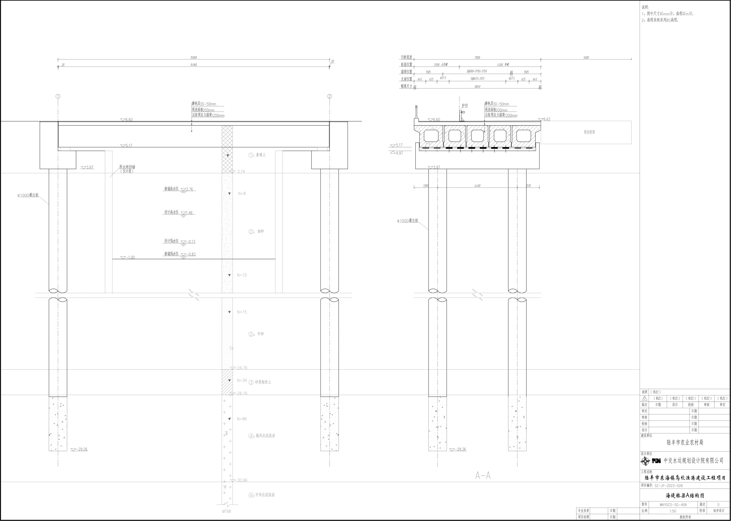
图 2.3.3-11b 海堤桥梁 A 断面图
