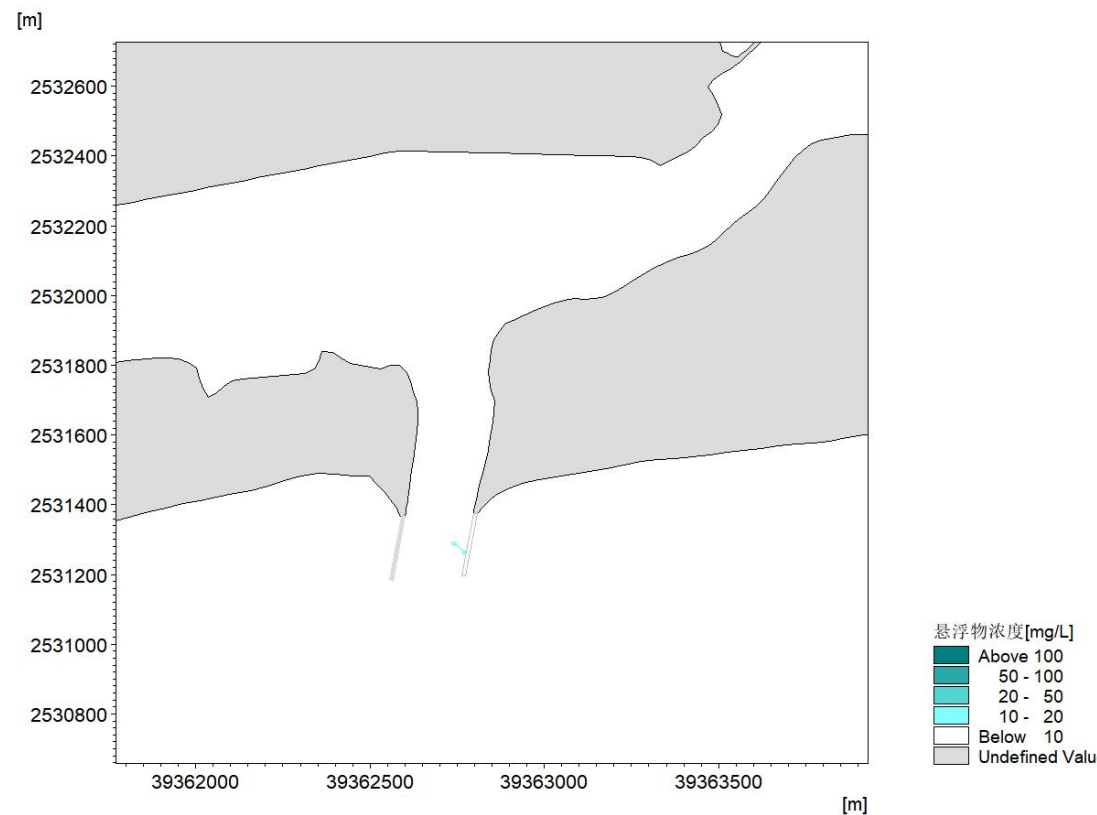
图 6.3.3-3a 东导堤拆除施工悬浮物影响范围
