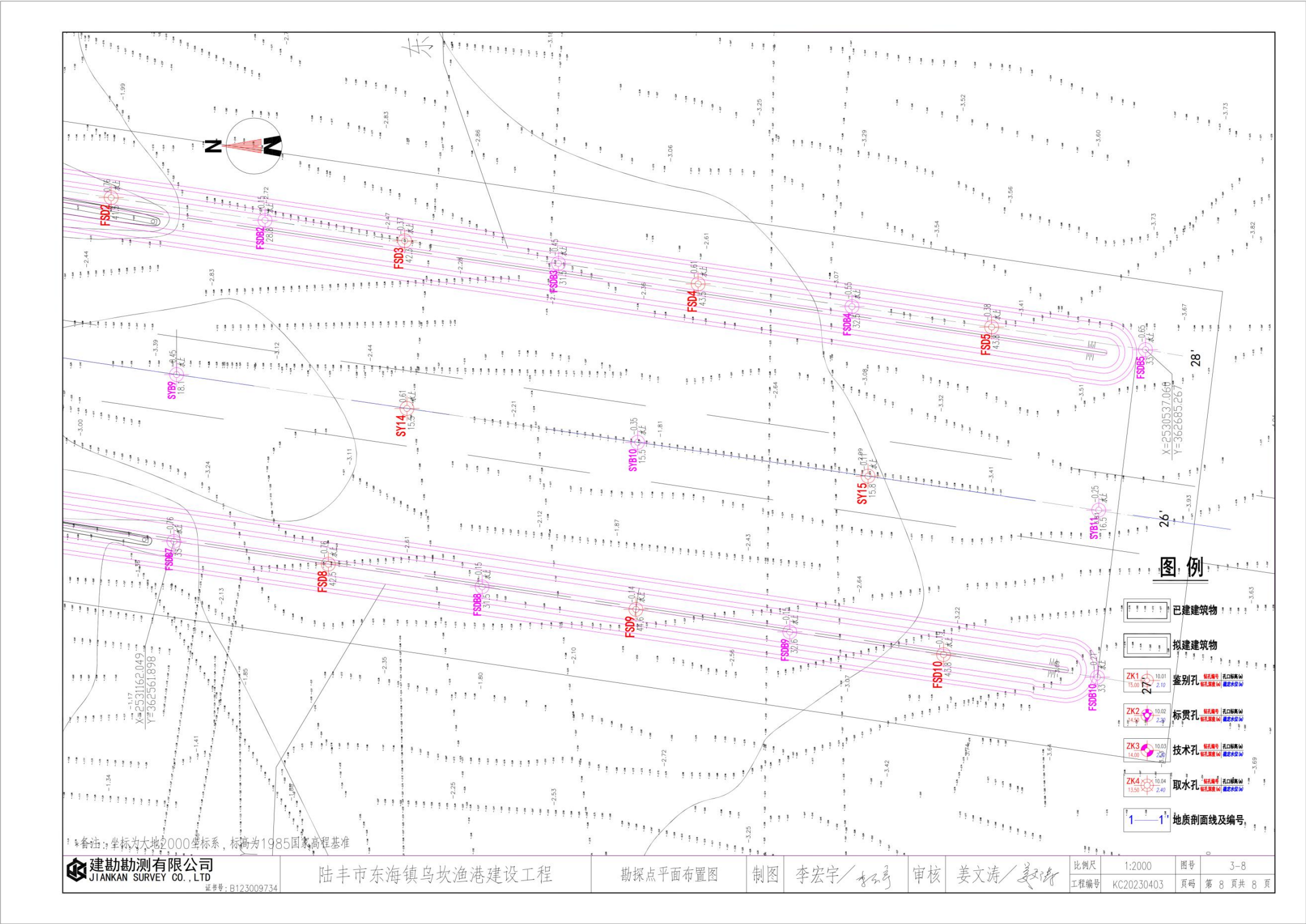
图 5.3.2—2g 地质勘察钻孔平面布置图（七）
