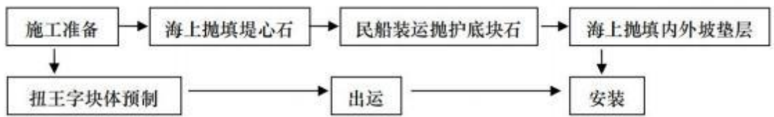
图 2.7.3-4 导堤施工工序
