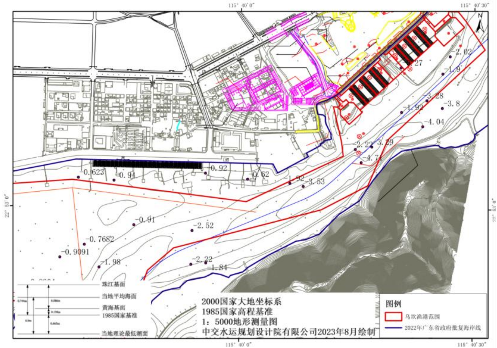
图 5.3.2-6a 项目所在海域水深地形图
