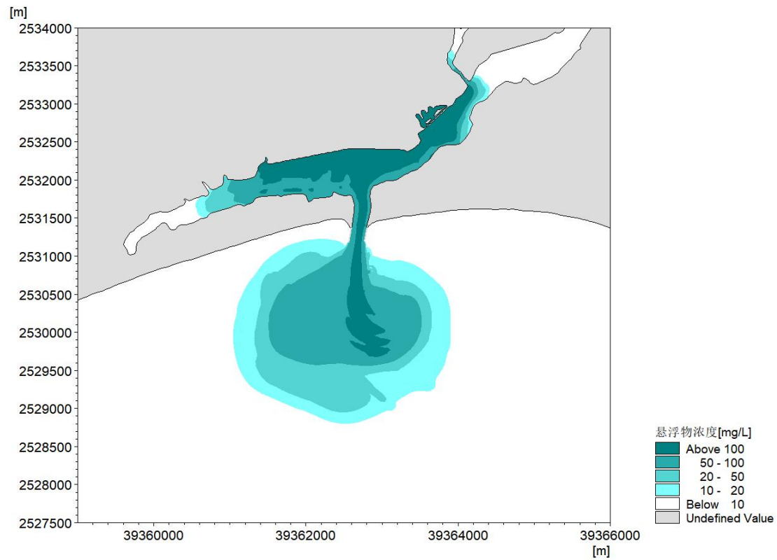
图 6.3.3-5a 疏浚施工悬浮泥沙扩散范围
