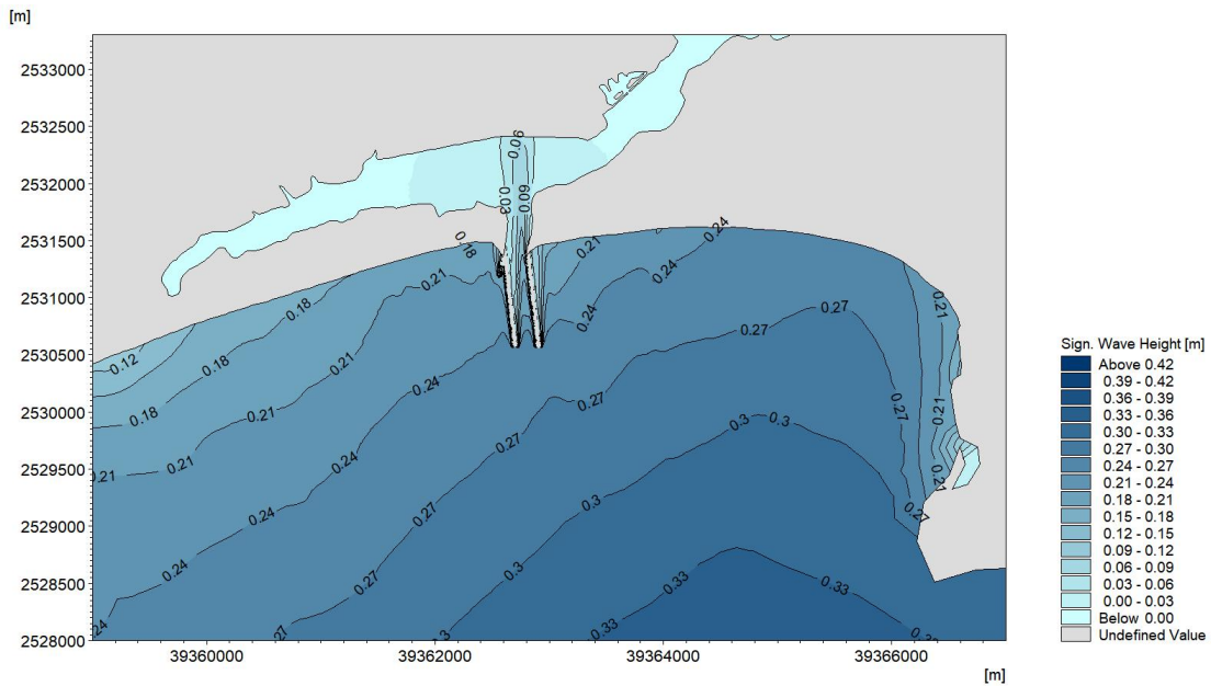
图 6.3.4-6b SW 向工程后有效波高波浪场分布
