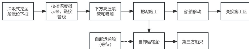
图 2.7.3-7 乌坎渔港外航道疏浚施工工艺流程图
