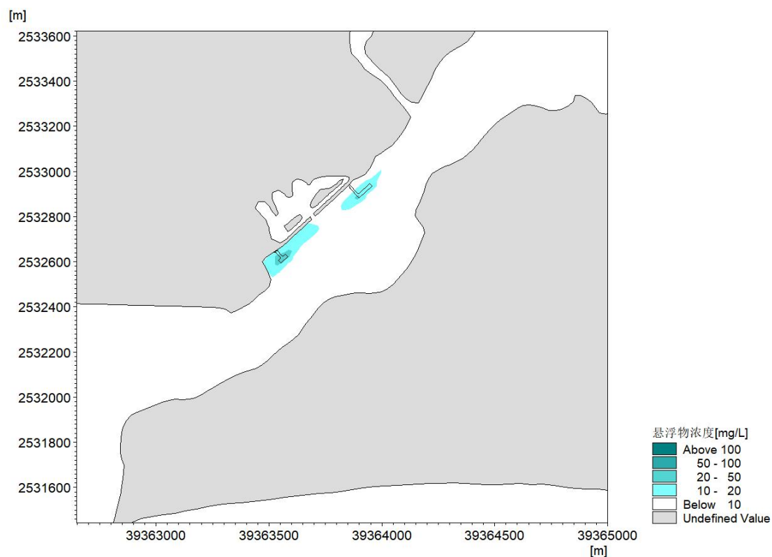
图 6.3.3-2a 码头施工悬浮物影响范围
