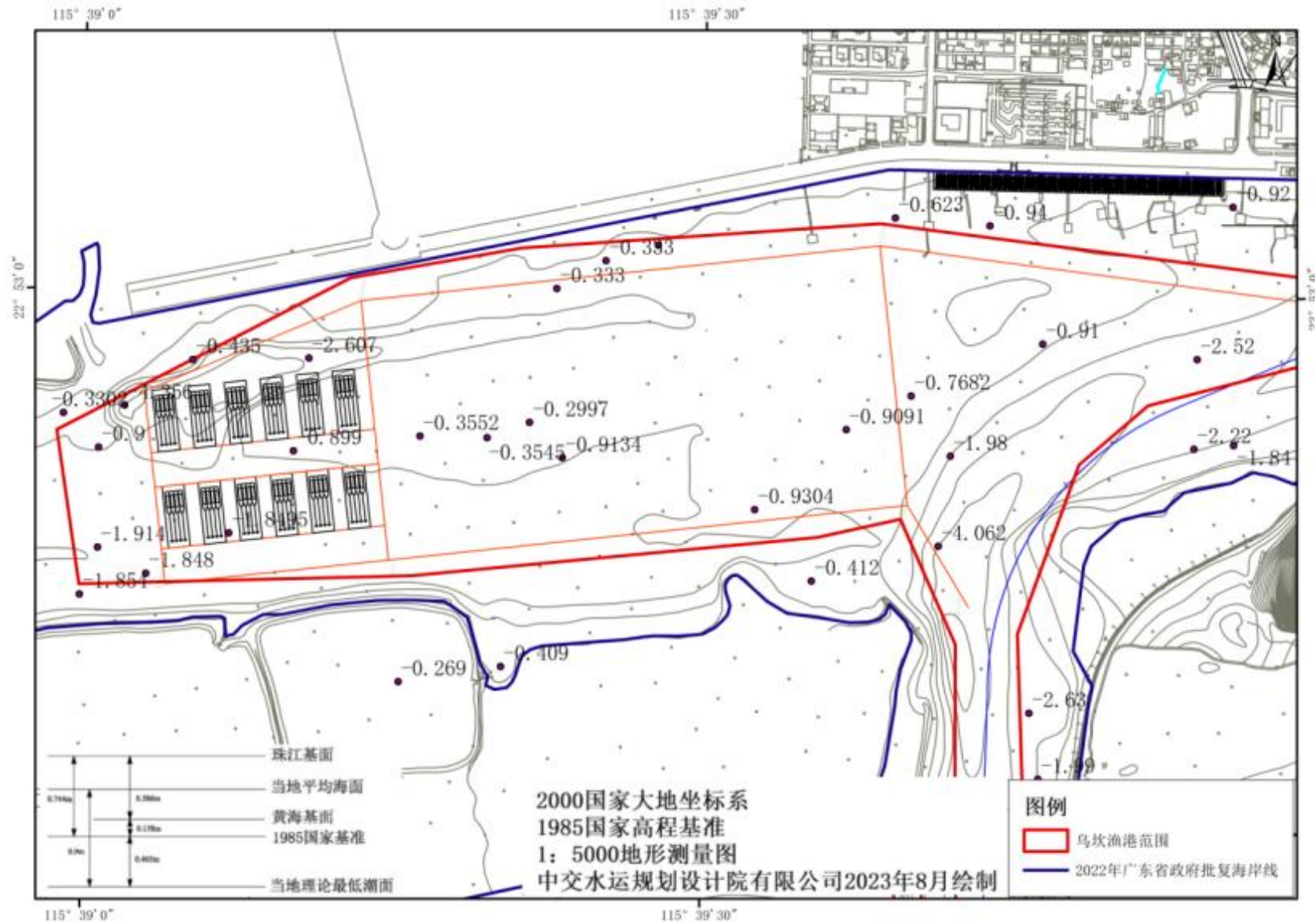
图 5.3.2-6b 项目所在海域水深地形图
