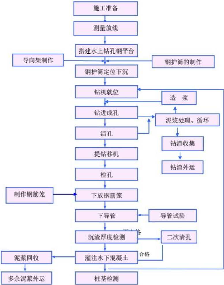
图 2.7.3-1 灌注桩施工工艺流程
