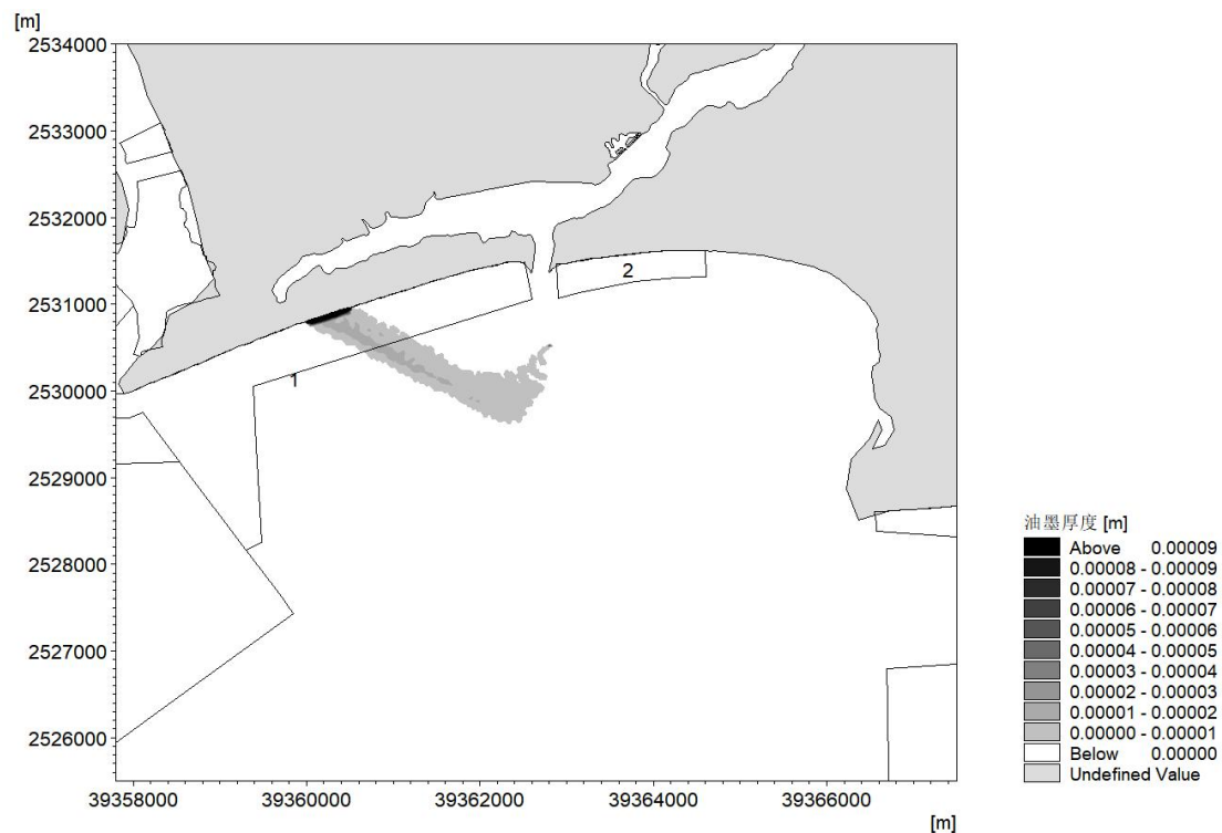
图 7.2.3-5a E 向平均风速落潮时溢油 48h 后最大扫海范围图
