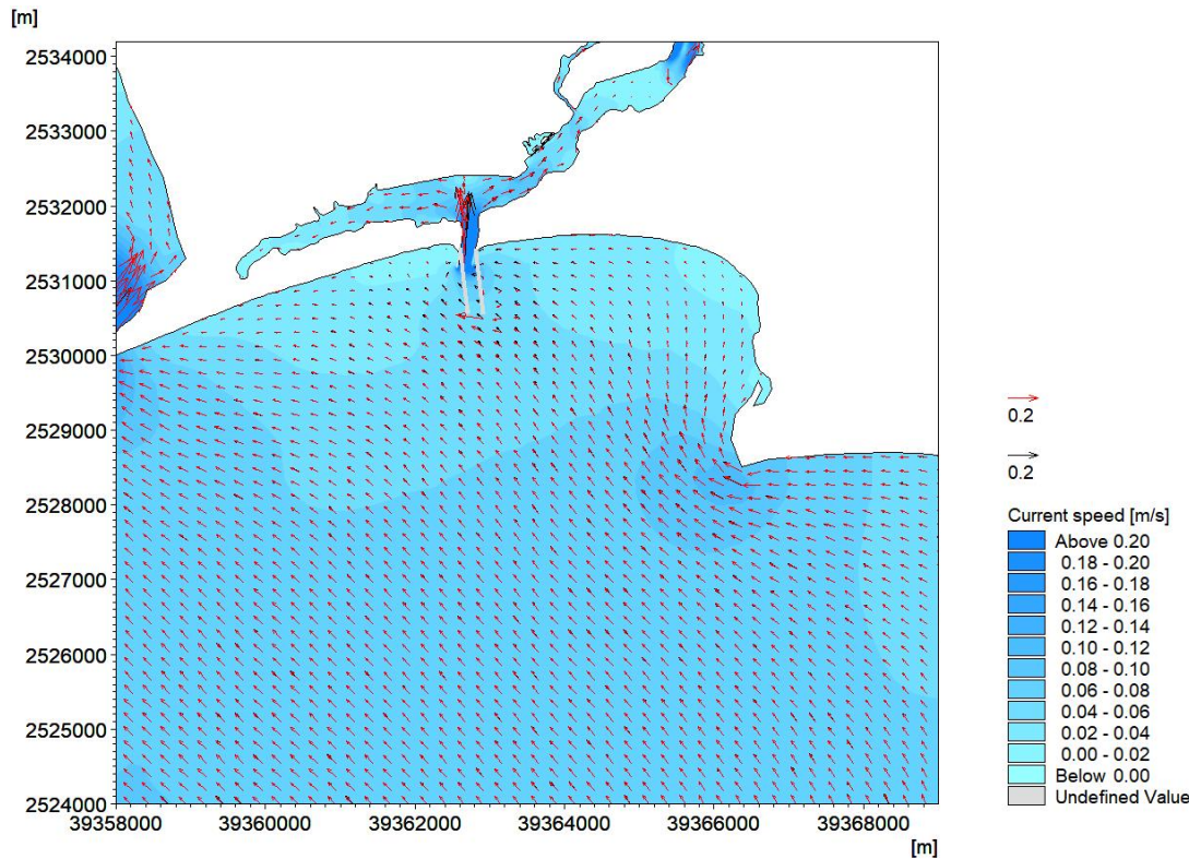
图 6.3.1-9b 工程后落急时刻工程附近海域流场图
