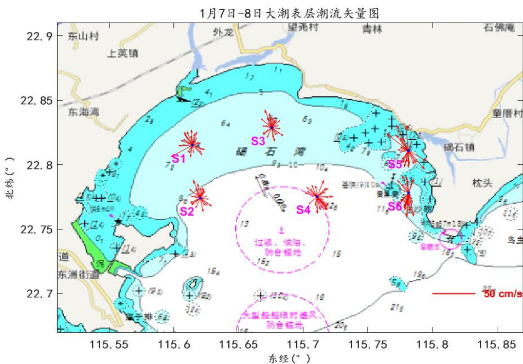
图 5.3.1-9 各站位表层潮流矢量图
