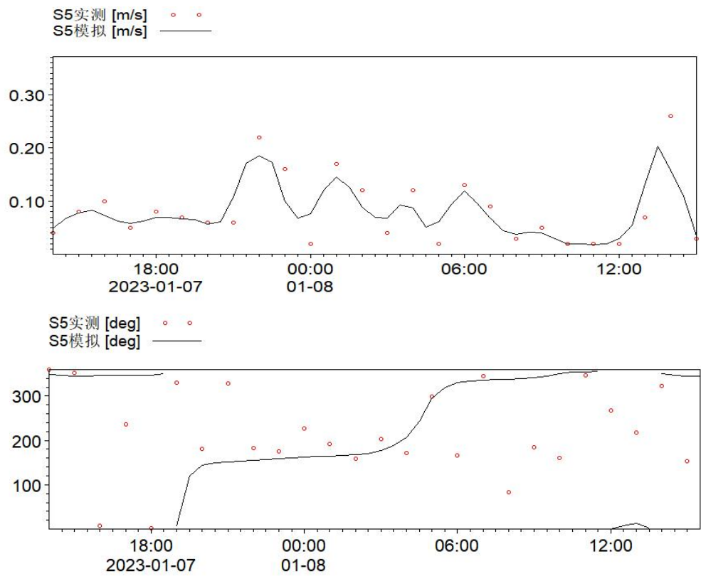
图 6.3.1-6e S5 站位流速流向验证图（2023 年 1 月 7 日—1 月 8 日）
