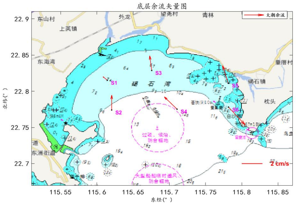
图 5.3.1-15 各站位底层矢量图
