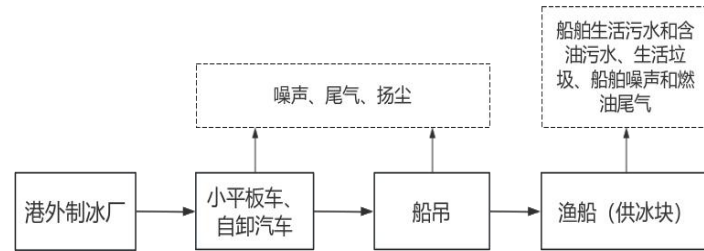
图 3.1.2-2 港外供冰泊位装卸工艺产污环节
