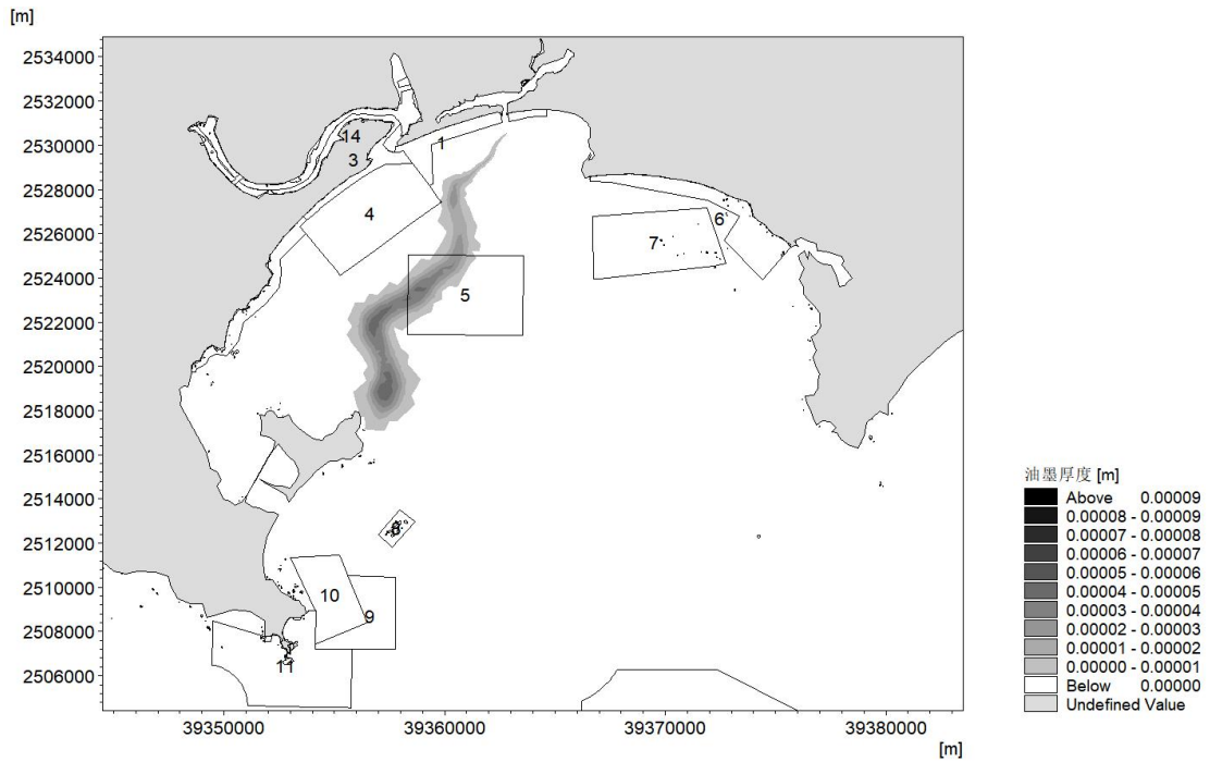
图 7.2.3-2a N 向平均风速涨潮时溢油 48h 后最大扫海范围图
