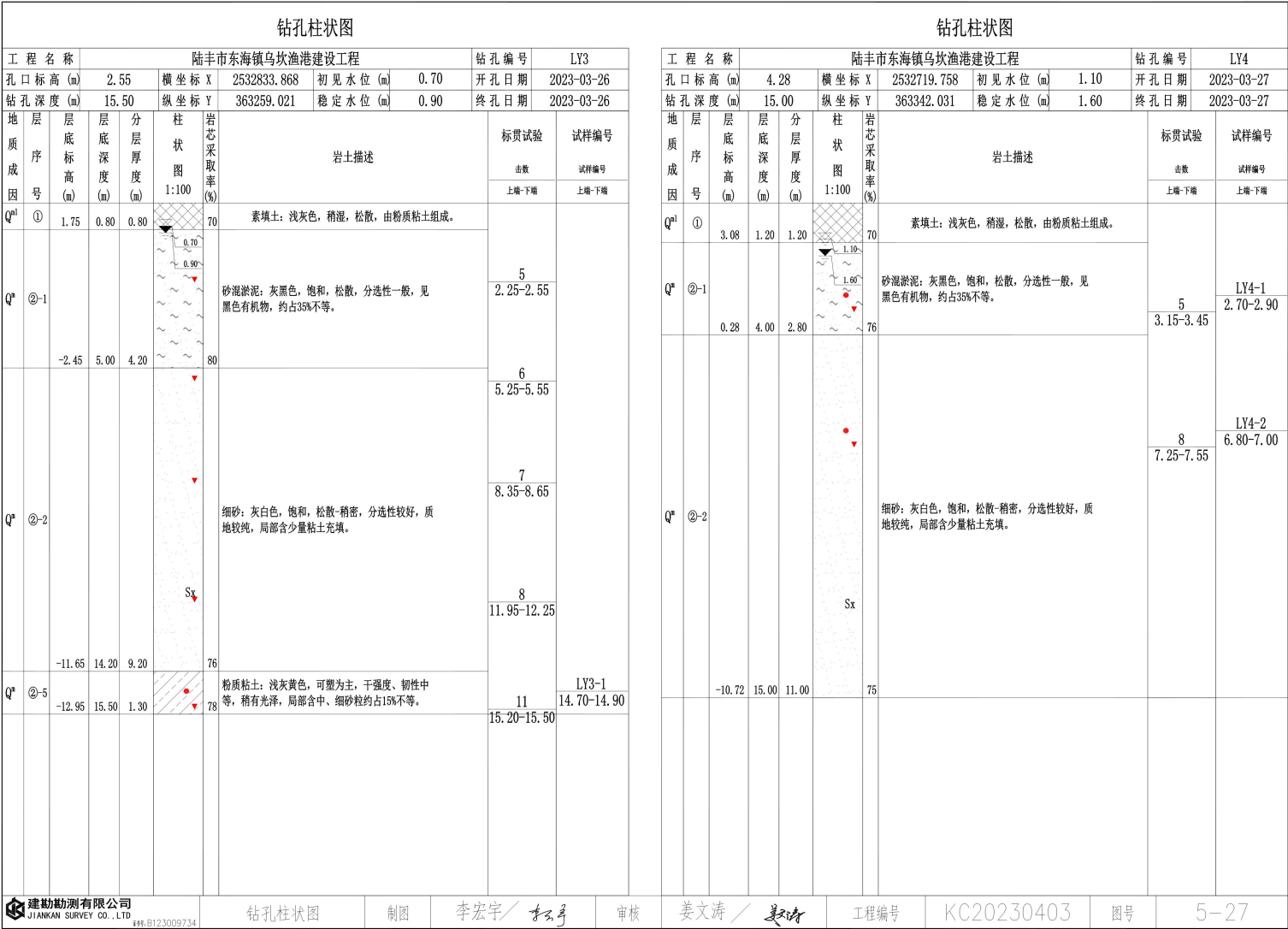
图 5.3.2-8 钻孔柱状图（港池、内航道）
