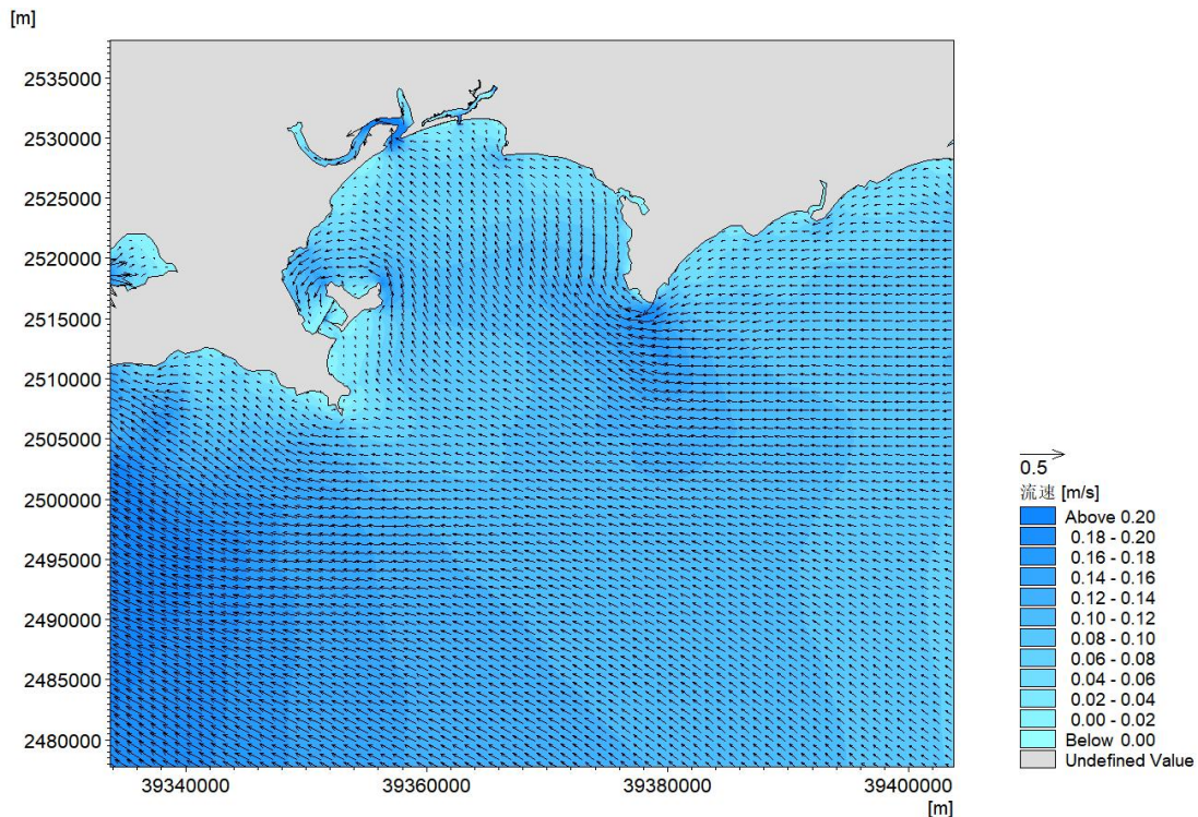
图 6.3.1-7a 工程前涨急时刻大范围海域流场图
