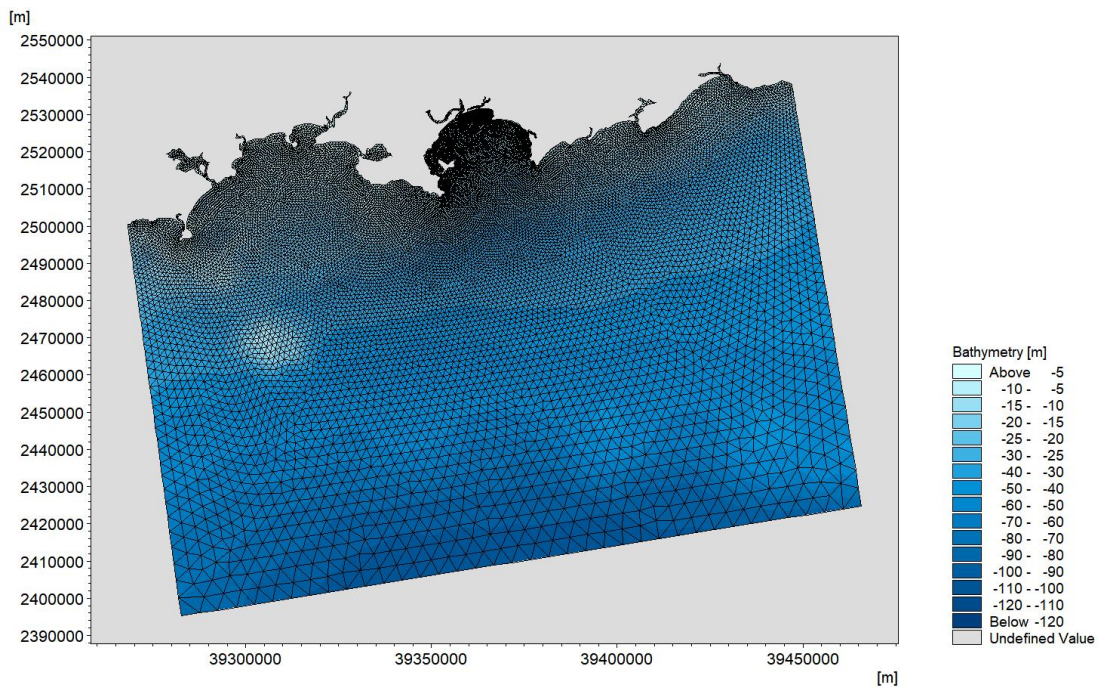
图 6.3.1-1 大海域计算范围和网格分布
