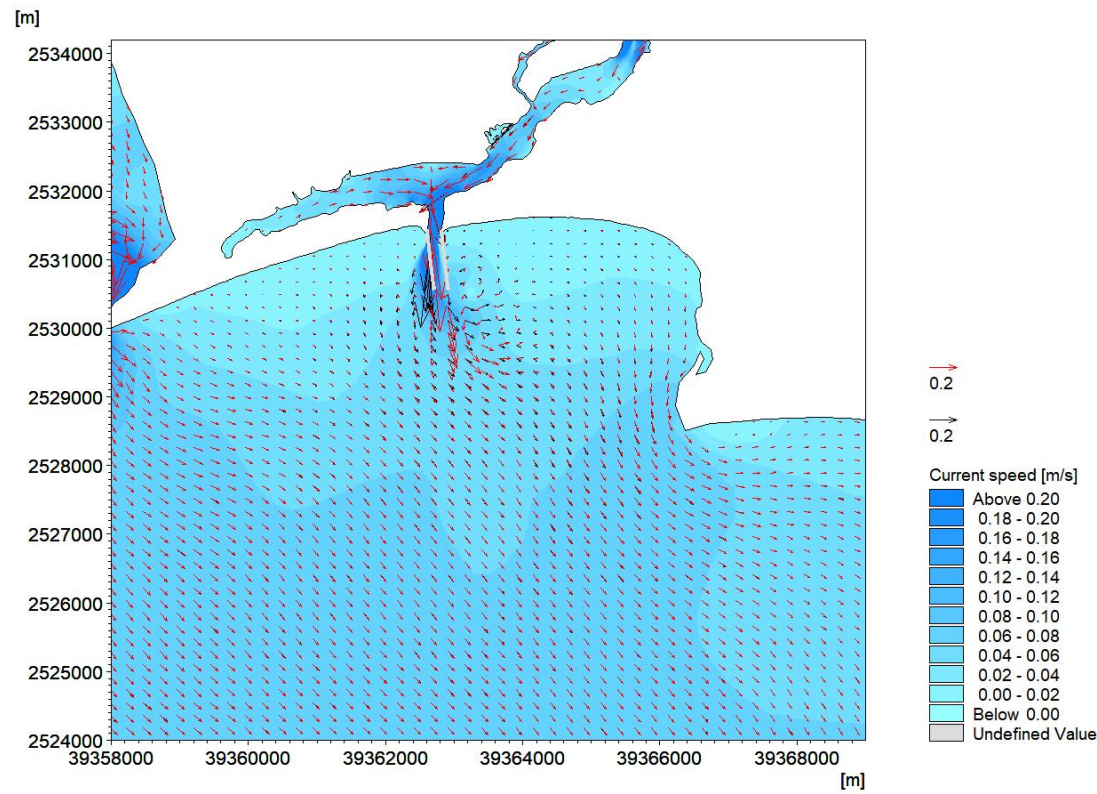
图 6.3.1-11a 工程前后落急流速变化图（黑色箭头：工程前，红色箭头：工程后）
