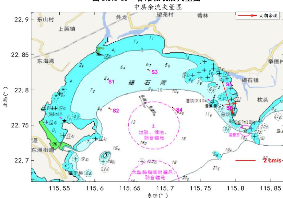
图 5.3.1-14 各站位中层矢量图
