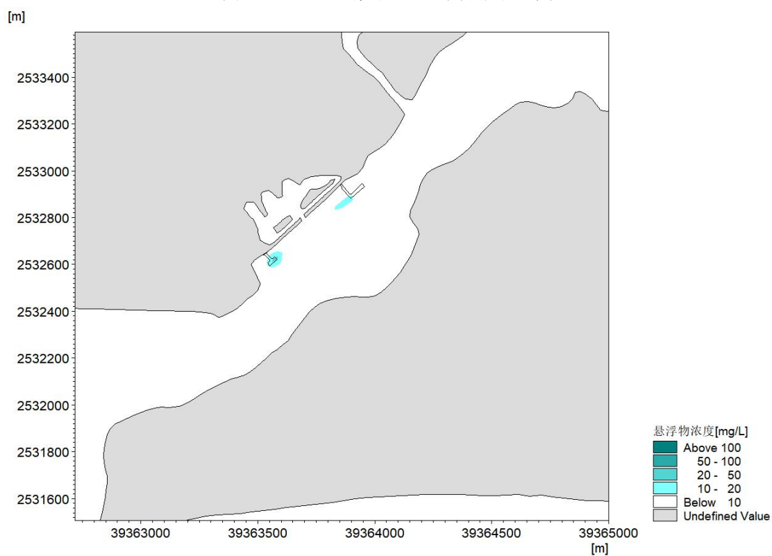
图 6.3.3-2b 码头施工典型工况悬浮物影响范围
