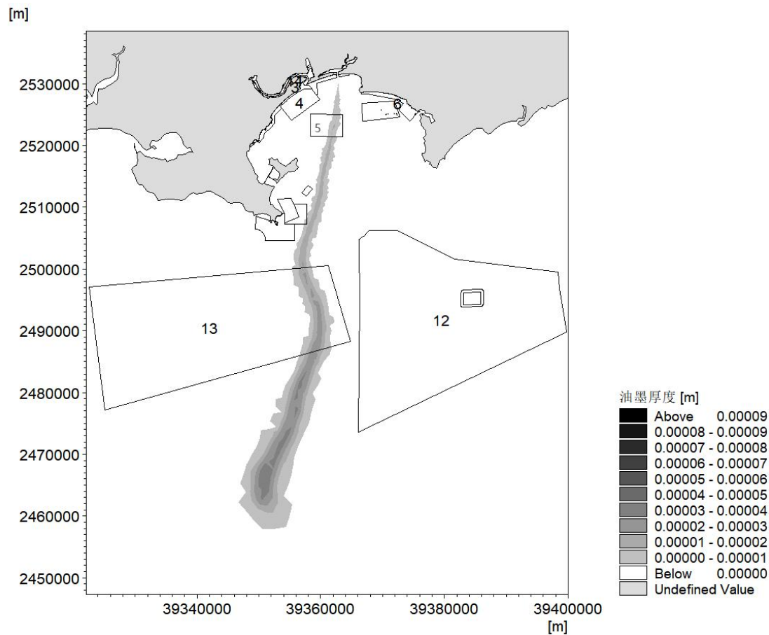
图 7.2.3-7a N 向不利风速落潮时溢油 48h 后最大扫海范围图
