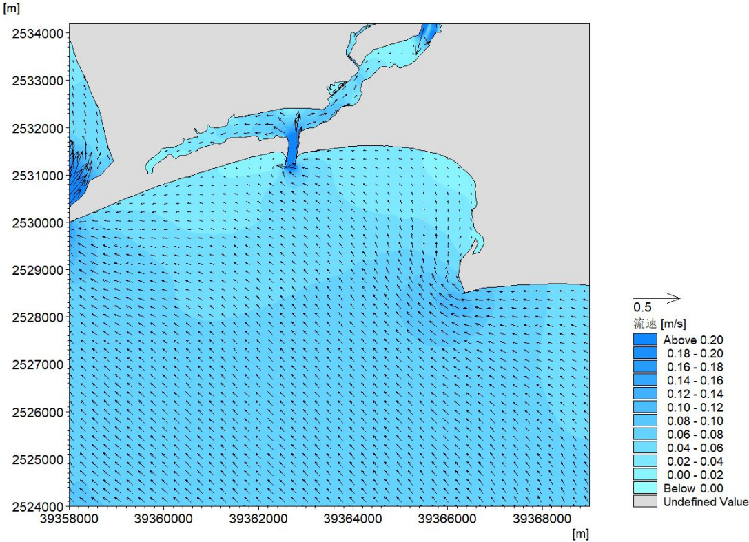
图 6.3.1-8a 工程前涨急时刻工程附近海域流场图
