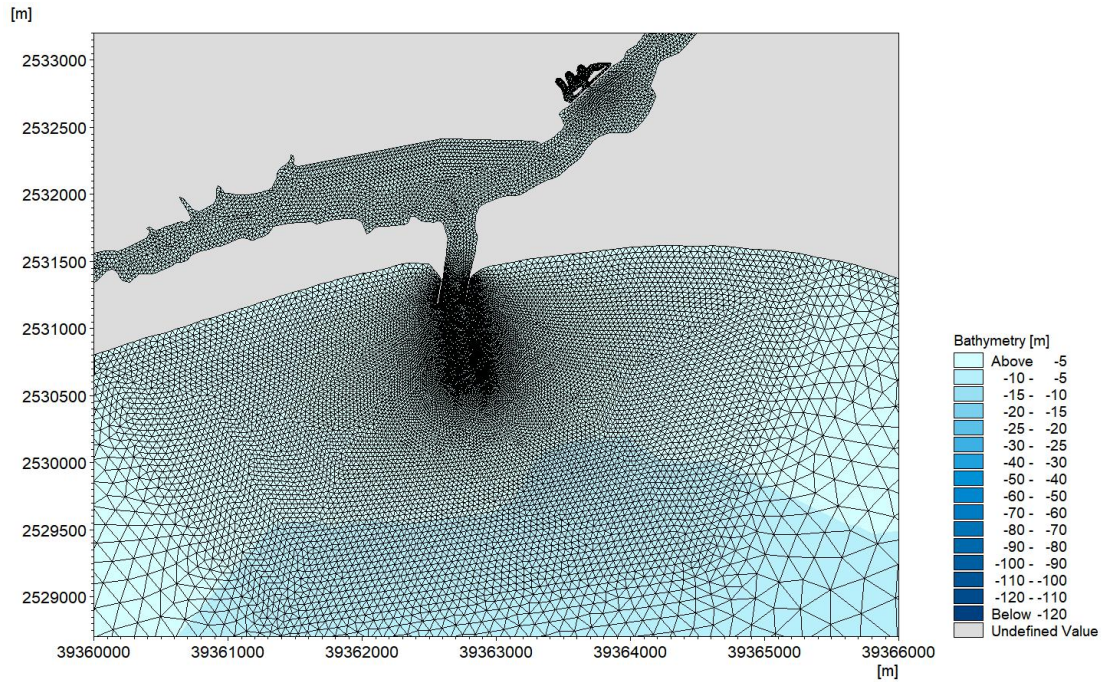
图 6.3.1-2a 工程前附近海域计算网格分布
