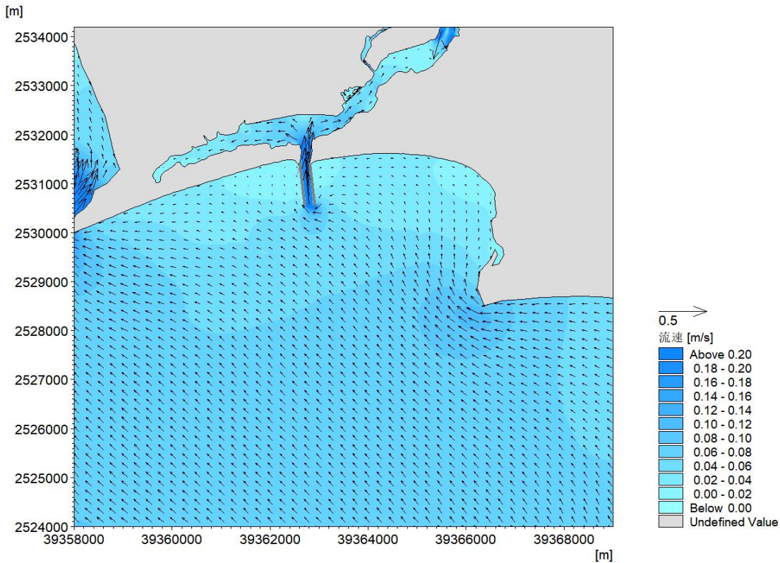
图 6.3.1-9a 工程后涨急时刻工程附近海域流场图
