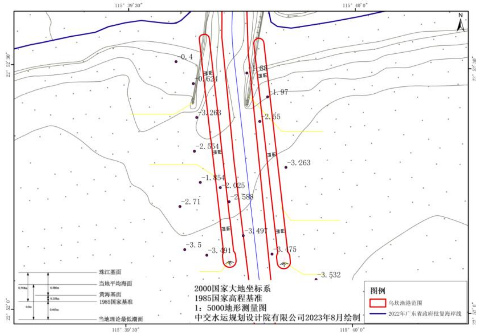
图 5.3.2-6c 项目所在海域水深地形图
