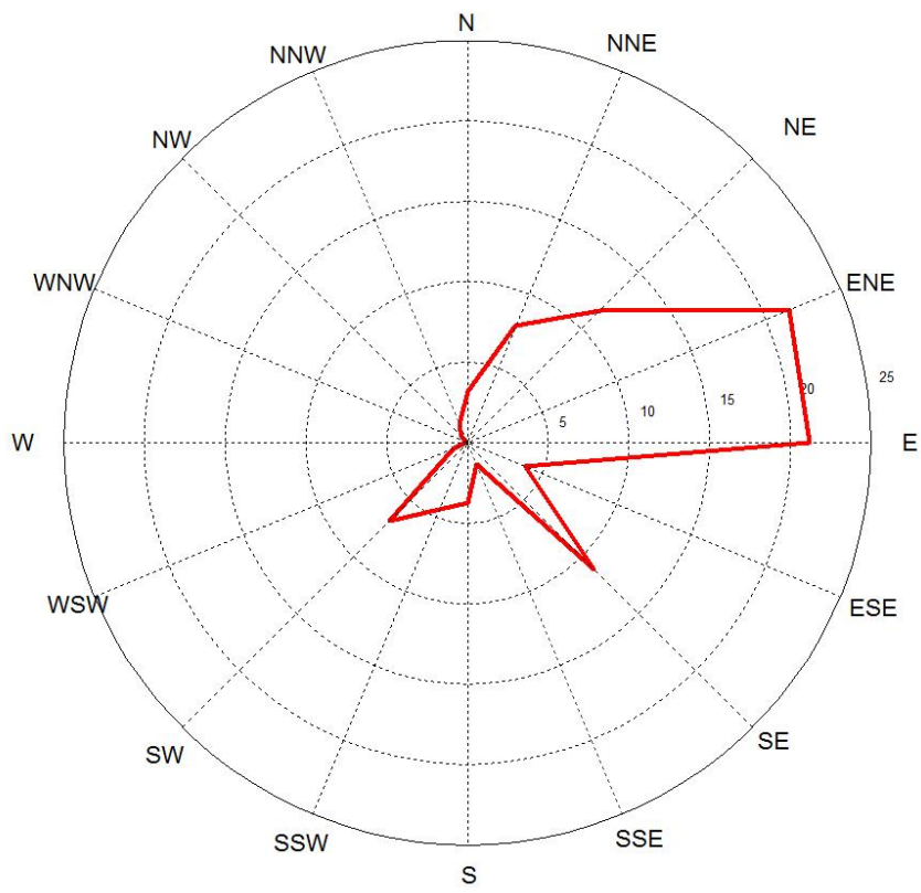
图 4.1.4-1 波浪玫瑰图
