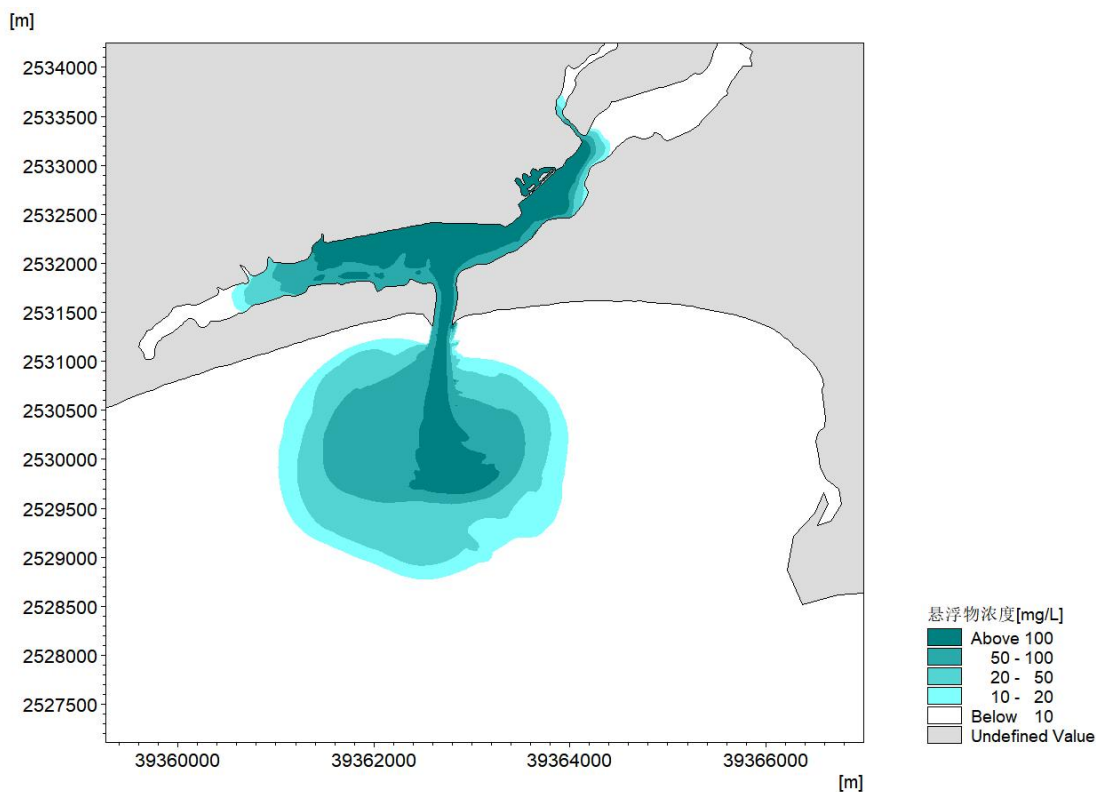
图 6.3.3-7 所有施工工况同时叠加悬浮泥沙扩散范围
