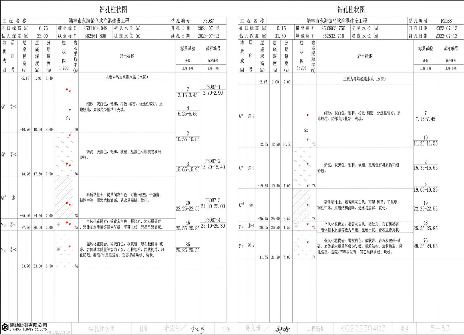
图 5.3.2-11 钻孔柱状图 (防波堤)
