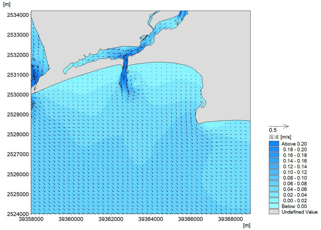
图 6.3.1-8b 工程前落急时刻工程附近海域流场图
