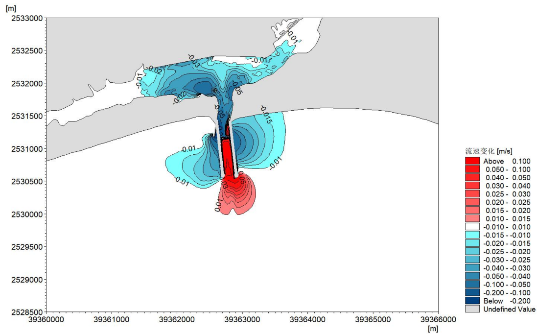
图 6.3.1-10b 工程前后涨急流向变化图
