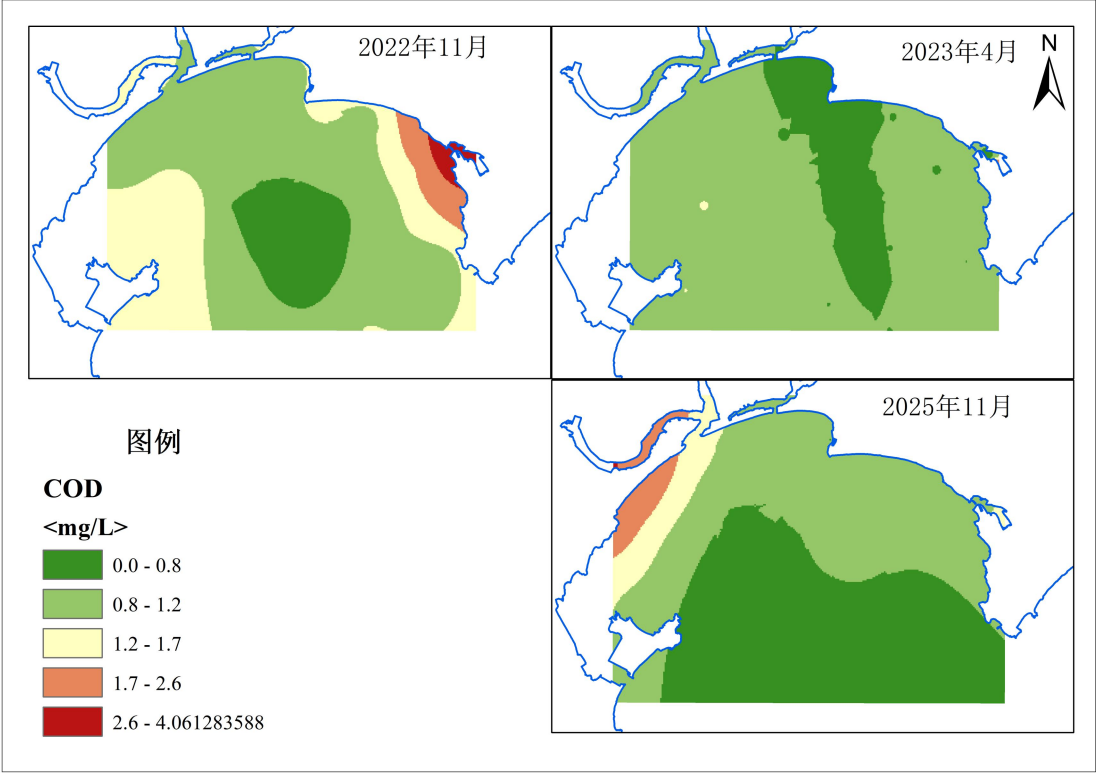
图 5.3.7-1 项目海域 COD 指标年际变化图
