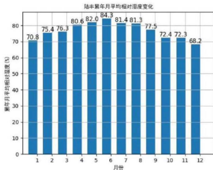
图 4.1.1-9 陆丰月平均相对湿度（纵轴为百分比）
