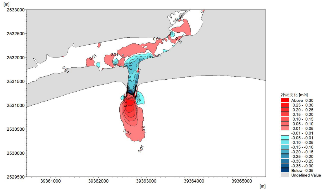
图 6.3.2-1 工程前冲淤环境
