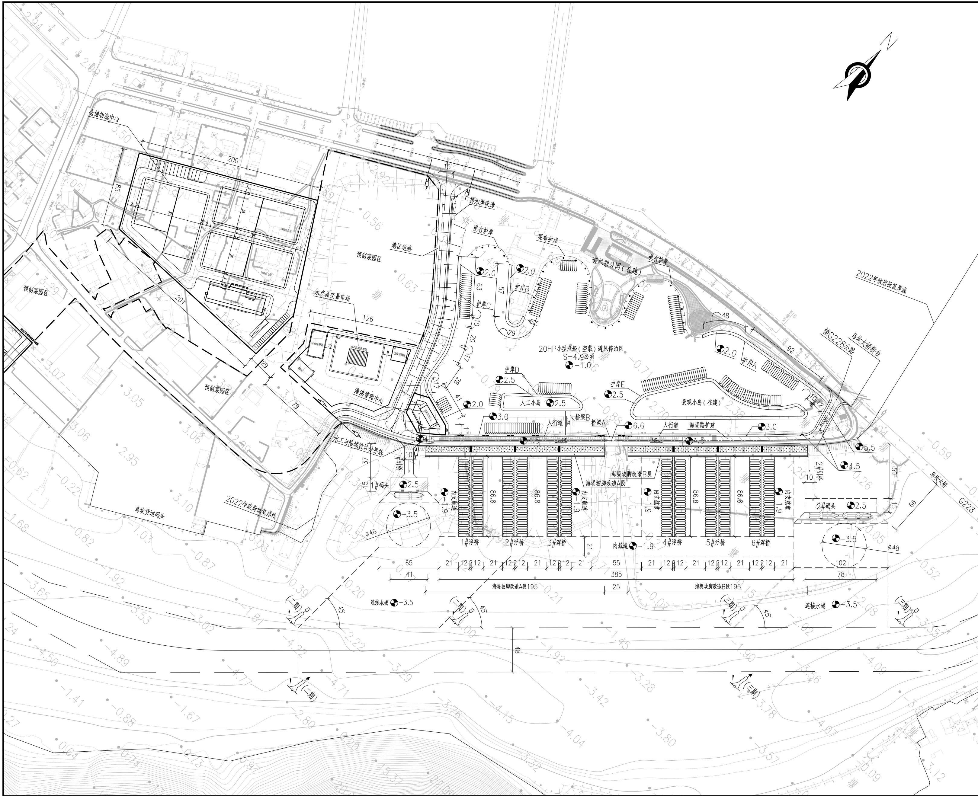
图 2.3.1-5 码头及部分陆域平面布置图
