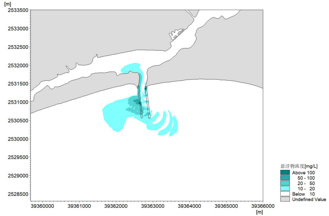
图 6.3.3-4a 东、西防波堤施工悬浮物影响范围
