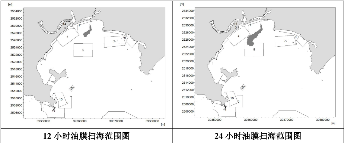
图 7.2.3-3b N 向平均风速落潮时溢油 12h、24h 后扫海范围图
