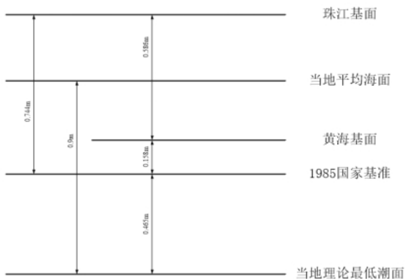
图 3-166 汕尾站各基面关系图
