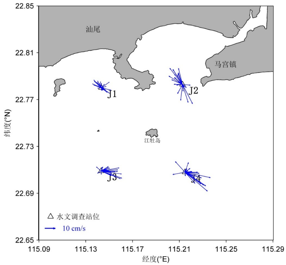
图 3-28 大潮期垂线平均海流平面分布矢量图
