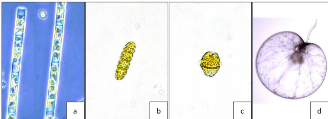
图 4-1 2021 年广东省海域发现的部分赤潮生物显微镜下照片 (a: 丹麦细柱藻, b: 链状裸甲藻, c: 红色赤潮藻, d: 夜光藻)
