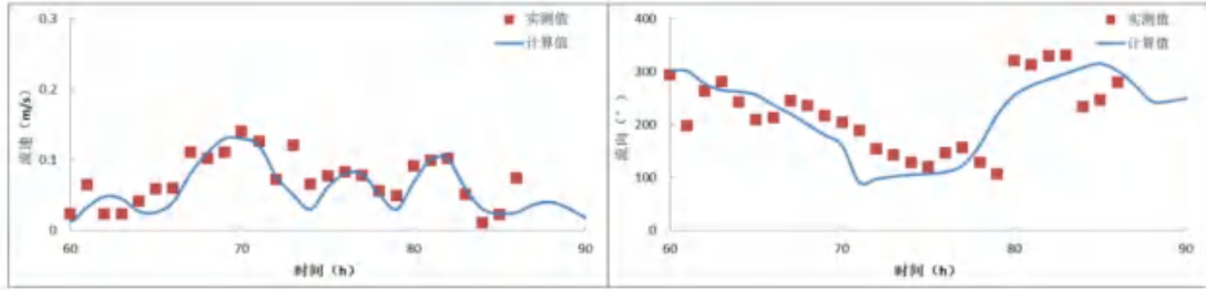
图 6.1.1-7i 冬季 SWL4 站流速、流向验证 (底层)
