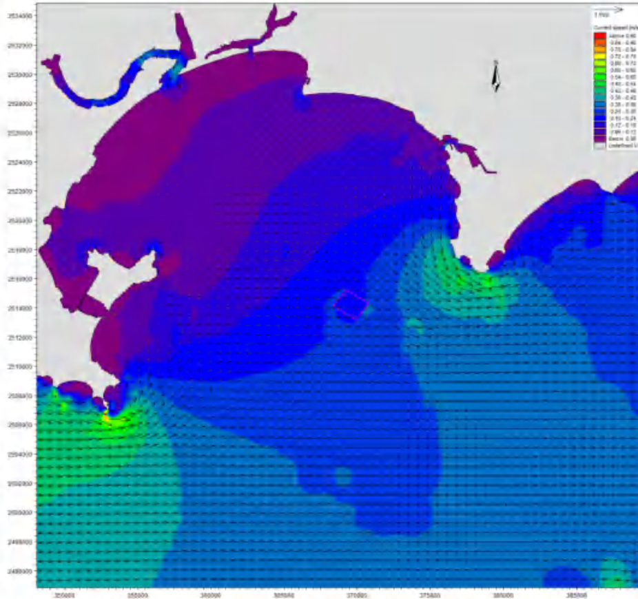
图 6.1.3-4e 工程实施后冬季大潮落急流场图（中层）
