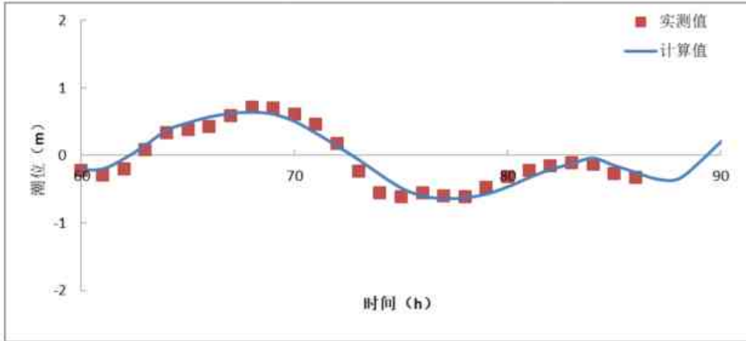
图 6.1.1-6a 冬季 SWC1 站潮位验证
