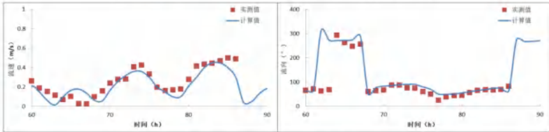
图 6.1.1-7h 冬季 SWL3 站流速、流向验证 (0.6 层)
