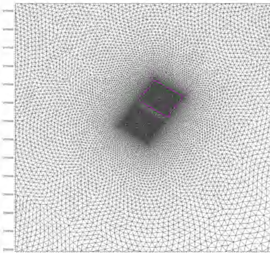
图 6.1.1-2a 工程区网格剖分图 (SW24-12 采砂区)
