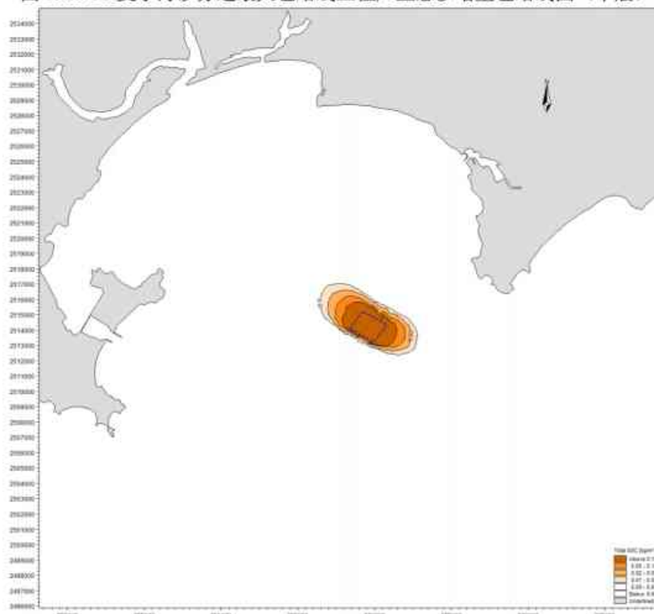
图 6.4.2-3c 夏季海砂分选最大包络线工程产生悬沙增量包络线图（底层）
