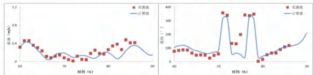
图 6.1.1-5d 夏季 SWL2 站流速、流向验证 (表层)
