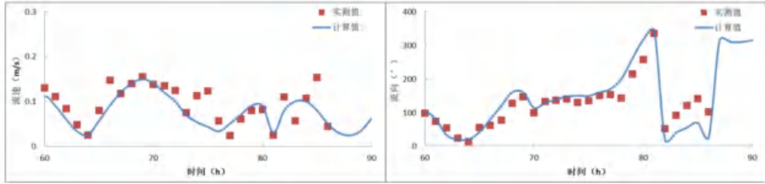
图 6.1.1-7b 冬季 SWL1 站流速、流向验证 (0.6 层)
