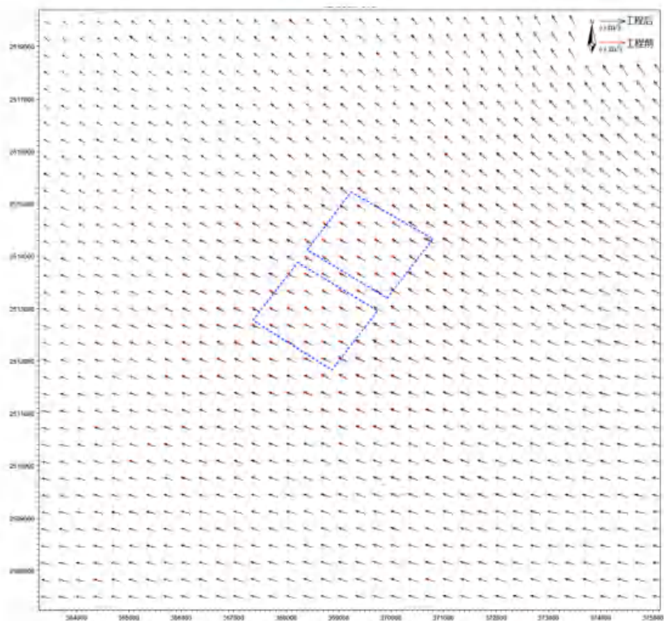
图 6.1.3-12a 工程实施前后冬季大潮涨急流场对比图（中层）
