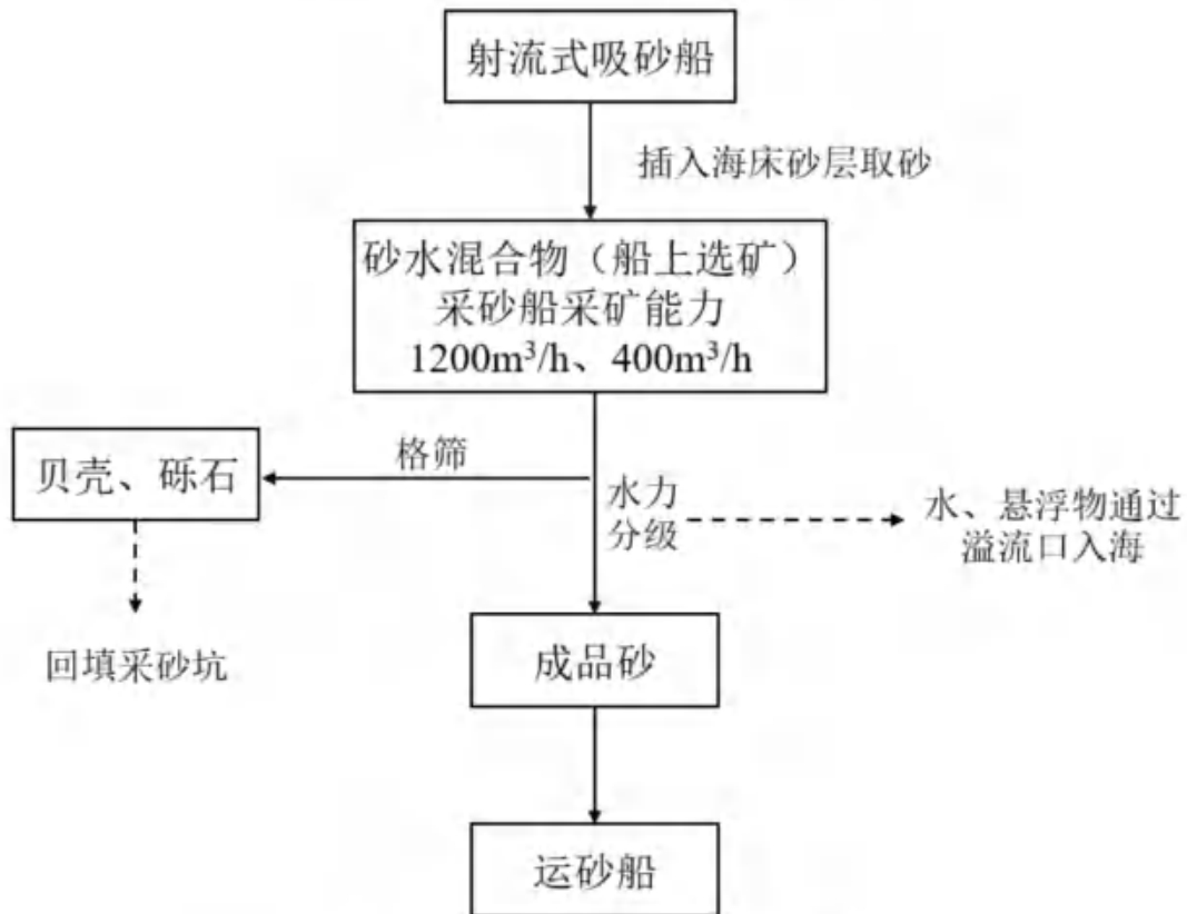
图 3.4-5 采砂工艺和溢流口工艺流程图
