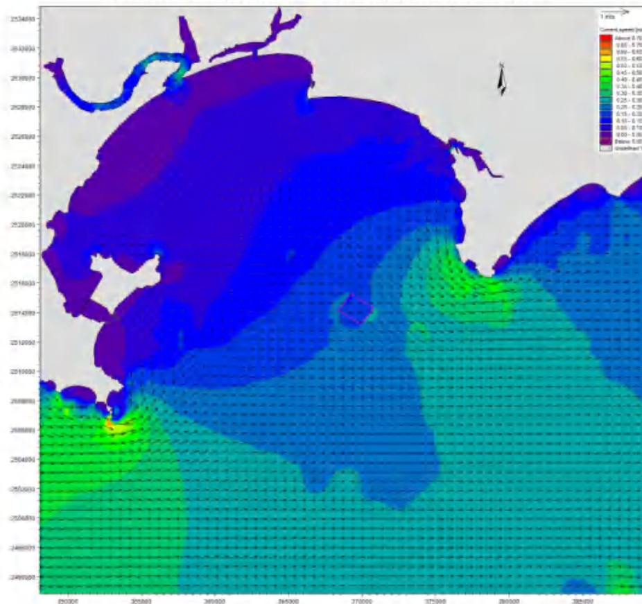
图 6.1.3-4f 工程实施后冬季大潮落急流场图（底层）
