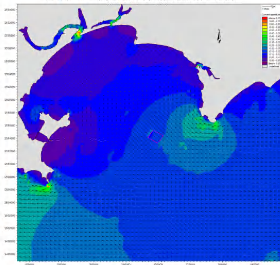
图 6.1.3-4b 工程实施后冬季大潮涨急流场图（中层）
