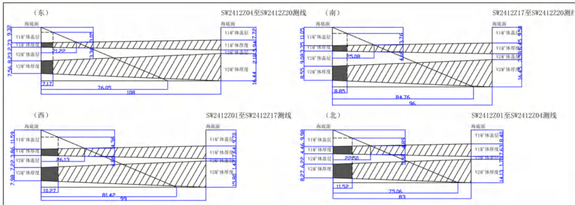
图 3.3.1-3 矿区开采剖面示意图（图中黑色部分为不可开采矿体截面）
