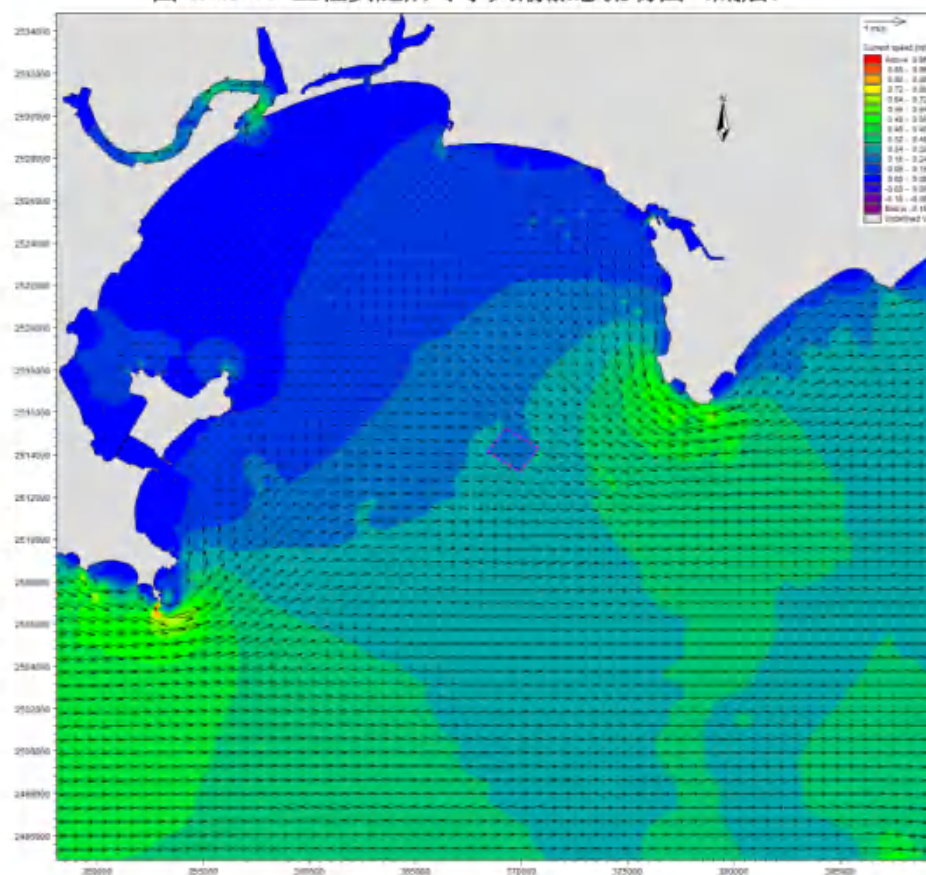
图 6.1.3-4d 工程实施后冬季大潮落急流场图（表层）
