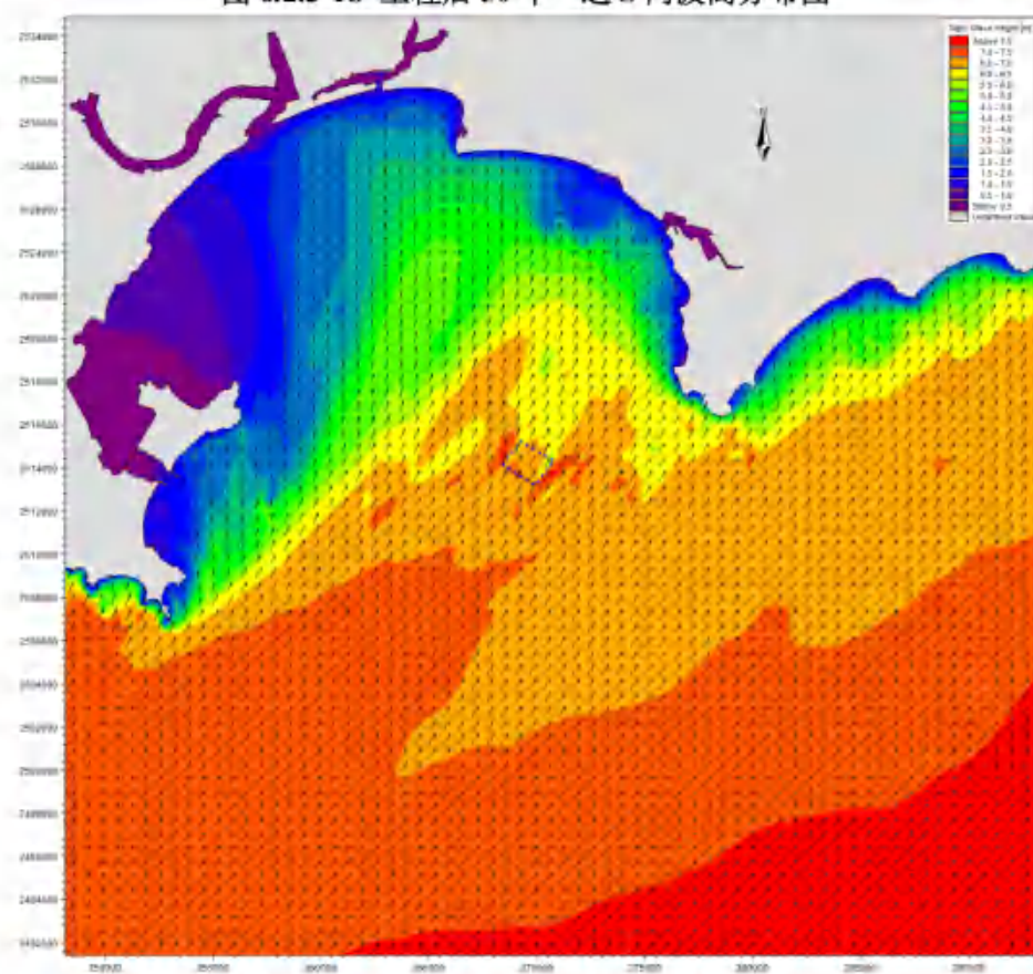
图 6.2.3-1c 工程后 50 年一遇 SW 向波高分布图
