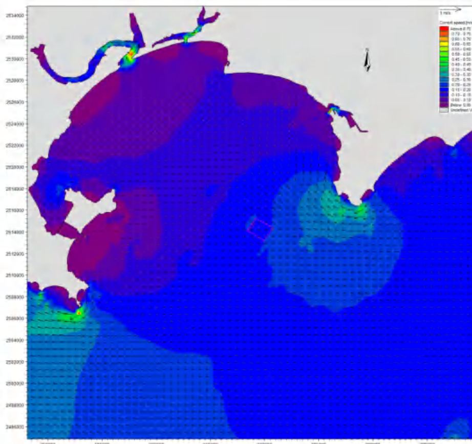
图 6.1.3-4a 工程实施后冬季大潮涨急流场图（表层）
