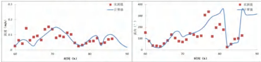
图 6.1.1-7c 冬季 SWL1 站流速、流向验证 (底层)
