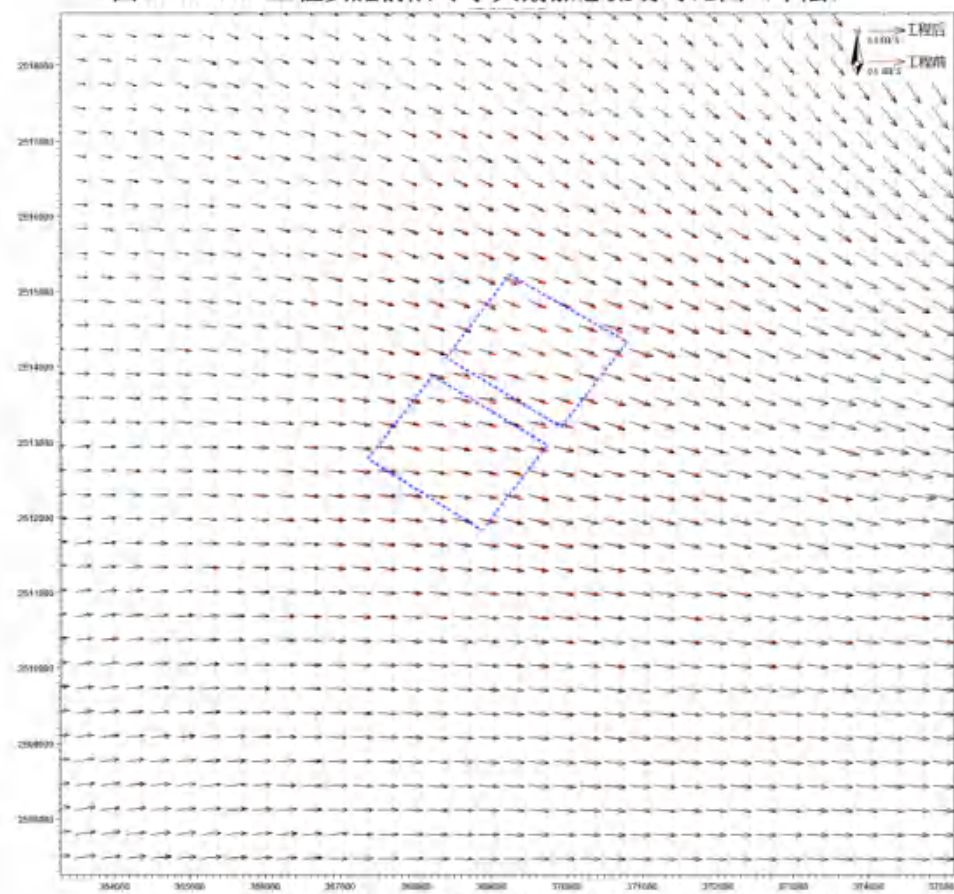
图 6.1.3-12b 工程实施前后冬季大潮落急流场对比图（中层）
