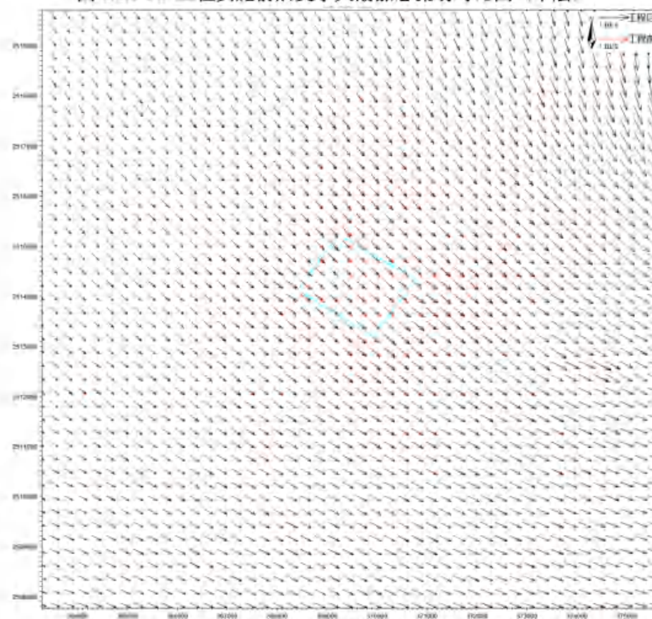
图 6.1.3-5b 工程实施前后夏季大潮落急流场对比图（中层）
