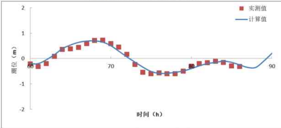
图 6.1.1-6b 冬季 SWC2 站潮位验证
