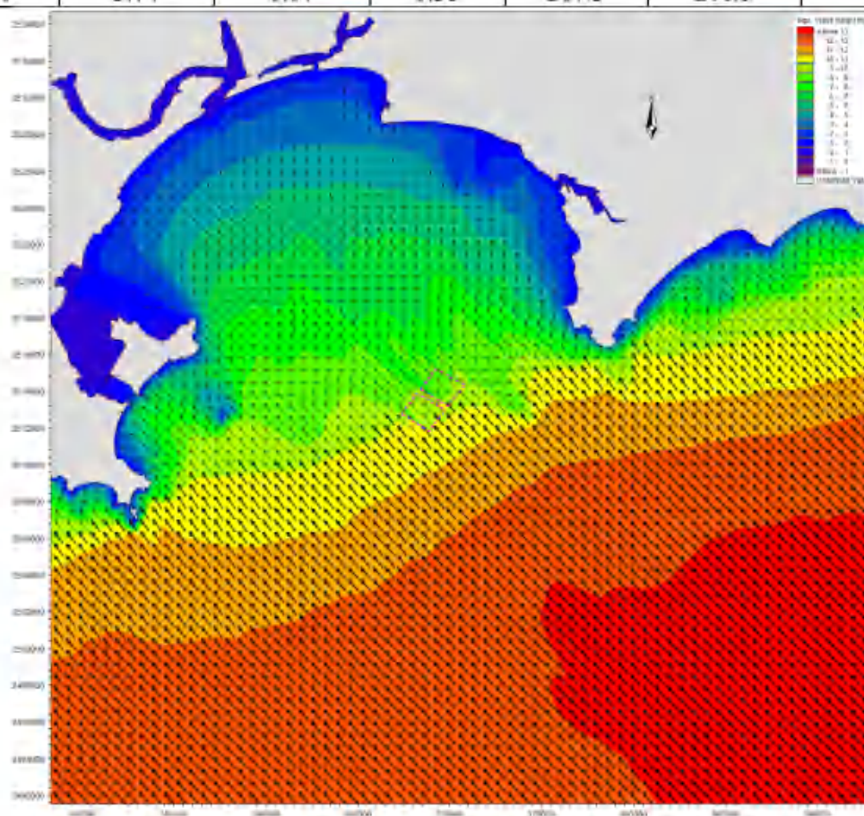
图 6.2.3-2a 工程后 50 年一遇 SE 向波高分布图
