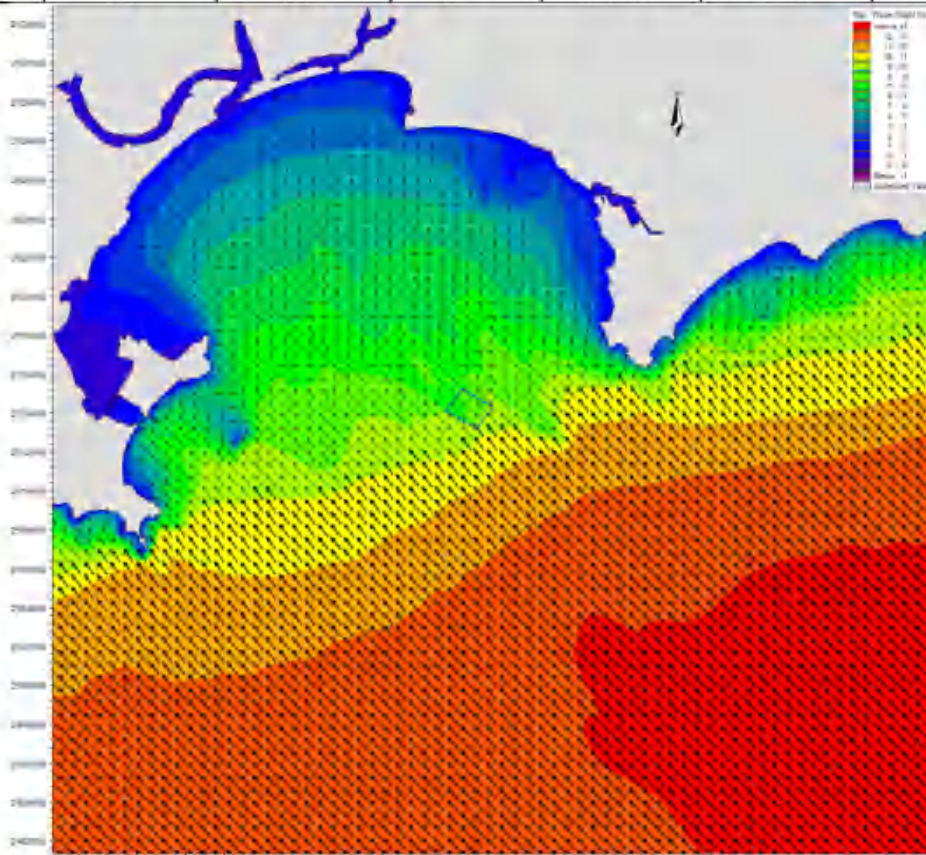
图 6.2.3-1a 工程后 50 年一遇 SE 向波高分布图
