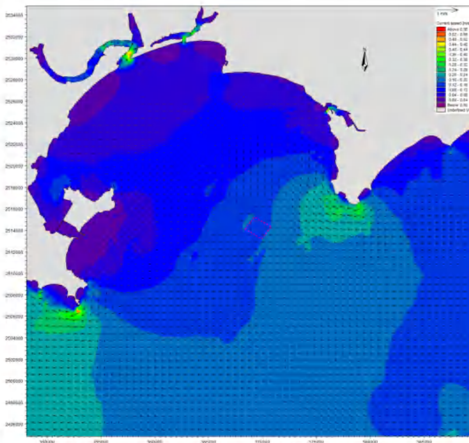
图 6.1.3-4c 工程实施后冬季大潮涨急流场图（底层）
