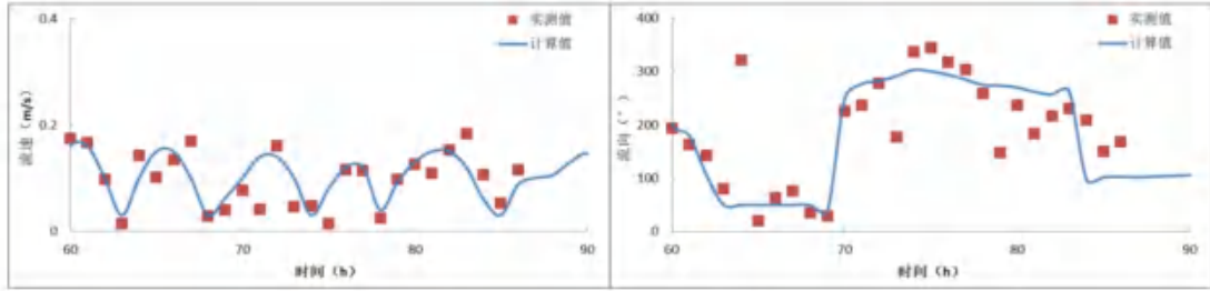
图 6.1.1-5j 夏季 SWL4 站流速、流向验证（表层）
