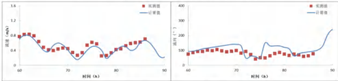
图 6.1.1-5q 夏季 SWL6 站流速、流向验证 (表层)
