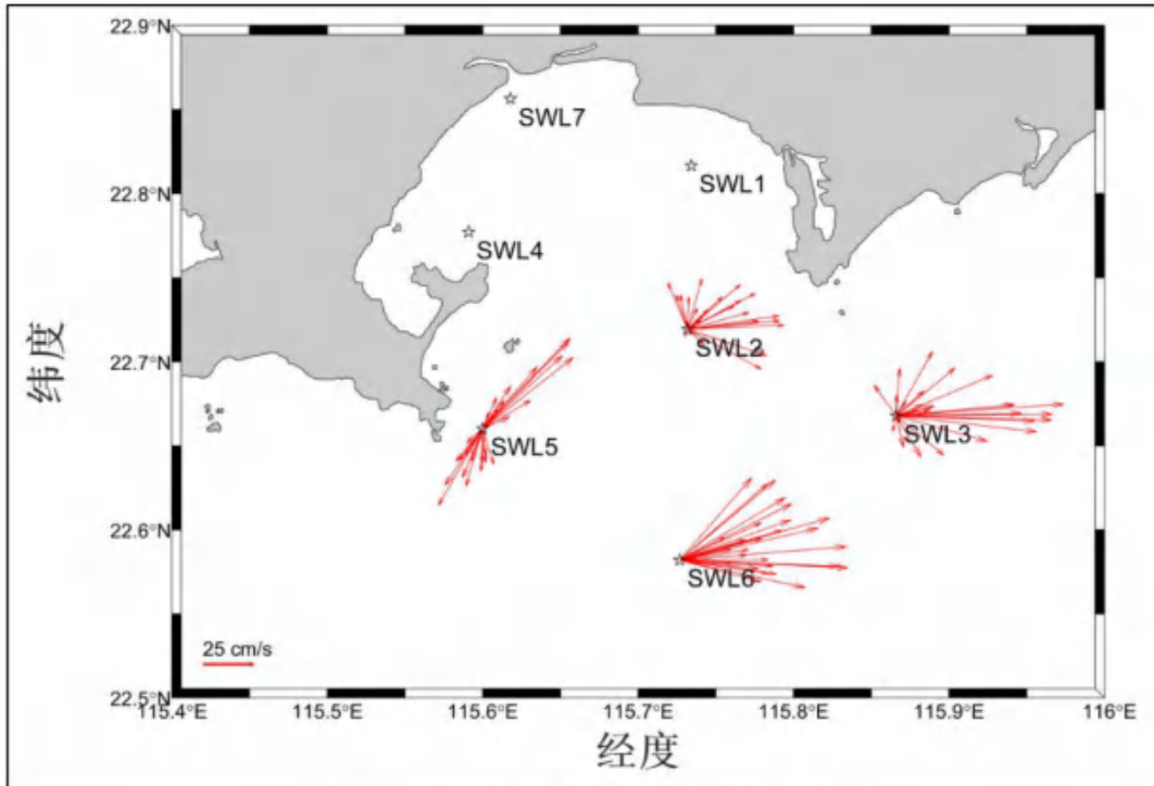
图 5.5.4-7 夏季表层海流平面分布矢量图
