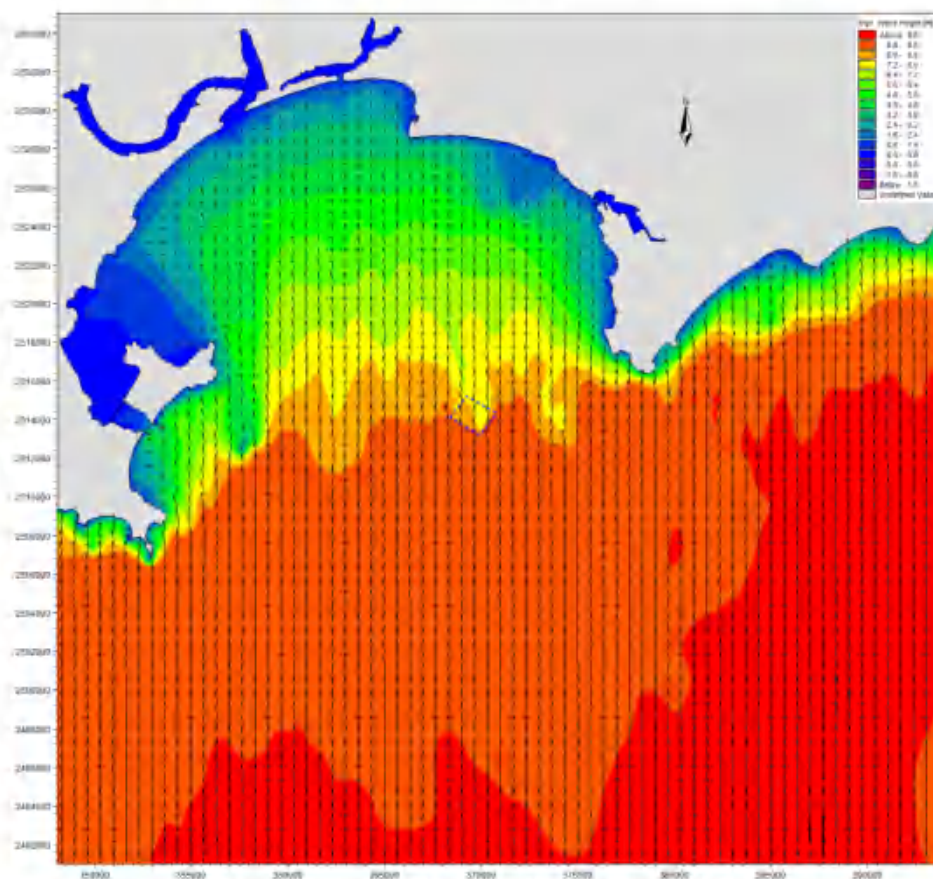
图 6.2.3-1b 工程后 50 年一遇 S 向波高分布图
