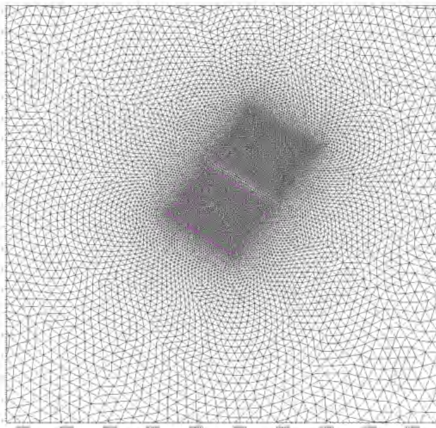
图 6.1.1-2a 工程区网格剖分图 (SW24-11 采砂区)
