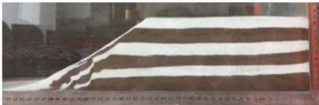
图 6.3.5-2b 采砂深度 11cm 实验照片
