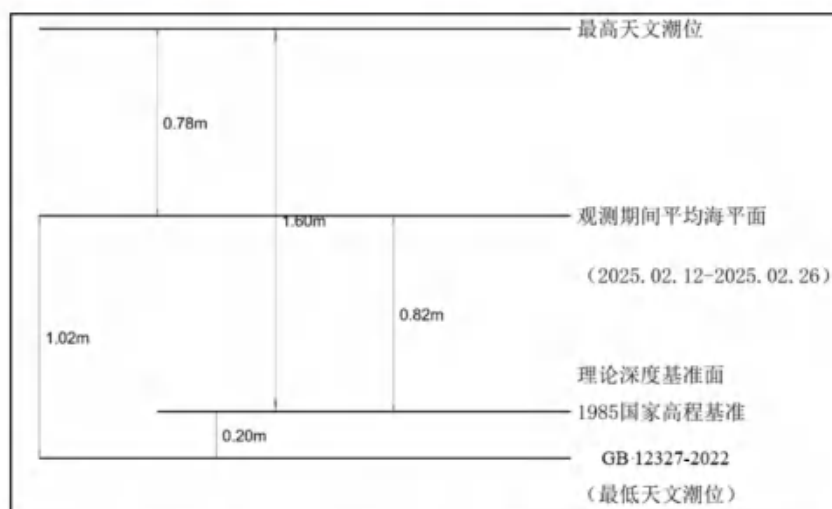
图 5.5.3-9 SWC1 临时潮位站各基准面的相互关系
