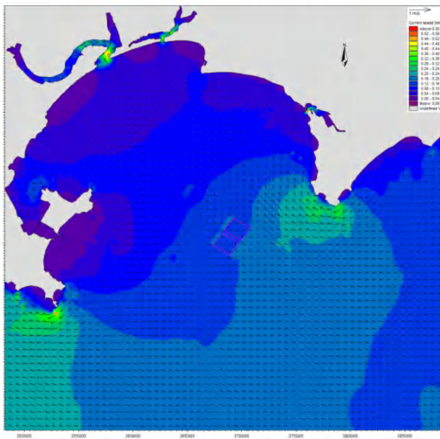
图 6.1.3-11c 工程实施后冬季大潮涨急流场图（底层）
