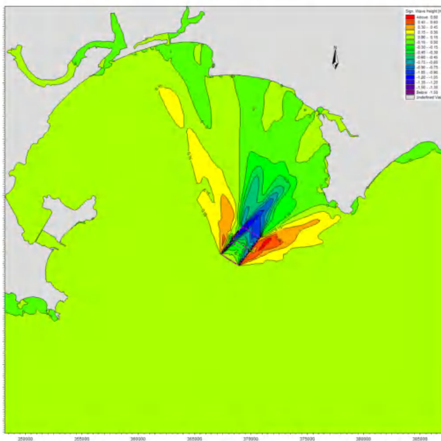
图 6.3.4-4c 砂区实施前后 SW 向 50 年一遇 H_{13} 波高变化等值线图
