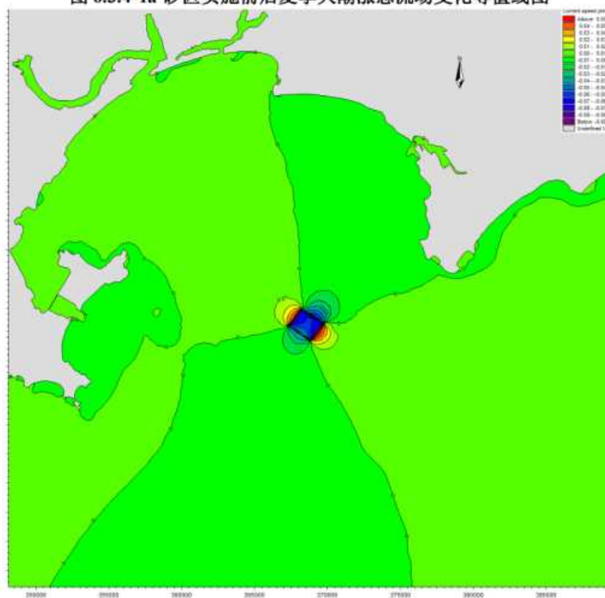
图 6.3.4-1b 砂区实施前后夏季大潮落急流场变化等值线图
