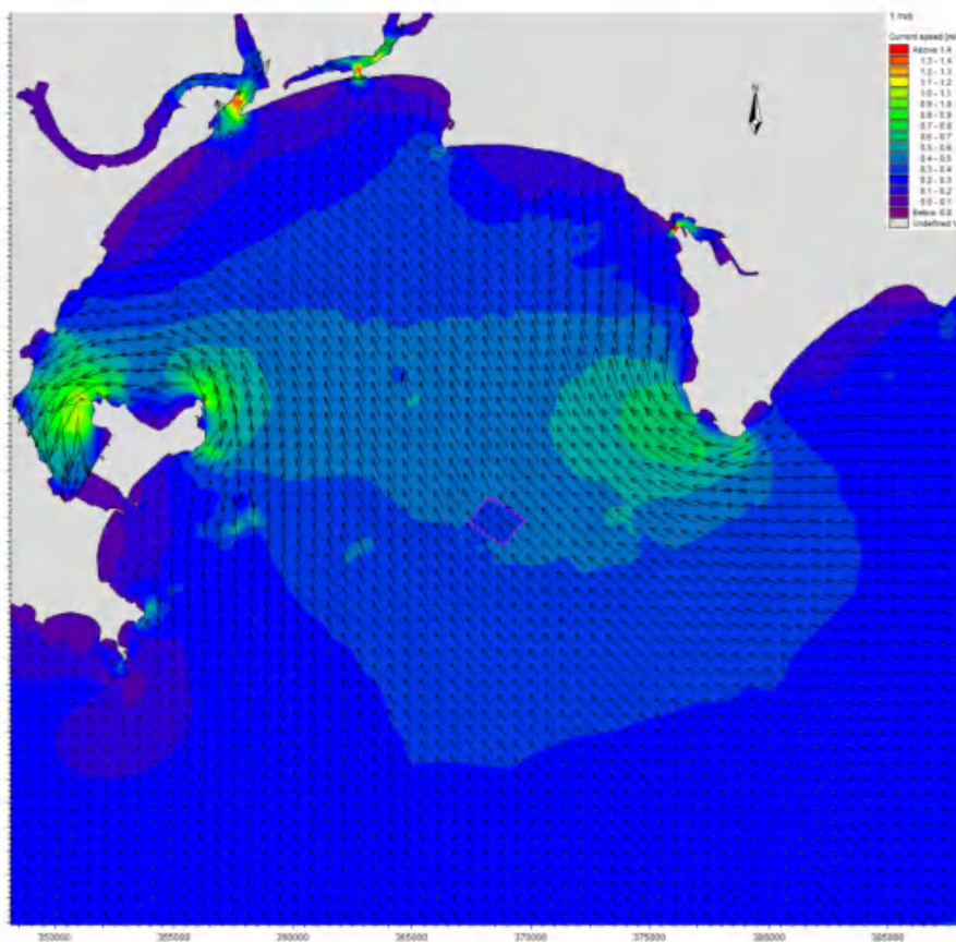
图 6.1.3-3a 工程实施后夏季大潮涨急流场图（表层）
