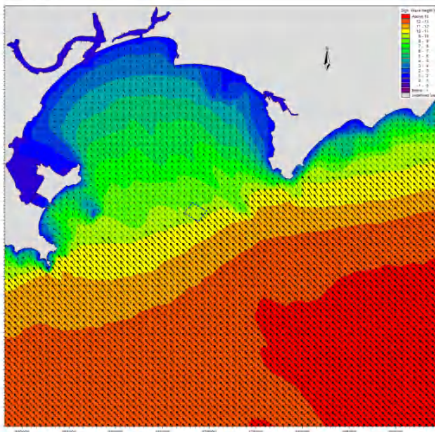
图 6.2.2-1a 工程前 50 年一遇 SE 向有效波高分布图
