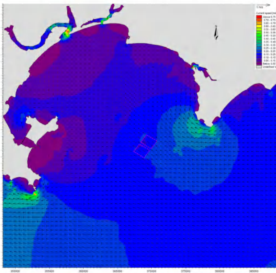
图 6.1.3-11a 工程实施后冬季大潮涨急流场图（表层）
