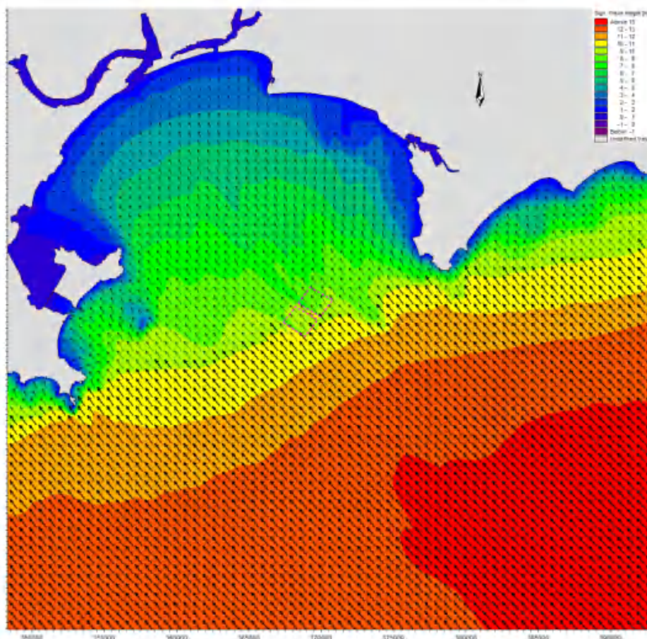
图 6.2.3-2a 工程后 50 年一遇 SE 向波高分布图
