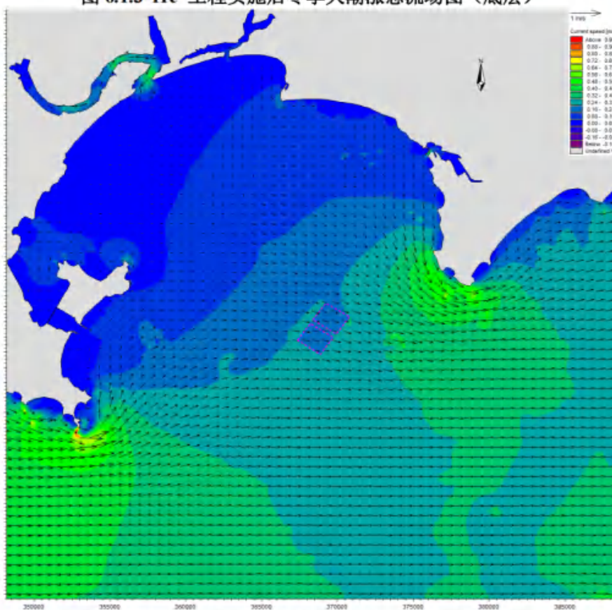
图 6.1.3-11d 工程实施后冬季大潮落急流场图（表层）
