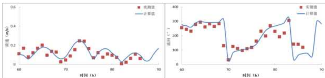
图 6.1.1-7d 冬季 SWL2 站流速、流向验证 (表层)
