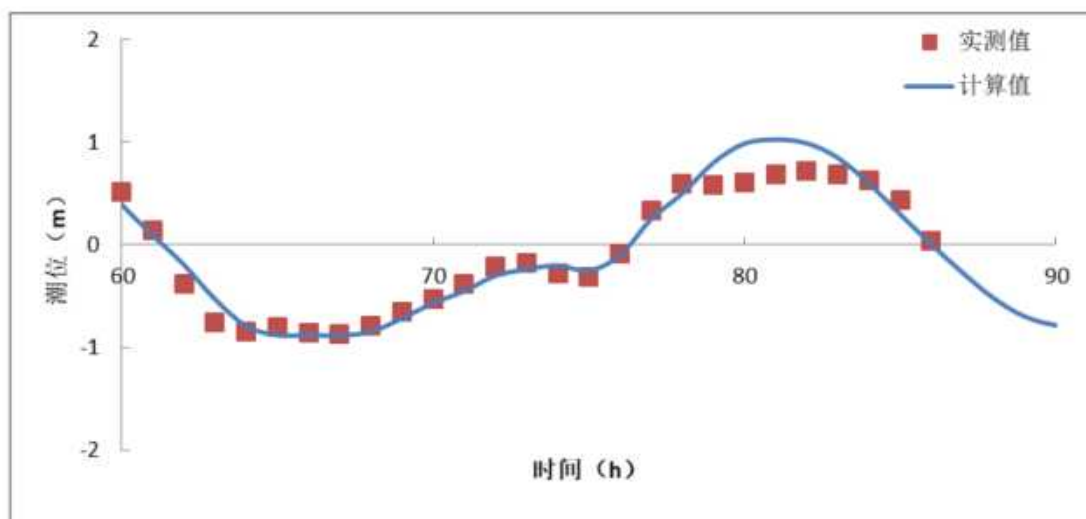
图 6.1.1-4b 夏季 SWC2 站潮位验证
