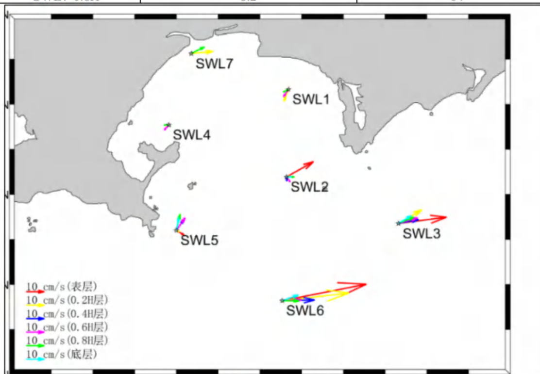
图 5.5.6-2 夏季观测期各站余流图
