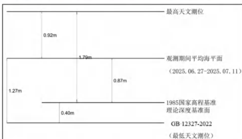
图 5.5.3-11 SWC1 临时潮位站各基准面的相互关系
