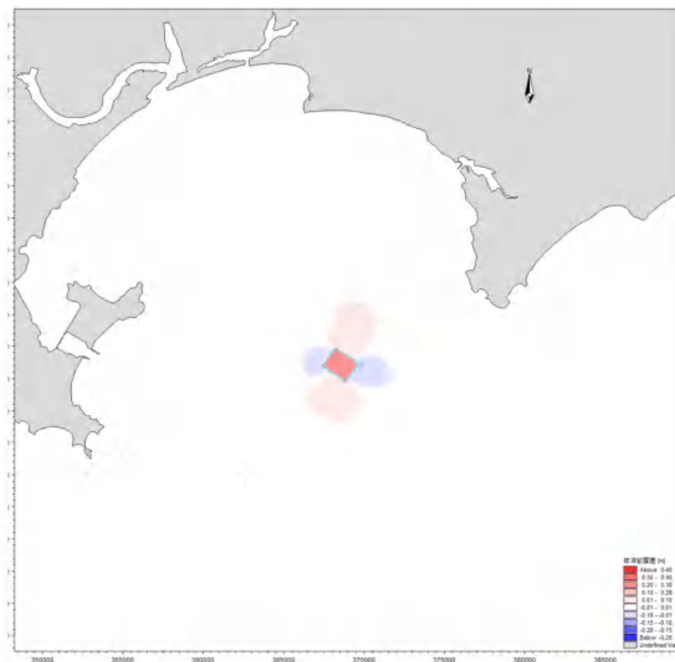
图 6.3.2-1 工程实施后年冲淤变化图
