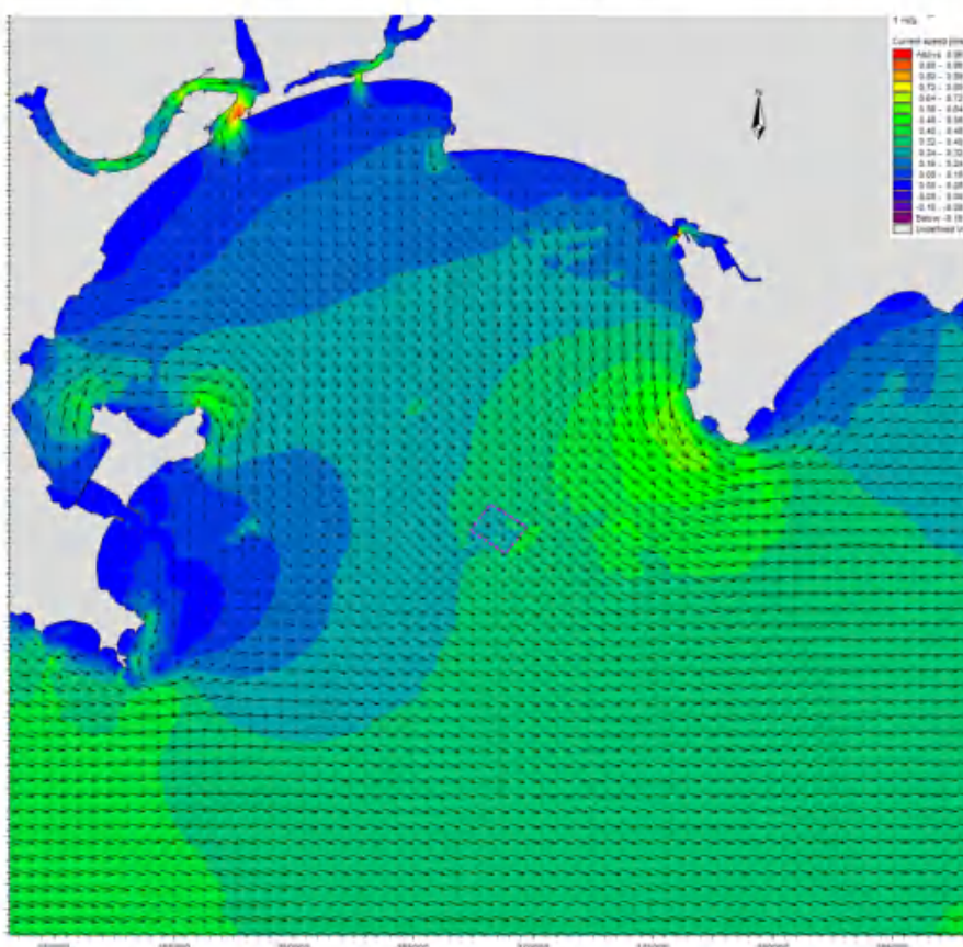
图 6.1.3-3f 工程实施后夏季大潮落急流场图（底层）
