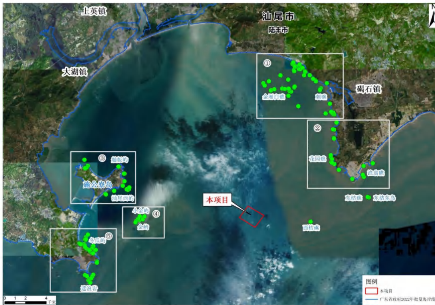
图 2.7.1-1d 项目周边环境敏感区分布图（岛礁）
