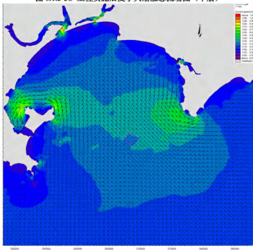
图 6.1.3-3c 工程实施后夏季大潮涨急流场图（底层）
