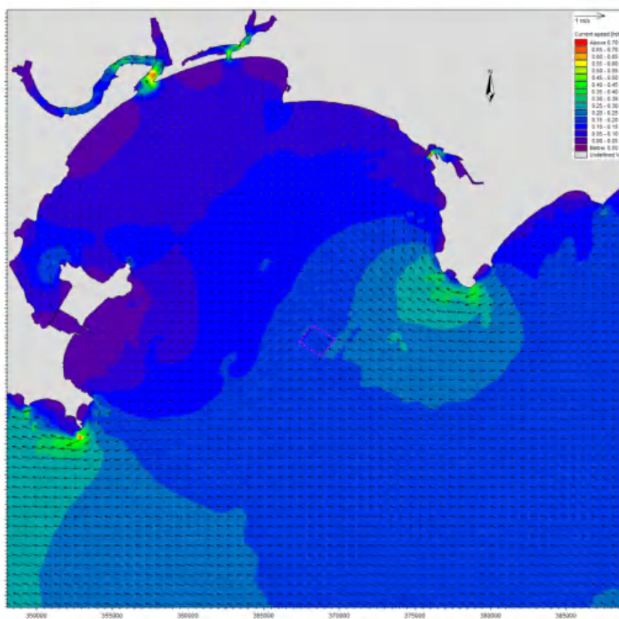
图 6.1.3-5b 工程实施后冬季大潮涨急流场图（中层）
