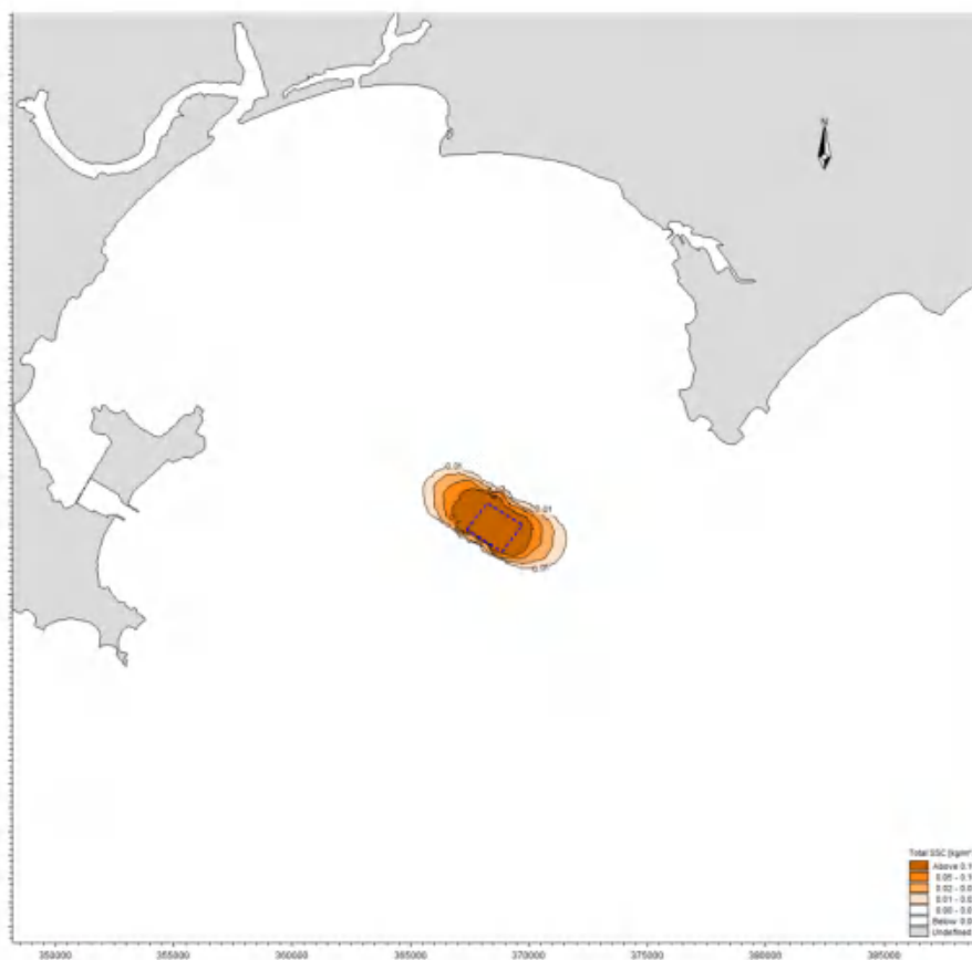
图 6.4.2-3a 夏季海砂分选最大包络线工况产生悬沙增量包络线图（表层）
