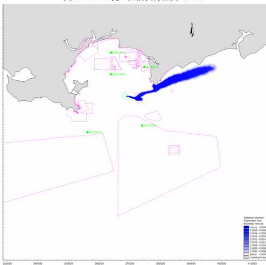
图 7.5.1-4 工况 4 溢油扫海范围 (48h)
