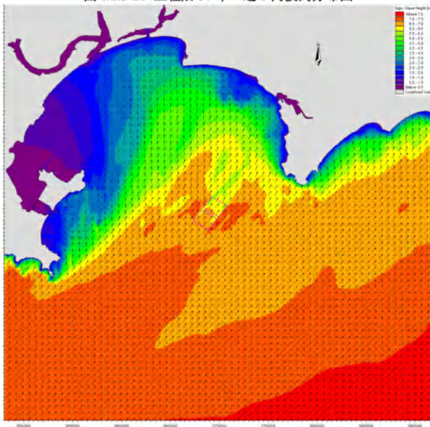
图 6.2.3-2c 工程后 50 年一遇 SW 向波高分布图
