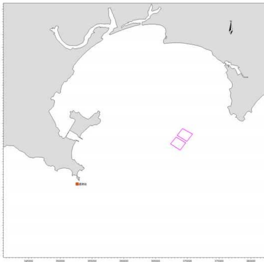
图 6.2.1-1 波浪验证点位置图
