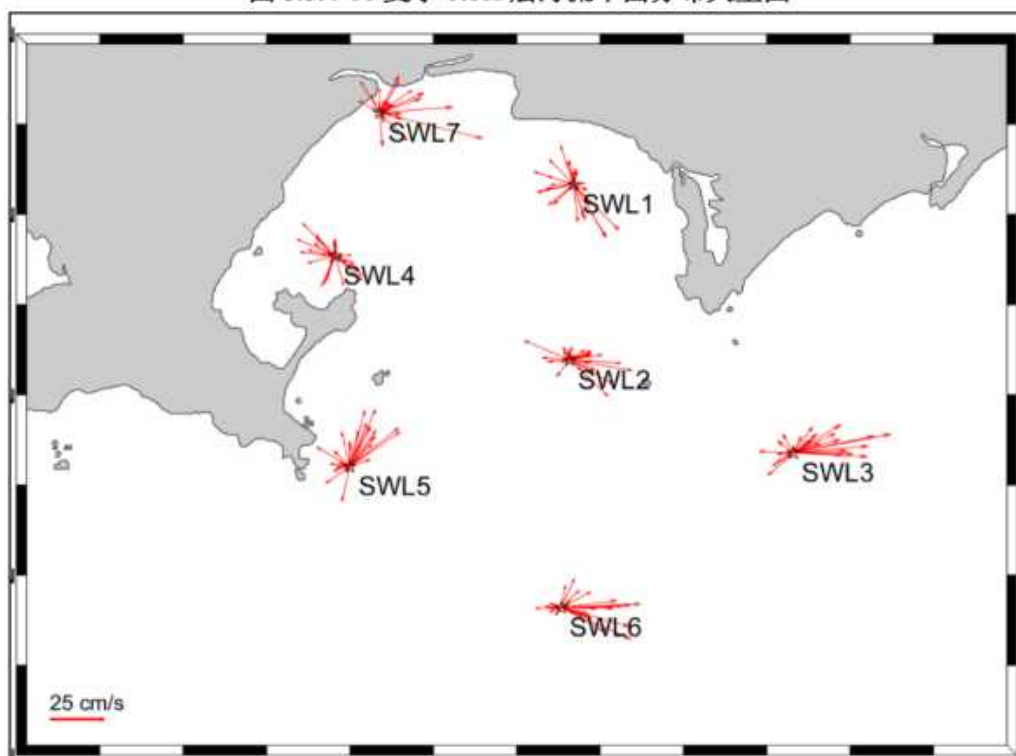
图 5.5.4-11 夏季 0.8H 层海流平面分布矢量图
