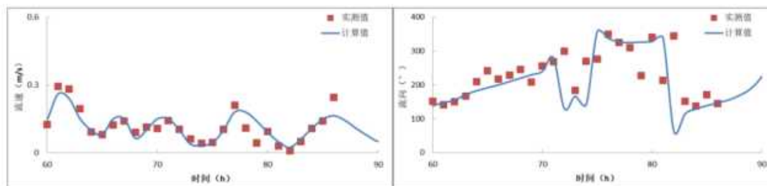
图 6.1.1-5b 夏季 SWL1 站流速、流向验证（0.6 层）
