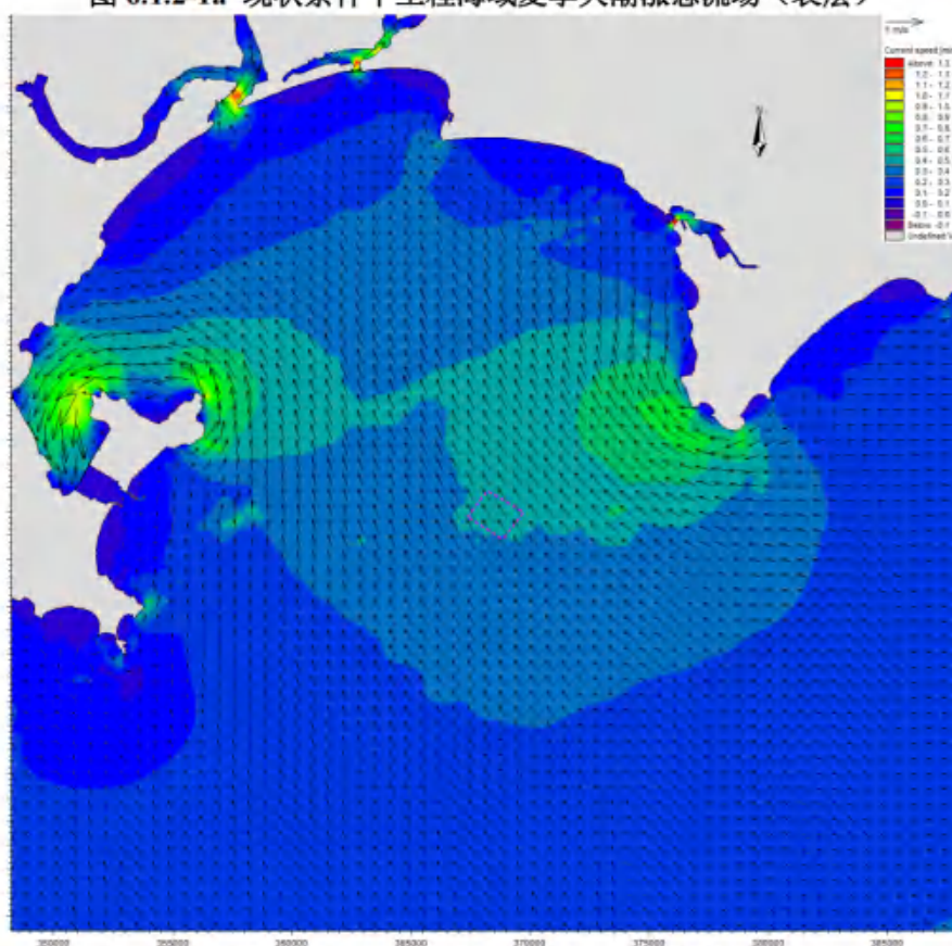
图 6.1.2-1b 现状条件下工程海域夏季大潮涨急流场（中层）
