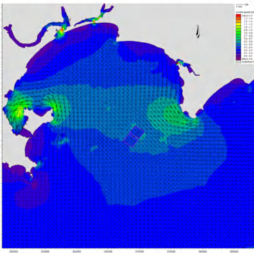
图 6.1.3-9a 工程实施后夏季大潮涨急流场图（表层）
