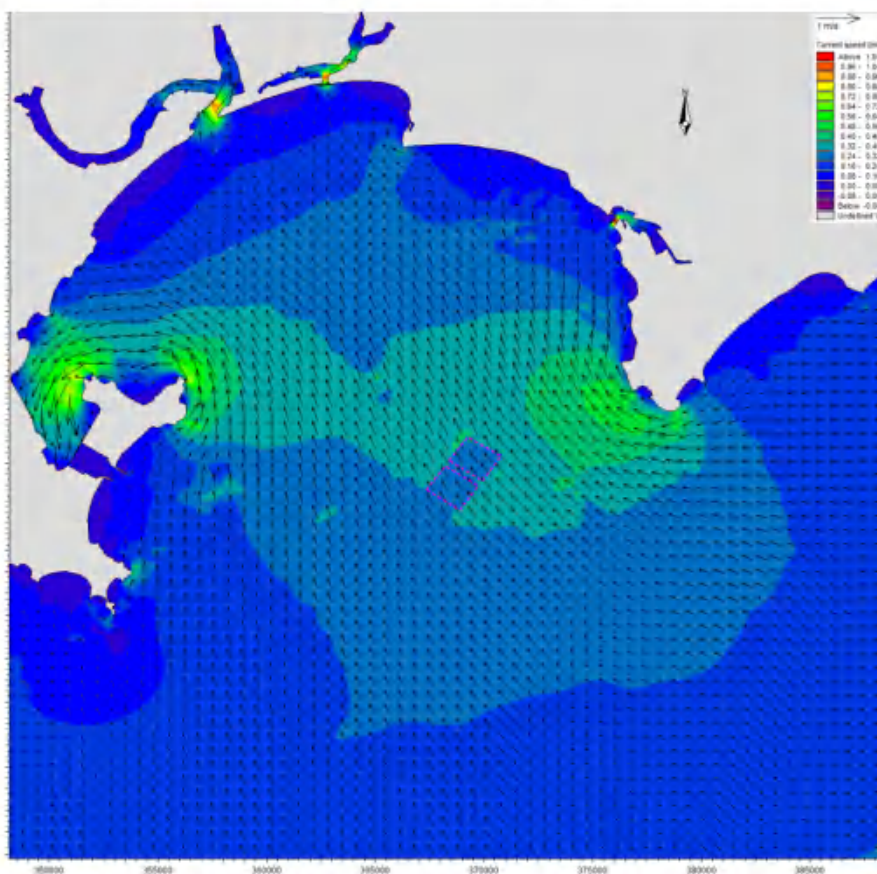
图 6.1.3-9c 工程实施后夏季大潮涨急流场图（底层）
