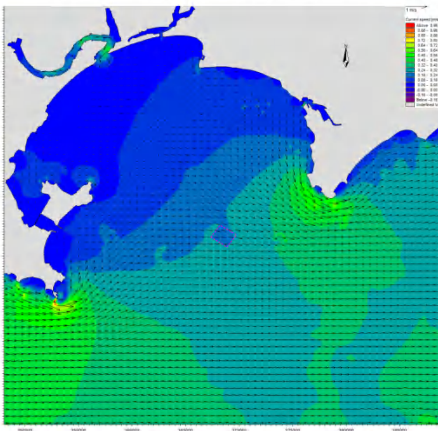
图 6.1.3-5d 工程实施后冬季大潮落急流场图（表层）
