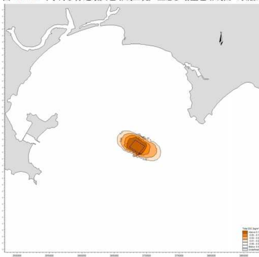
图 6.4.2-4b 冬季海砂分选最大包络线工况产生悬沙增量包络线图（中层）
