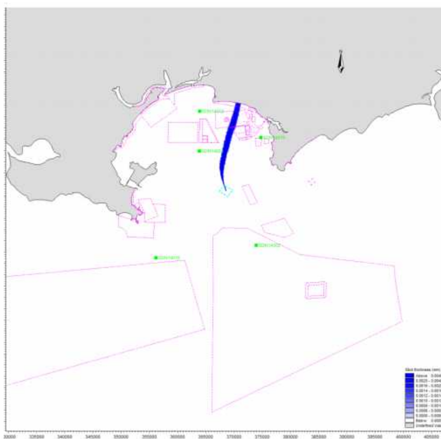
图 7.5.1-5 工况 5 溢油扫海范围 (48h)
