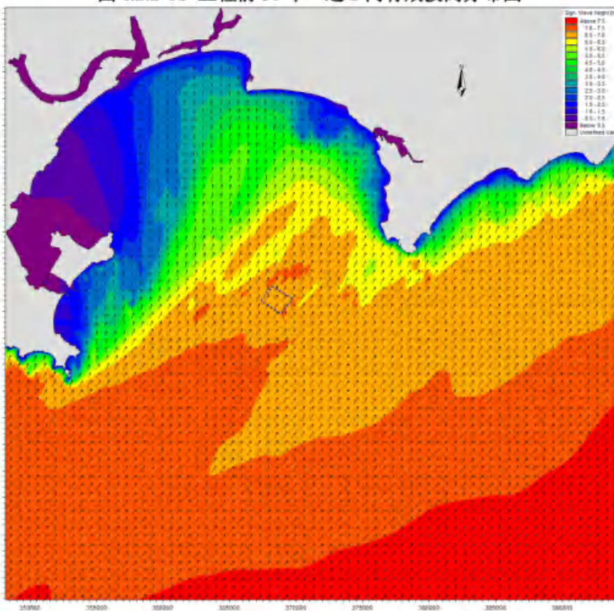
图 6.2.2-1c 工程前 50 年一遇 SW 向有效波高分布图
