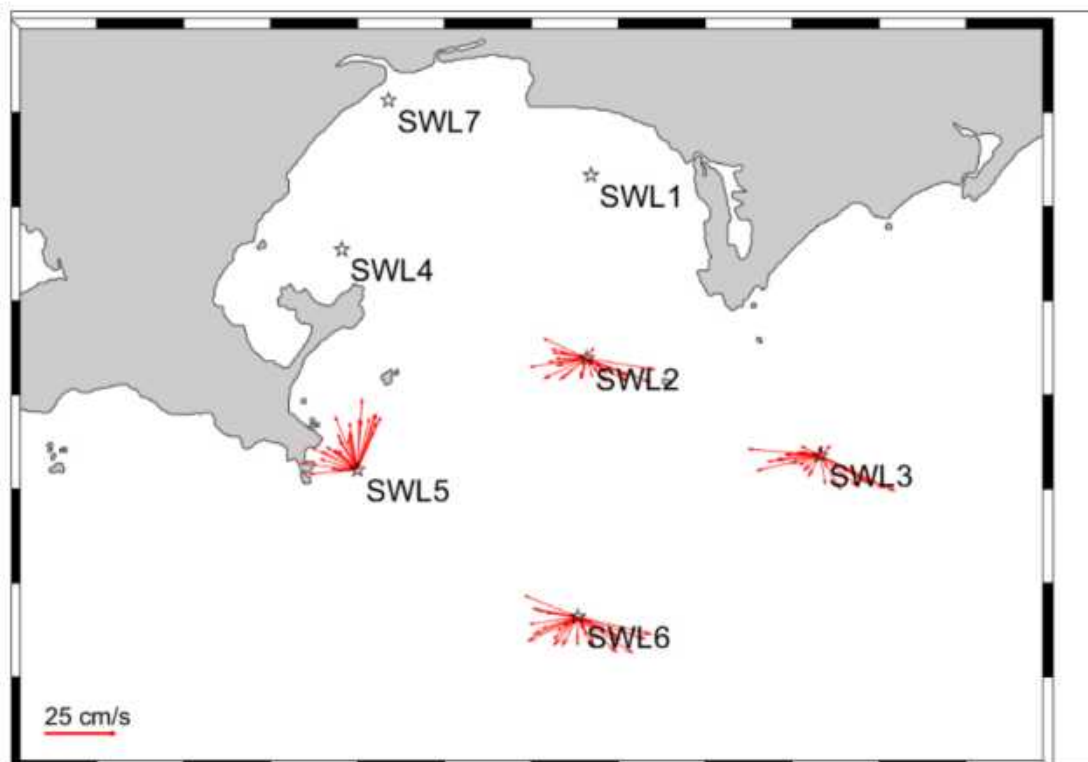
图 5.5.4-1 冬季表层海流平面分布矢量图
