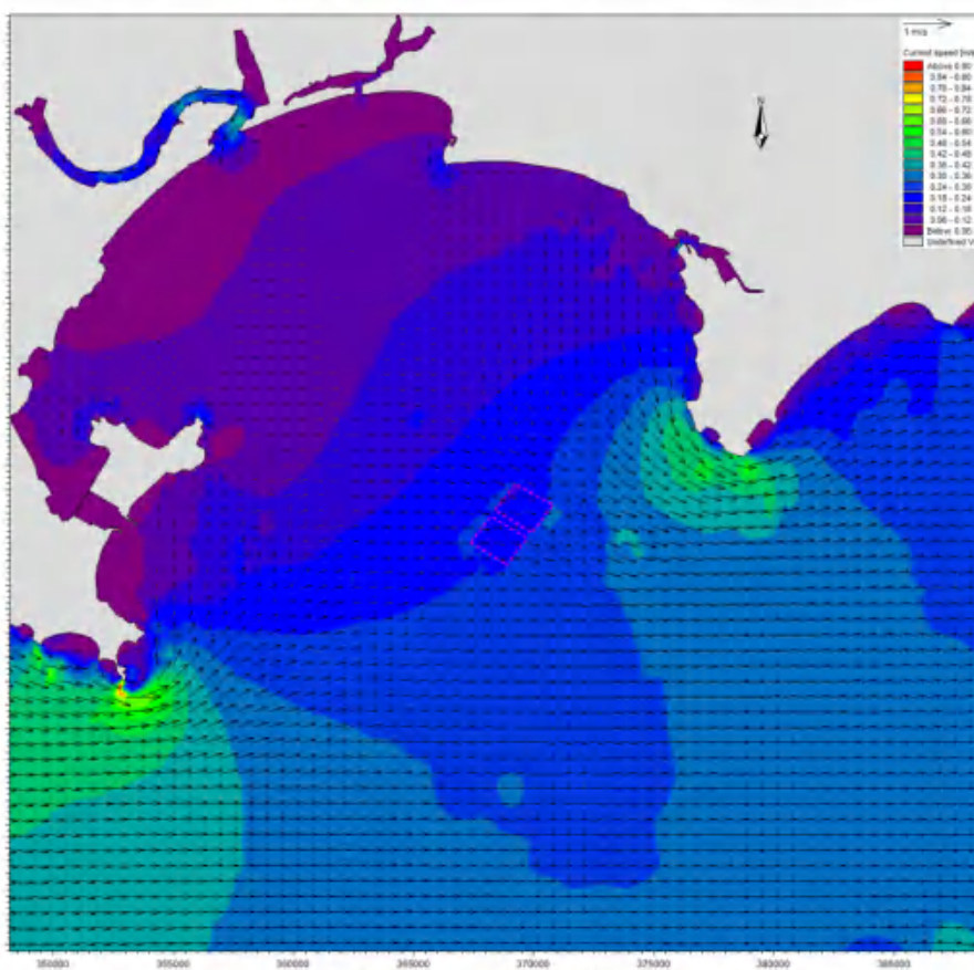
图 6.1.3-11e 工程实施后冬季大潮落急流场图（中层）
