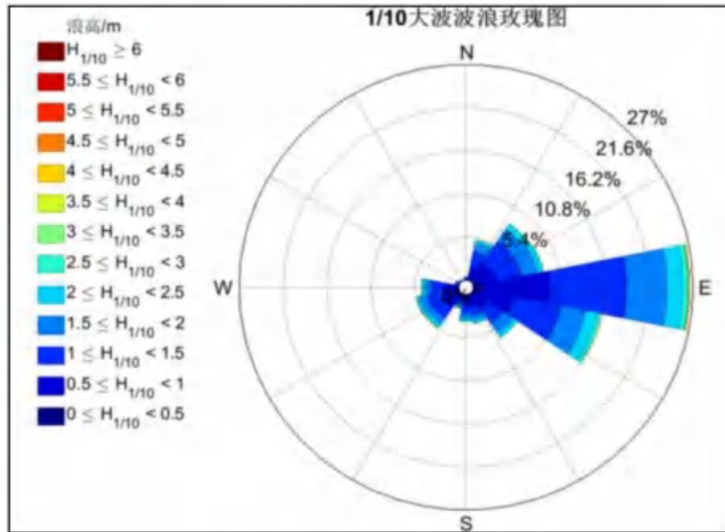
图 4.1.2-1 遮浪站波浪玫瑰图
