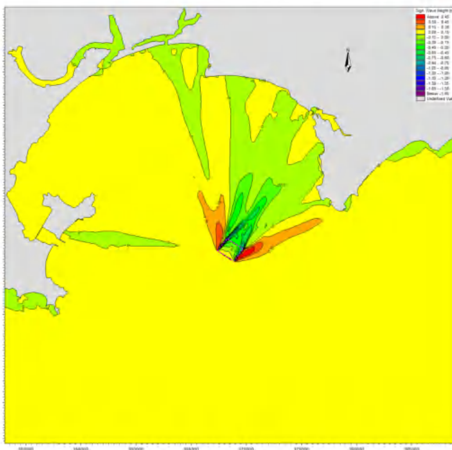
图 6.3.4-2c 砂区实施前后 SW 向 50 年一遇 H_{13} 波高变化等值线图
