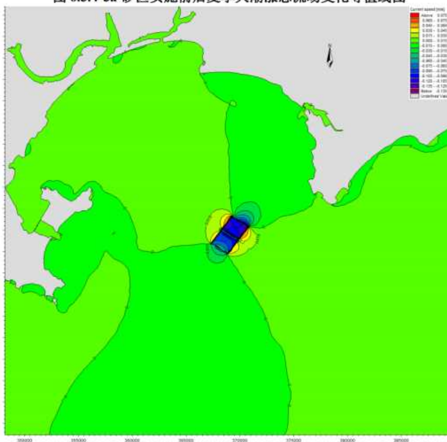
图 6.3.4-3b 砂区实施前后夏季大潮落急流场变化等值线图
