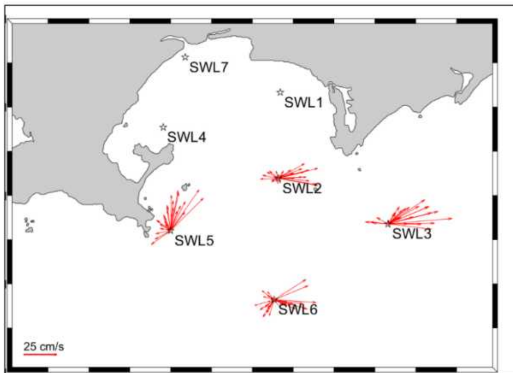
图 5.5.4-3 冬季 0.4H 层海流平面分布矢量图
