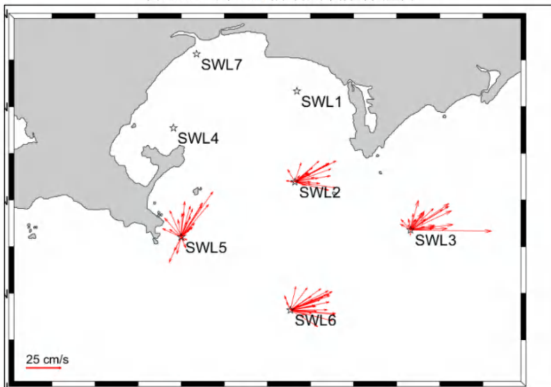
图 5.5.4-6 冬季底层海流平面分布矢量图
