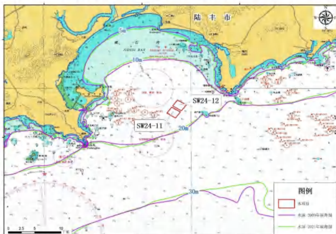
图 5.6.2-1 项目所在海域冲淤变化
