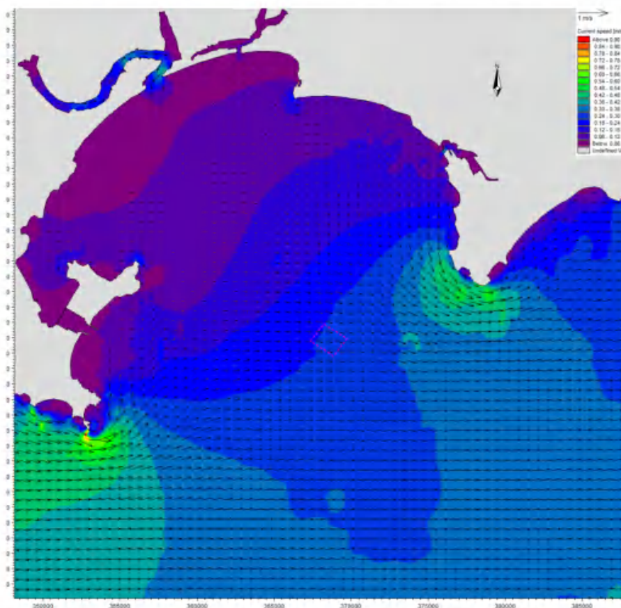
图 6.1.2-2e 现状条件下工程海域冬季大潮落急流场（中层）
