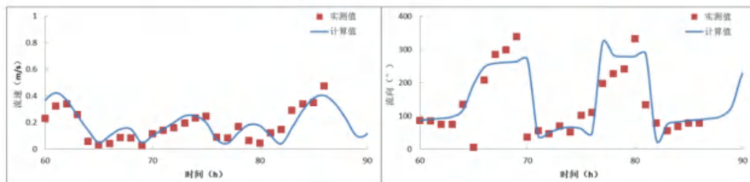
图 6.1.1-5h 夏季 SWL3 站流速、流向验证 (0.6 层)
