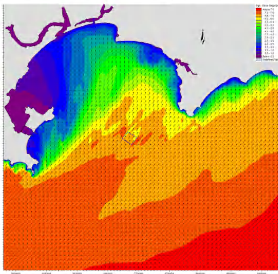
图 6.2.3-1c 工程后 50 年一遇 SW 向波高分布图
