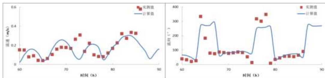
图 6.1.1-7i 冬季 SWL3 站流速、流向验证 (底层)
