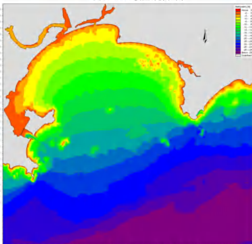
图 6.1.1-1b 工程前采砂区水深地形图
