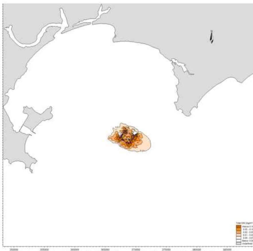
图 6.4.2-5c 夏季海砂分选典型工况产生悬沙增量包络线图（底层）
