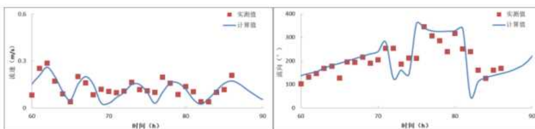
图 6.1.1-5a 夏季 SWL1 站流速、流向验证（表层）
