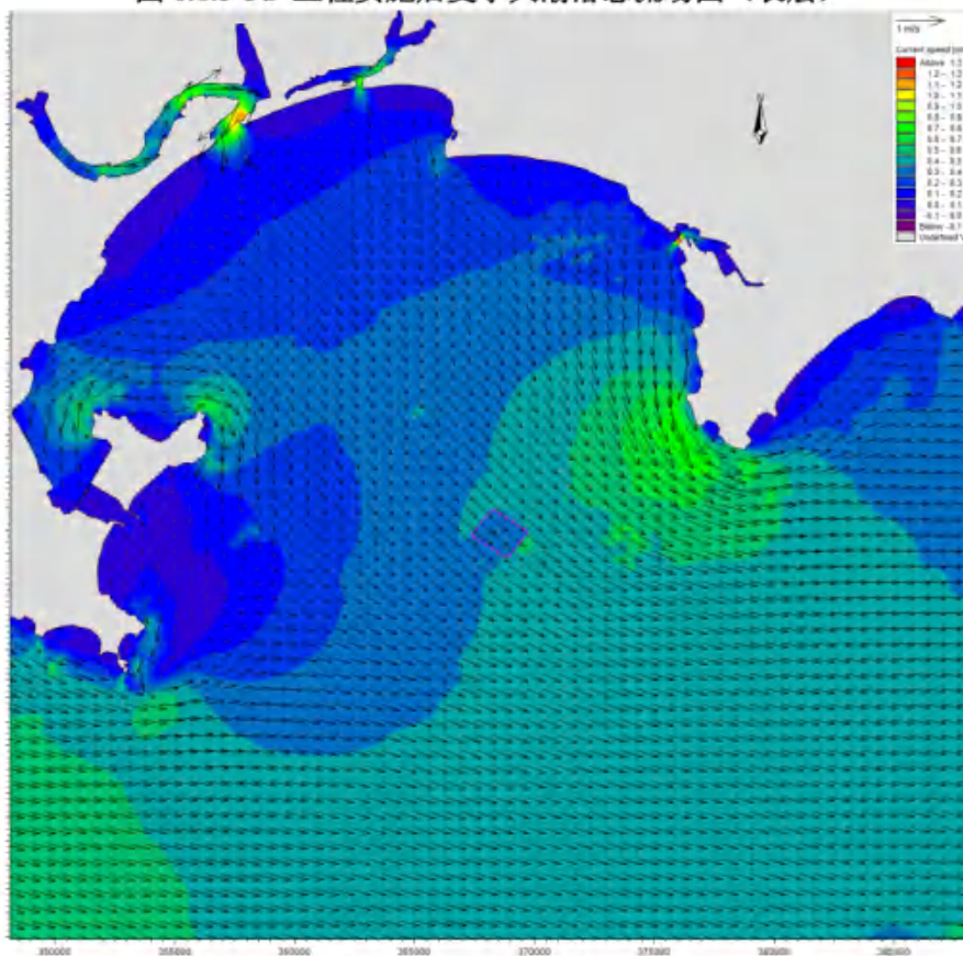
图 6.1.3-3e 工程实施后夏季大潮落急流场图（中层）
