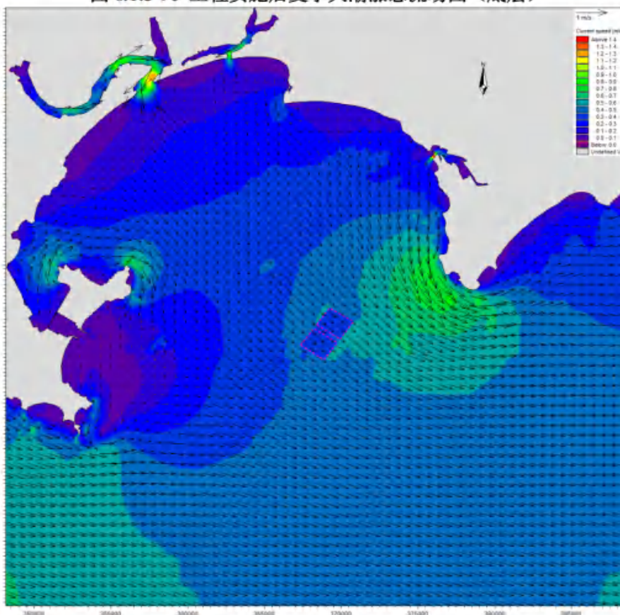
图 6.1.3-9d 工程实施后夏季大潮落急流场图（表层）
