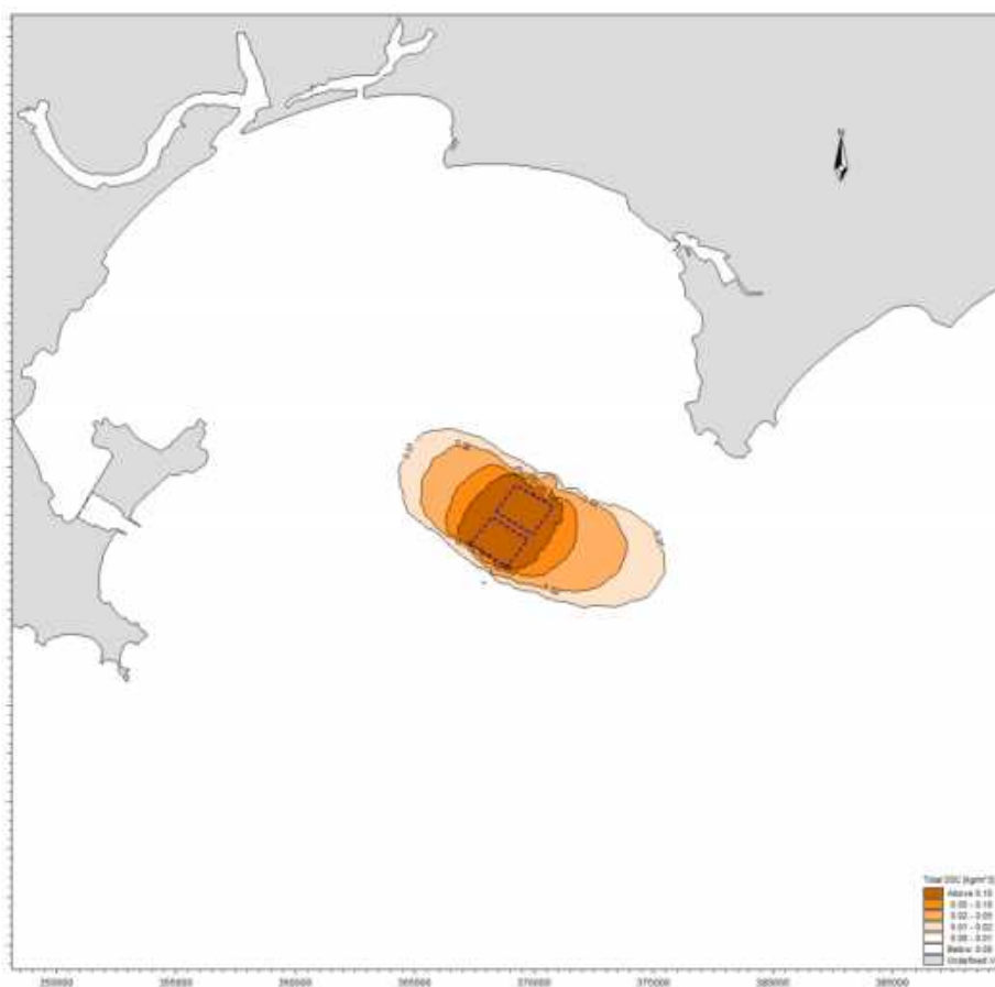
图 6.4.3-3c 夏季海砂分选最大包络线产生悬沙增量包络线图（底层）（2 个矿区）
