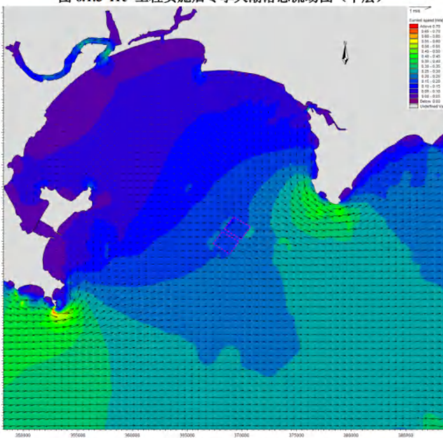
图 6.1.3-11f 工程实施后冬季大潮落急流场图（底层）
