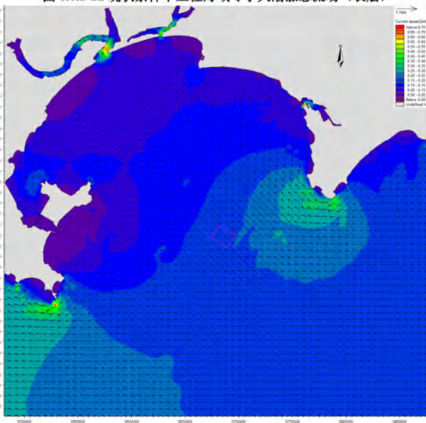
图 6.1.2-2b 现状条件下工程海域冬季大潮涨急流场（中层）
