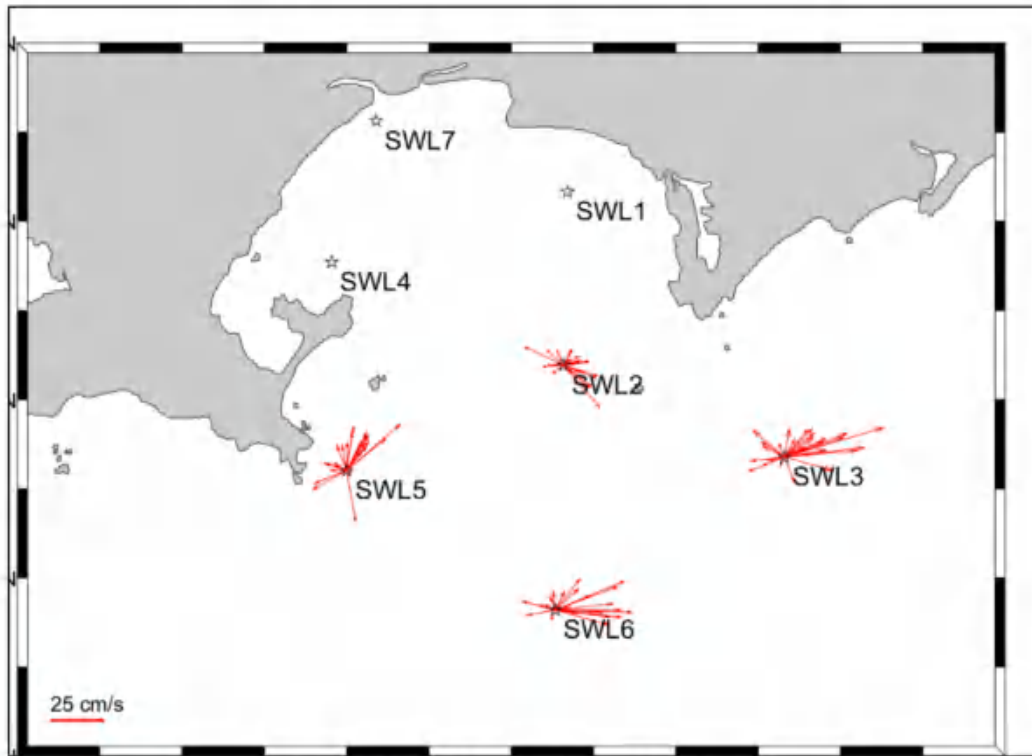
图 5.5.4-12 夏季底层海流平面分布矢量图
