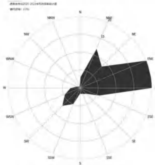
图 4.1.1-2 遮浪站风向玫瑰图
