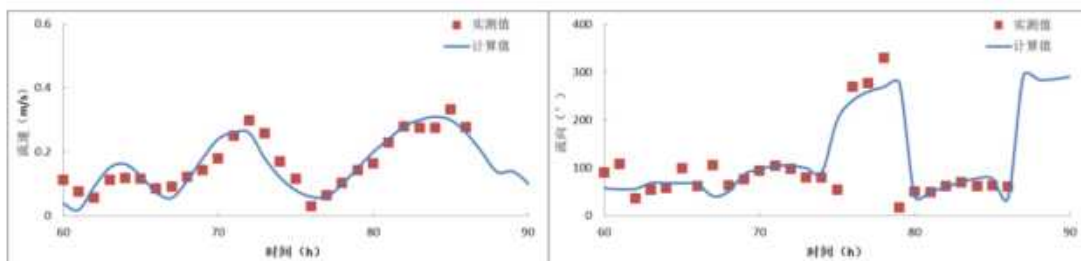
图 6.1.1-7f 冬季 SWL2 站流速、流向验证 (底层)
