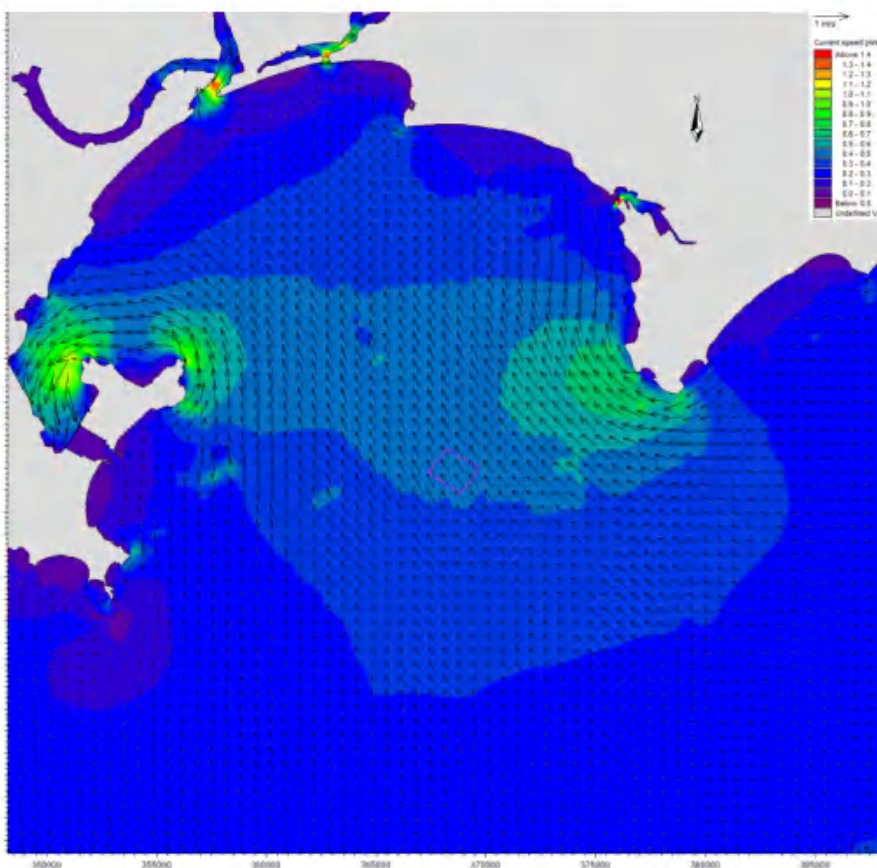
图 6.1.2-1a 现状条件下工程海域夏季大潮涨急流场（表层）
