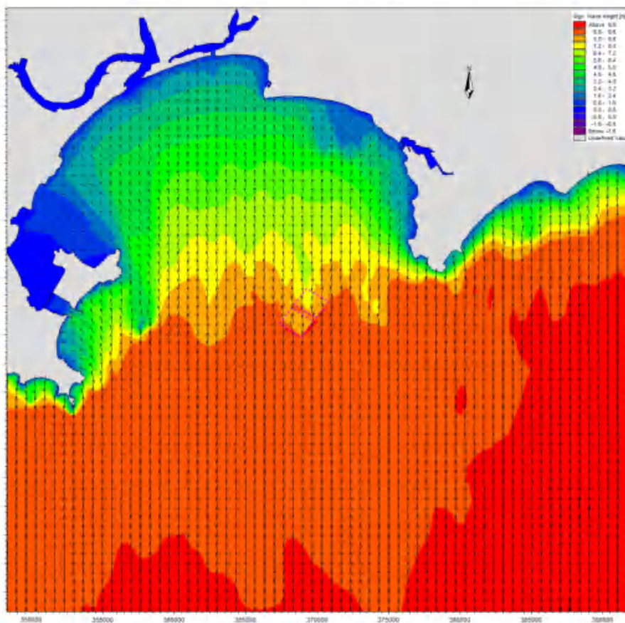
图 6.2.3-2b 工程后 50 年一遇 S 向波高分布图
