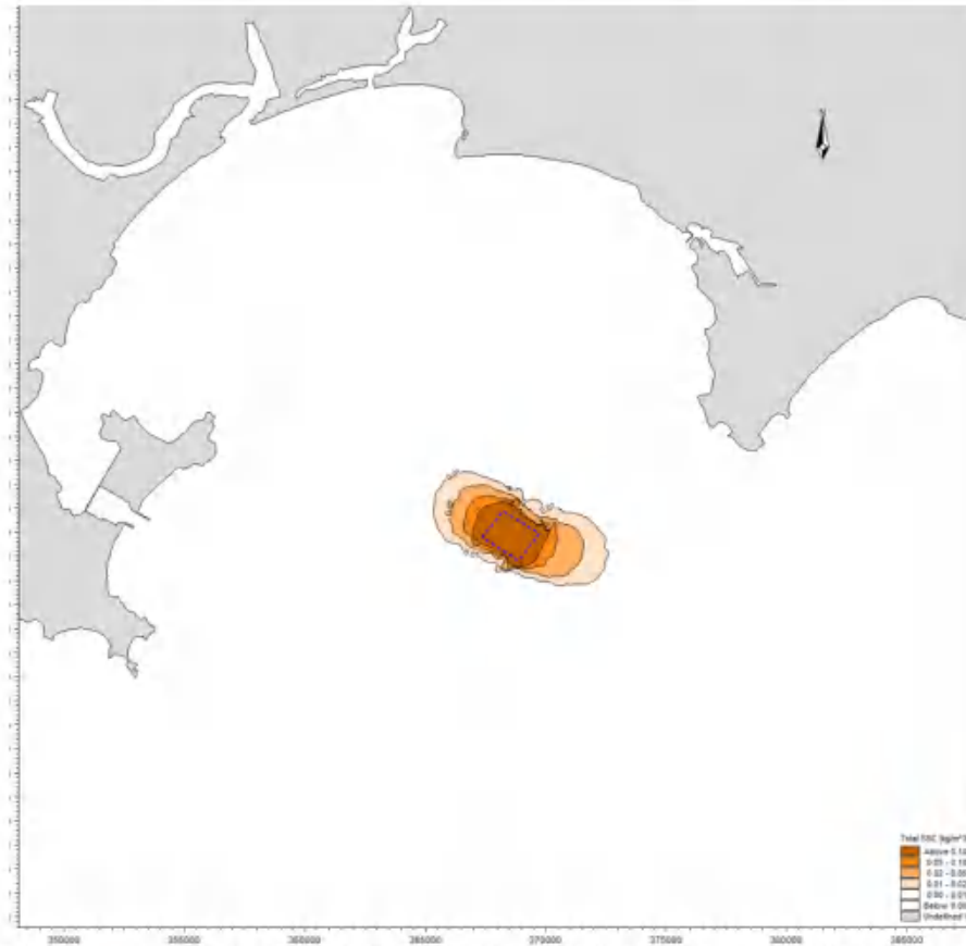
图 6.4.2-4c 冬季海砂分选最大包络线工况产生悬沙增量包络线图（底层）
