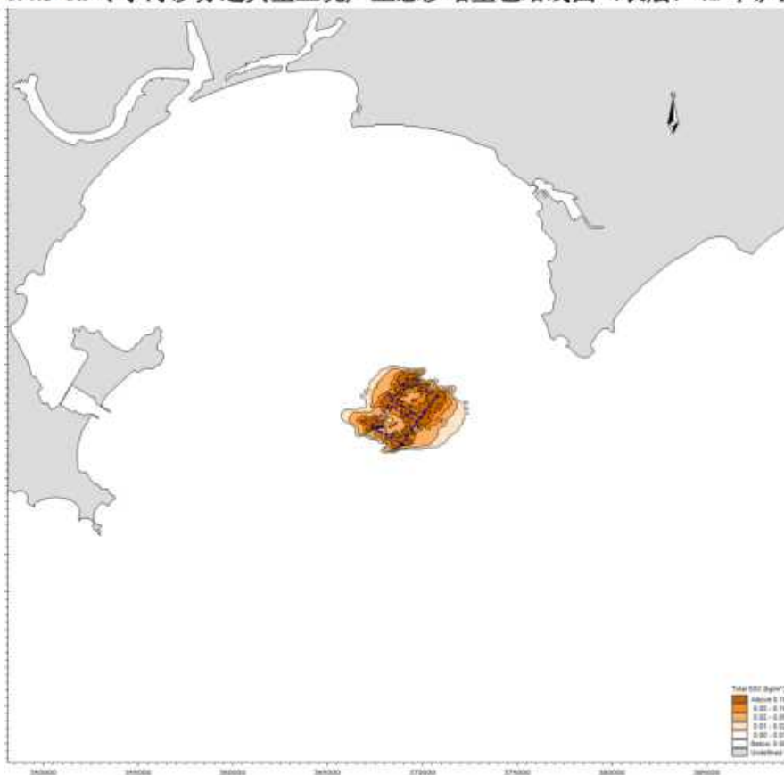
图 6.4.3-6b 冬季海砂分选典型工况产生悬沙增量包络线图（中层）（2 个矿区）
