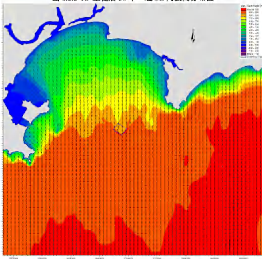
图 6.2.3-1b 工程后 50 年一遇 S 向波高分布图
