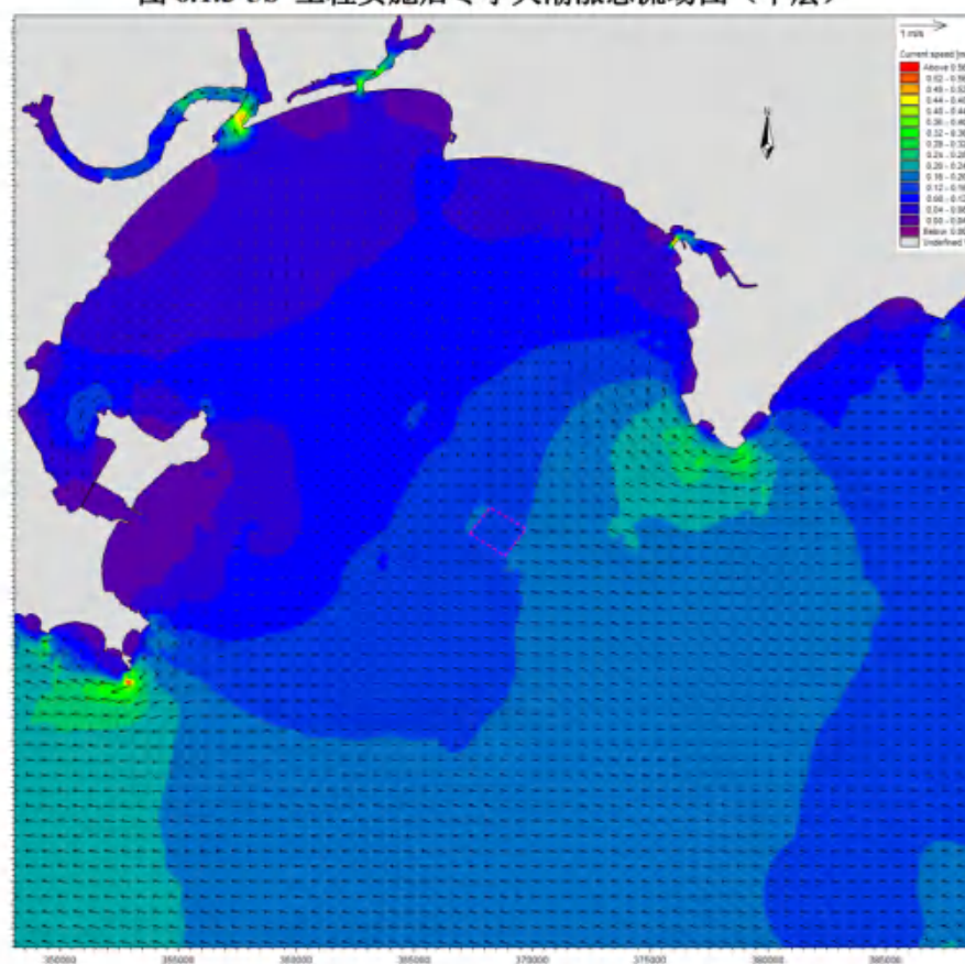
图 6.1.3-5c 工程实施后冬季大潮涨急流场图（底层）
