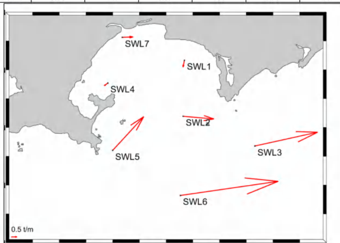
图 5.5.8-2 夏季净输沙示意图
