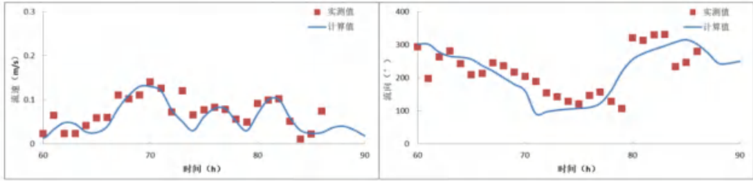
图 6.1.1-7l 冬季 SWL4 站流速、流向验证 (底层)
