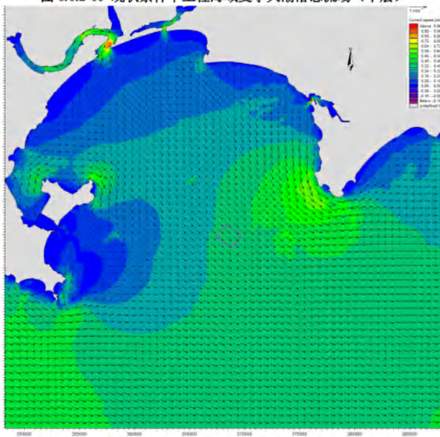
图 6.1.2-1f 现状条件下工程海域夏季大潮落急流场（底层）
