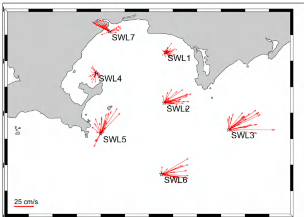
图 5.5.4-5 冬季 0.8H 层海流平面分布矢量图
