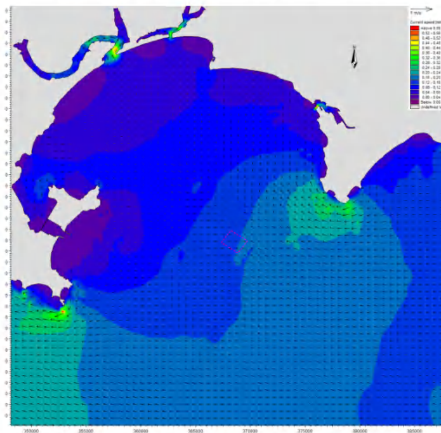
图 6.1.2-2c 现状条件下工程海域冬季大潮涨急流场（底层）
