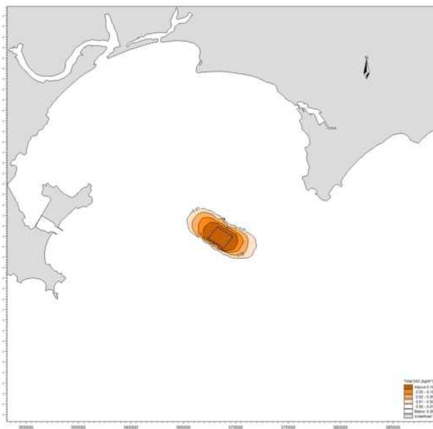
图 6.4.2-3b 夏季海砂分选最大包络线工况产生悬沙增量包络线图（中层）
