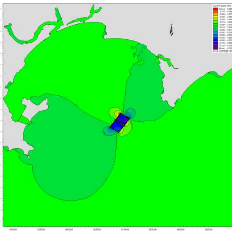
图 6.3.4-3a 砂区实施前后夏季大潮涨急流场变化等值线图
