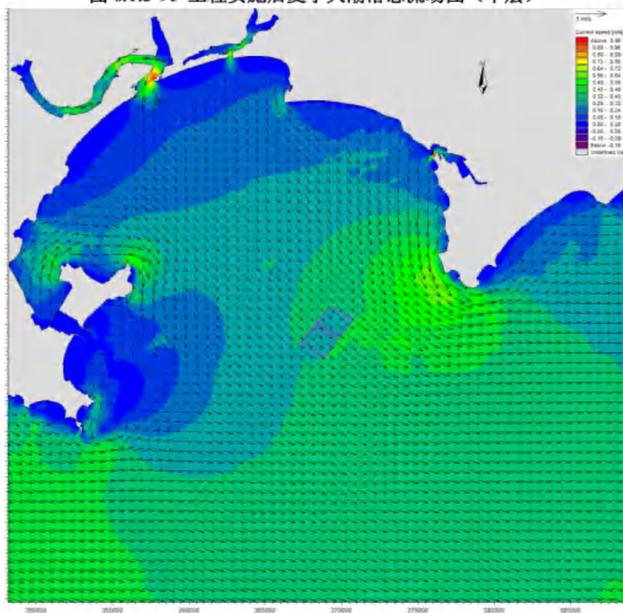
图 6.1.3-9f 工程实施后夏季大潮落急流场图（底层）
