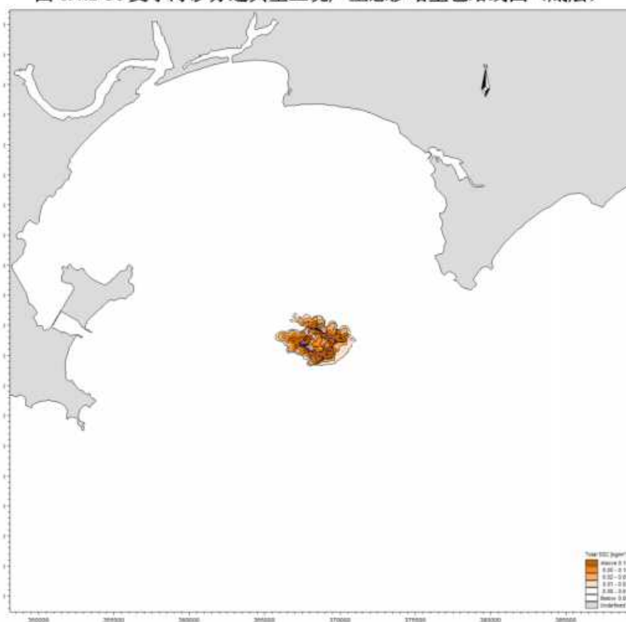
图 6.4.2-6a 冬季海砂分选典型工况产生悬沙增量包络线图（表层）
