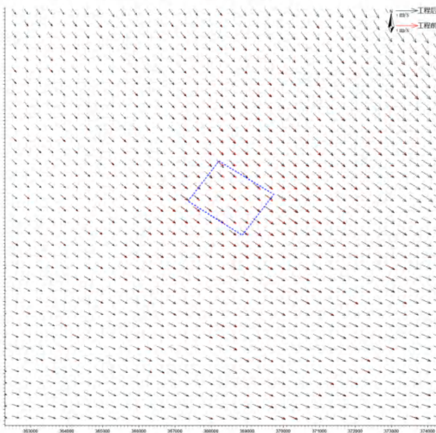
图 6.1.3-4b 工程实施前后夏季大潮落急流场对比图（中层）
