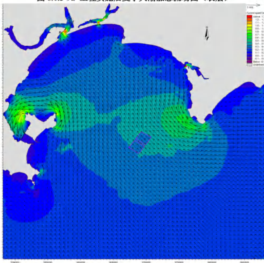
图 6.1.3-9b 工程实施后夏季大潮涨急流场图（中层）
