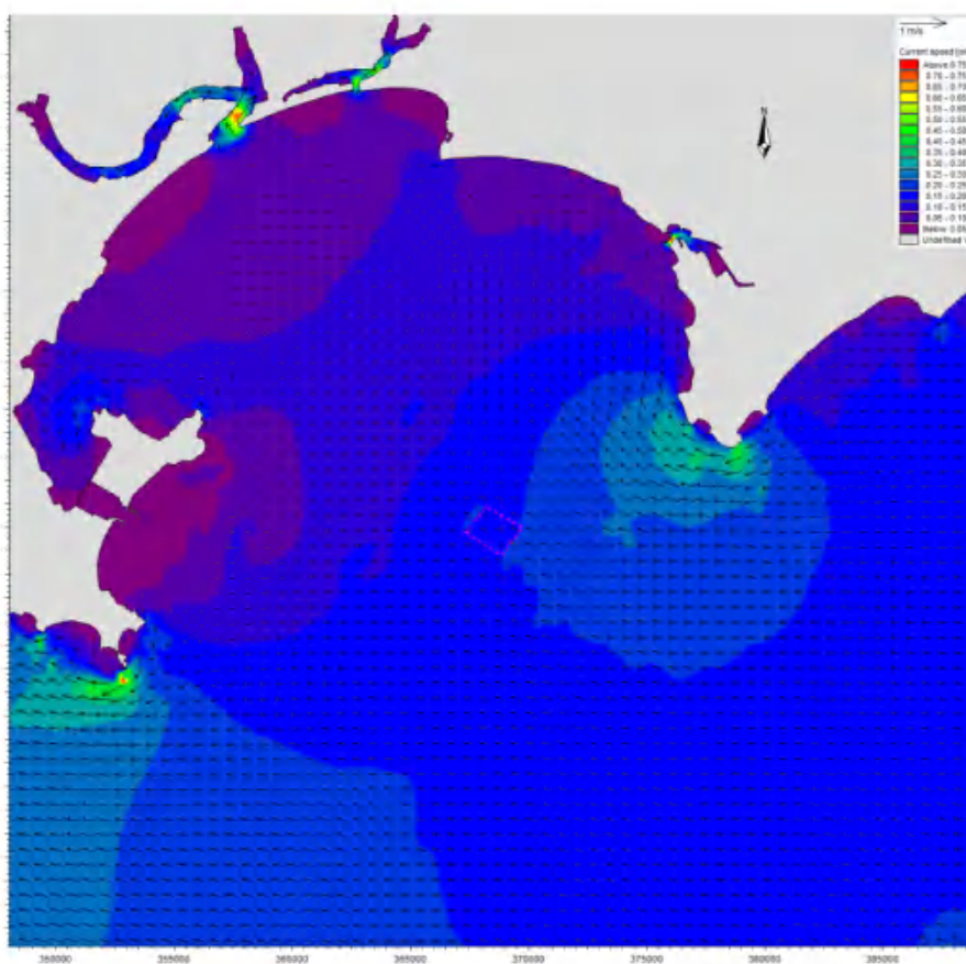
图 6.1.3-5a 工程实施后冬季大潮涨急流场图（表层）
