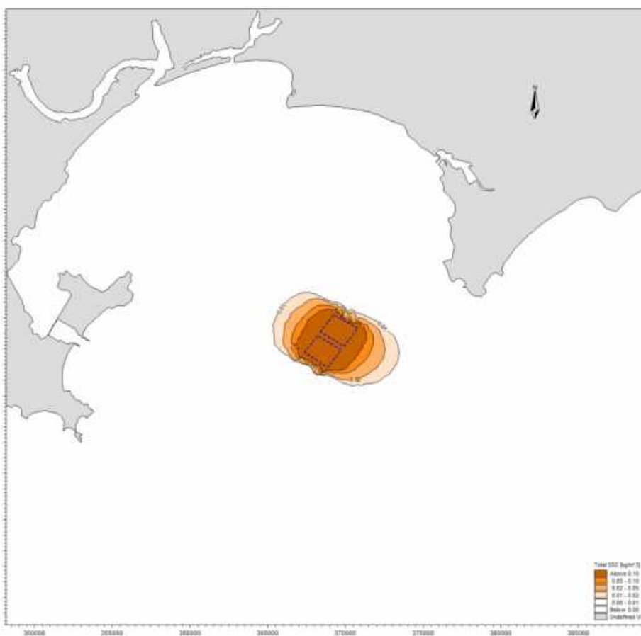
图 6.4.3-4a 冬季海砂分选最大包络线产生悬沙增量包络线图（表层）（2 个矿区）
