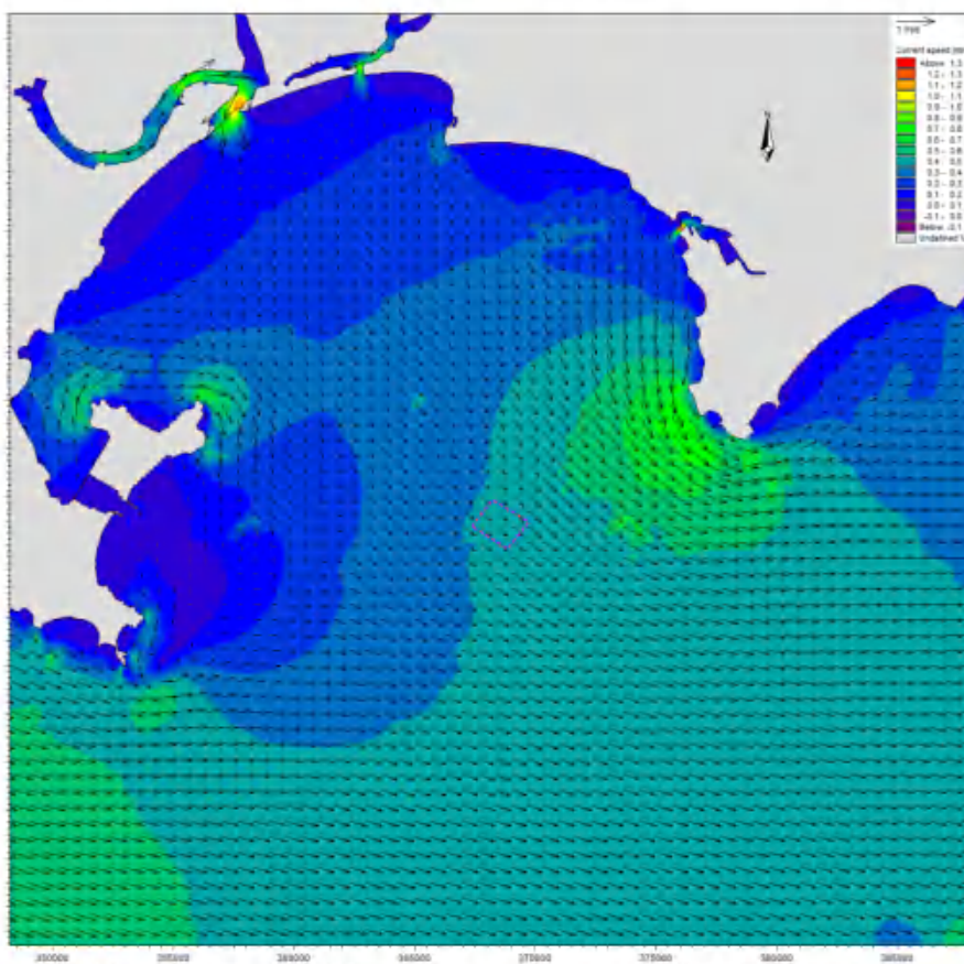
图 6.1.2-1e 现状条件下工程海域夏季大潮落急流场（中层）
