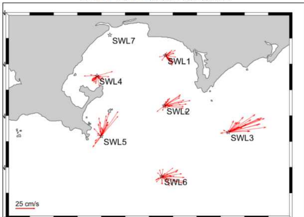
图 5.5.4-4 冬季 0.6H 层海流平面分布矢量图
