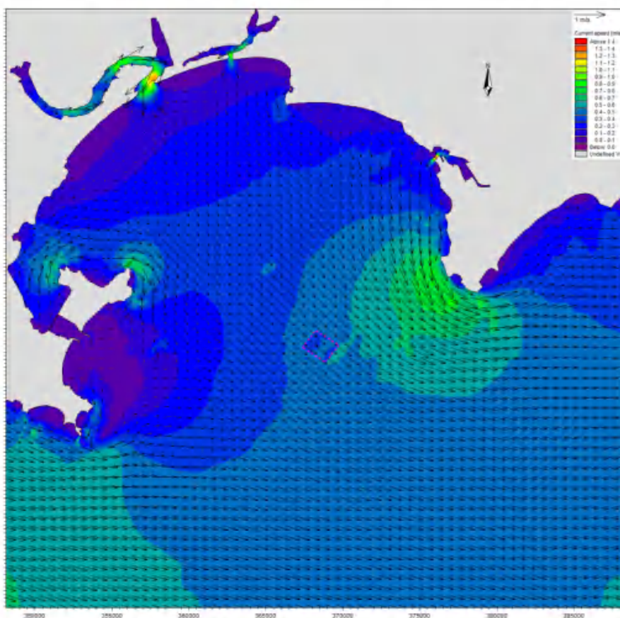
图 6.1.3-3d 工程实施后夏季大潮落急流场图（表层）
