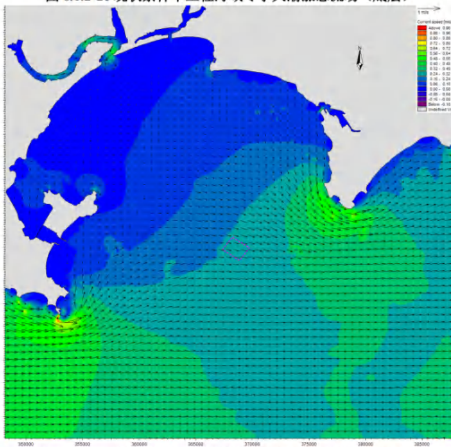
图 6.1.2-2d 现状条件下工程海域冬季大潮落急流场（表层）
