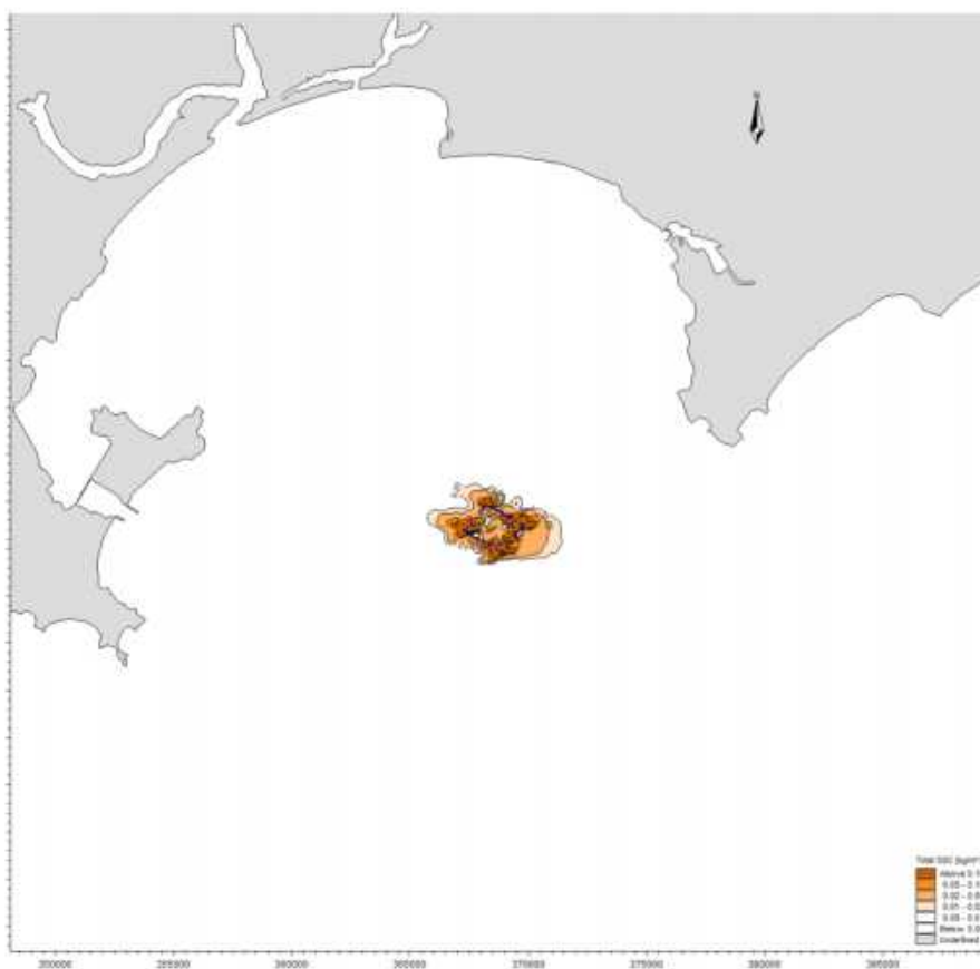
图 6.4.2-6b 冬季海砂分选典型工况产生悬沙增量包络线图（中层）
