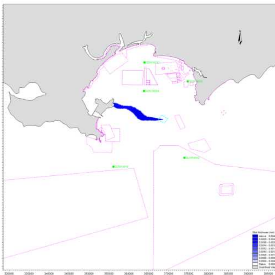
图 7.5.1-1 工况 1 溢油扫海范围 (48h)
