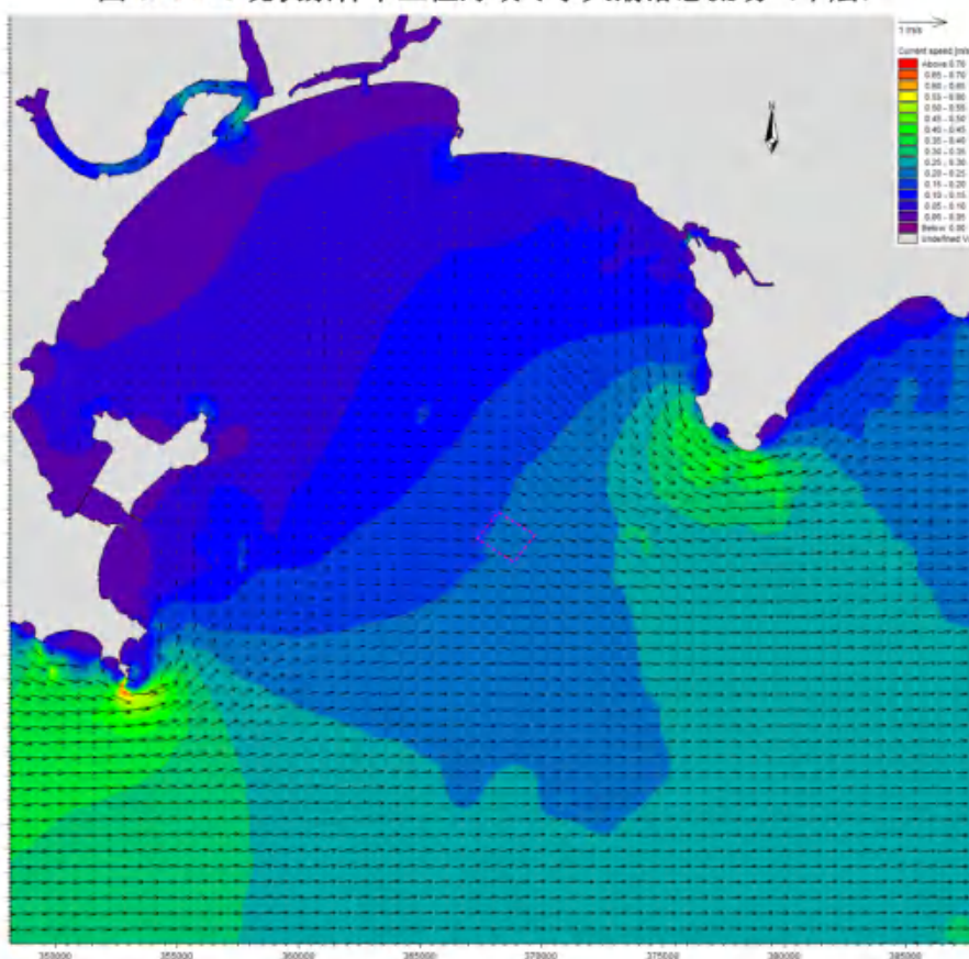
图 6.1.2-2f 现状条件下工程海域冬季大潮落急流场（底层）
