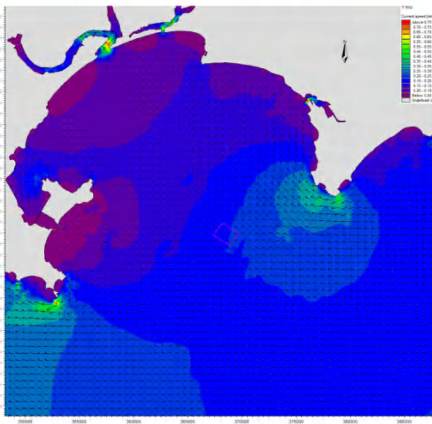
图 6.1.2-2a 现状条件下工程海域冬季大潮涨急流场（表层）
