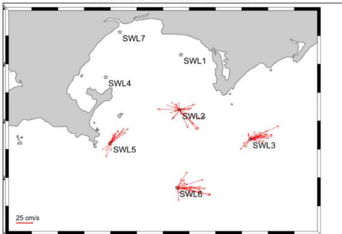
图 5.5.4-9 夏季 0.4H 层海流平面分布矢量图
