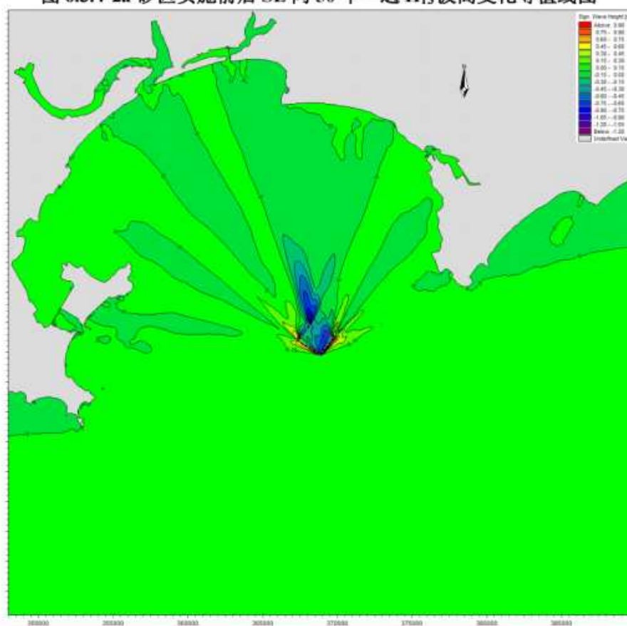
图 6.3.4-2b 砂区实施前后 S 向 50 年一遇 H_{13} 波高变化等值线图
