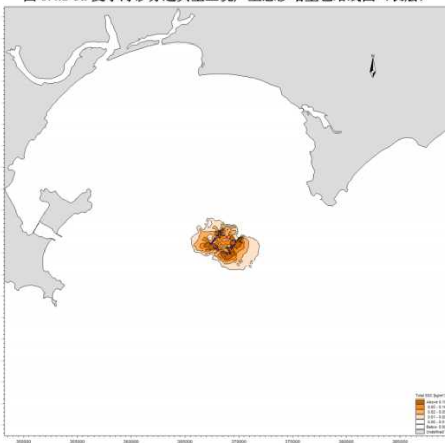
图 6.4.2-5b 夏季海砂分选典型工况产生悬沙增量包络线图（中层）
