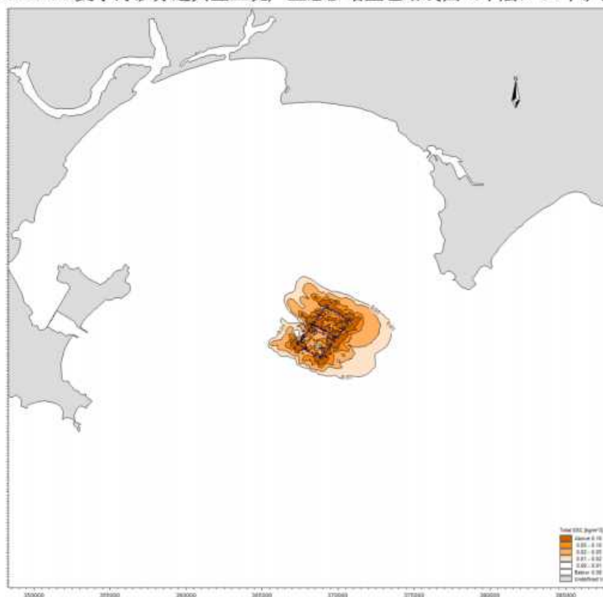
图 6.4.3-5c 夏季海砂分选典型工况产生悬沙增量包络线图（底层）（2 个矿区）
