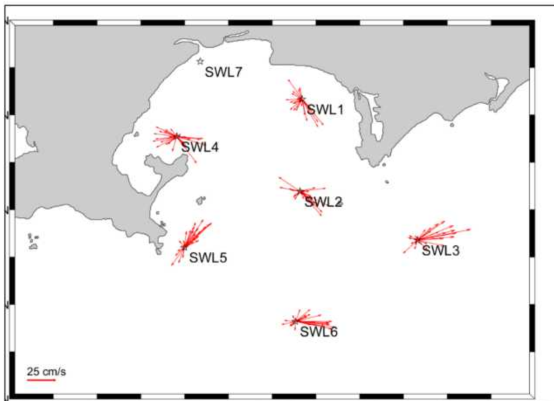
图 5.5.4-10 夏季 0.6H 层海流平面分布矢量图
