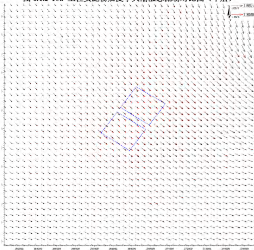
图 6.1.3-10b 工程实施前后夏季大潮落急流场对比图（中层）
