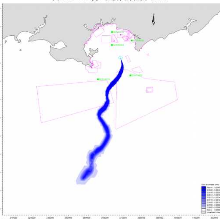
图 7.5.1-8 工况 8 溢油扫海范围 (48h)
