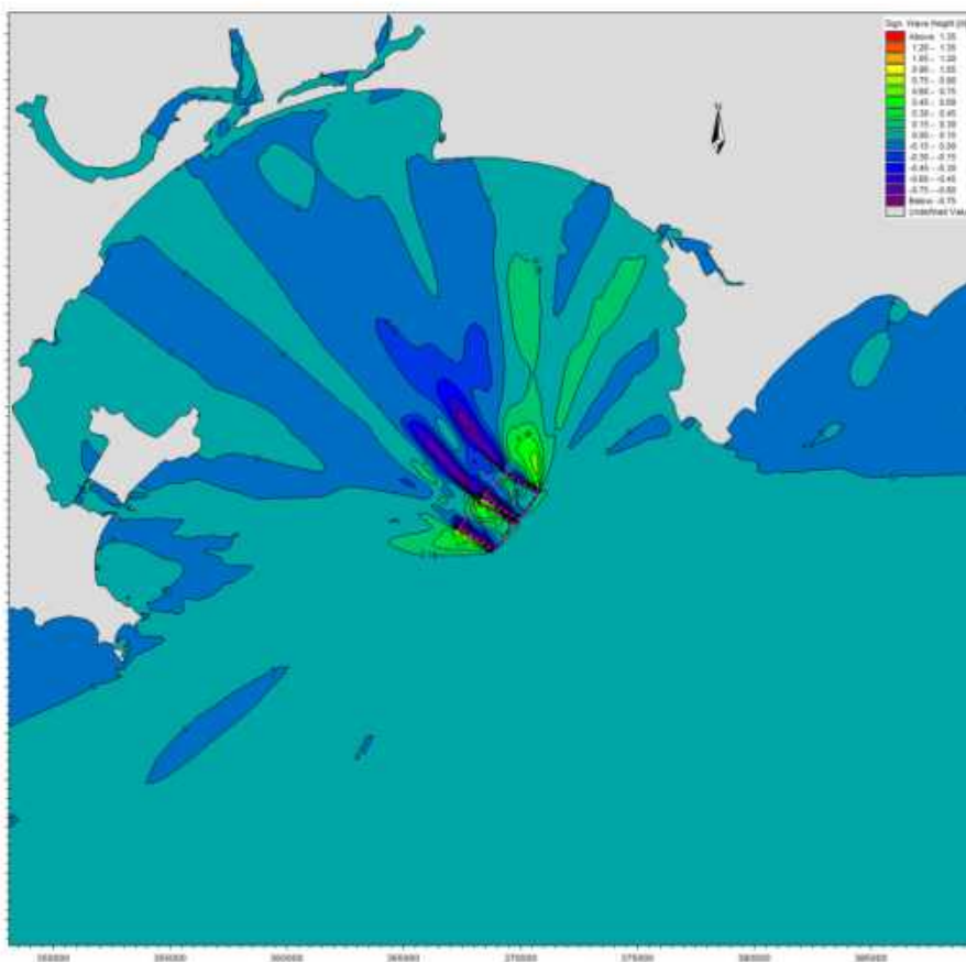
图 6.3.4-4a 砂区实施前后 SE 向 50 年一遇 H_{13} 波高变化等值线图
