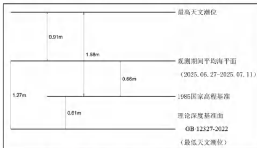
图 5.5.3-12 SWC2 临时潮位站各基准面的相互关系
