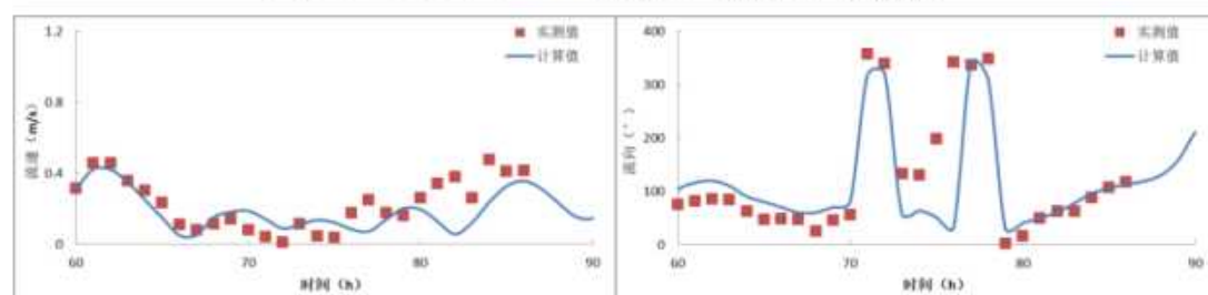
图 6.1.1-5d 夏季 SWL2 站流速、流向验证（表层）
