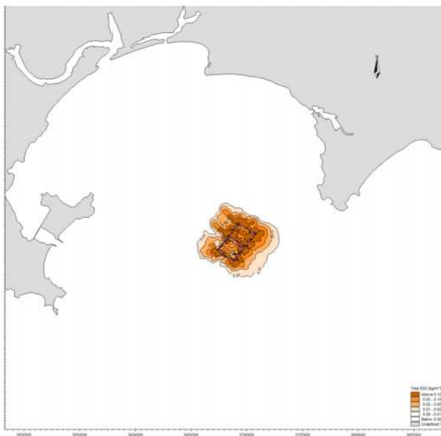
图 6.4.3-5b 夏季海砂分选典型工况产生悬沙增量包络线图（中层）（2 个矿区）
