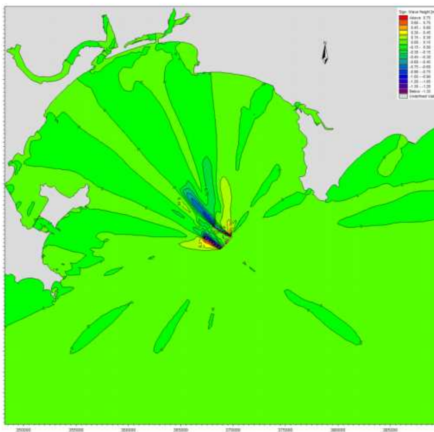
图 6.3.4-2a 砂区实施前后 SE 向 50 年一遇 H_{13} 波高变化等值线图
