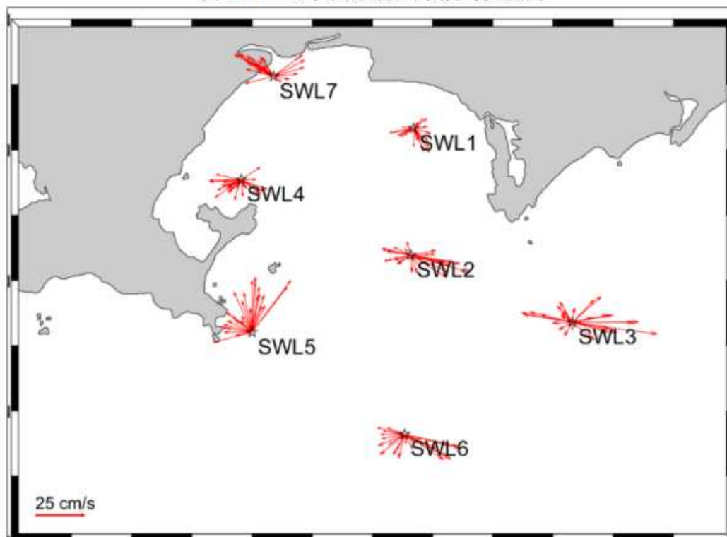
图 5.5.4-2 冬季 0.2H 层海流平面分布矢量图
