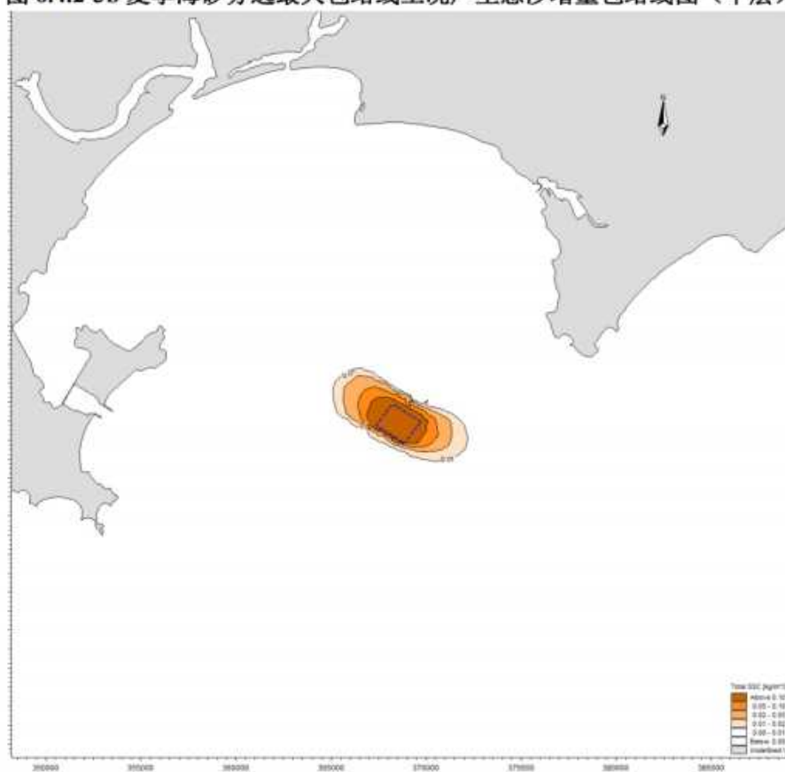
图 6.4.2-3c 夏季海砂分选最大包络线工况产生悬沙增量包络线图（底层）
