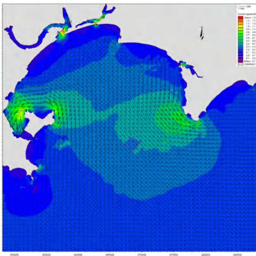
图 6.1.3-3b 工程实施后夏季大潮涨急流场图（中层）
