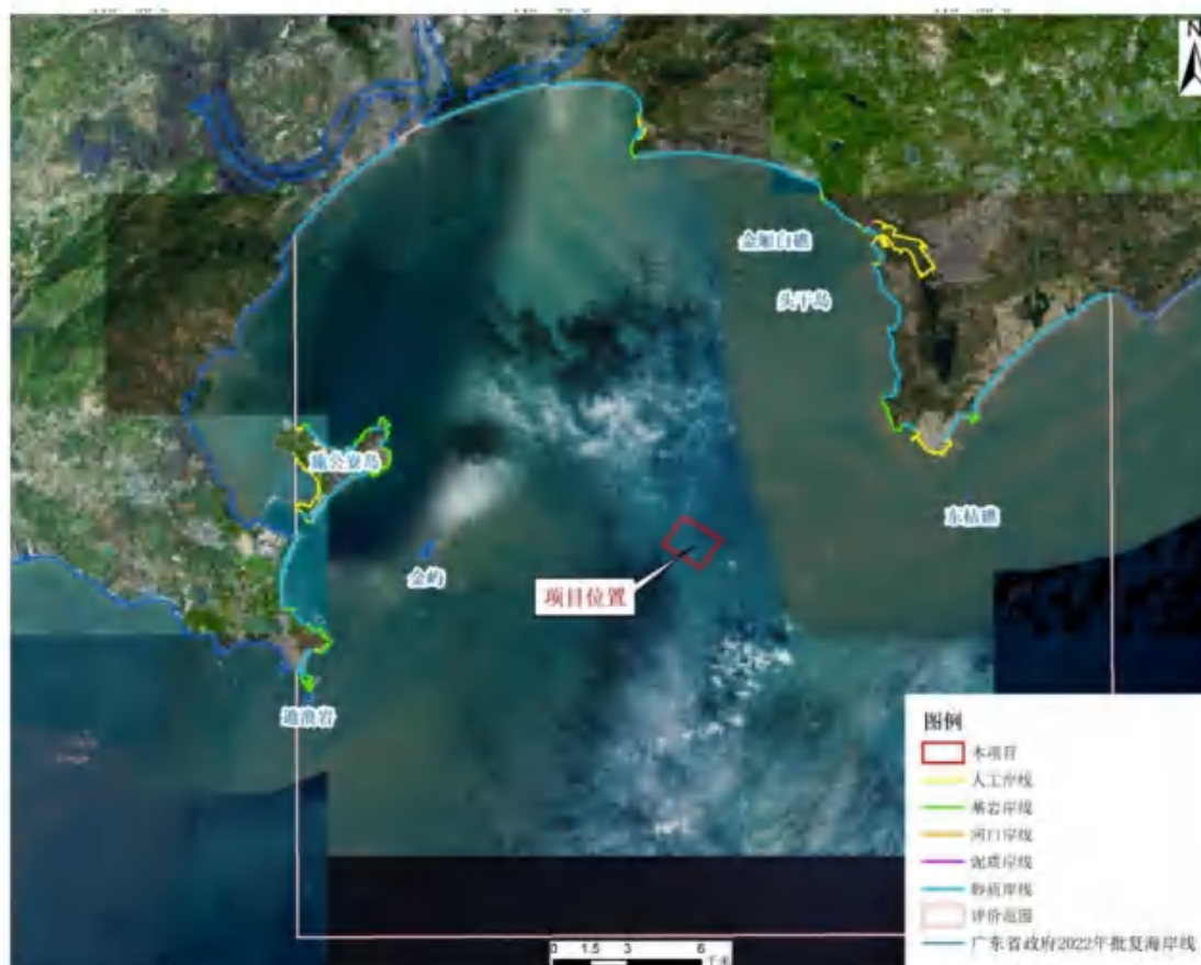
图 4.2.1-1 评价范围内岸线分布
