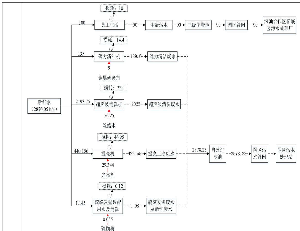
图 2 项目远期水平衡图 (t/a)
