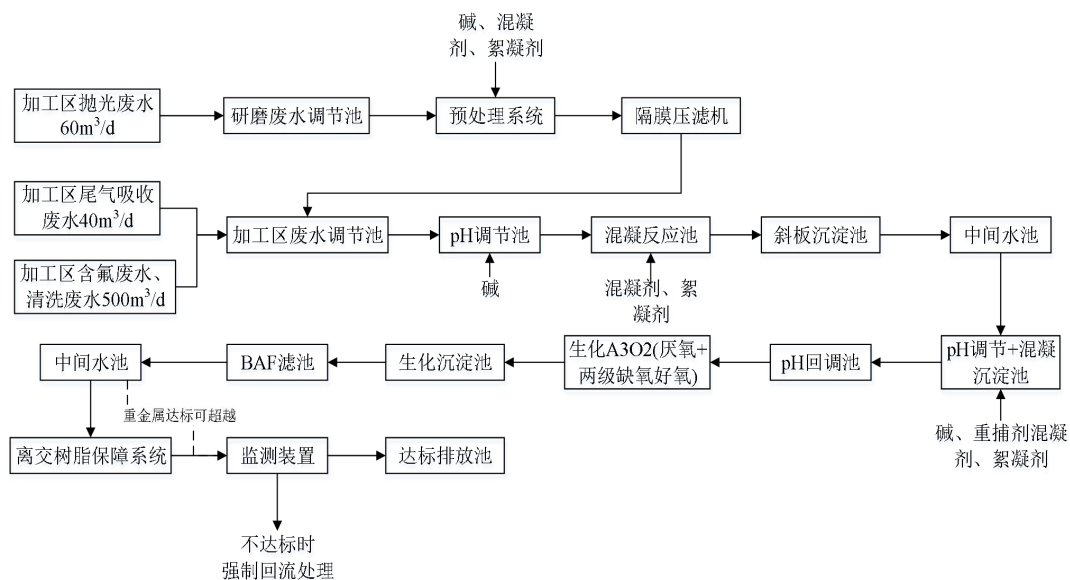
图 6 海丰首饰产业环保集聚区污水处理厂加工区废水处理工艺图
