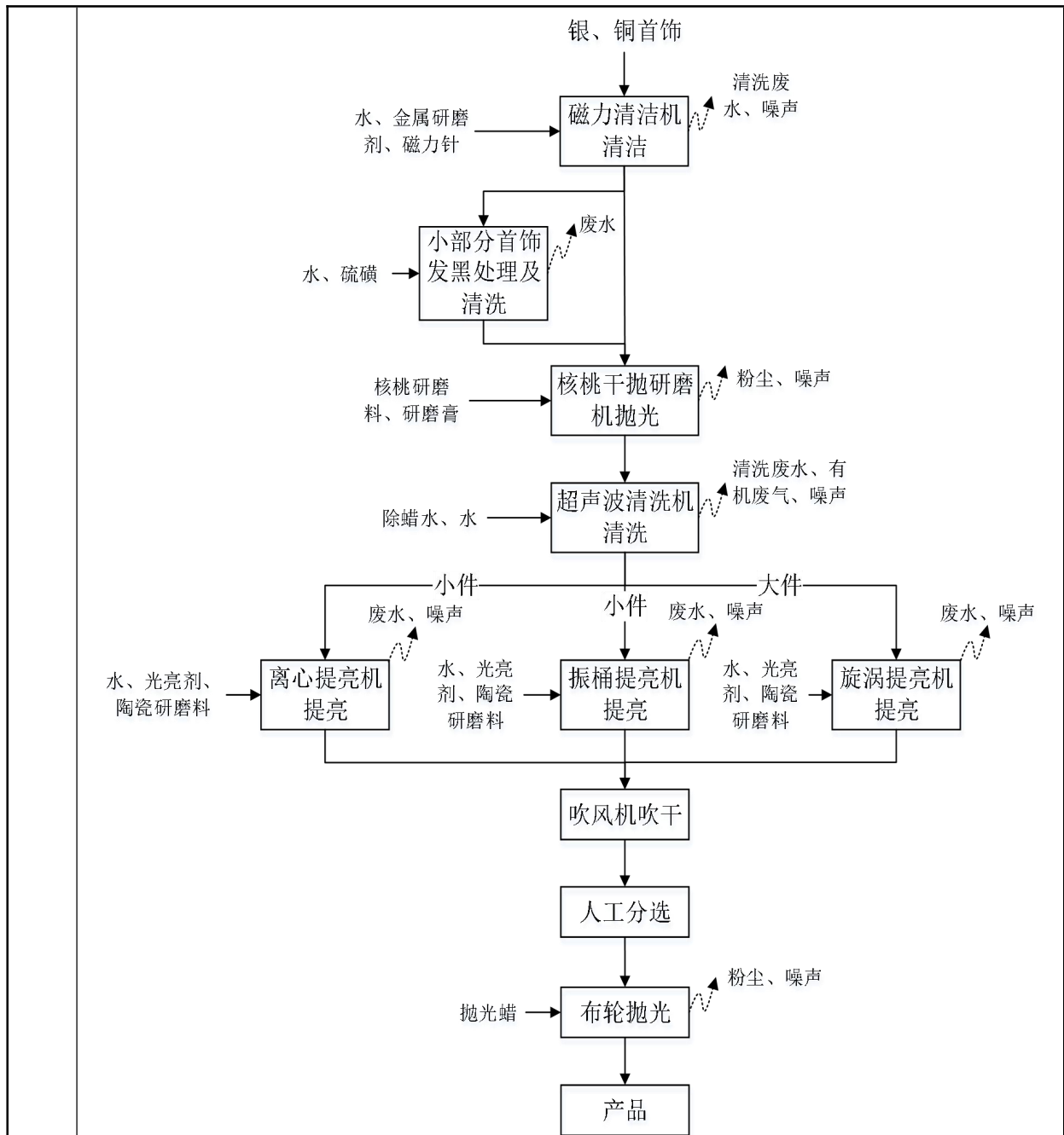
图 4 项目加工工艺流程图
