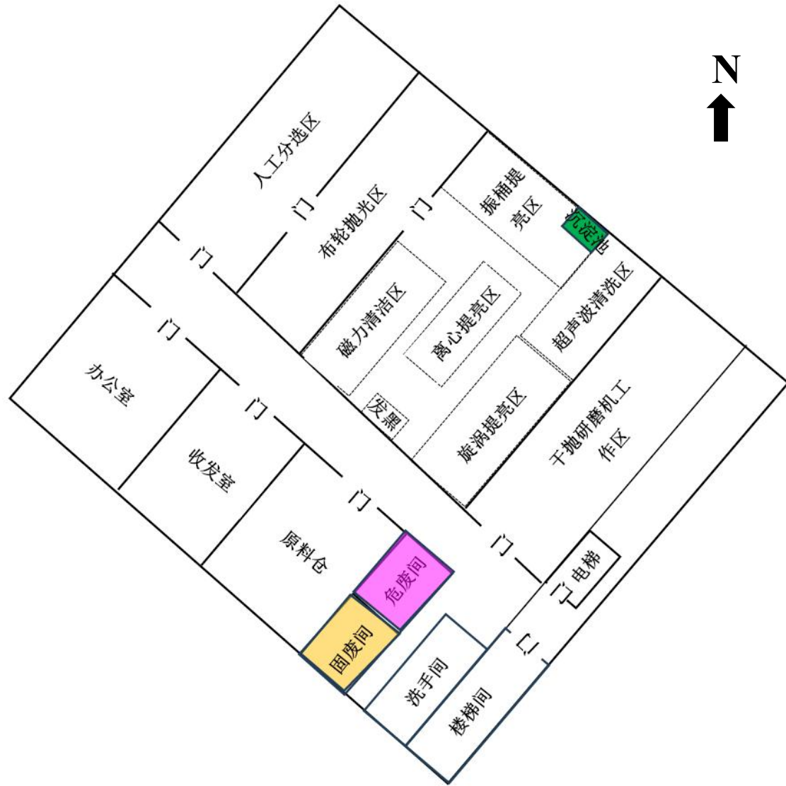
附图 5 项目车间平面布置图 (5F)
