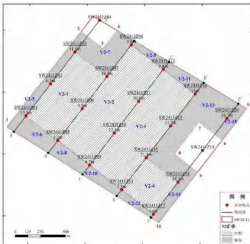
图 3.3.1-2 矿区 V2 矿体块段及资源量类型分布平面图
