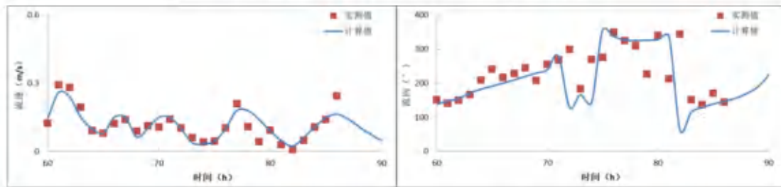
图 6.1.1-5b 夏季 SWL1 站流速、流向验证（0.6 层）
