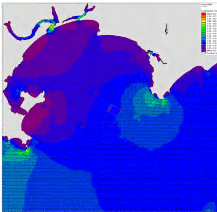
图 6.1.3-4a 工程实施后冬季大潮涨急流场图（表层）
