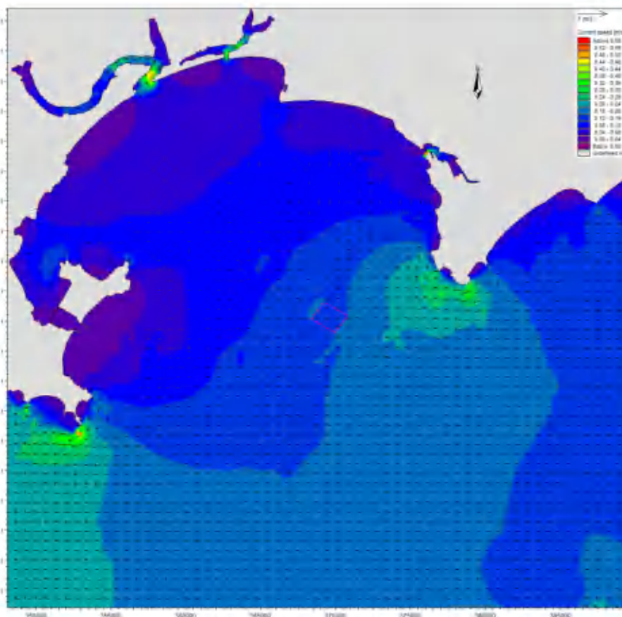
图 6.1.3-4c 工程实施后冬季大潮涨急流场图（底层）
