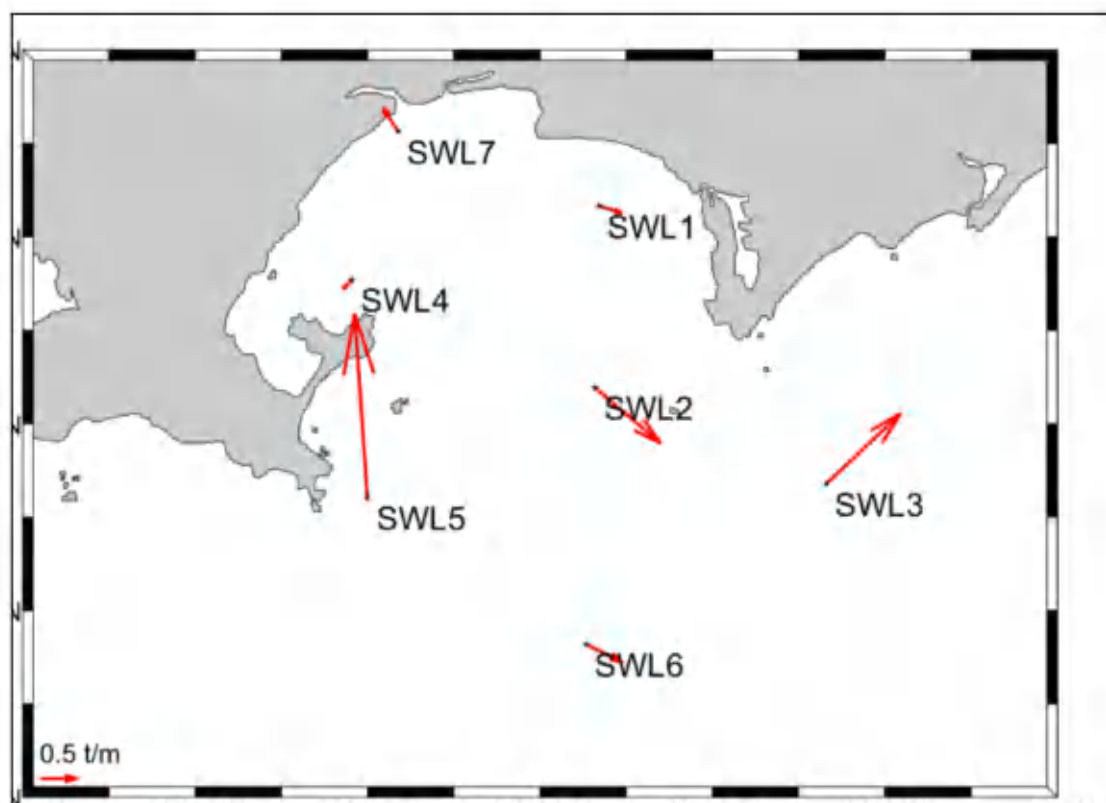
图 5.5.8-1 冬季净输沙示意图
