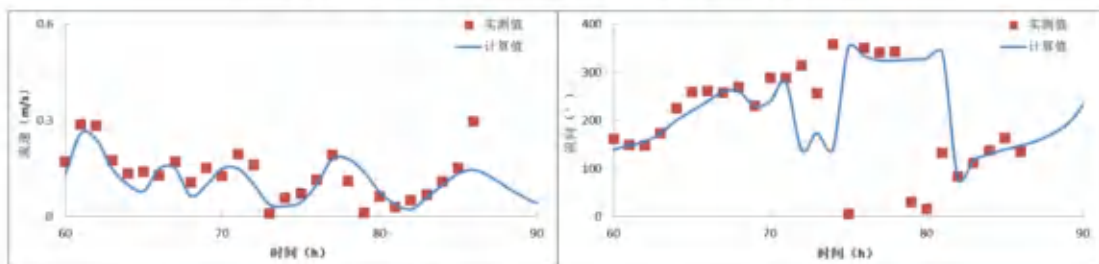
图 6.1.1-5c 夏季 SWL1 站流速、流向验证（底层）
