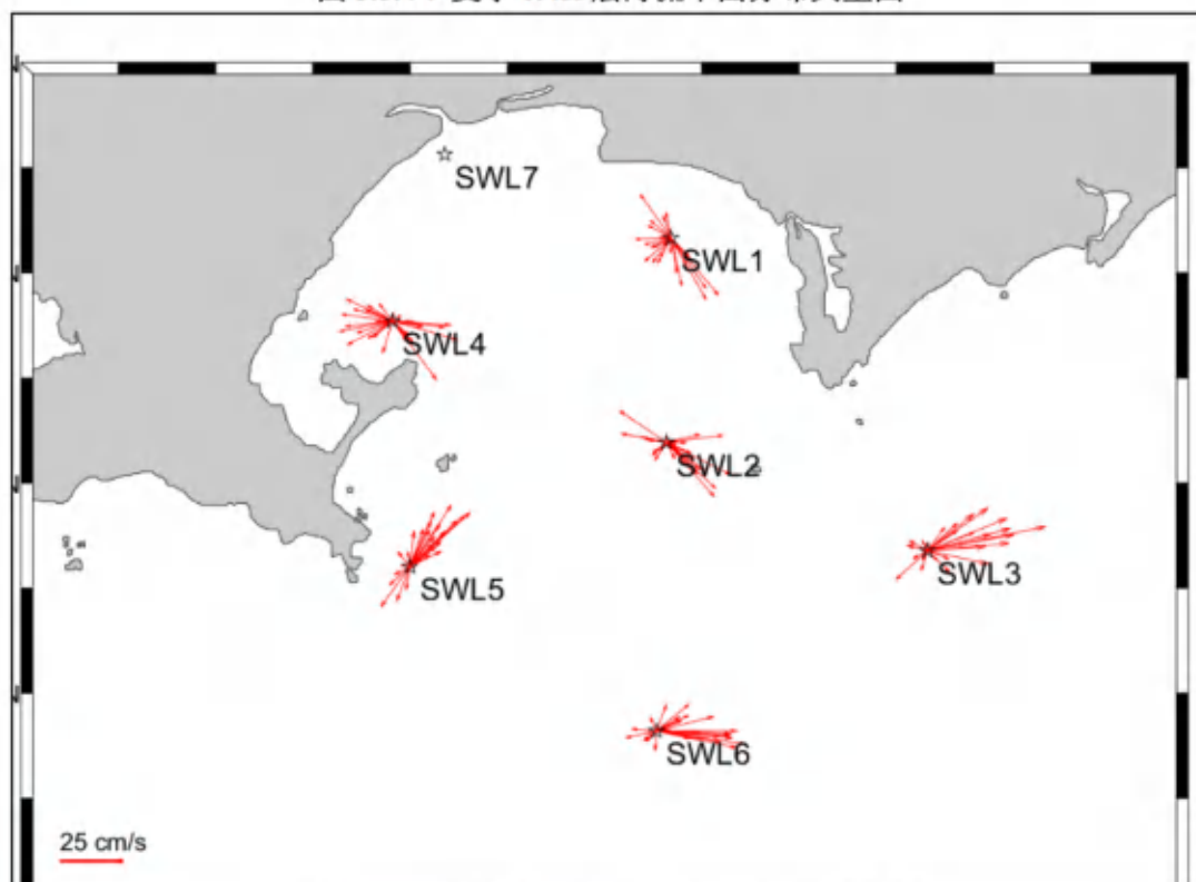
图 5.5.4-10 夏季 0.6H 层海流平面分布矢量图
