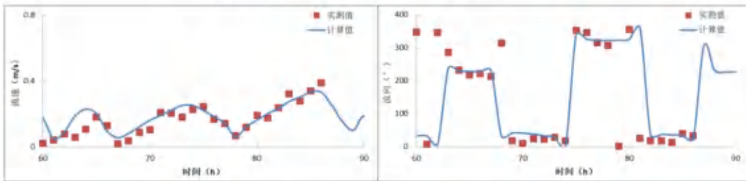
图 6.1.1-7n 冬季 SWL5 站流速、流向验证 (0.6 层)
