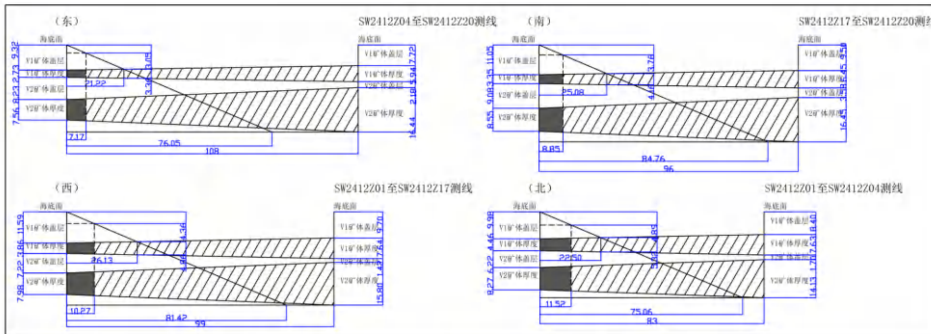
图 3.3.1-3 矿区开采剖面示意图 (图中黑色部分为不可开采矿体截面)
