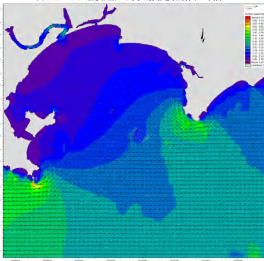
图 6.1.3-4f 工程实施后冬季大潮落急流场图（底层）
