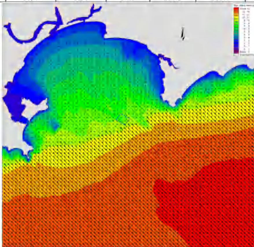
图 6.2.3-1a 工程后 50 年一遇 SE 向波高分布图
