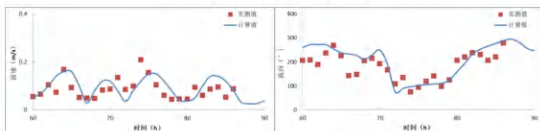
图 6.1.1-7k 冬季 SWL4 站流速、流向验证 (0.6 层)
