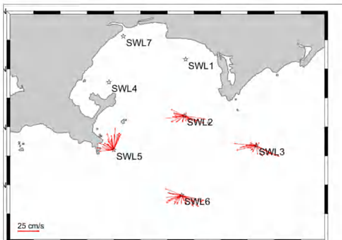
图 5.5.4-1 冬季表层海流平面分布矢量图
