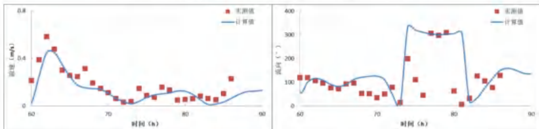
图 6.1.1-5t 夏季 SWL7 站流速、流向验证 (表层)
