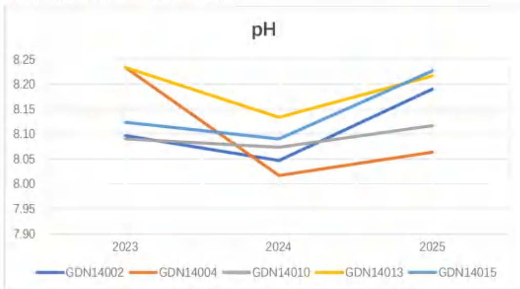
图 5.1.2-3 国控站位 2023 年~2025 年 pH 变化趋势
