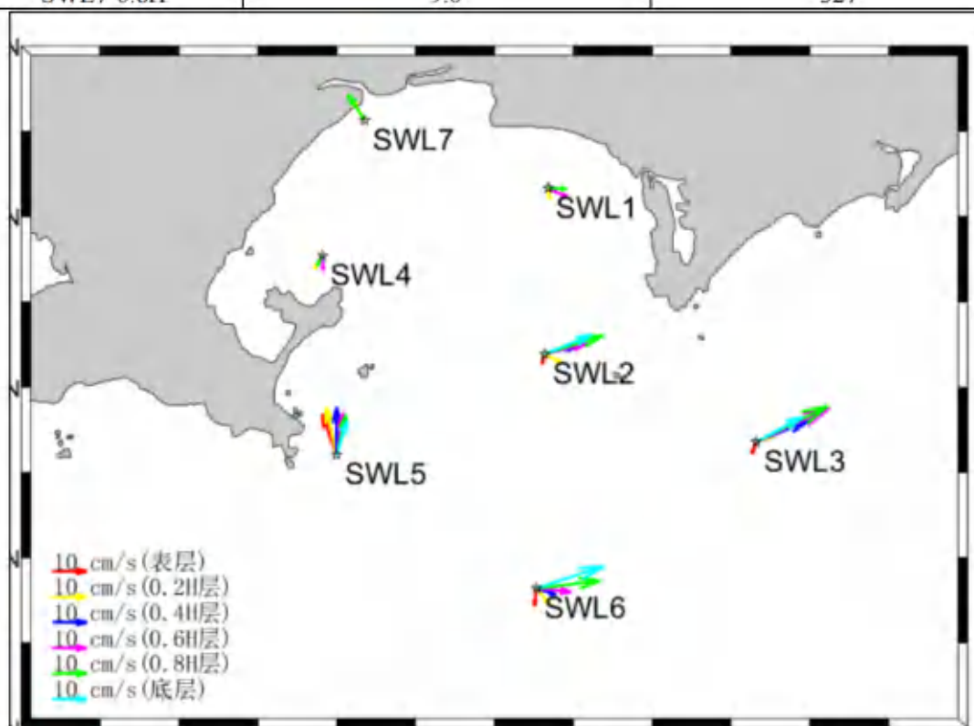
图 5.5.6-1 冬季观测期各站余流图
