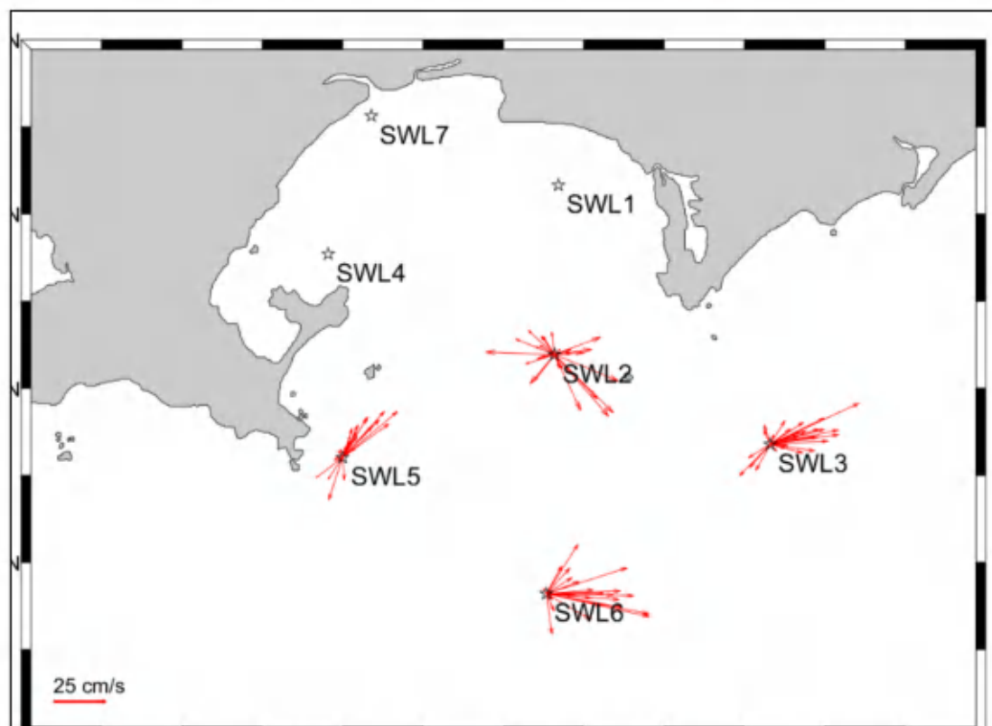
图 5.5.4-9 夏季 0.4H 层海流平面分布矢量图
