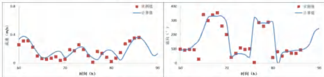
图 6.1.1-5s 夏季 SWL6 站流速、流向验证 (底层)
