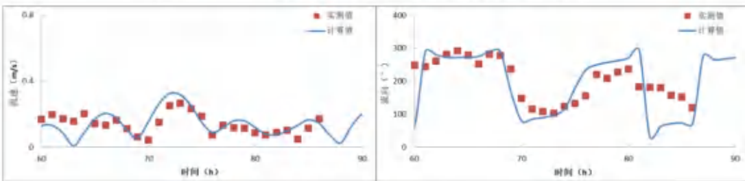
图 6.1.1-7p 冬季 SWL6 站流速、流向验证 (表层)
