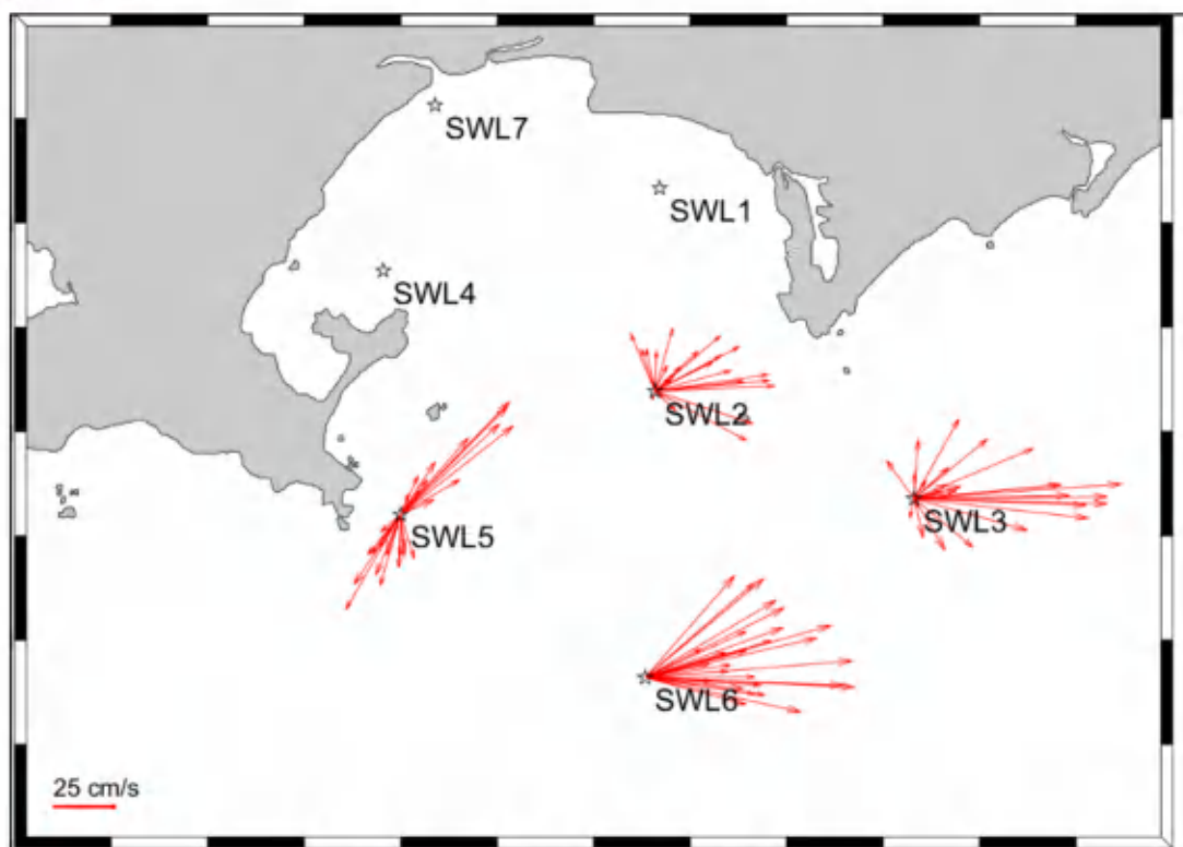
图 5.5.4-7 夏季表层海流平面分布矢量图
