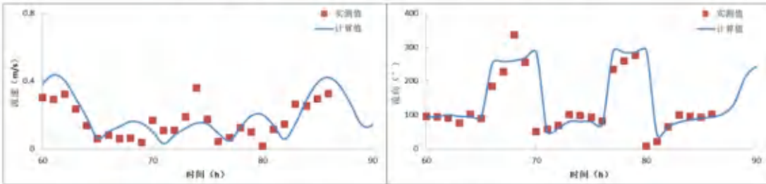
图 6.1.1-5r 夏季 SWL6 站流速、流向验证 (0.6 层)
