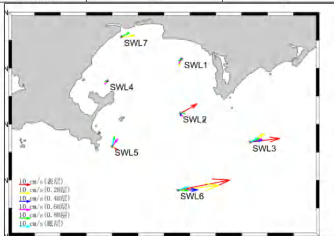
图 5.5.6-2 夏季观测期各站余流图
