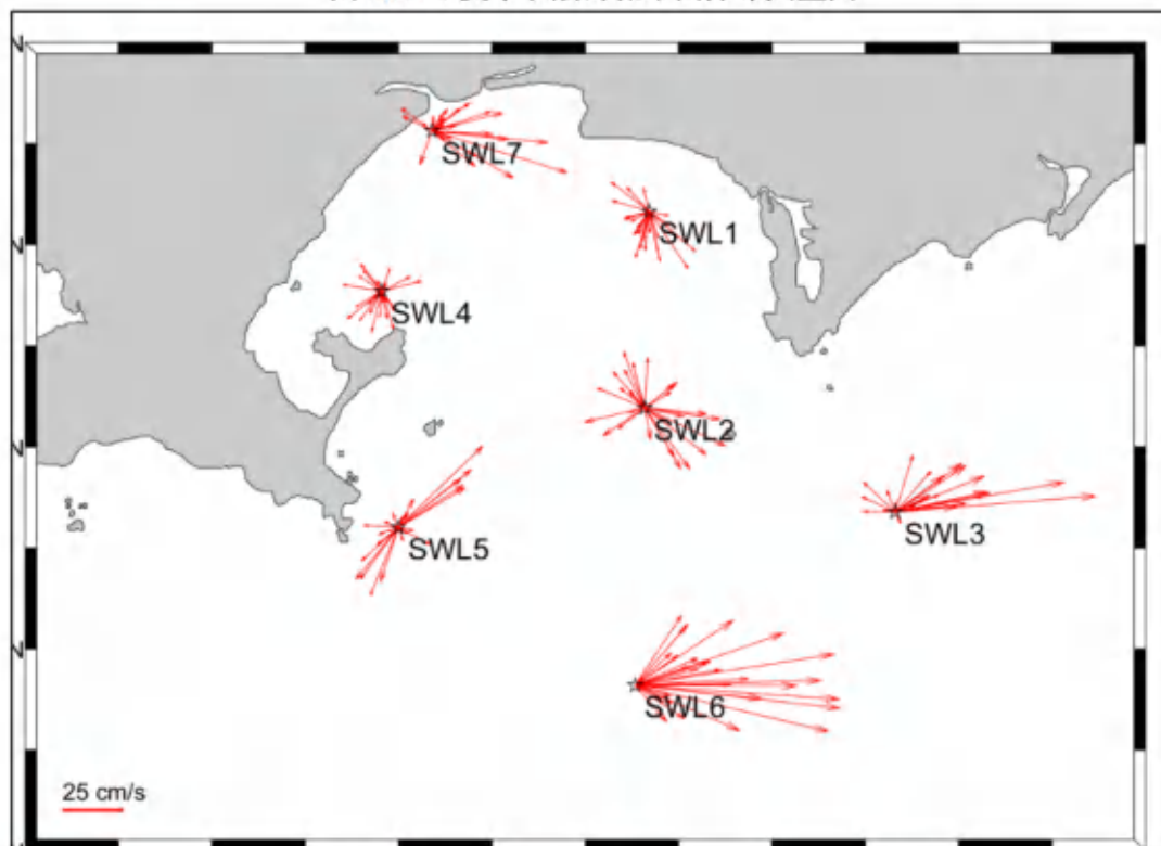
图 5.5.4-8 夏季 0.2H 层海流平面分布矢量图
