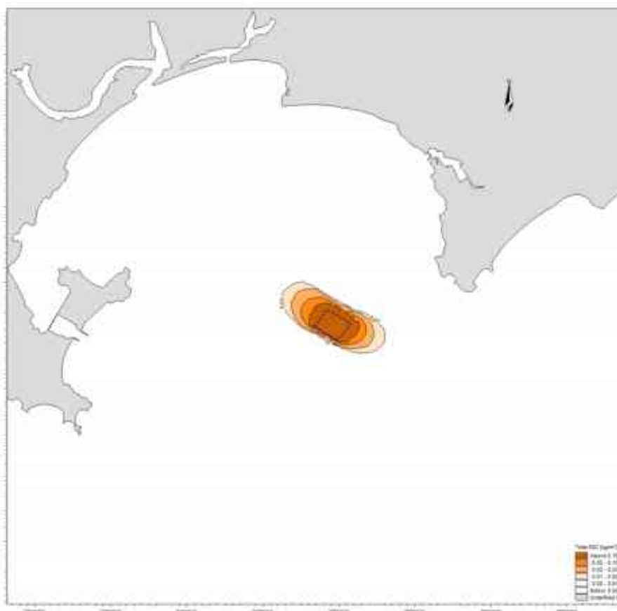
图 6.4.2-3b 夏季海砂分选最大包络线工程产生悬沙增量包络线图（中层）
