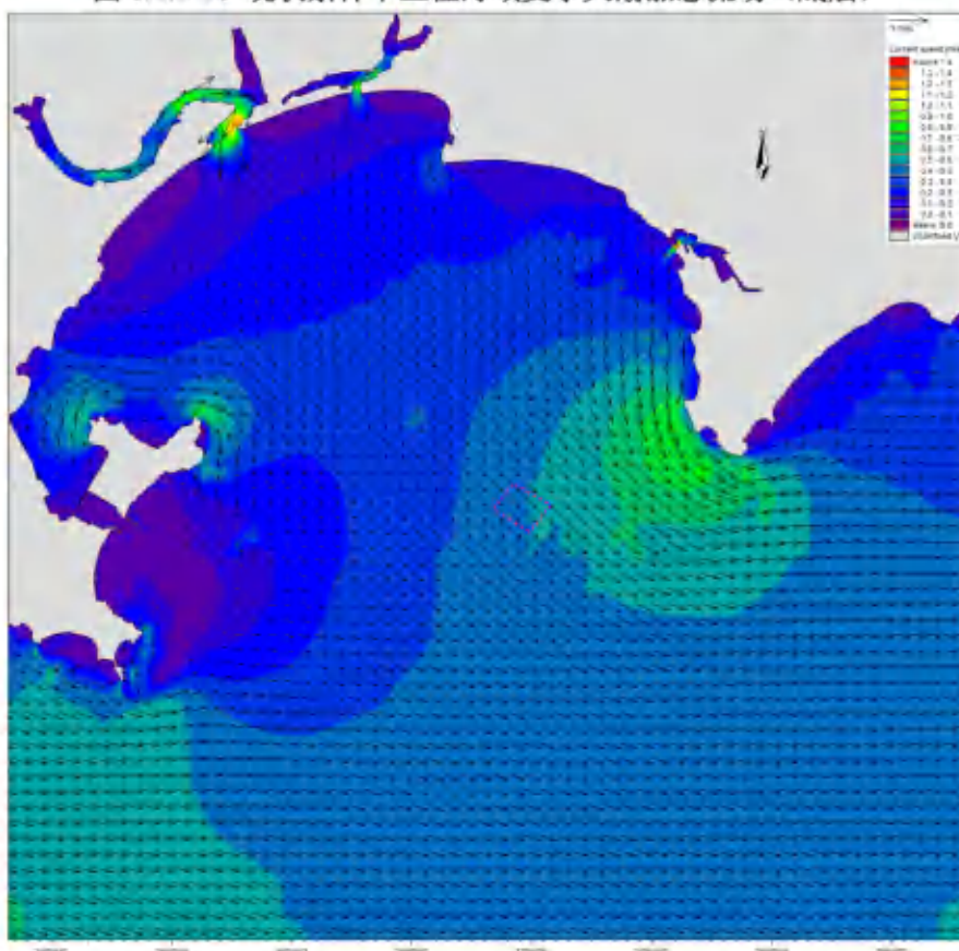
图 6.1.2-1d 现状条件下工程海域夏季大潮落急流场（表层）
