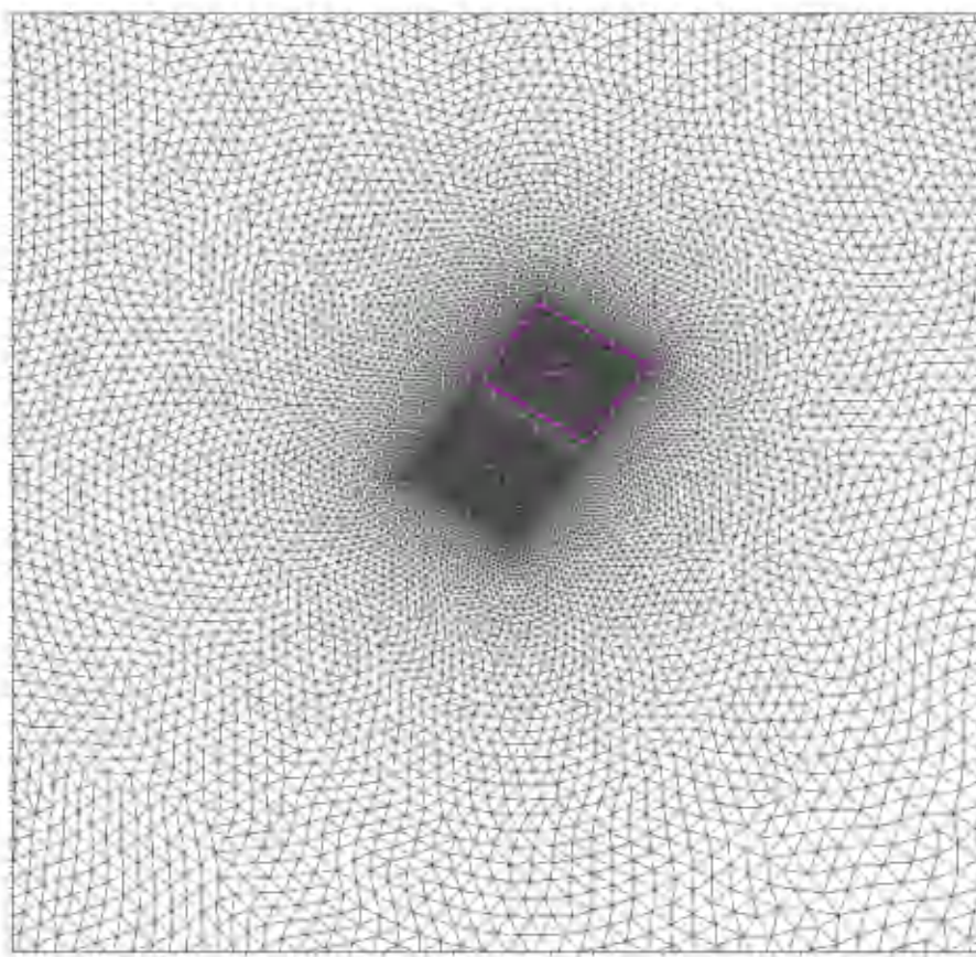
图 6.1.1-2a 工程区网格剖分图 (SW24-12 采砂区)
