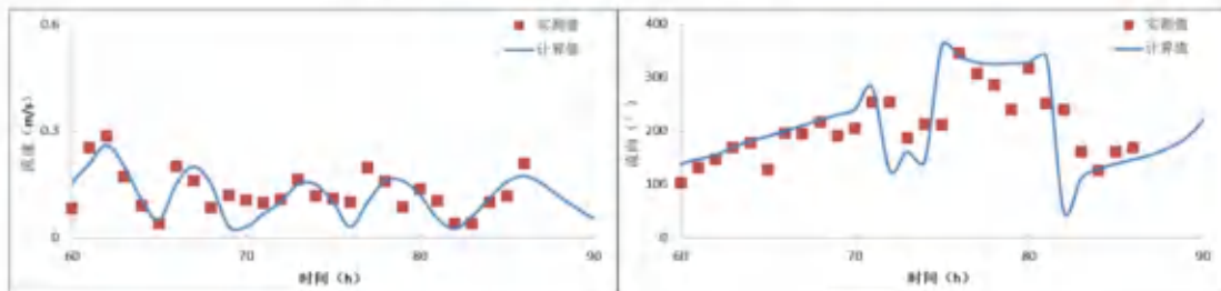
图 6.1.1-5a 夏季 SWL1 站流速、流向验证（表层）
