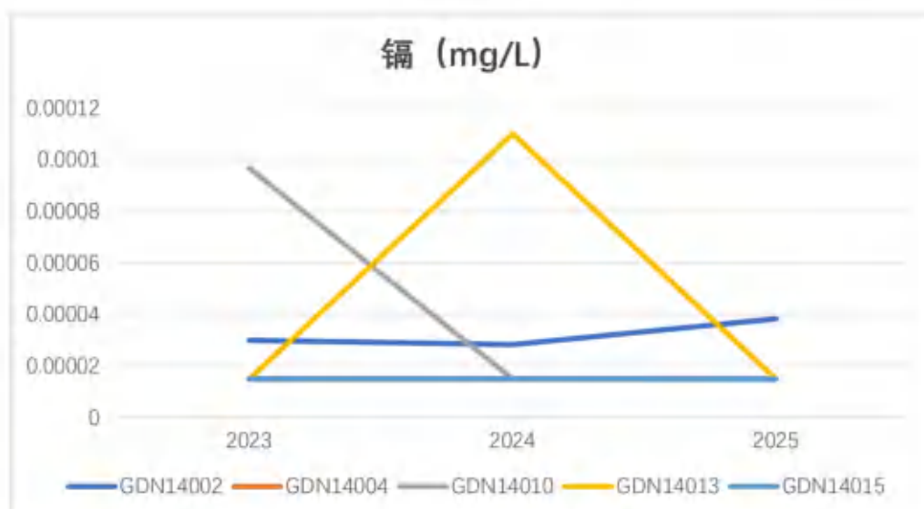
图 5.1.2-11 国控站位 2023 年~2025 年镉含量变化趋势
