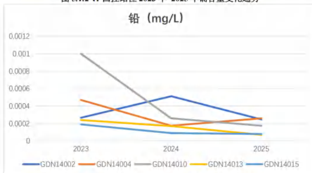
图 5.1.2-12 国控站位 2023 年~2025 年铅含量变化趋势
