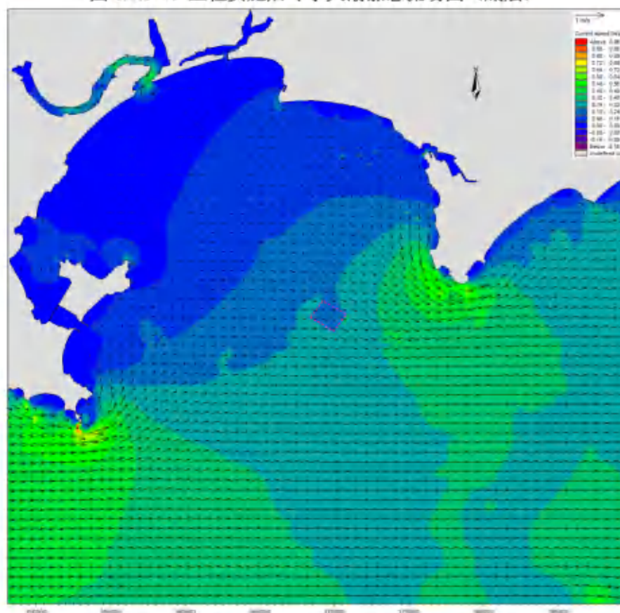
图 6.1.3-4d 工程实施后冬季大潮落急流场图（表层）
