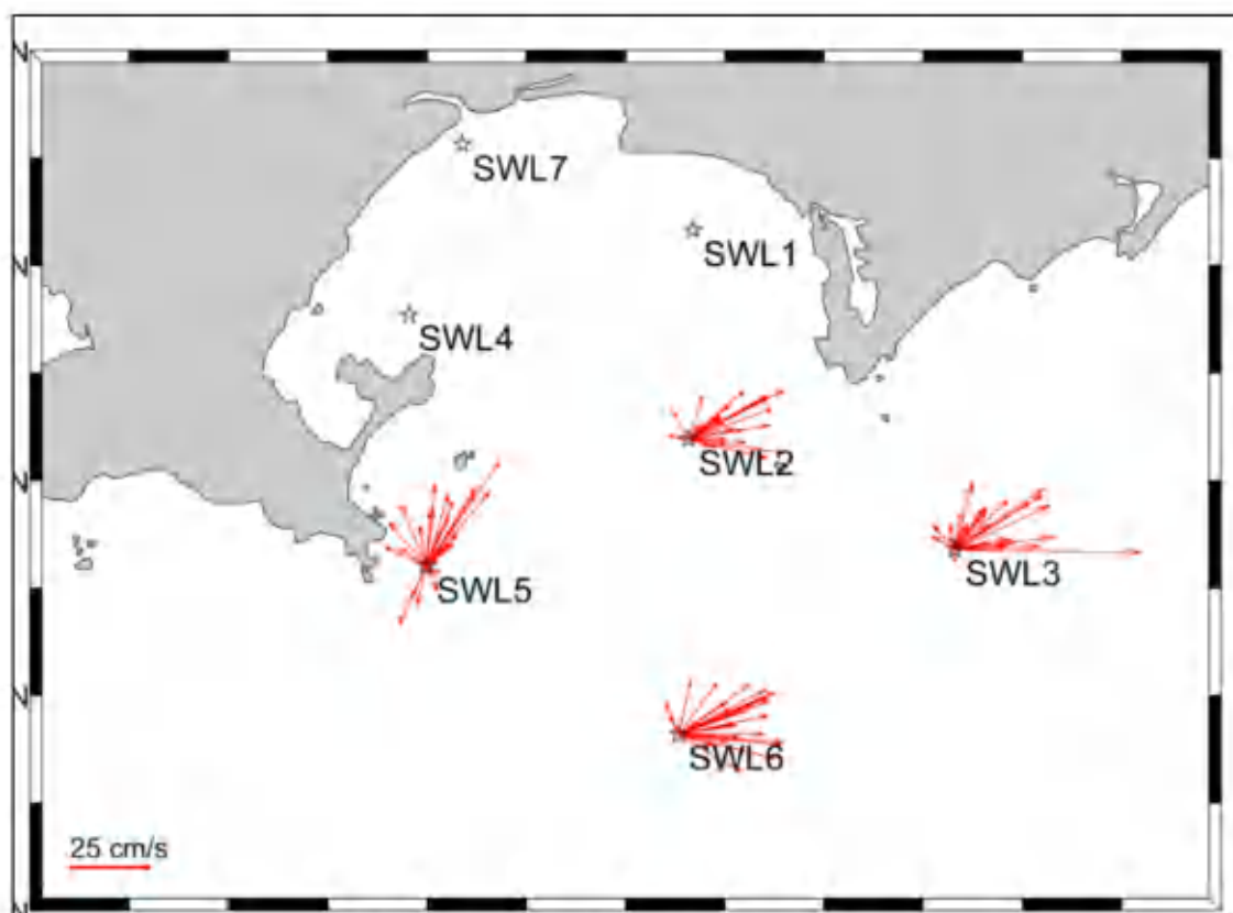
图 5.5.4-6 冬季底层海流平面分布矢量图
