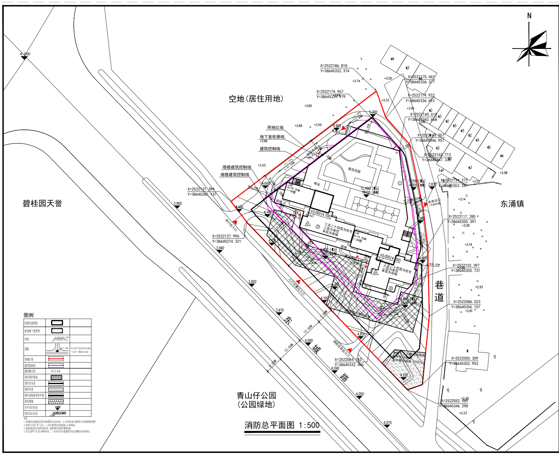
变更前消防总平面图
