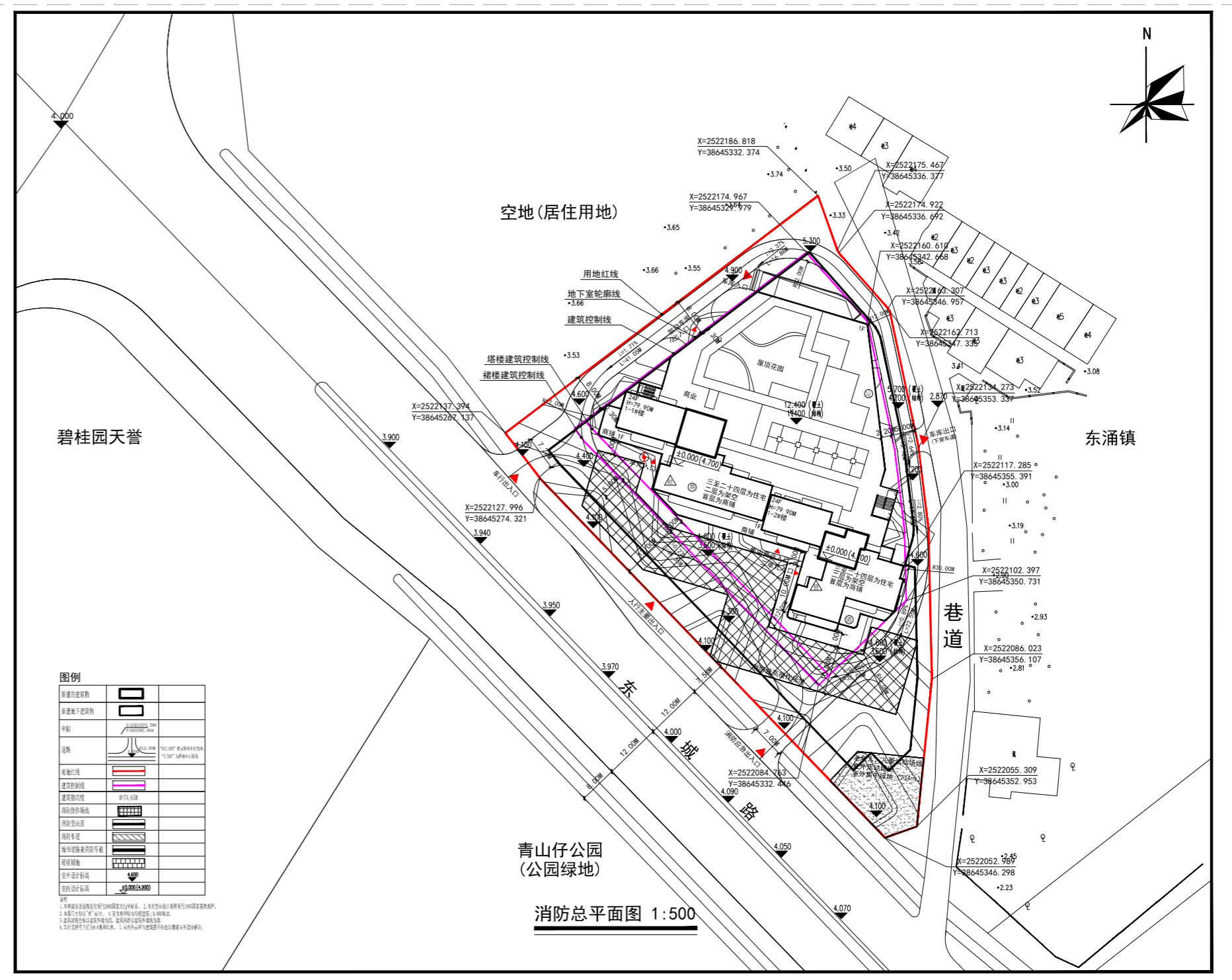
变更后消防总平面图
