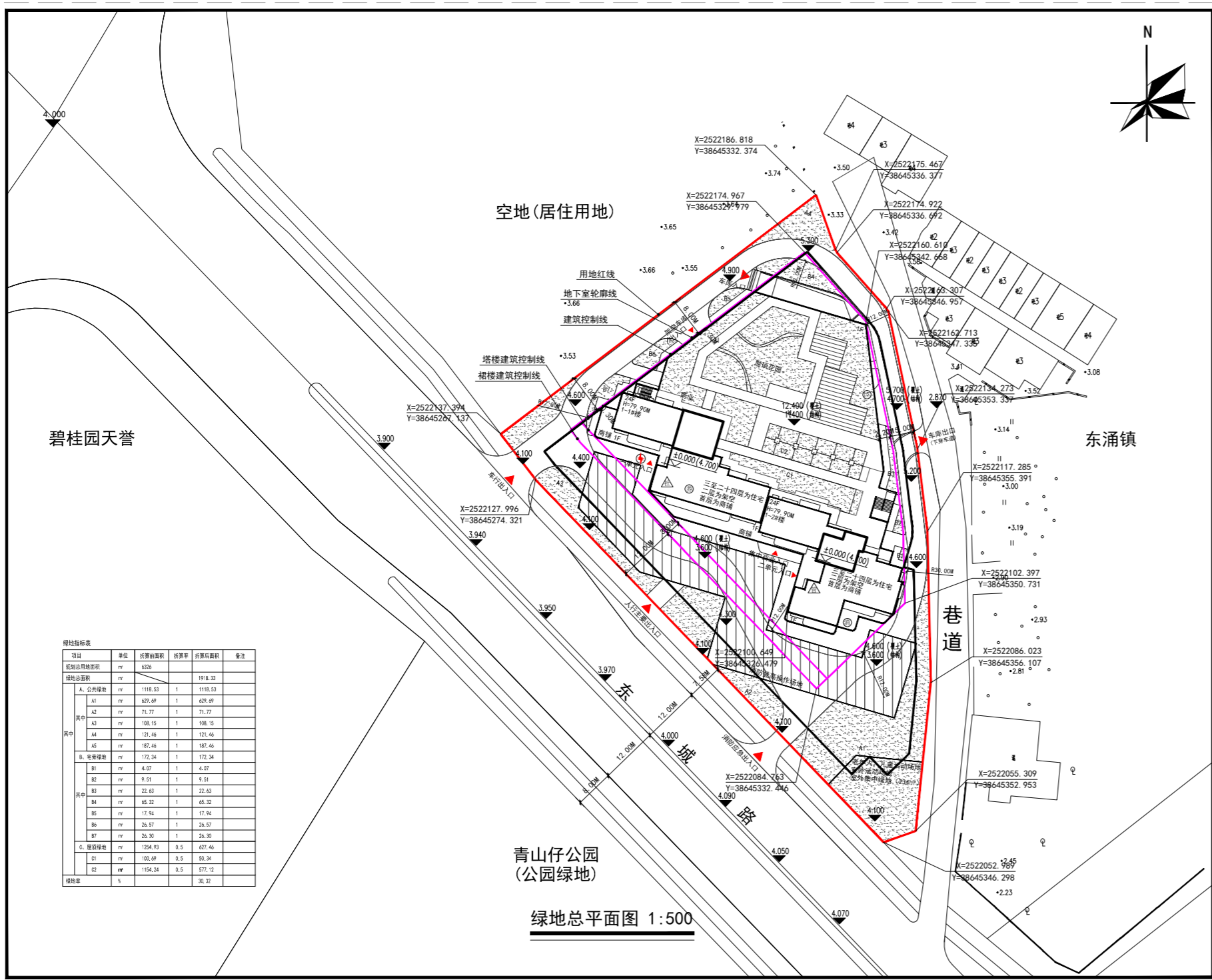
变更前绿地总平面图
