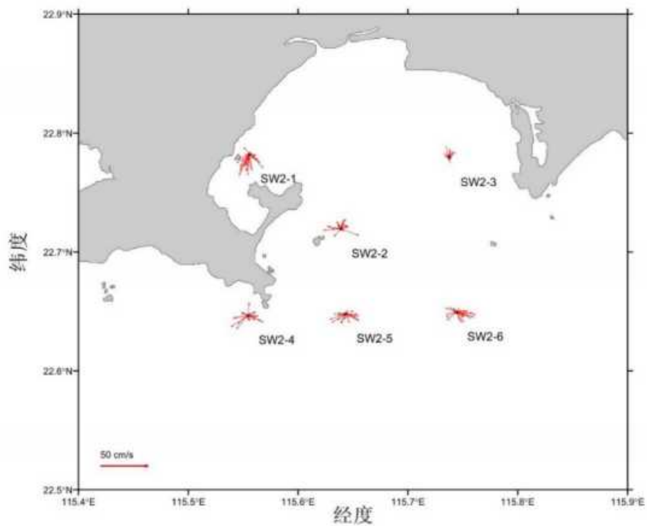
图 4.4.13 垂向平均海流平面分布矢量图
