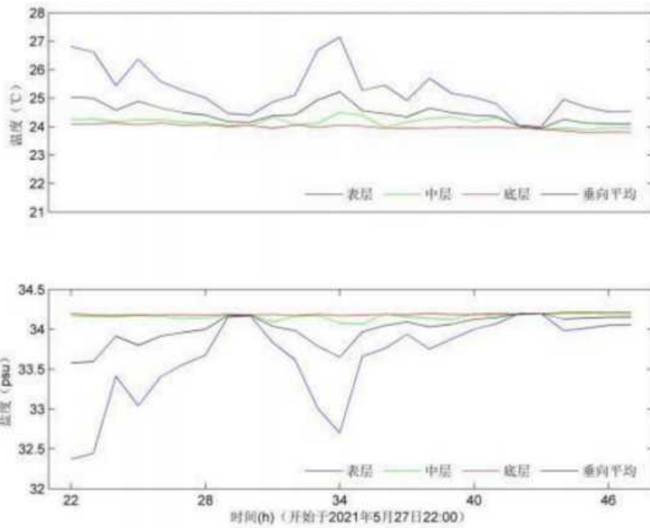
图 4.4.7-4SW2-4 站水温与盐度过程曲线
