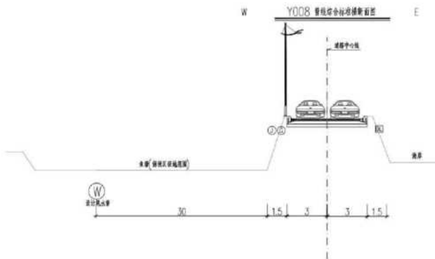
图 3.2.4-4 Y008 段管道横断面图
