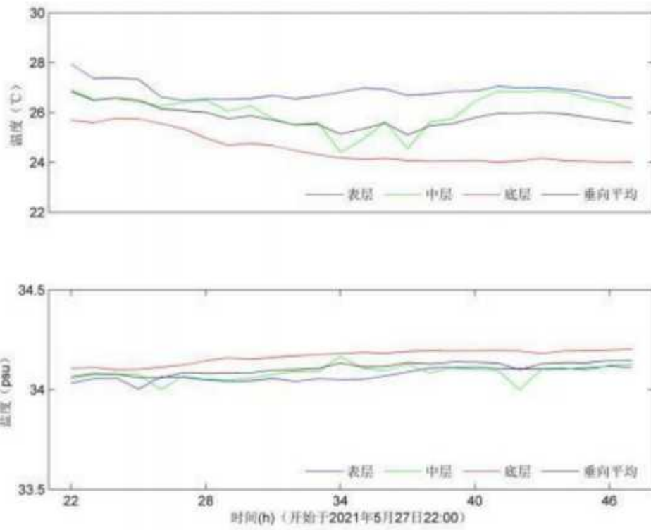
图 4.4.7-2SW2-2 站水温与盐度过程曲线
