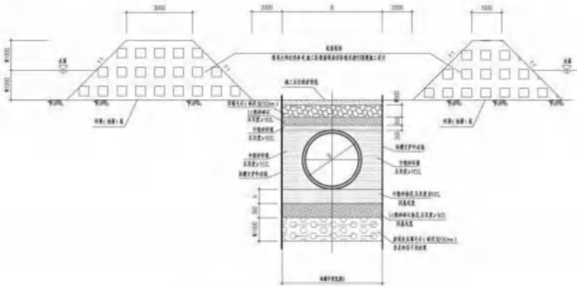
图 3.4.2-2 过河涌（池）段围堰横断面图
