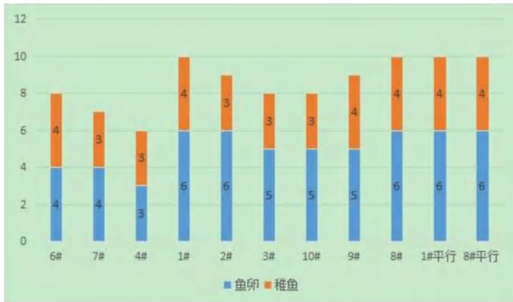
图 4.6.7-5 各站位鱼卵仔鱼发育阶段占比
