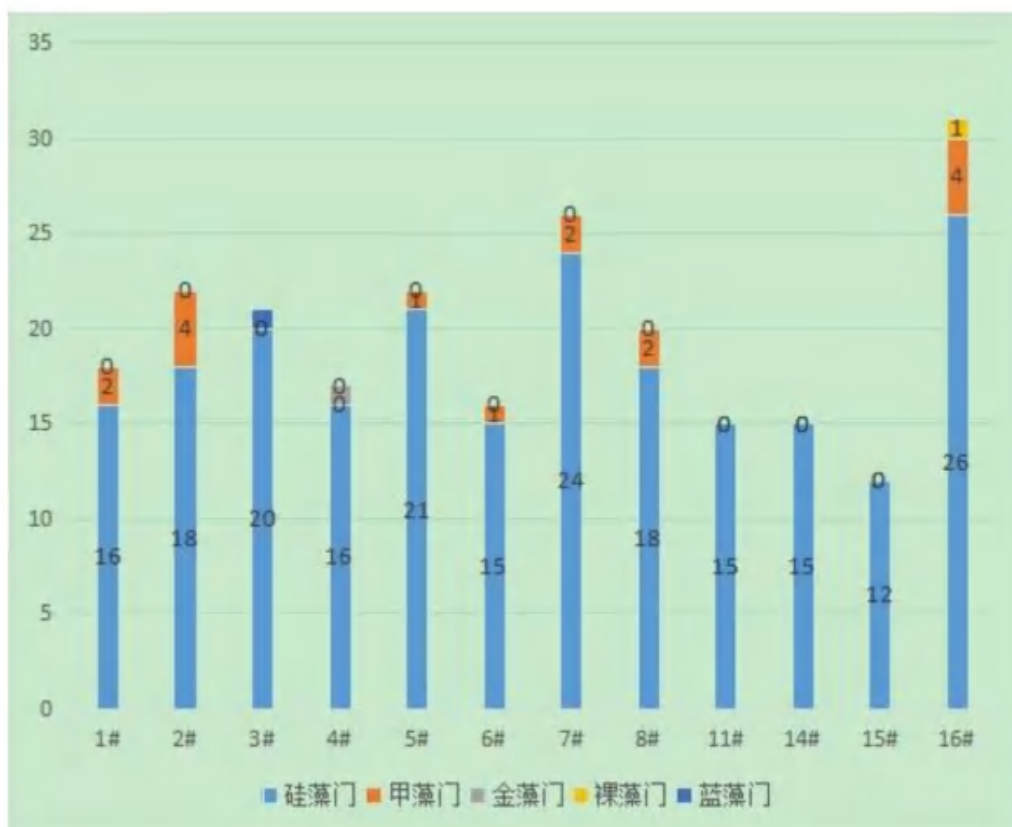
图 4.6.7-7 各站位浮游植物种类数占比
