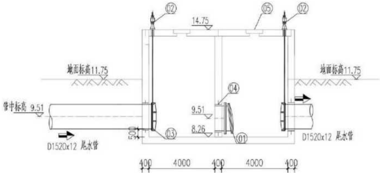
图 3.2.4-10 高位井设计图
