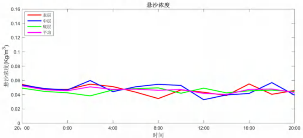
图 4.4.6-7SW2-1 站悬沙浓度时间过程曲线图
