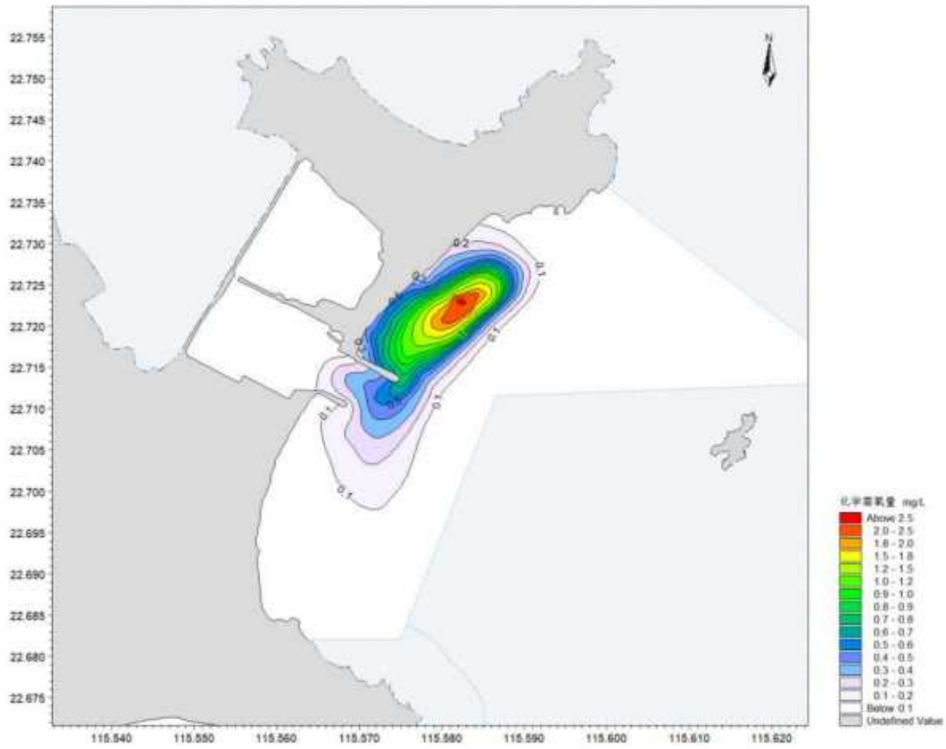
图 5.3.4-1 春季近期正常排放工况下 COD Mn 预测浓度增值包络线图
