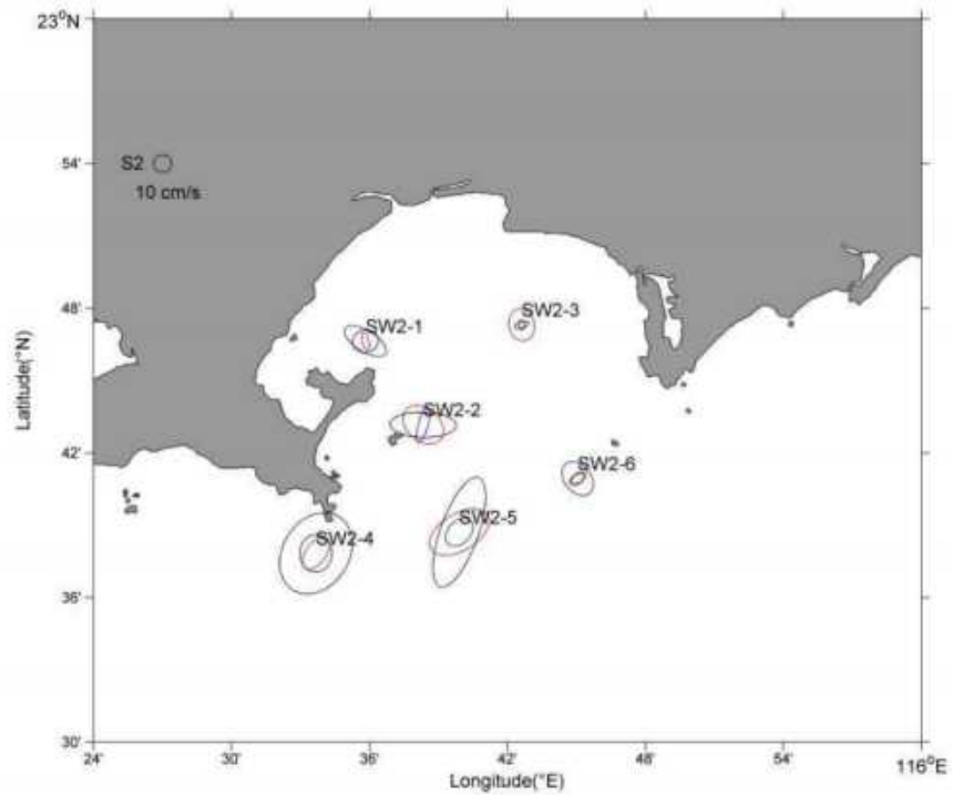
图 4.4.5-2 各测站 S2 分潮潮流椭圆图
