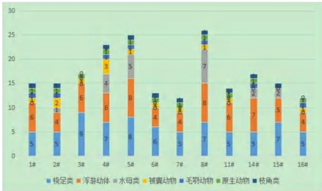
图 4.6.7-8 各站位浮游动物种类组成
