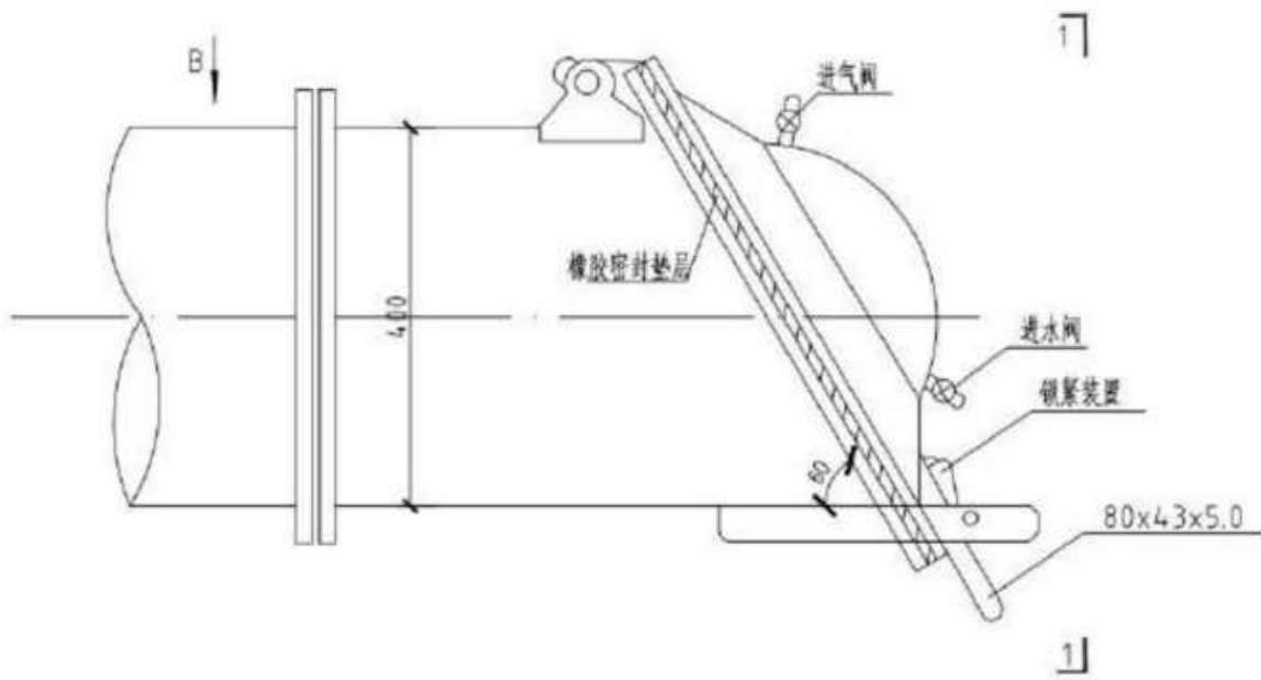
图 3.2.4-15 冲洗阀门设计大样图
