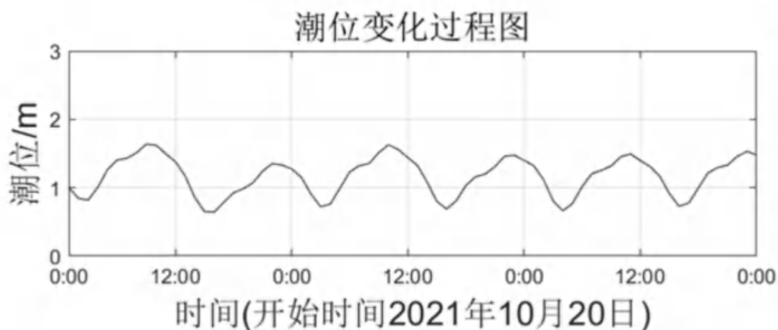
图 4.4.3-4 SWC3 站潮位过程曲线
