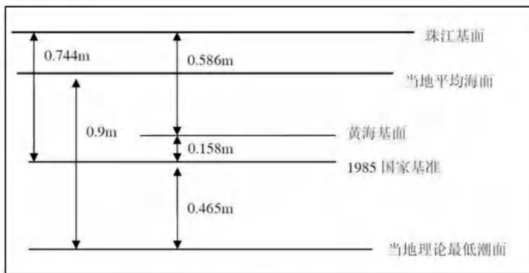
图 4.4.3-1 汕尾站基面关系图（单位：m）
