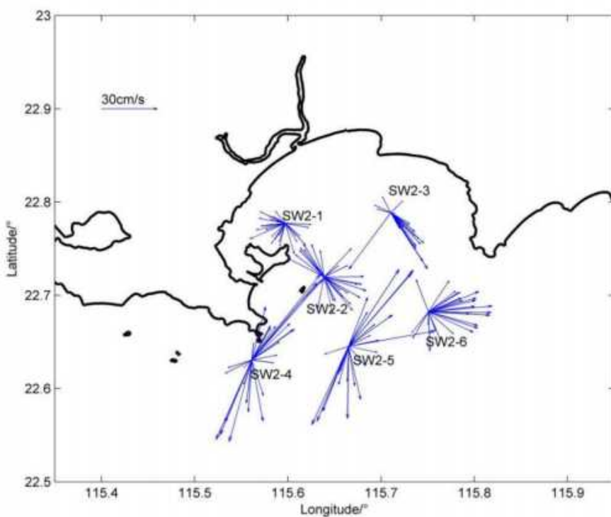
图 4.4.4-2 各站中层海流平面分布矢量图
