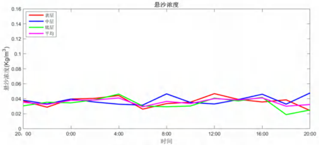
图 4.4.6-12SW2-6 站悬沙浓度时间过程曲线图
