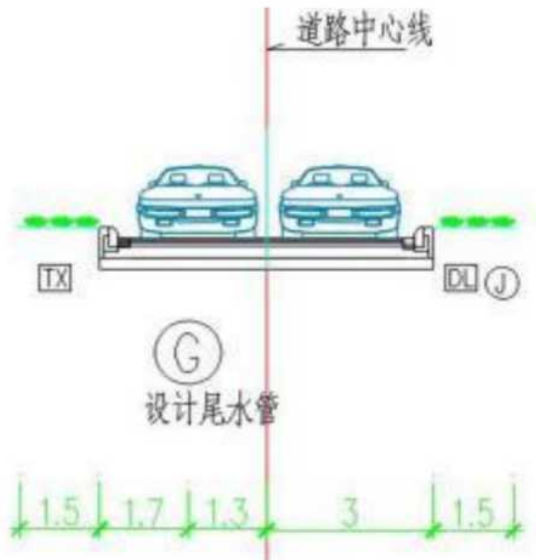
图 3.2.4-7 新湖路管线综合标准横断面图
