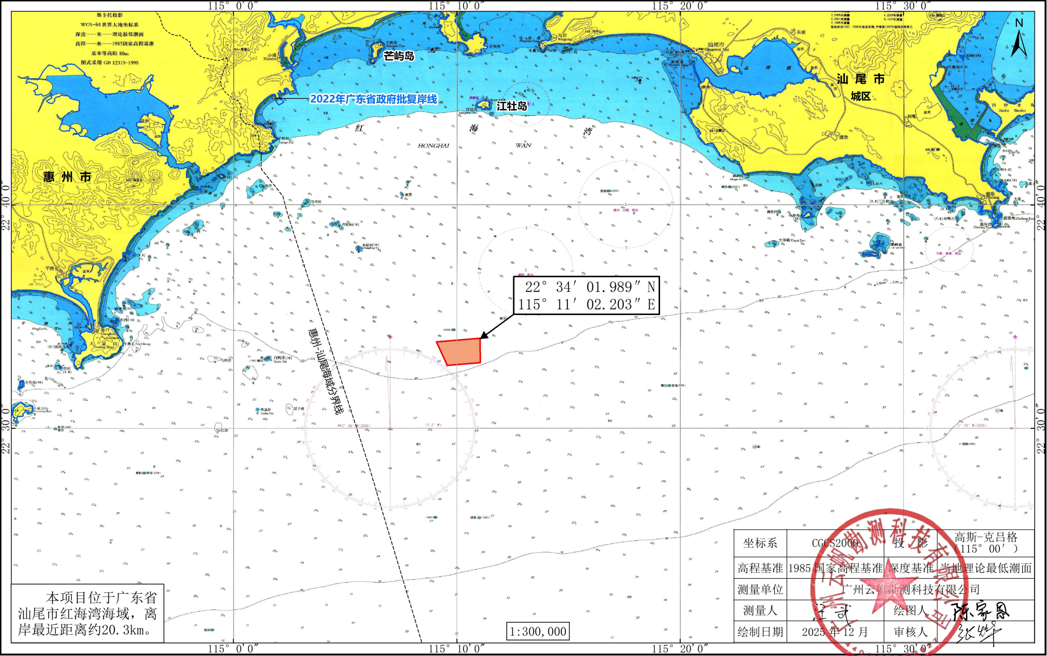
汕尾市红海湾现代化海洋牧场创新园-红海湾中远期海域（五区A区）项目宗海位置图
