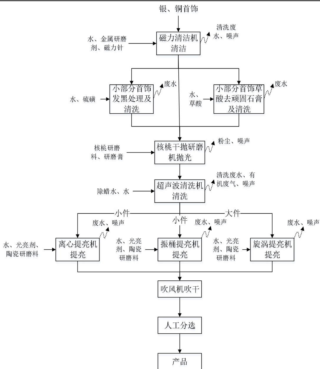
图 3 项目加工工艺流程图
