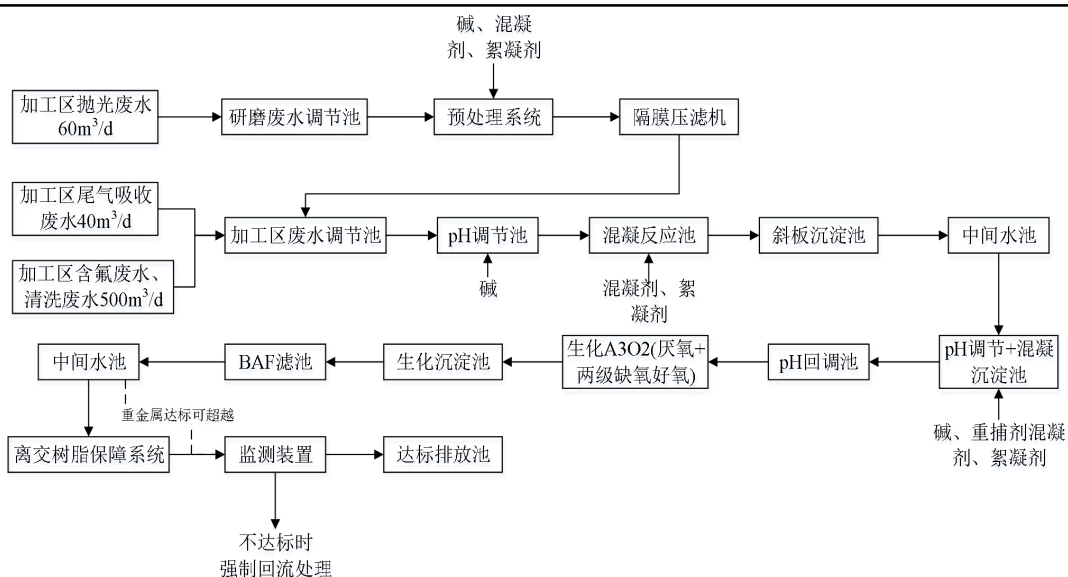
图 5 海丰首饰产业环保集聚区污水处理厂加工区废水处理工艺图
