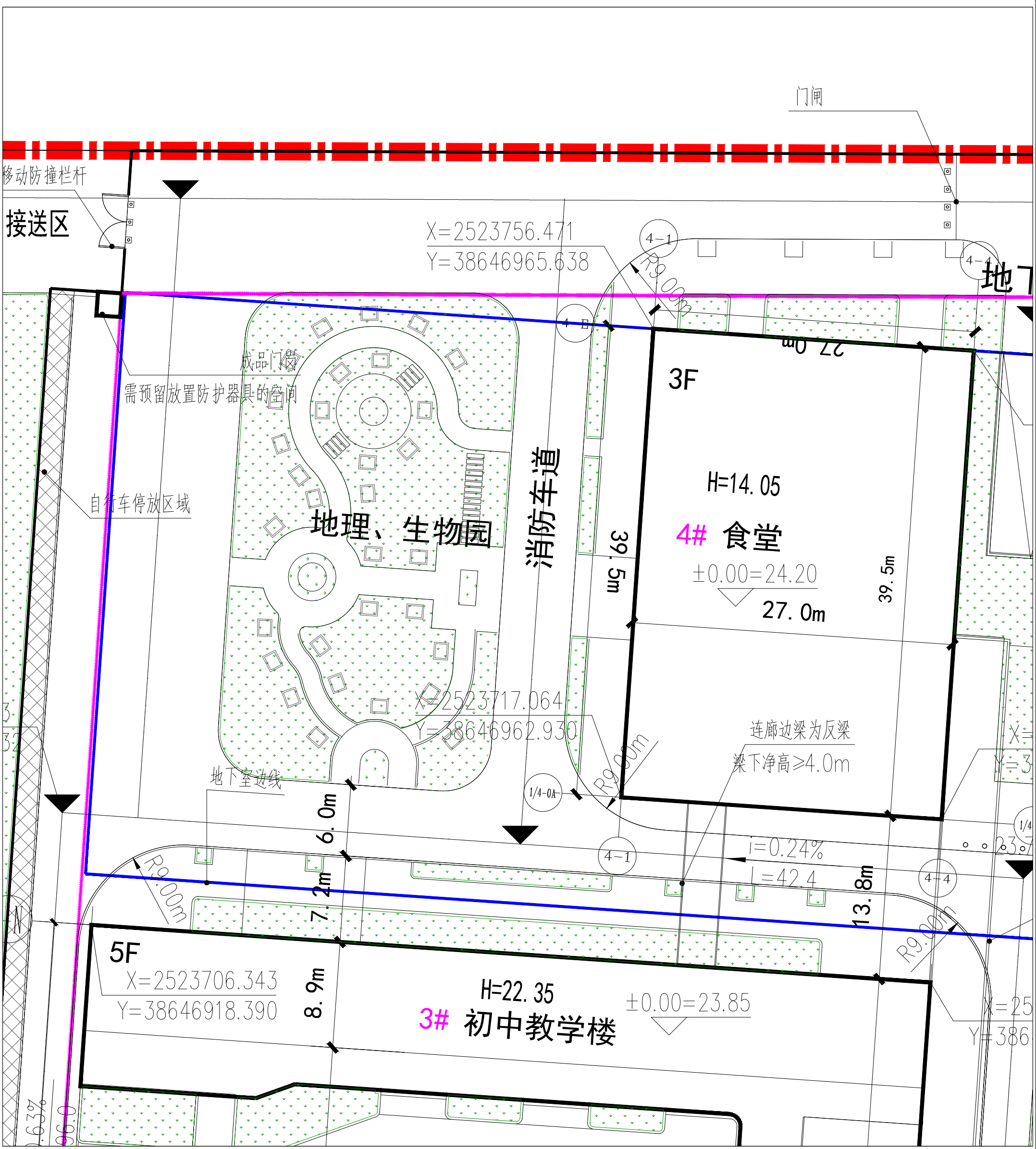
变更后4#食堂总平面图
