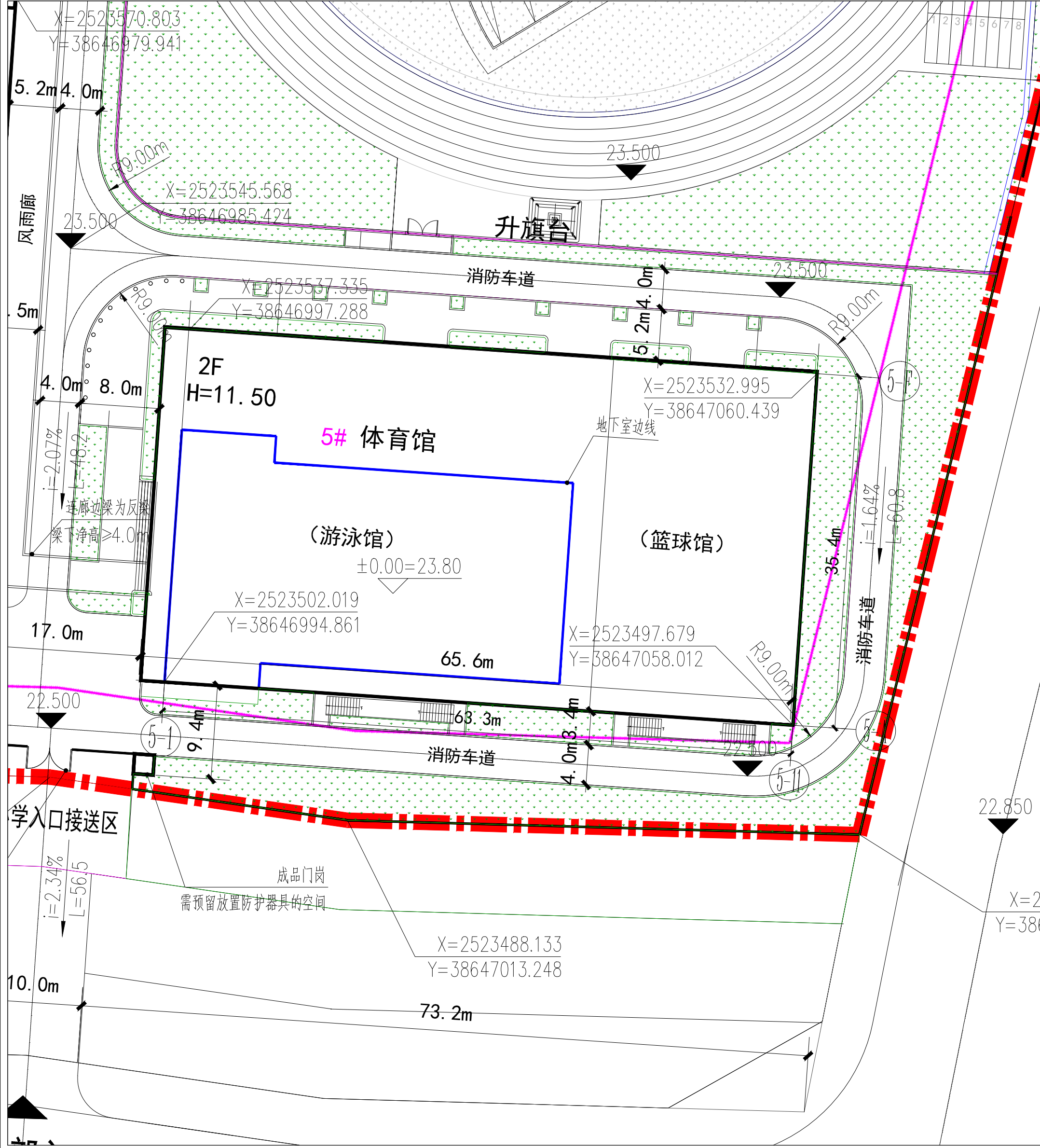
变更前5#体育馆总平面图
