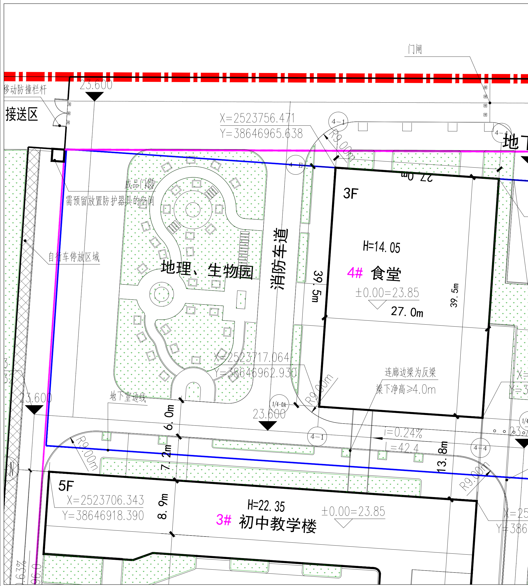
变更前4#食堂总平面图
