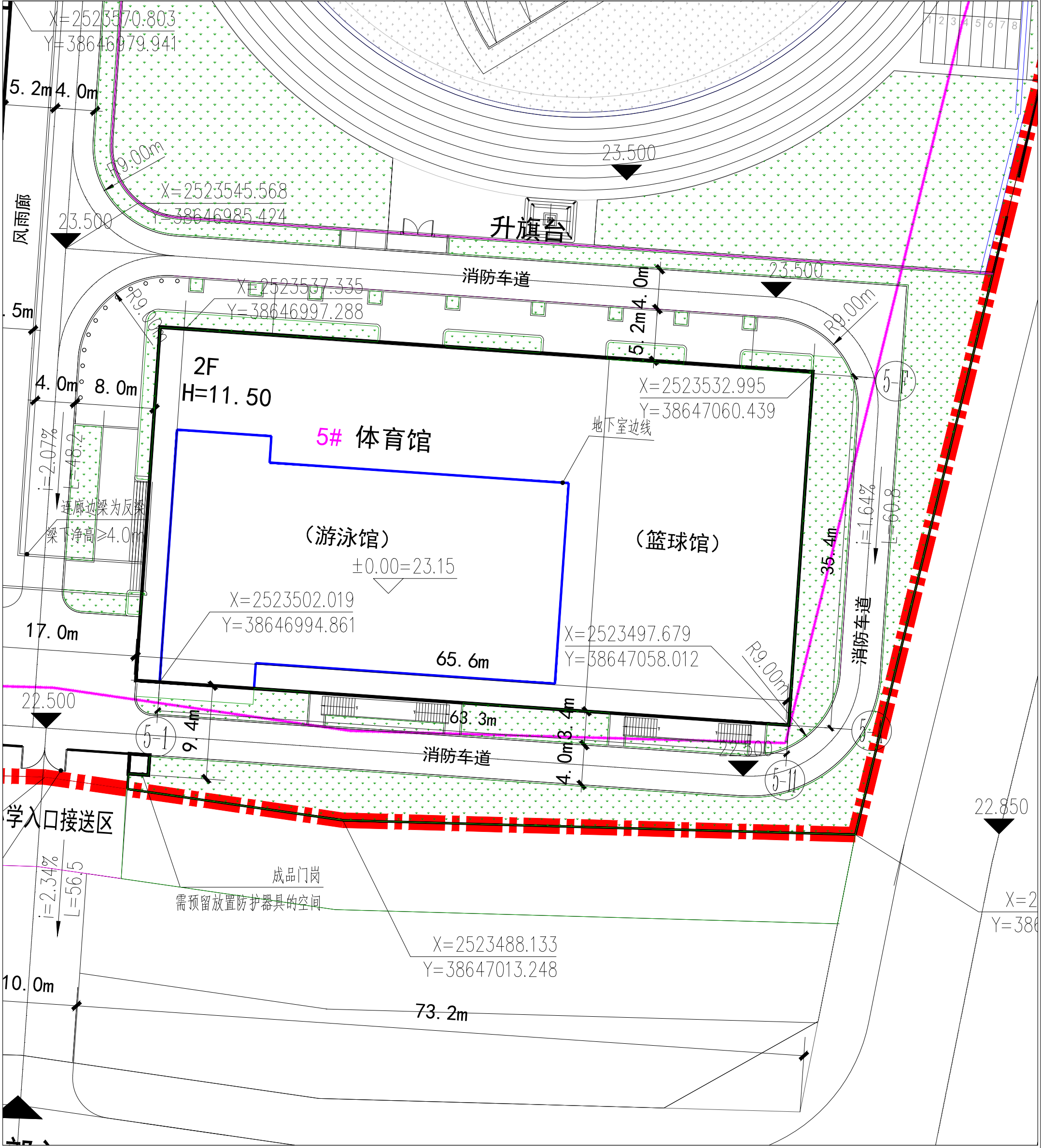
变更后5#体育馆总平面图
