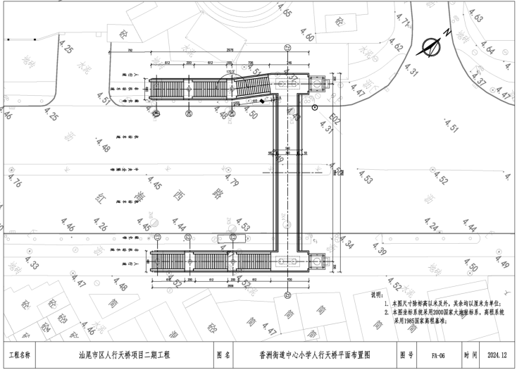
香洲街道中心小学人行天桥 变更后总平面规划图、天桥平面图
