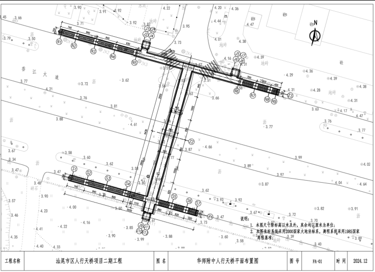
华师附中人行天桥 变更后总平面规划图、天桥平面图
