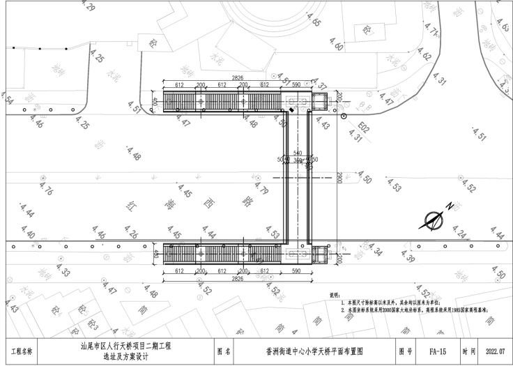
香洲街道中心小学人行天桥 变更前总平面规划图、天桥平面图
