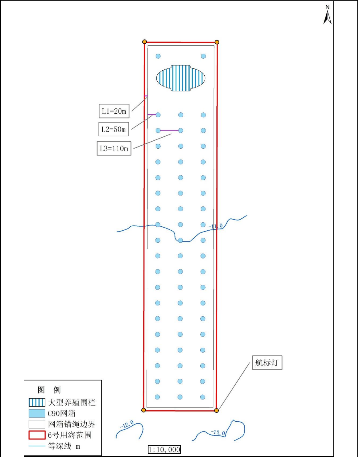
图 1.3.1-1 养殖区平面布置示意图
