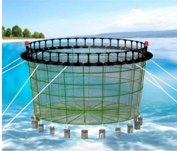
图 1.3.2-2 重力式网箱结构示意图
