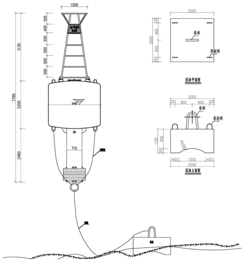
图 1.3.3-1 浮标配置标准图
