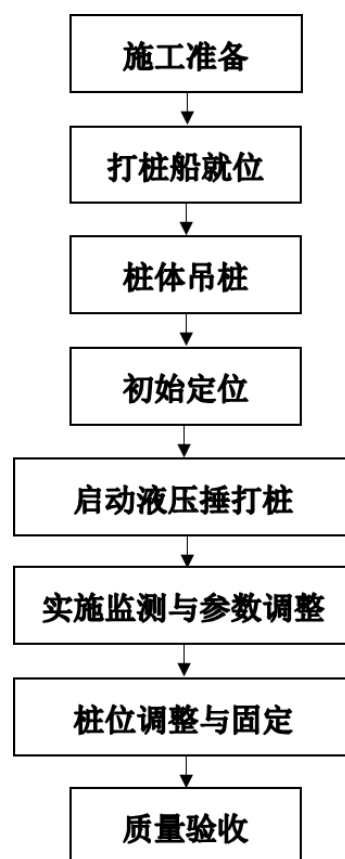
图 1.4.2-1 液压施工工艺流程图
