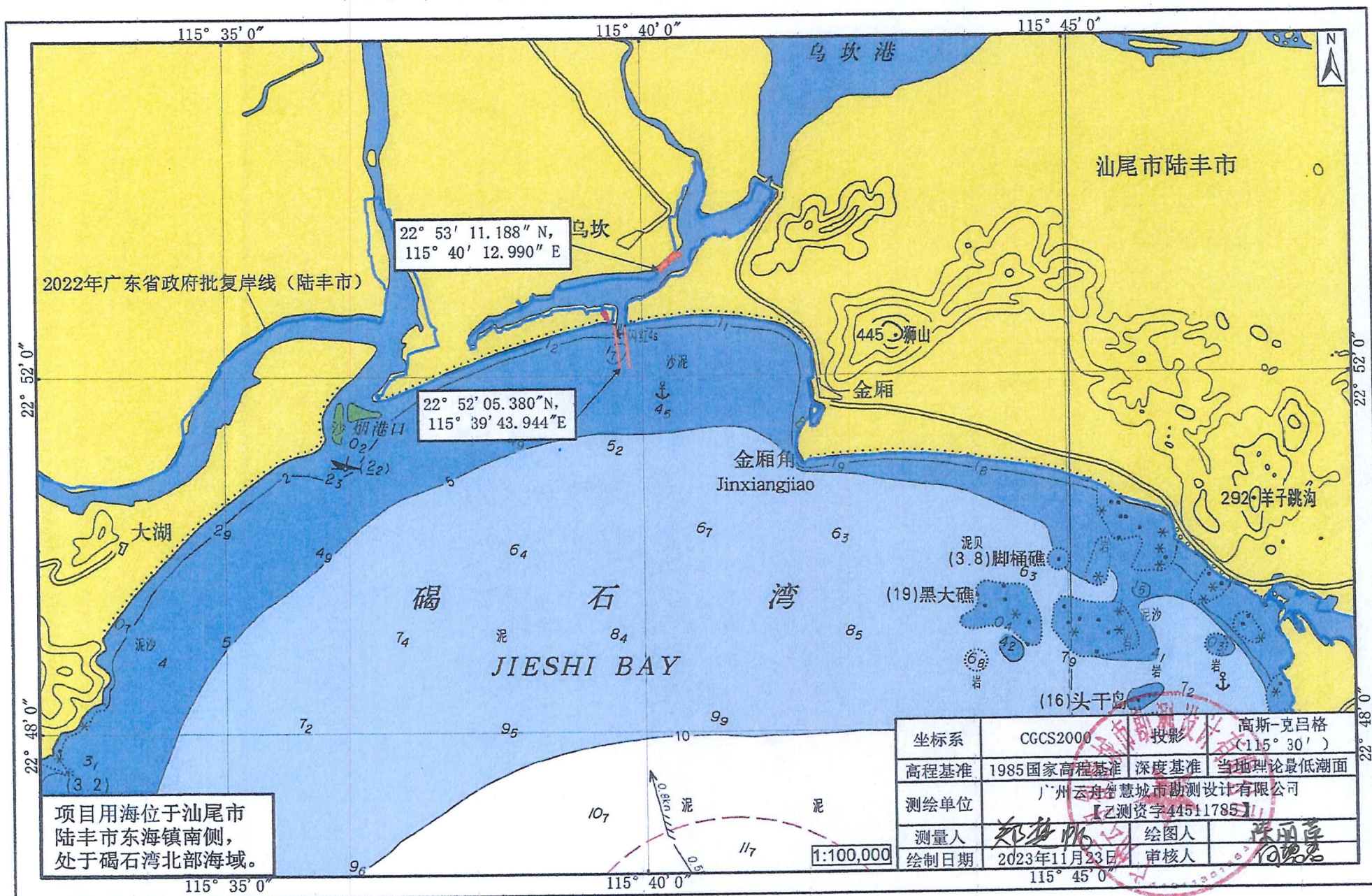
陆丰市东海镇乌坎渔港建设工程项目宗海位置图
