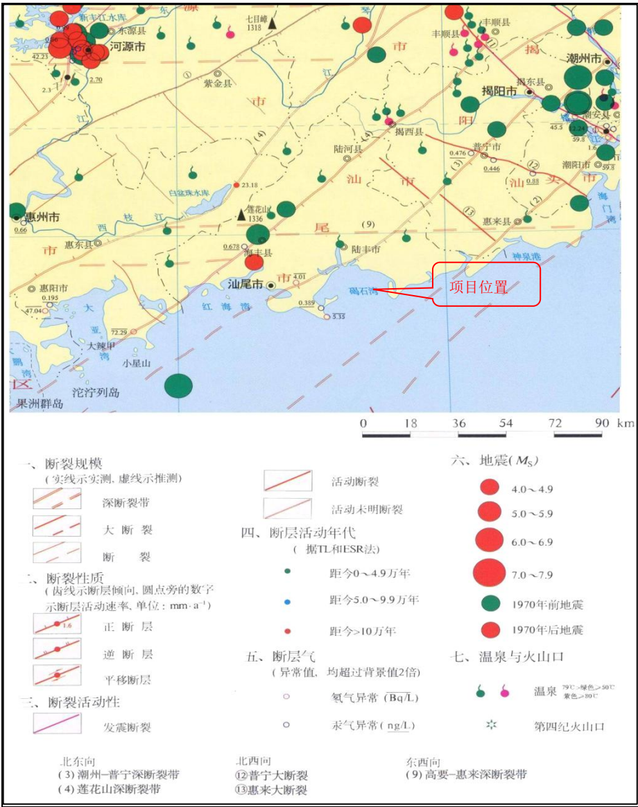
图 2.2.4-1 项目附近断裂分布图 (广东省地震局, 2000)
