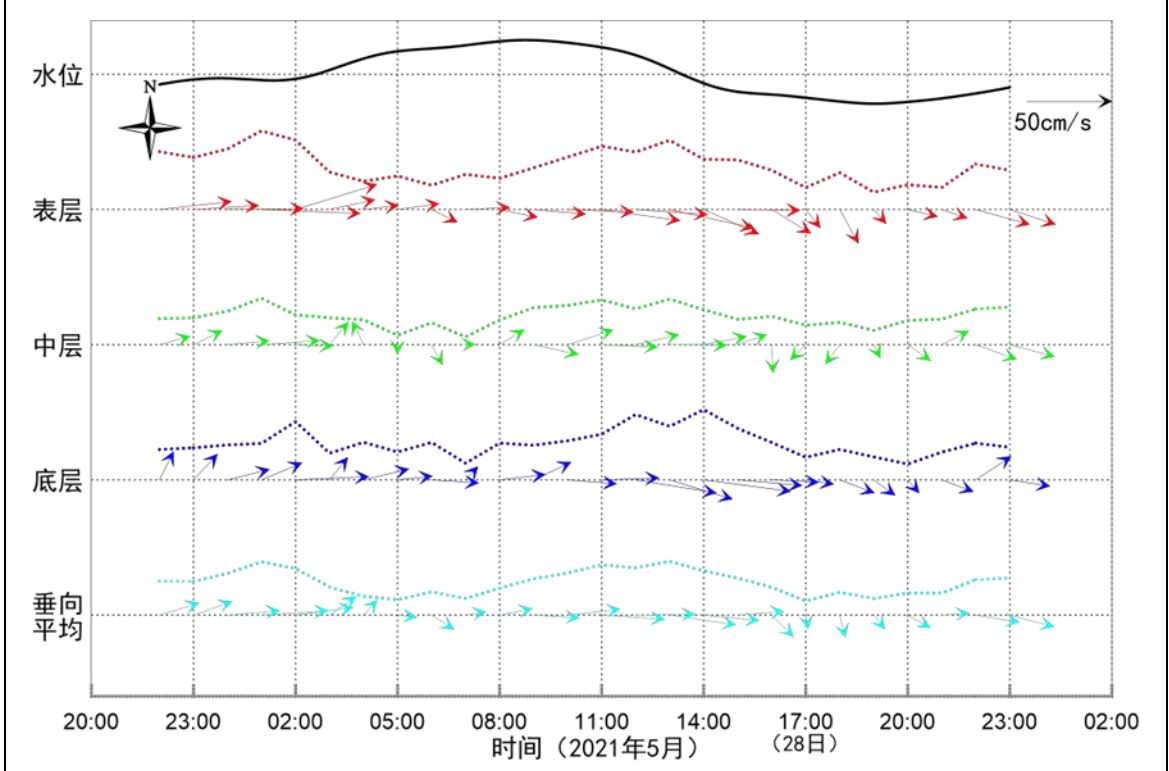
图 2.2.2-10 海流矢量时间变化序列图 (SW2-6 站)
