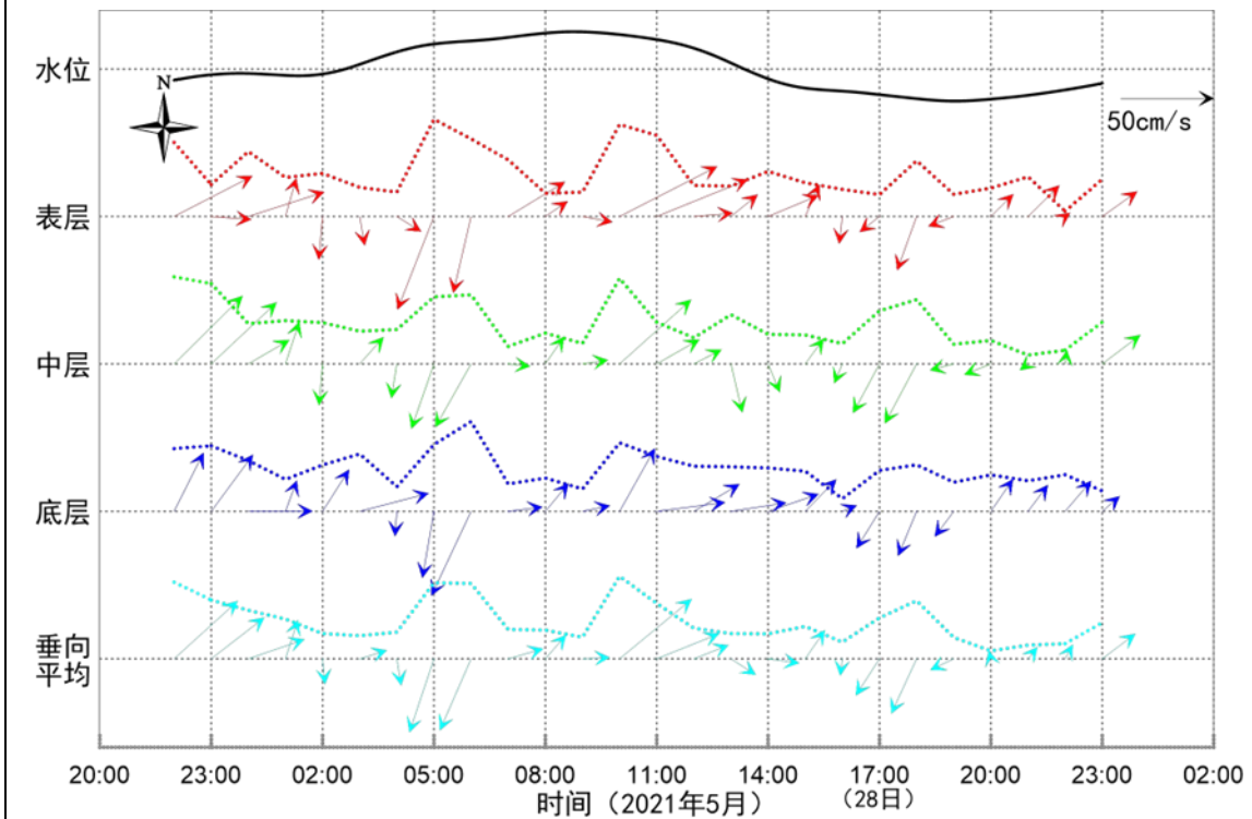
图 2.2.2-8 海流矢量时间变化序列图 (SW2-4 站)
