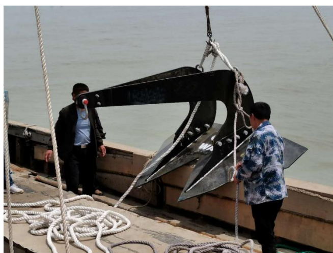
图 1.3.2-3 重力式网箱双齿梨锚
