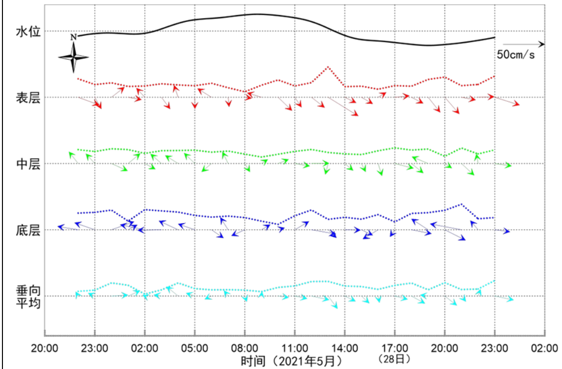
图 2.2.2-6 海流矢量时间变化序列图 (SW2-2 站)
