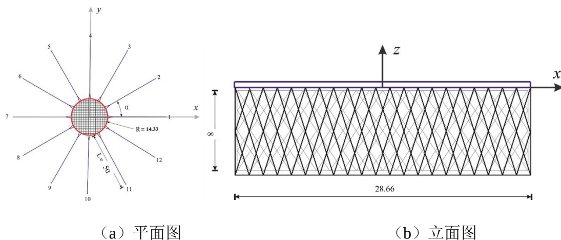
图 1.3.2-1 网箱及其系泊系统布置示意图（单位：米）
