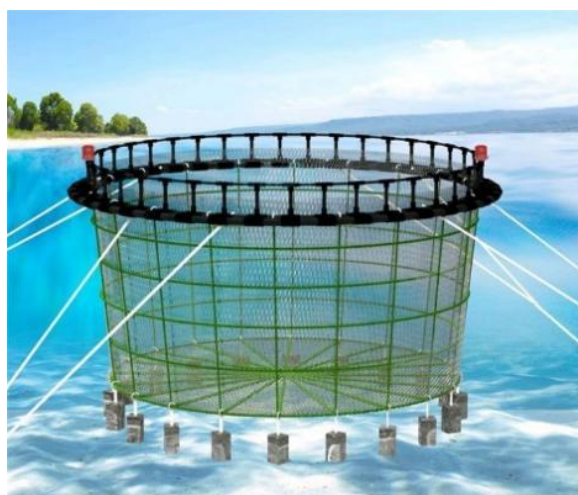
图 1.3.2-2 重力式网箱示意图
