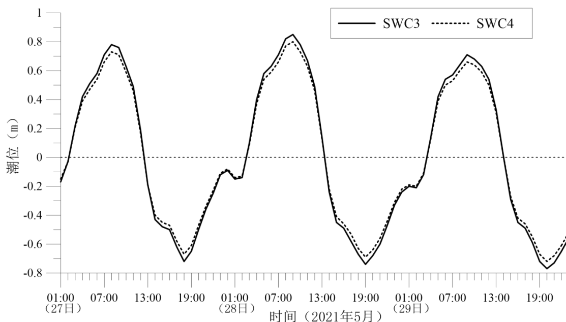
图 2.2.2-4 2021 年 5 月 27~29 日调查站位实测潮位变化
