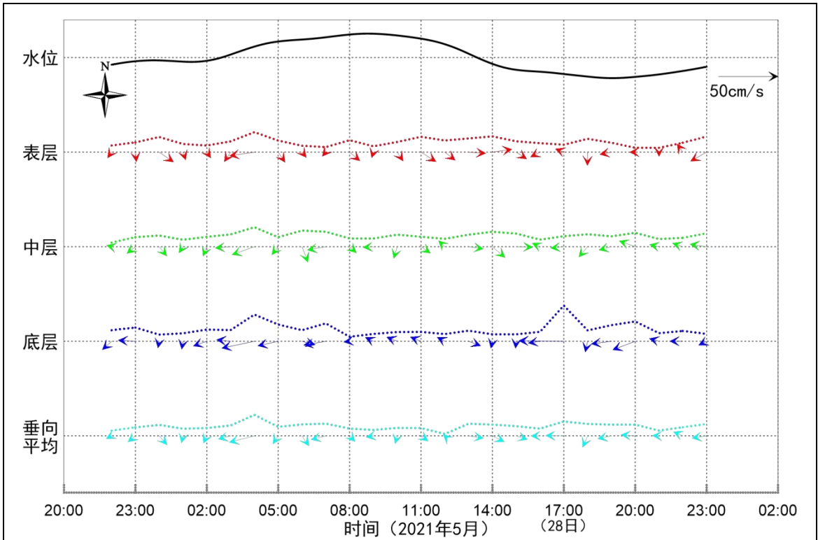
图 2.2.2-5 海流矢量时间变化序列图 (SW2-1 站)
