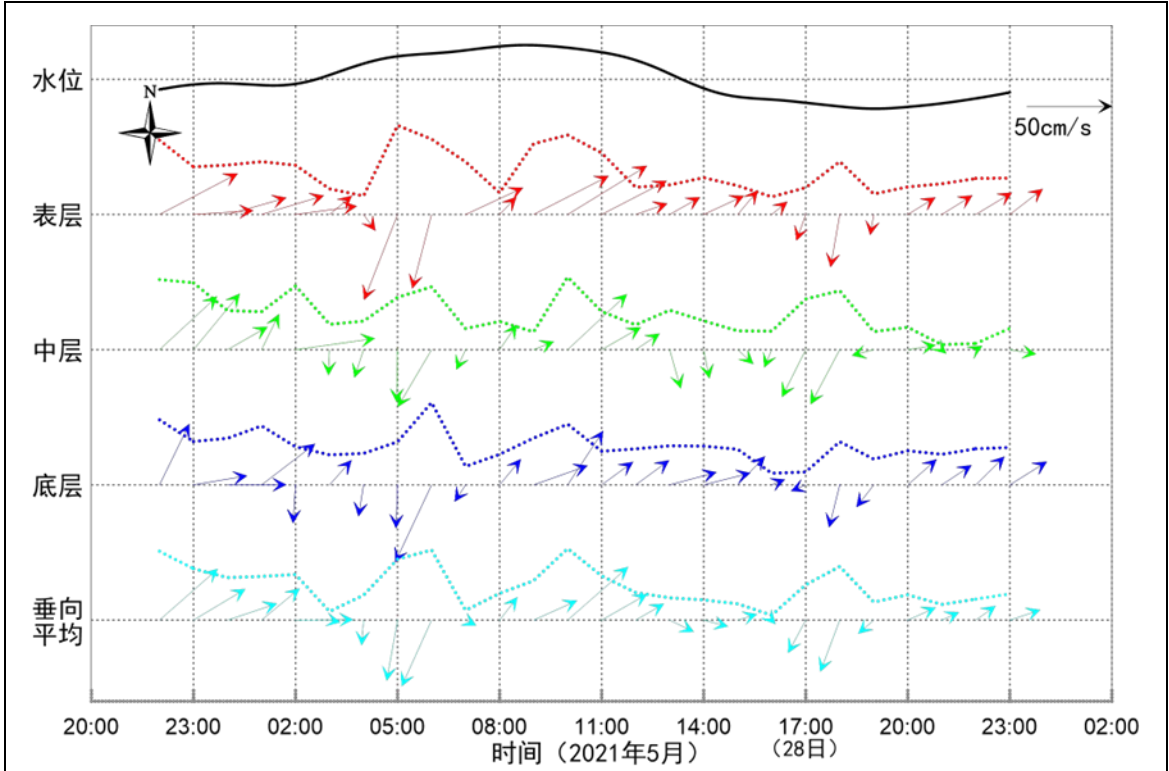
图 2.2.2-9 海流矢量时间变化序列图 (SW2-5 站)
