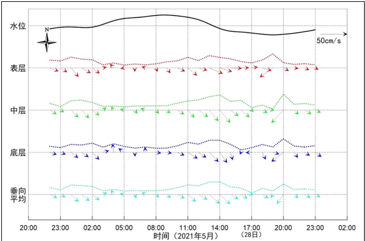
图 2.2.2-7 海流矢量时间变化序列图 (SW2-3 站)
