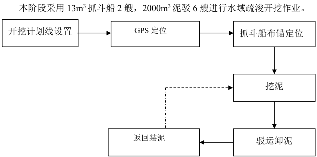
图 2.3-3 抓斗船挖泥施工流程图
