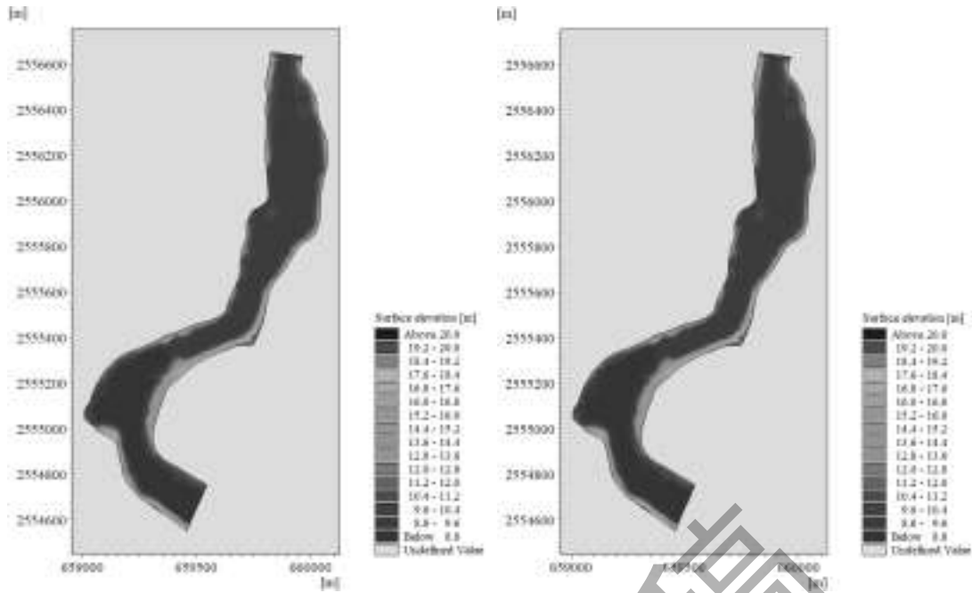
图 5.1.1-7 多年平均 10 月取水前后水位情况图
