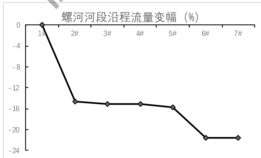
图 5.1.1-16 工程实施前后枯水年来水螺河下游主要河段的流量沿程变化图
