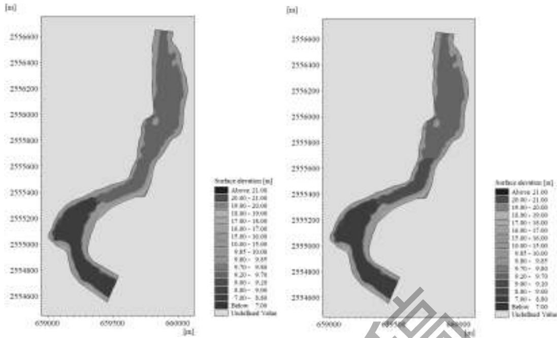
图 5.1.1-4 90%枯水年9月取水前后水位情况图
