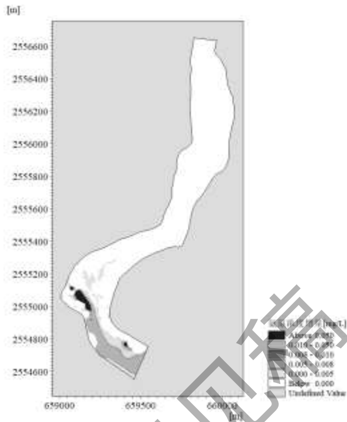
图 5.1.1-13 取水前后氮浓度增量示意图
