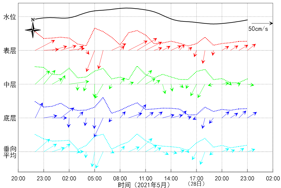
图 3.1.2.2-5 海流矢量时间变化序列图 (SW2-5 站)
