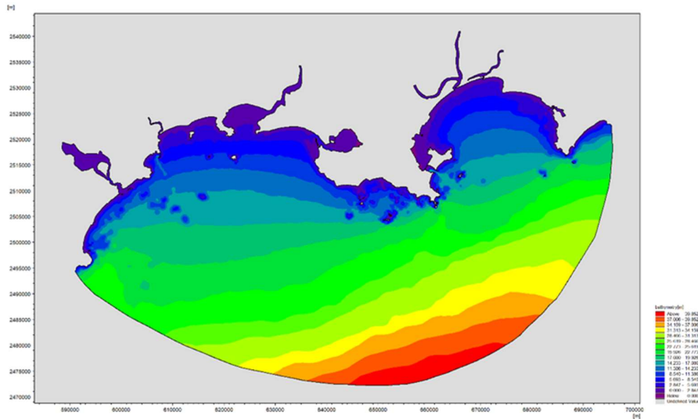
图 4.1.1.1-1 模型计算范围及网格地形
