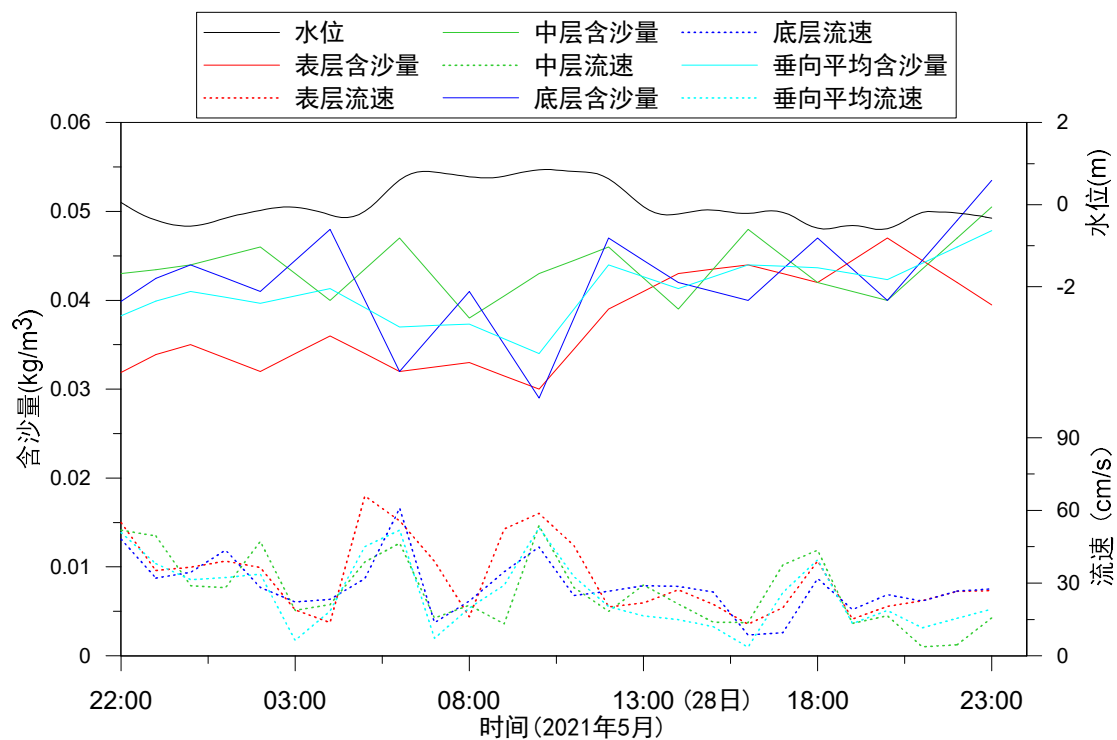
图 3.1.2.4-5 SW2-5 测站潮位与含沙量变化过程图
