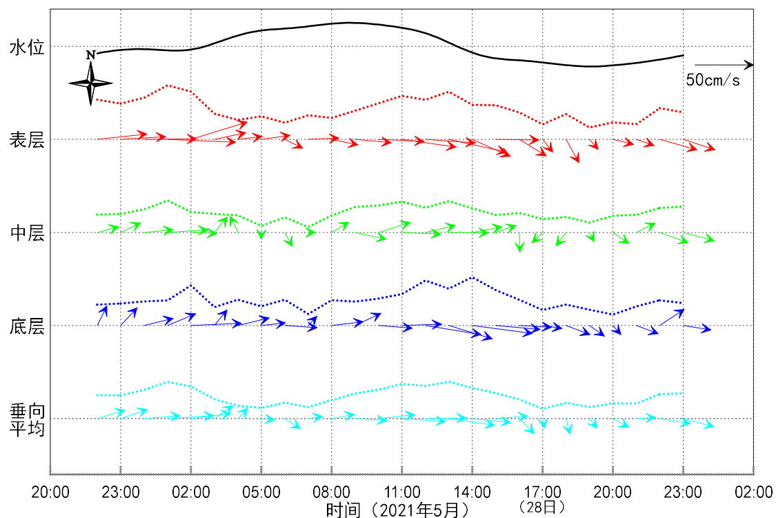
图 3.1.2.2-6 海流矢量时间变化序列图 (SW2-6 站)
