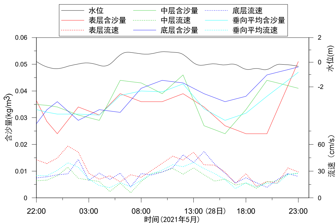
图 3.1.2.4-6 SW2-6 测站潮位与含沙量变化过程图
