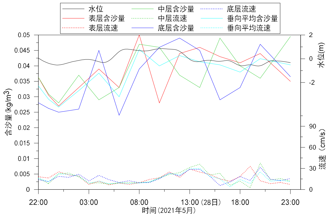
图 3.1.2.4-3 SW2-3 测站潮位与含沙量变化过程图
