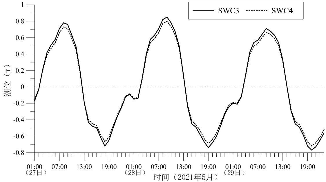
图 3.1.2.1-2 2021 年 5 月 27~29 日调查站位实测潮位变化
