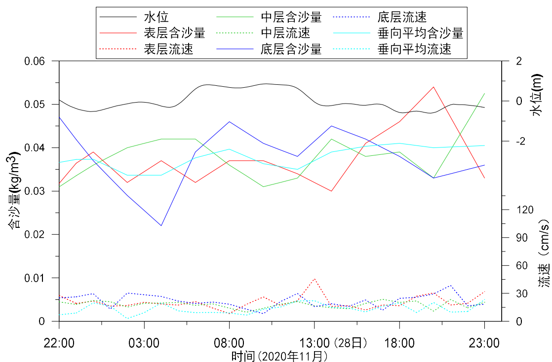
图 3.1.2.4-2 SW2-2 测站潮位与含沙量变化过程图
