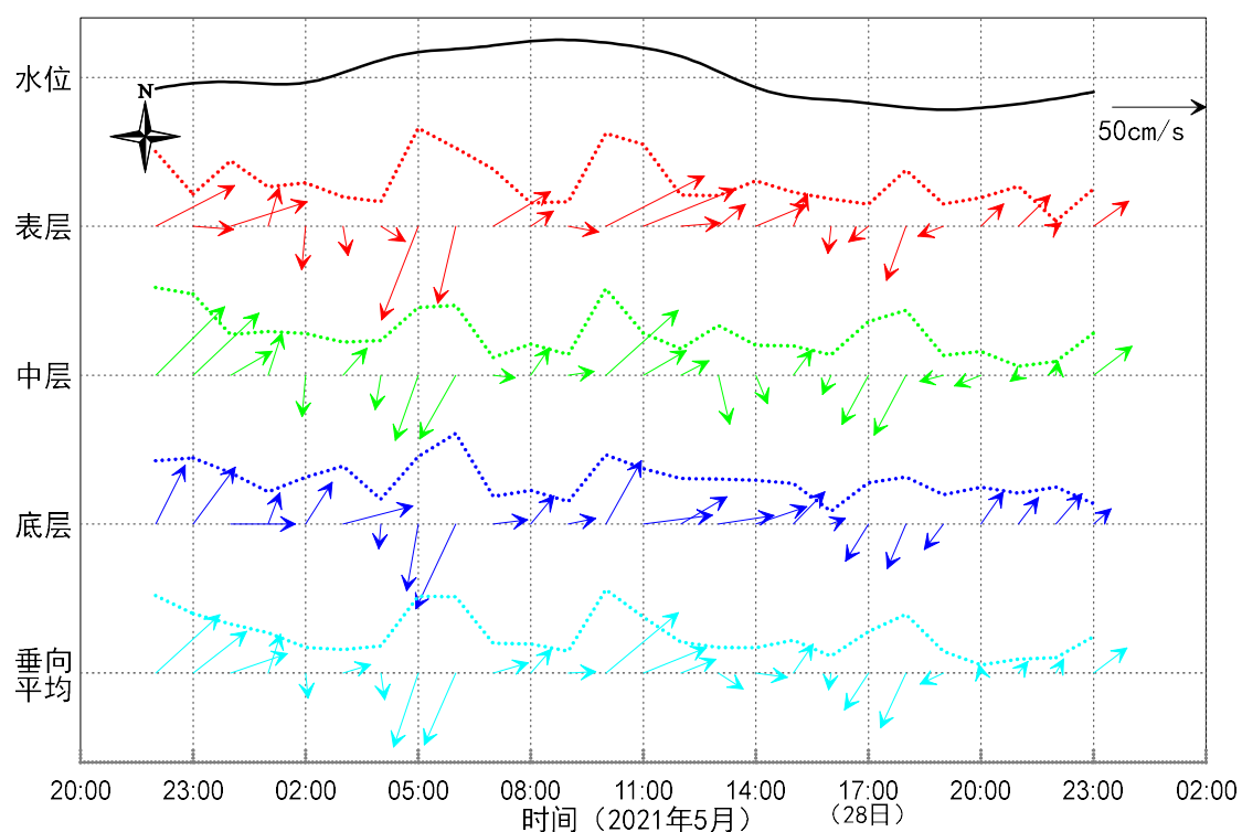
图 3.1.2.2-4 海流矢量时间变化序列图 (SW2-4 站)
