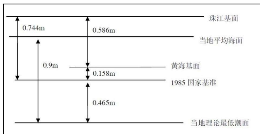
图 3.1.2.1-1 汕尾站基面关系图 (单位: m)
