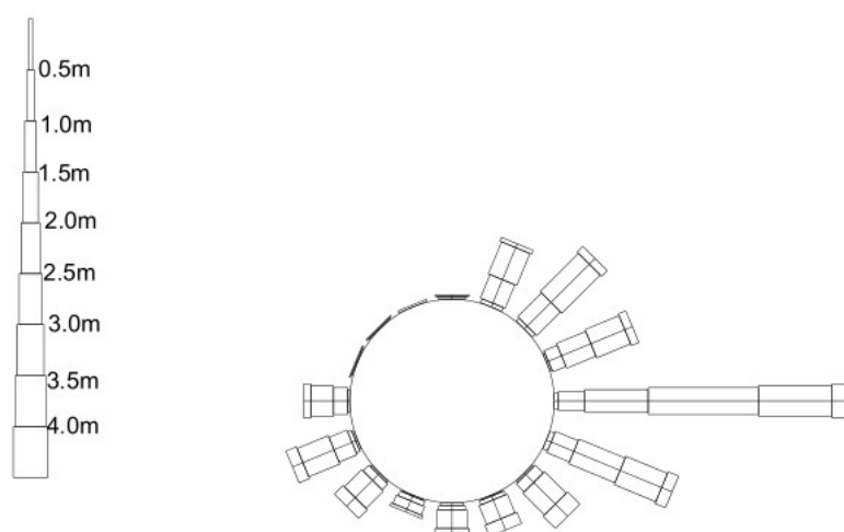
图 3.1.2.3-2 遮浪站年 H1/10 波高玫瑰图
