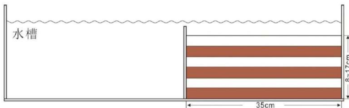
图 4.1.3.3-1 采砂深度分析实验模型设置
