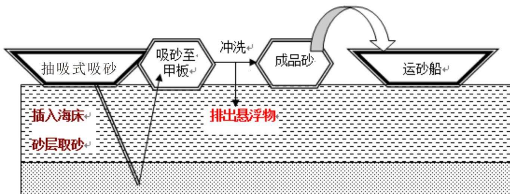
图 2.3.1-1 海砂开采作业流程示意图
