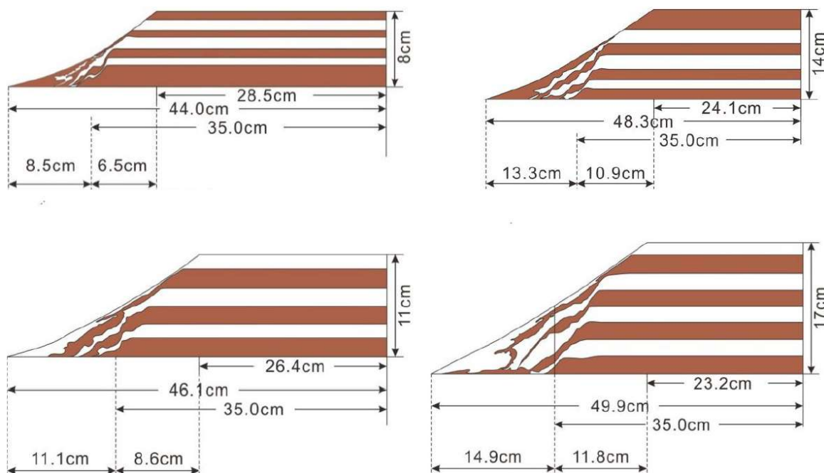
图 4.1.3.3-3 采砂深度分析实验数据示意图
