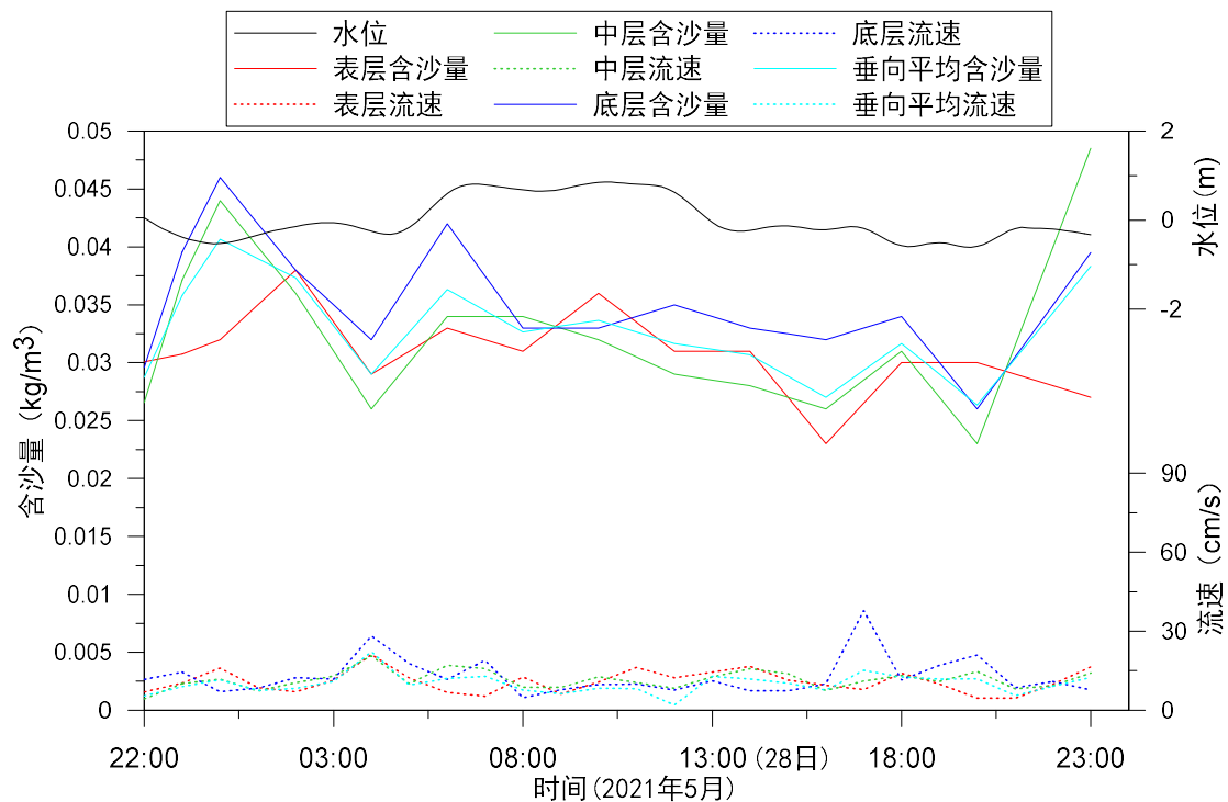
图 3.1.2.4-1 SW2-1 测站潮位与含沙量变化过程图
