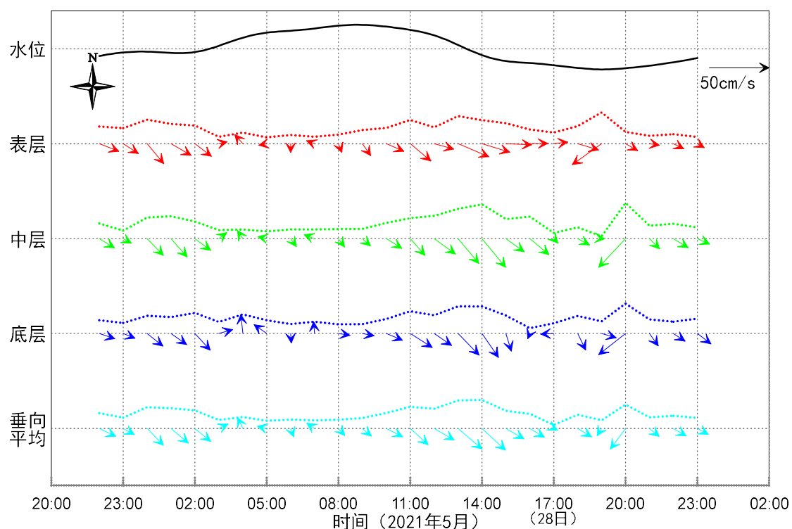
图 3.1.2.2-3 海流矢量时间变化序列图 (SW2-3 站)
