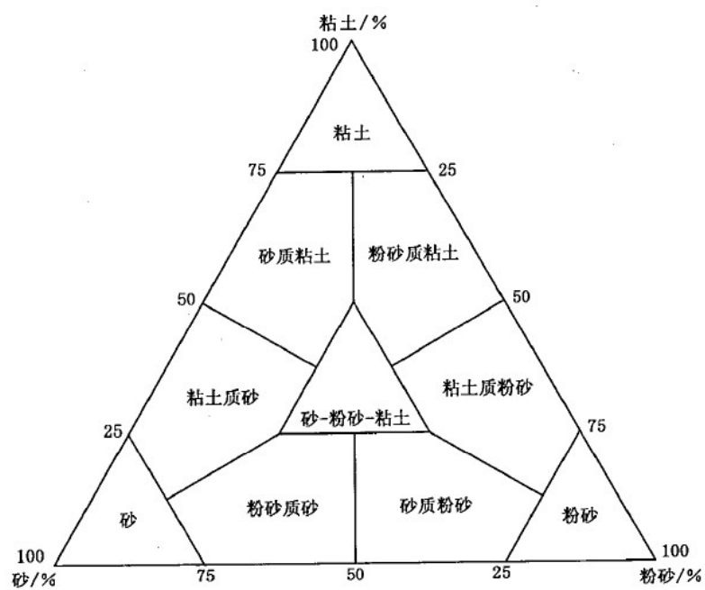
图 3.1.2.4-9 沉积物粒度三角图分类
