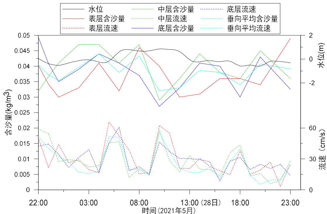
图 3.1.2.4-4 SW2-4 测站潮位与含沙量变化过程图
