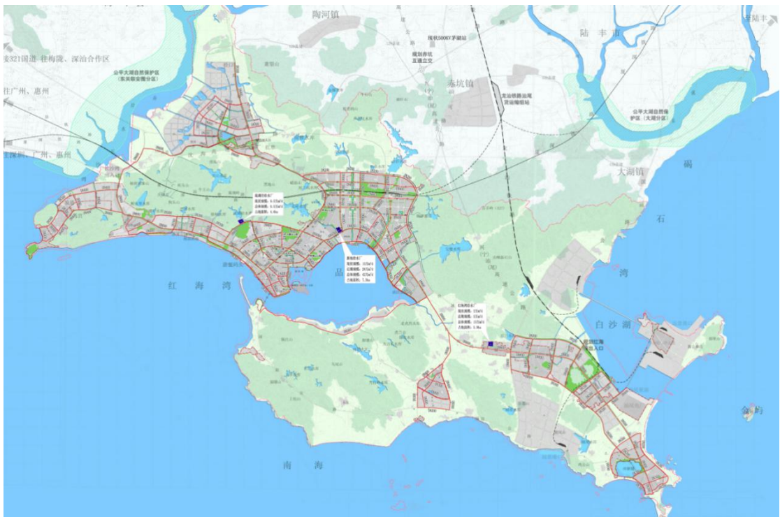
图 6.2-1 汕尾市城市供水管网规划图
