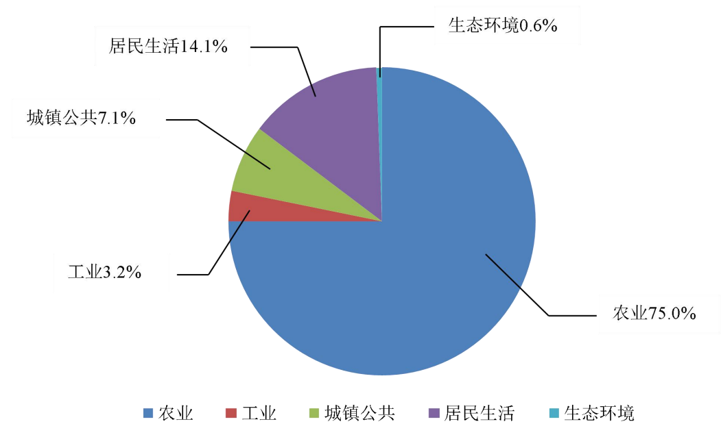
图 1.3-5 2019 年汕尾市耗水量结构图
