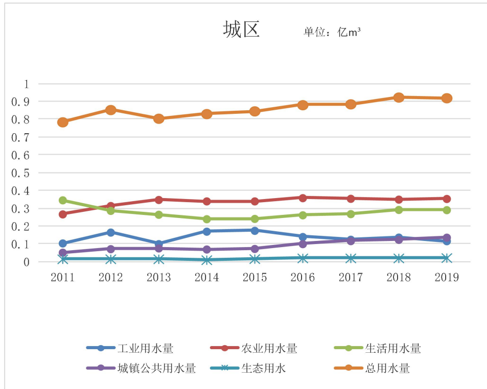
图 1.4-2 2011~2019 年城区各类用水量变化趋势图
