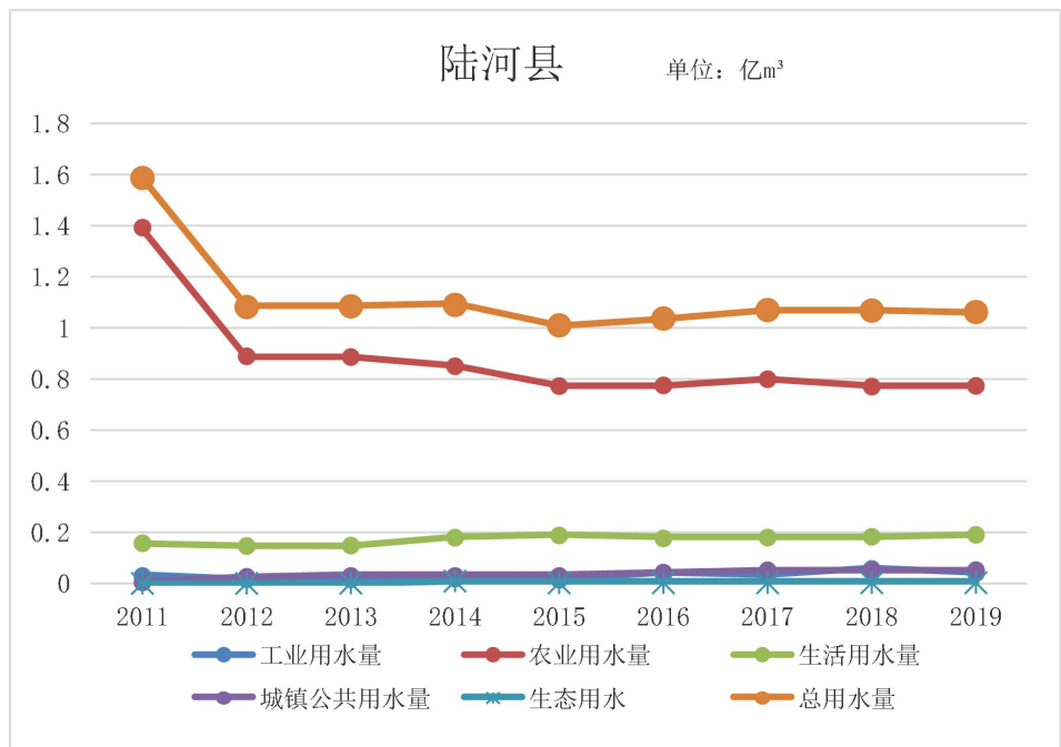
图 1.4-5 2011~2019 年陆河县各类用水量变化趋势图
