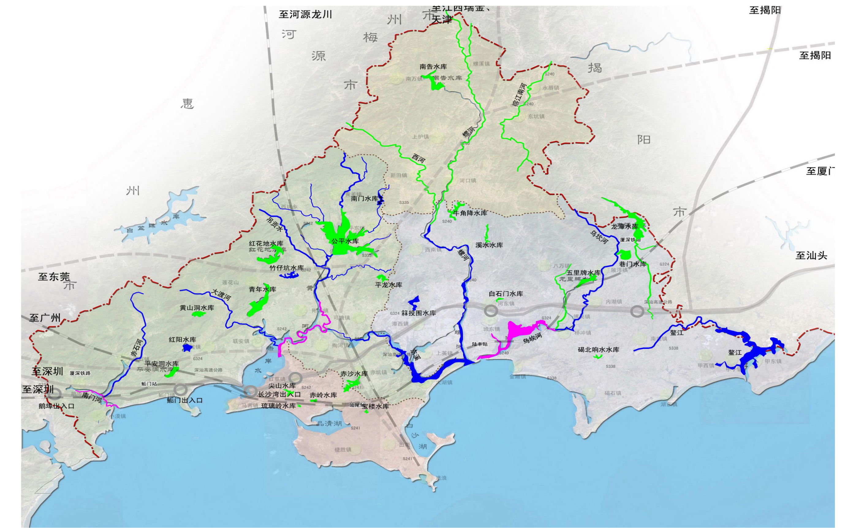
附图 2 汕尾市水功能区划示意图
