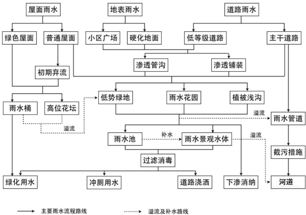
图 5.7-1 雨水利用流程图
